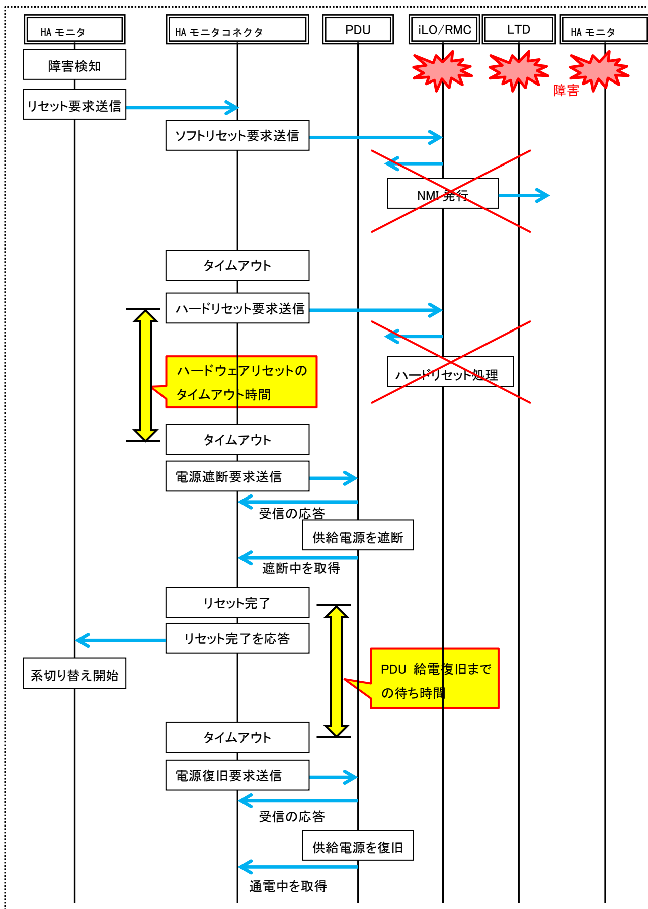
PDU からの給電遮断による系切り替えのフロー
