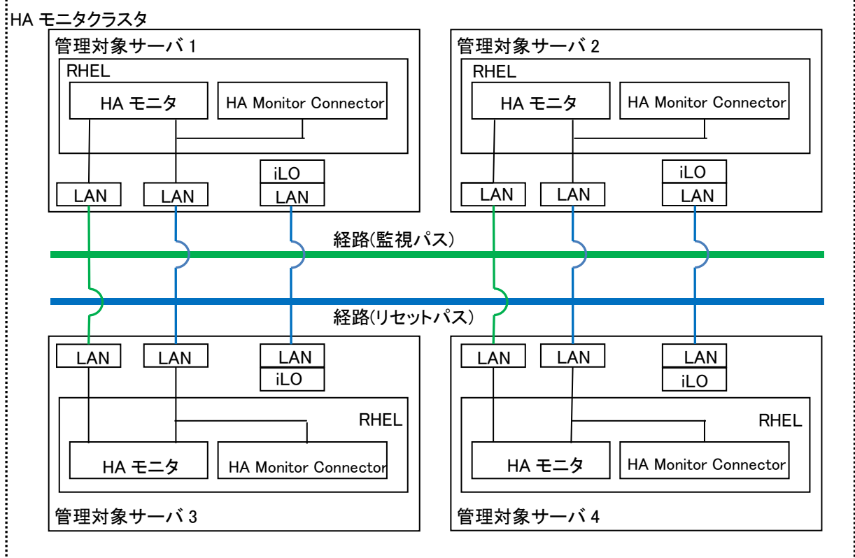
図 5-1 前提 HA モニタクラスタ構成(物理サーバ)
