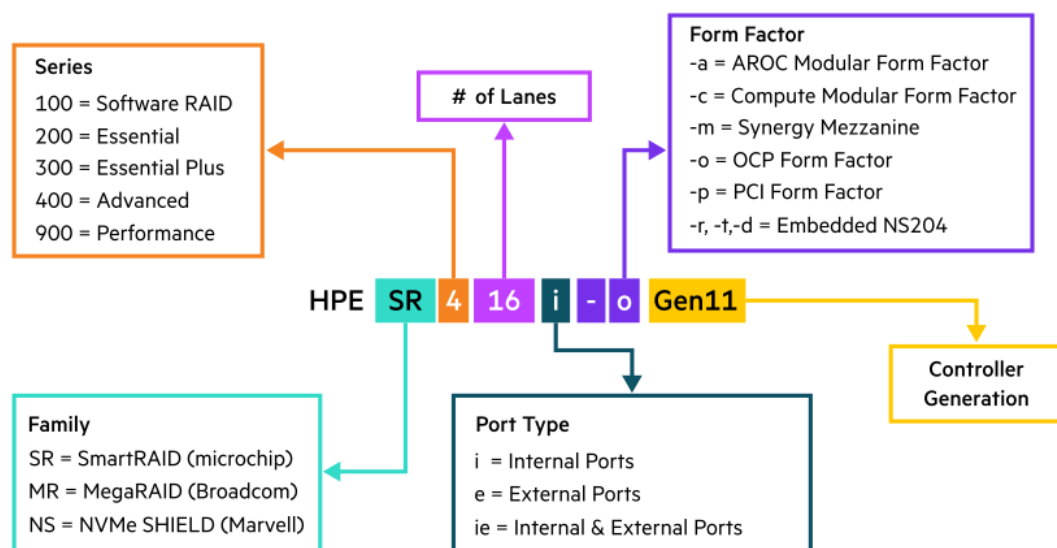
図 1. HPE Gen11ストレージコントローラーの命名フレームワーク
