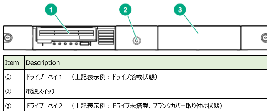
テープエンクロージャ4 フロントパネル
