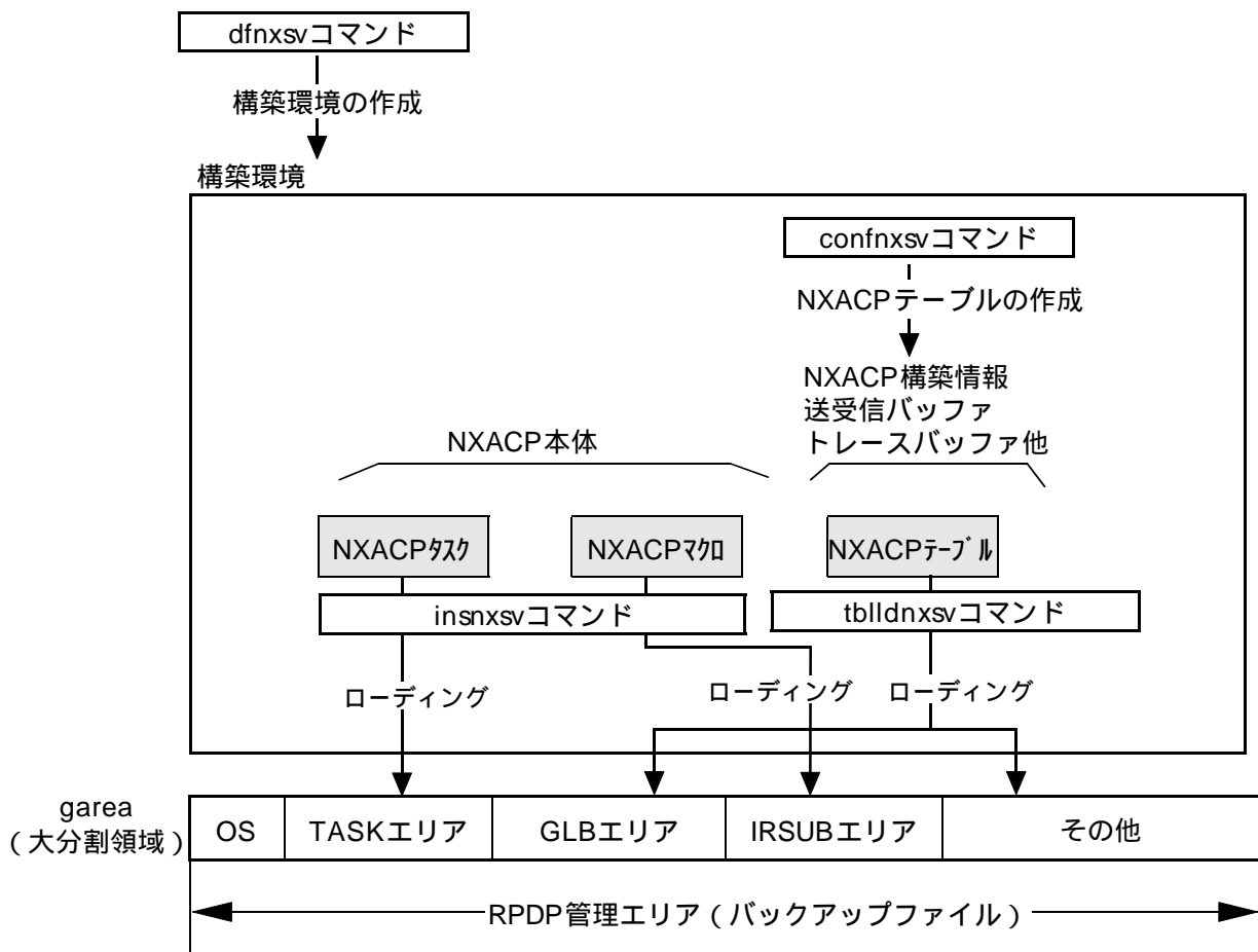
図 2 - 67 リソースの配置
