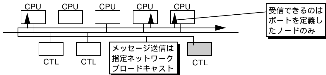
図 2 - 10 マルチキャストと選択受信
