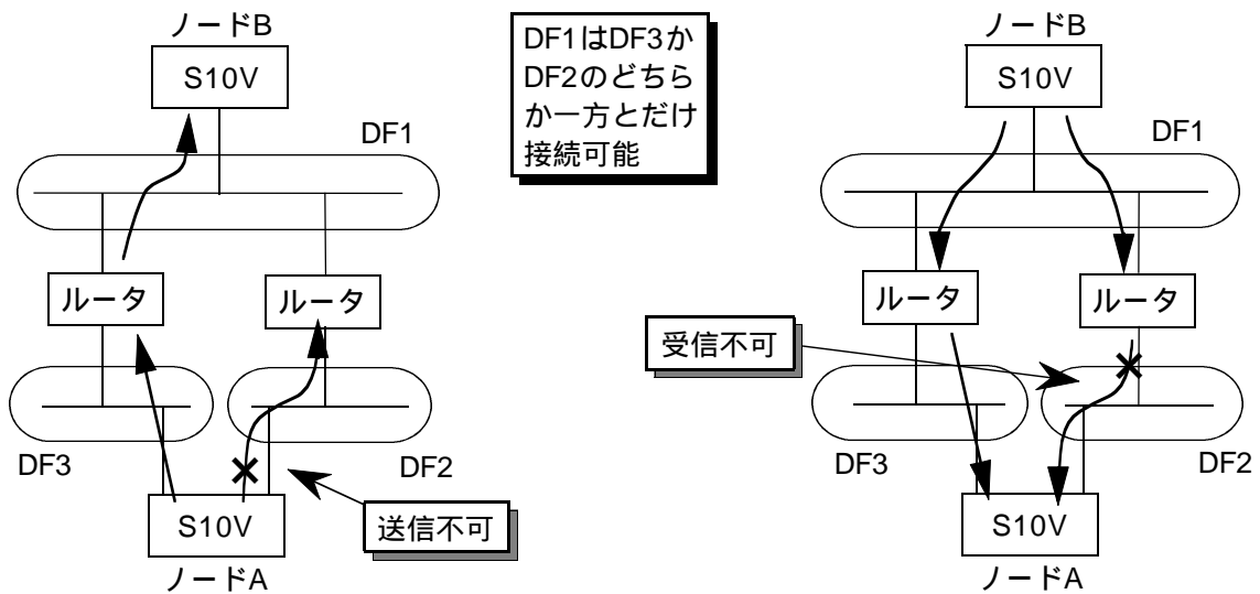
図2-25 リモートデータフィールド(2)
