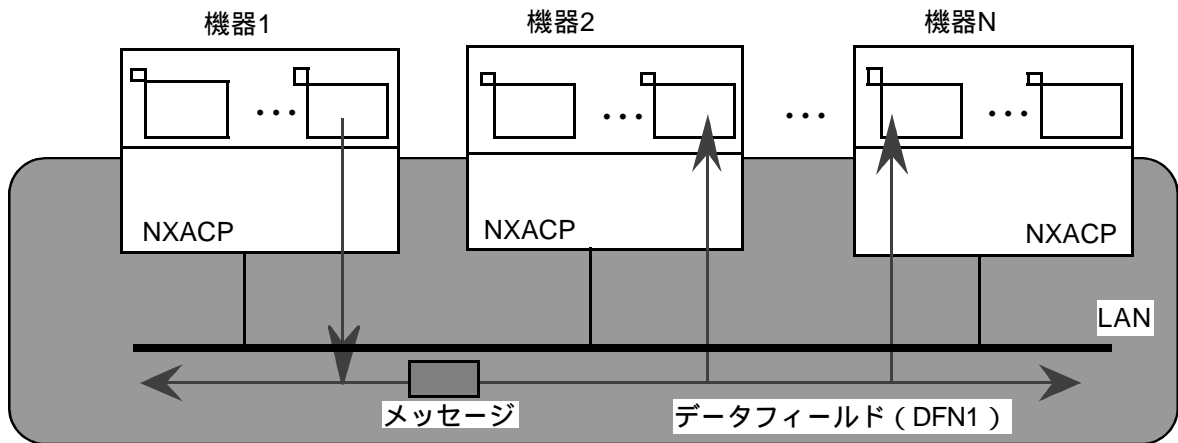
図1 - 5 データフィールド
