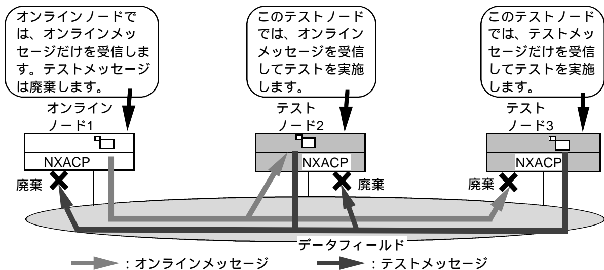
図1 - 23 テスト機能
