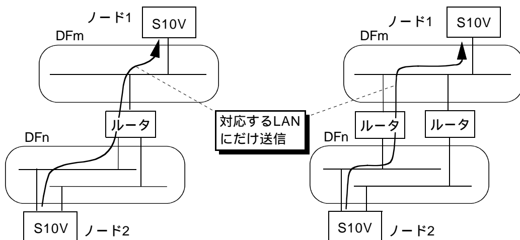
図2 - 35 二重化LANとリモートデータフィールド (4)
