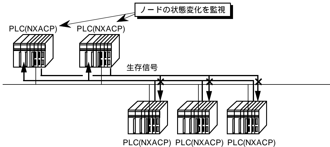
図1 - 20 状態監視ノード（2）
