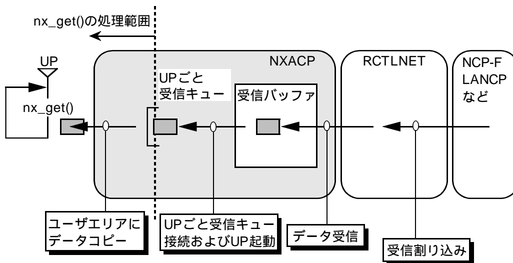
図2 - 4 nx_get マクロ
