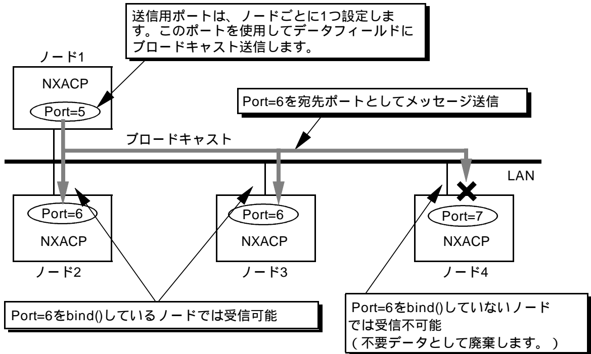
図1 - 11 ポート
