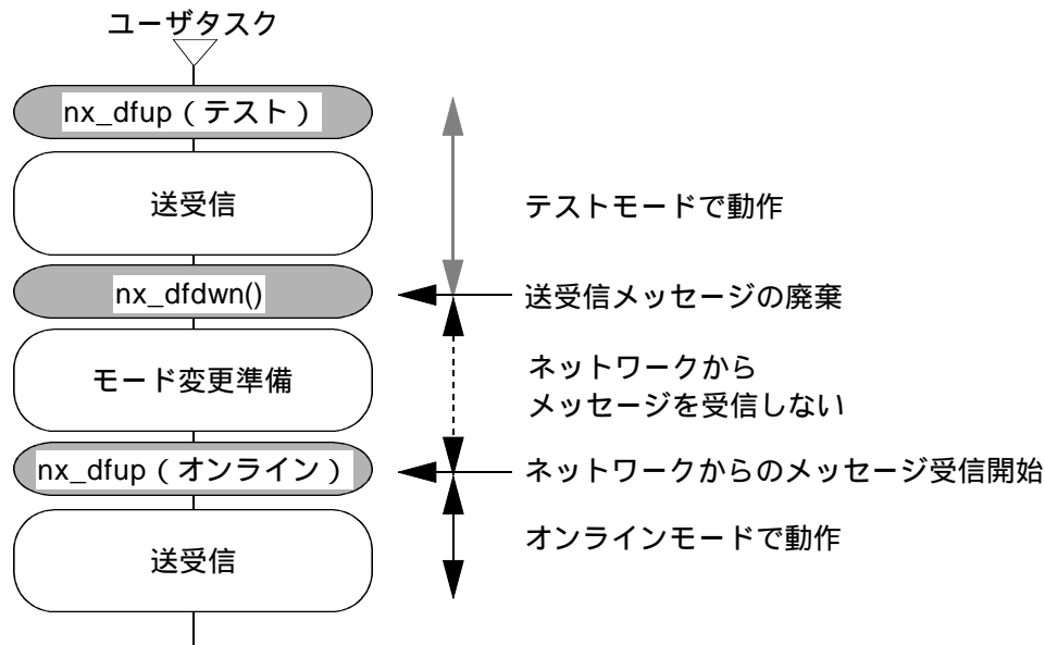
図2-54 モード変更手順
