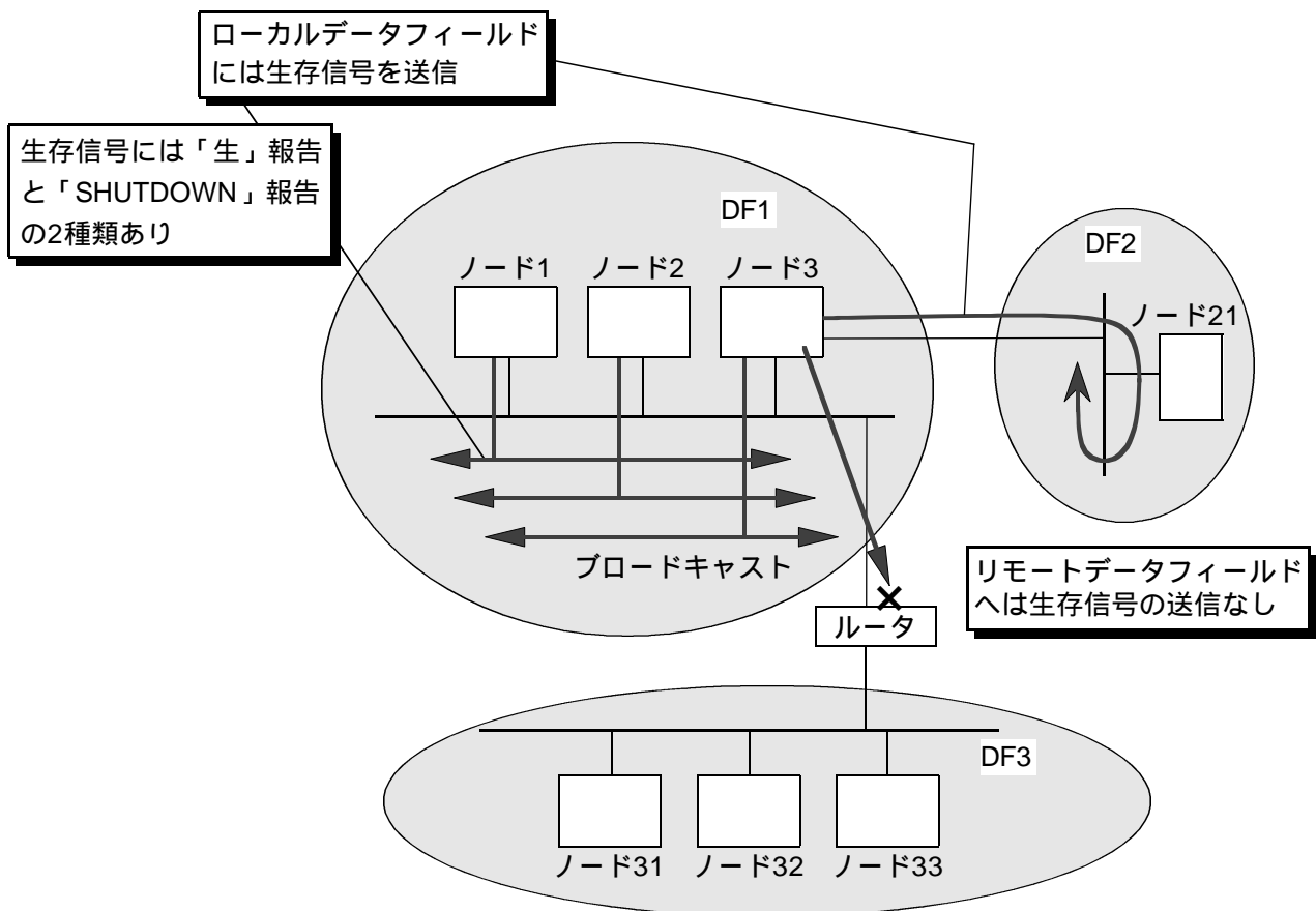
図2 - 27 生存信号
