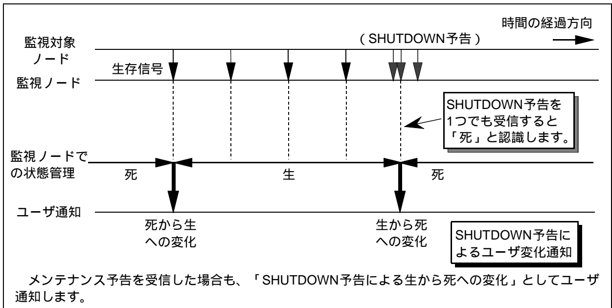
図2 - 30 変化通知のタイムシーケンス (SHUTDOWN予告)
