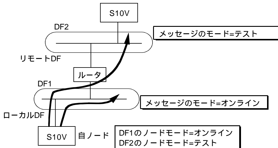
図2 - 41 リモートデータフィールドとモード (1)
