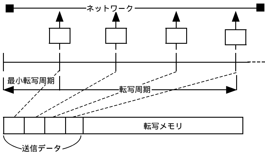
図2 - 64 分割送信型ソフト転写
