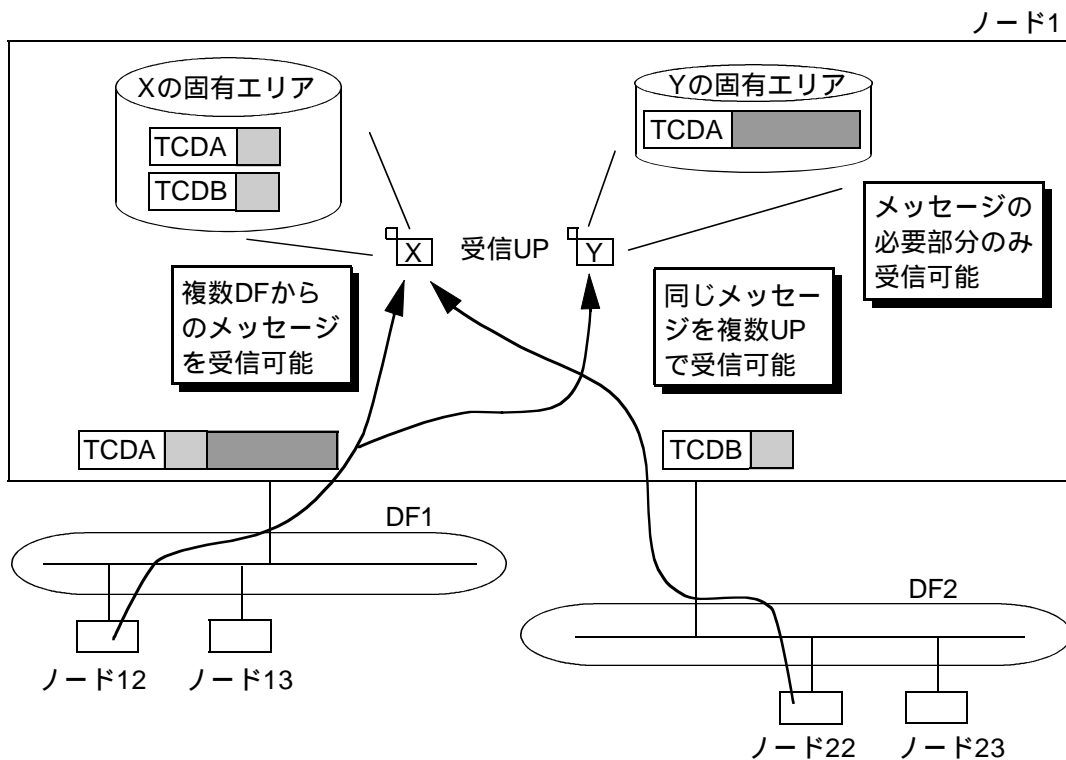
図2 - 17 nx_get() の特長
