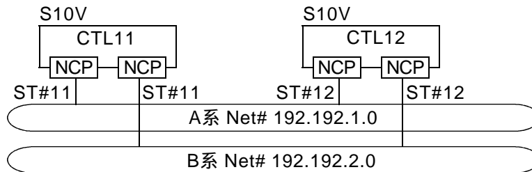
図2 - 70 二重化ネットワーク構成
