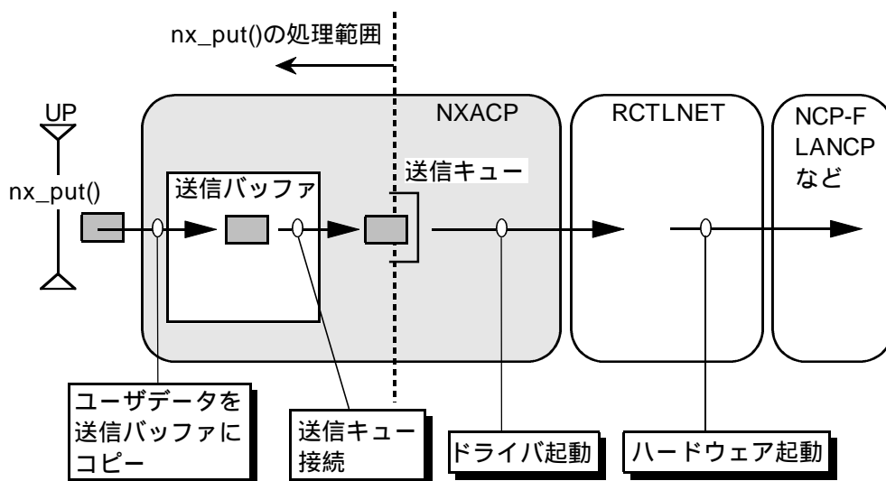
図2 - 2 nx_putマクロ
