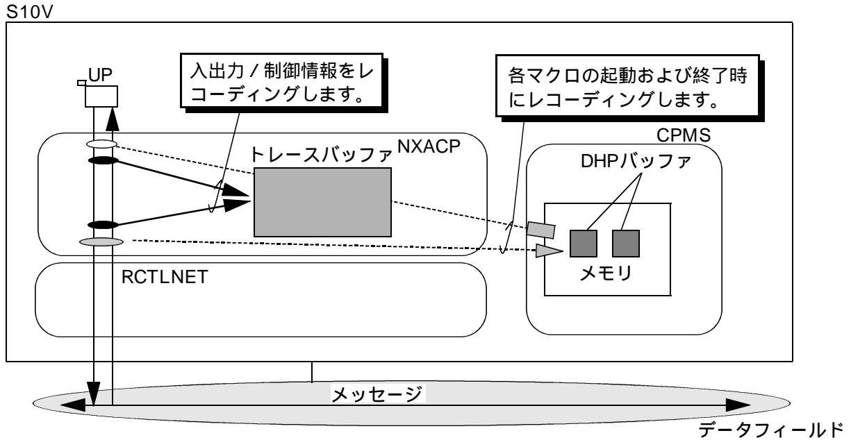
図1 - 25 トレース
