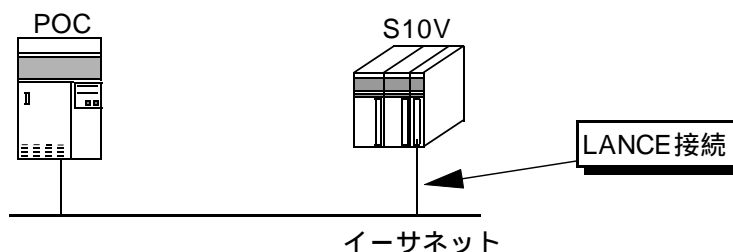
図1-1 ネットワーク最小構成
