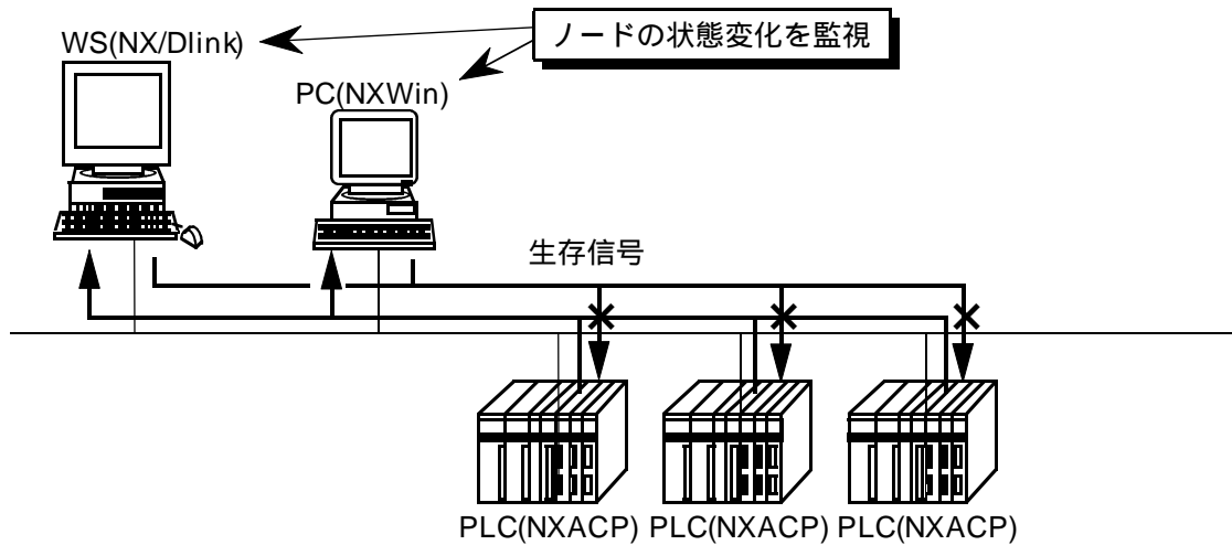
図1 - 19 状態監視ノード（1）
