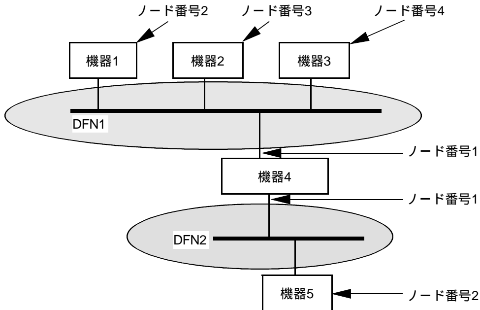
図1 - 9 論理ノード
