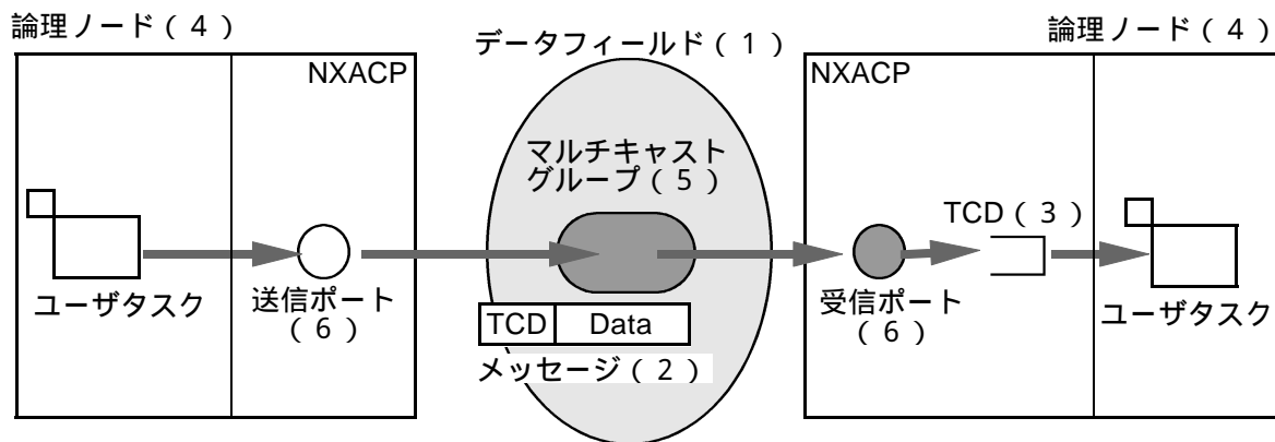
図1-4 NXACP要素の説明
