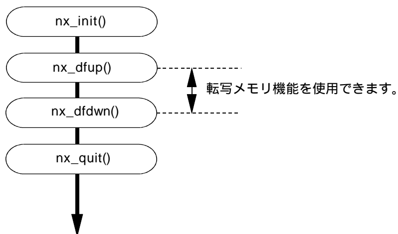
図2 - 66 転写メモリとデータフィールド状態
