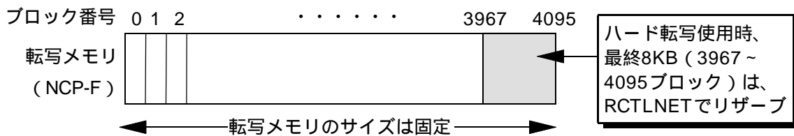
図2 - 56 ハード転写メモリ
