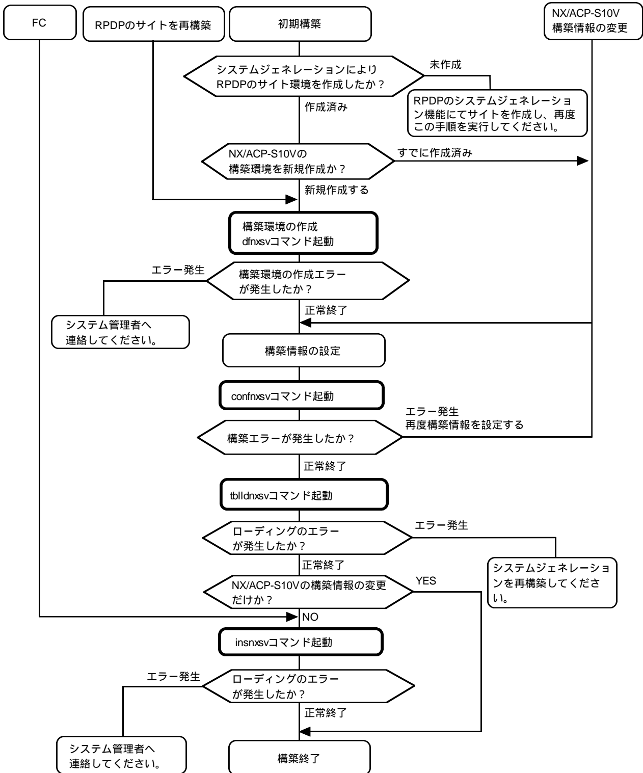
図 2 - 68 NXACPの構築手順
