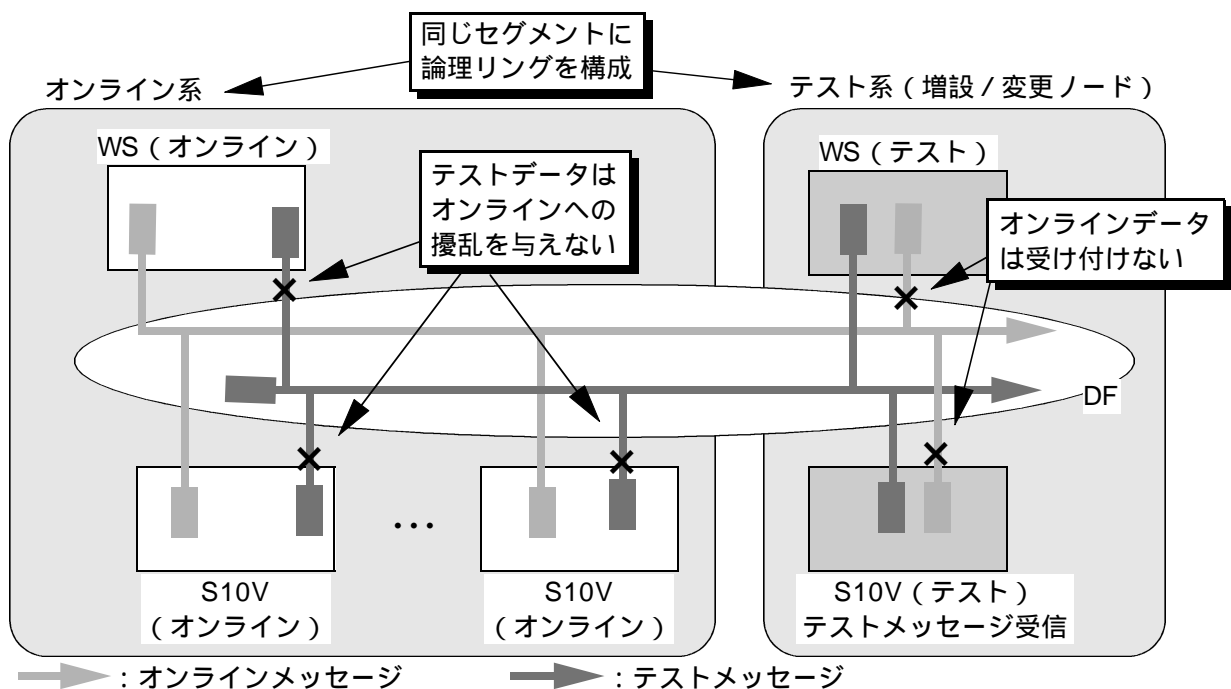
図2 - 39 テスト形態 (2)
