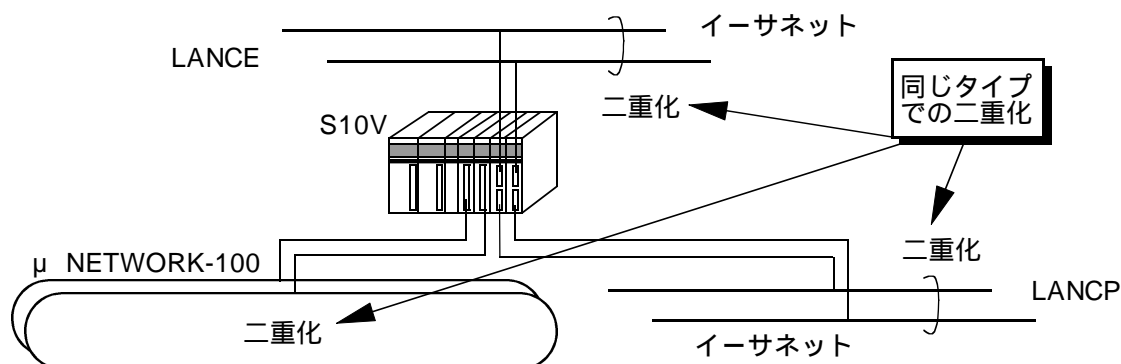
図1-2 ネットワーク最大構成
