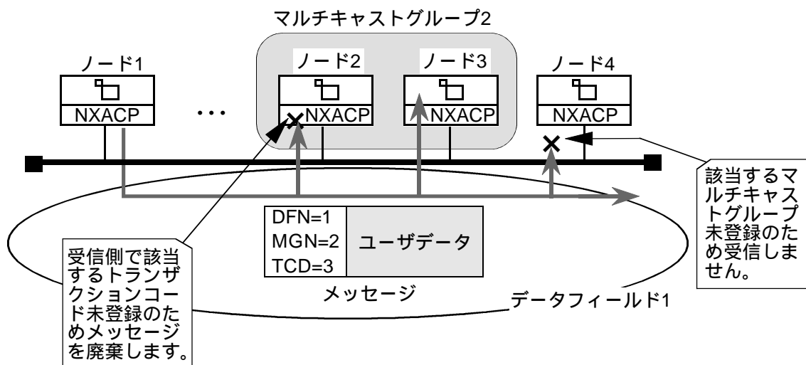
図1-12 マルチキャスト通信
