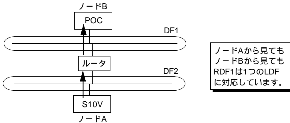
図2-24 リモートデータフィールド(1)
