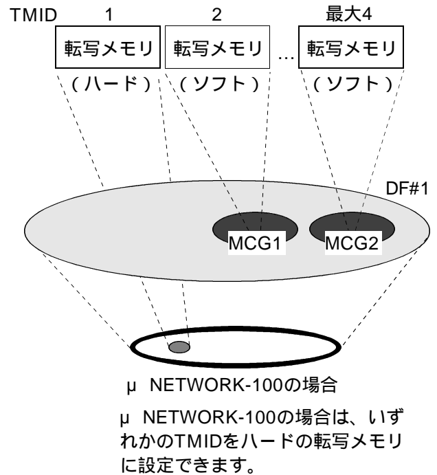
図2 - 60 転写メモリ認識とマルチキャストグループ
