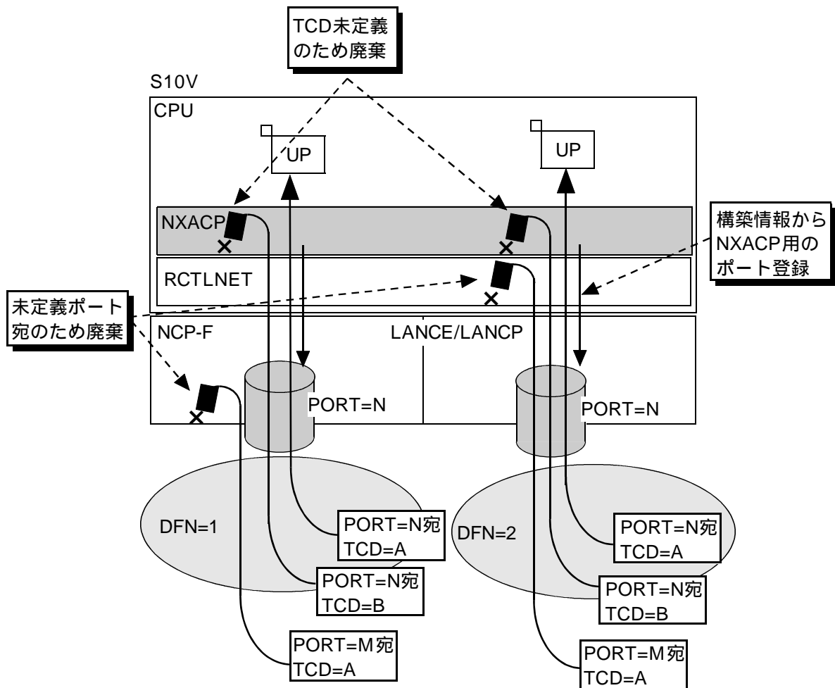
図1 - 16 メッセージのフィルタリング
