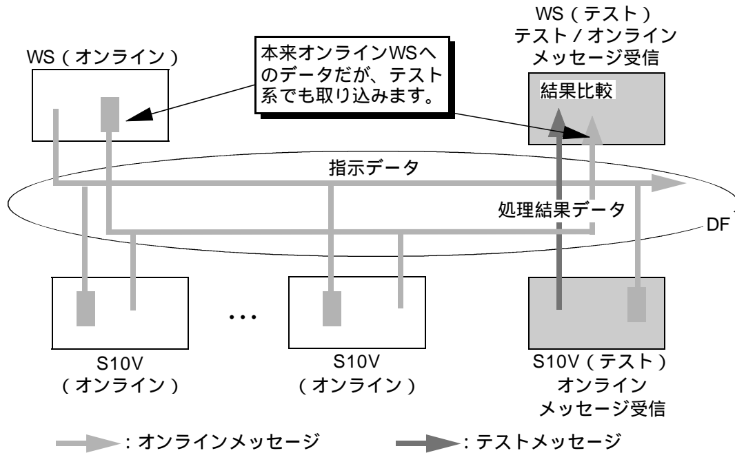
図2 - 40 テスト形態 (3)
