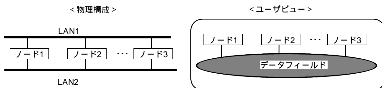
図1-21 LANの二重化
