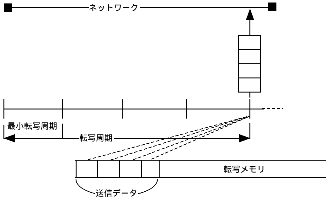
図2 - 63 周期送信型ソフト転写
