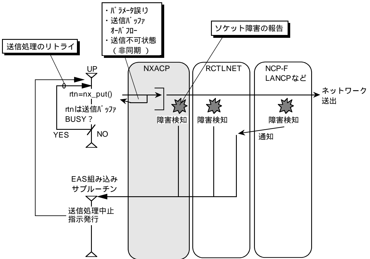
図2-3 障害情報の検知(送信)
