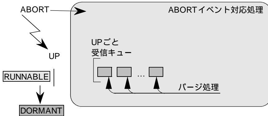
図2 - 47 ABORT後処理
