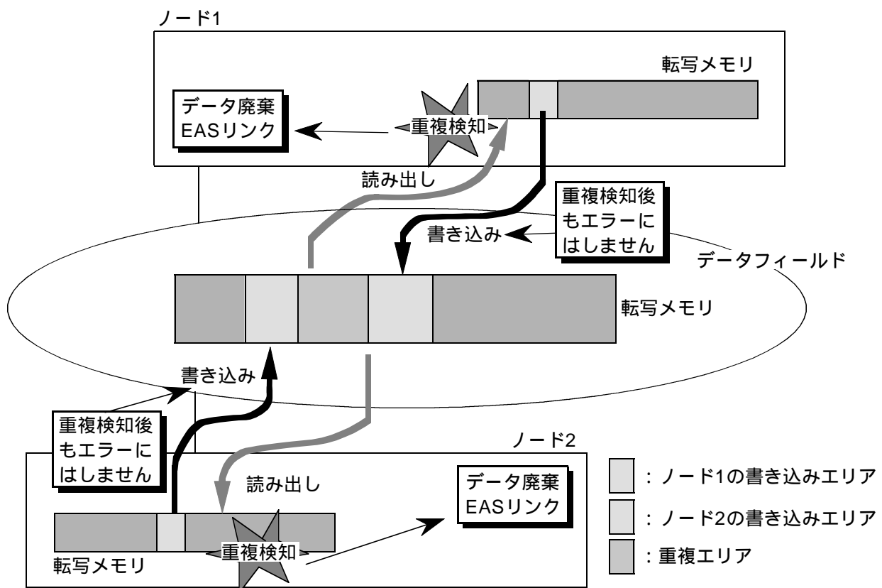
図2 - 62 ソフト転写時の重複チェック
