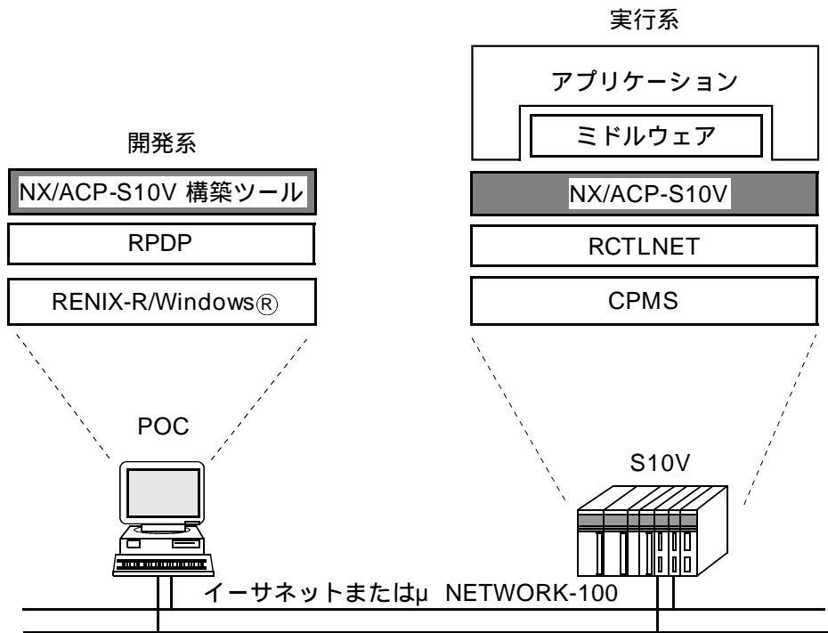
図1-3 ソフトウェア構成
