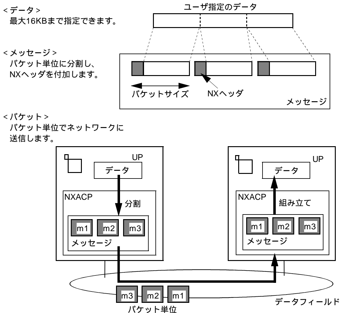
図2 - 1 通信単位
