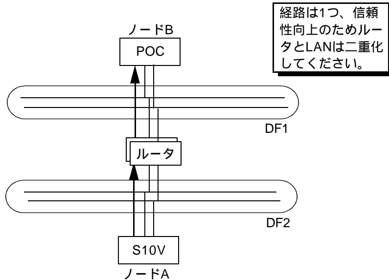
図2 - 13 リモートデータフィールド (3)
