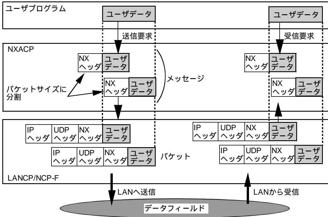
図1 - 7 メッセージ
