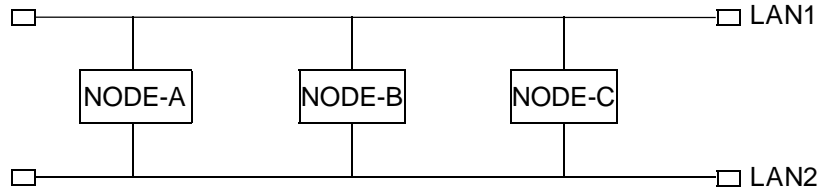
図2 - 44 構成例
