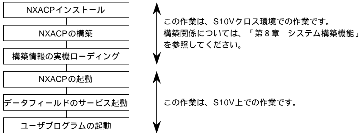
図2 - 48 NXACPの運用
