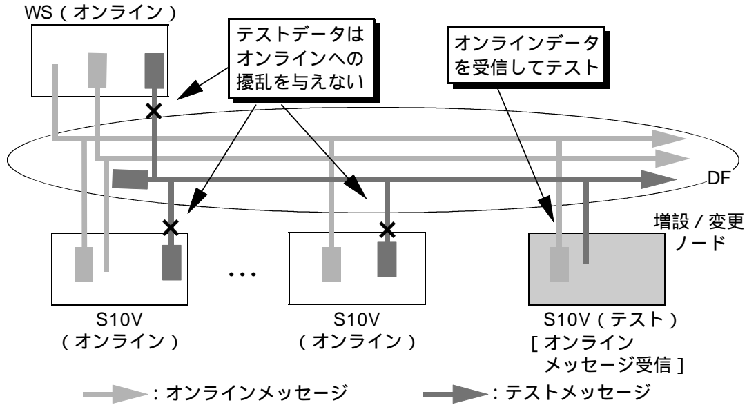
図2 - 38 テスト形態 (1)
