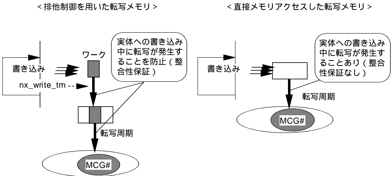
図2 - 61 ソフト転写時の排他制御
