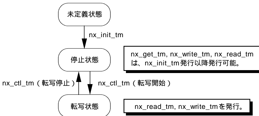
図2 - 65 転写メモリの状態遷移
