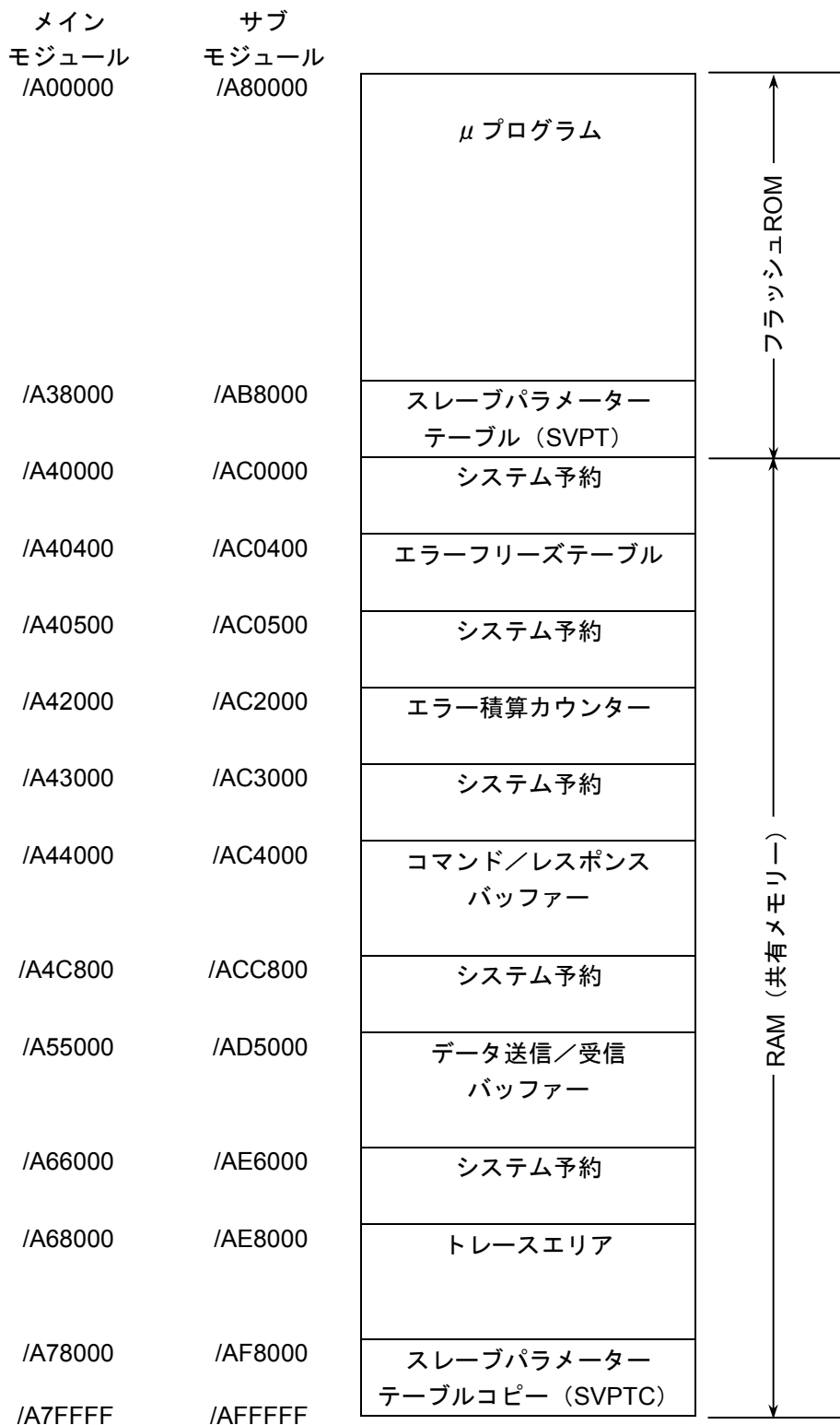
図7-7 J.NET-INTモジュールのメモリーマップ
