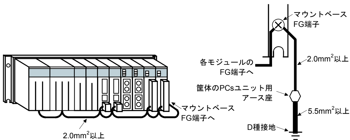
図3-2 アース配線
