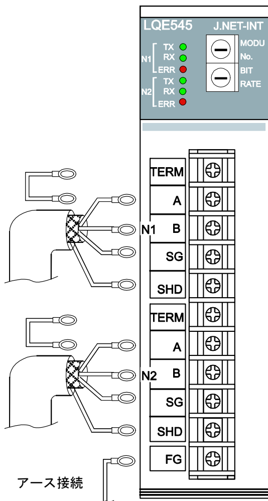
図3-3 モジュールへの配線
