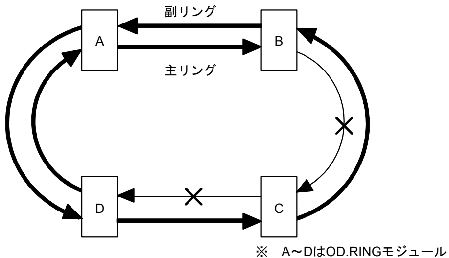
図5-7 片方のリングが複数箇所断線した場合
