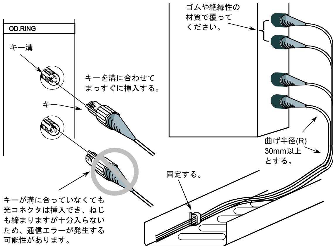
図3-4 光ファイバケーブルの取り扱い
