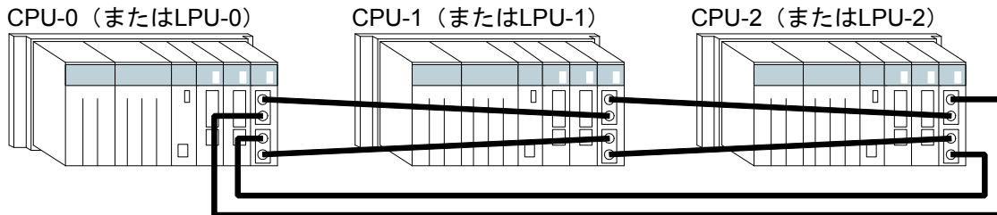
図5-1 システム構成例
