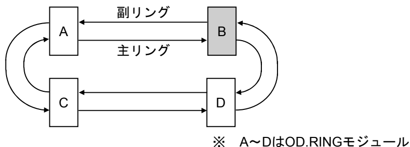
図6-1 システム構成例
