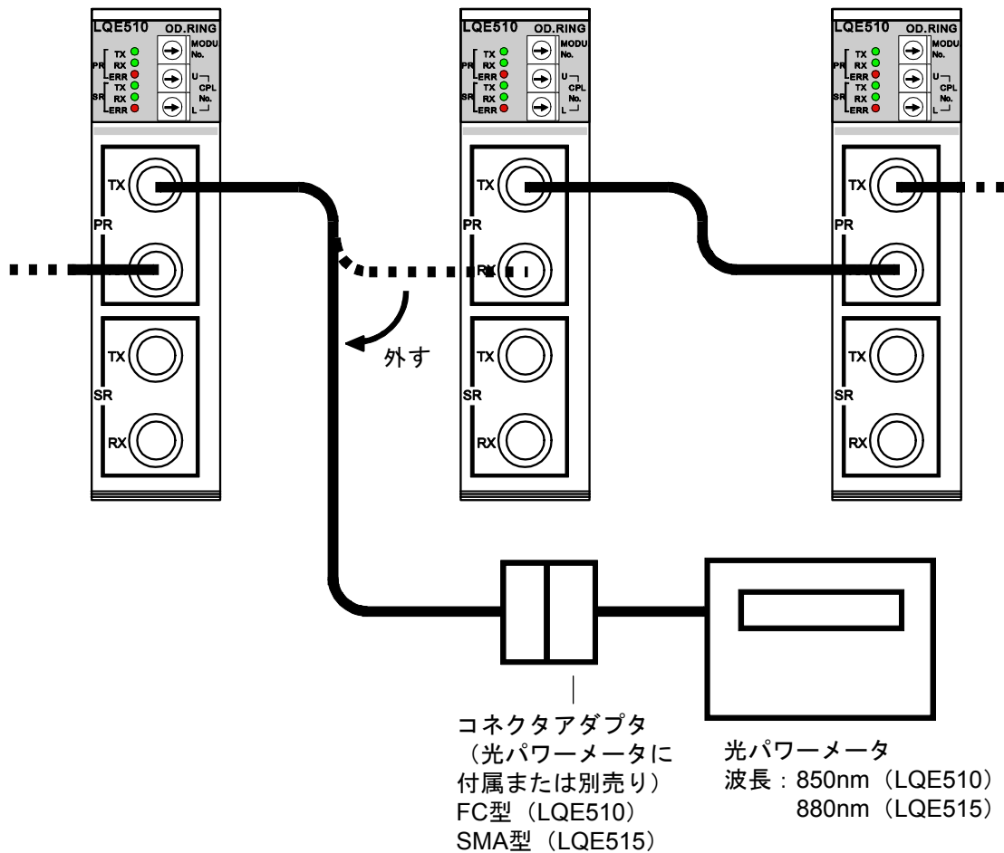
図 6-2 光受信レベルの測定例
