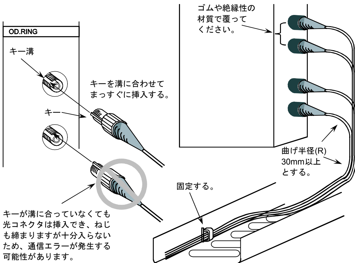
図3-4 光ファイバケーブルの取り扱い
