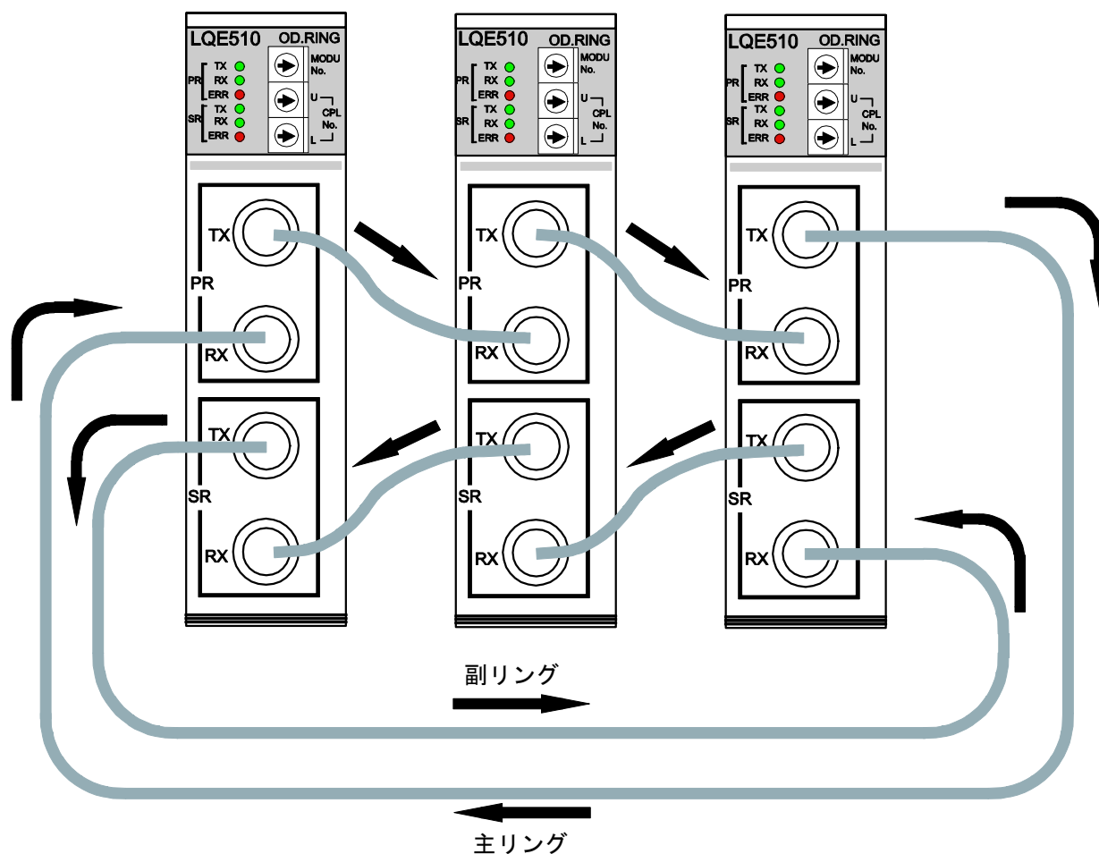
図3-3 光ファイバケーブルの接続
