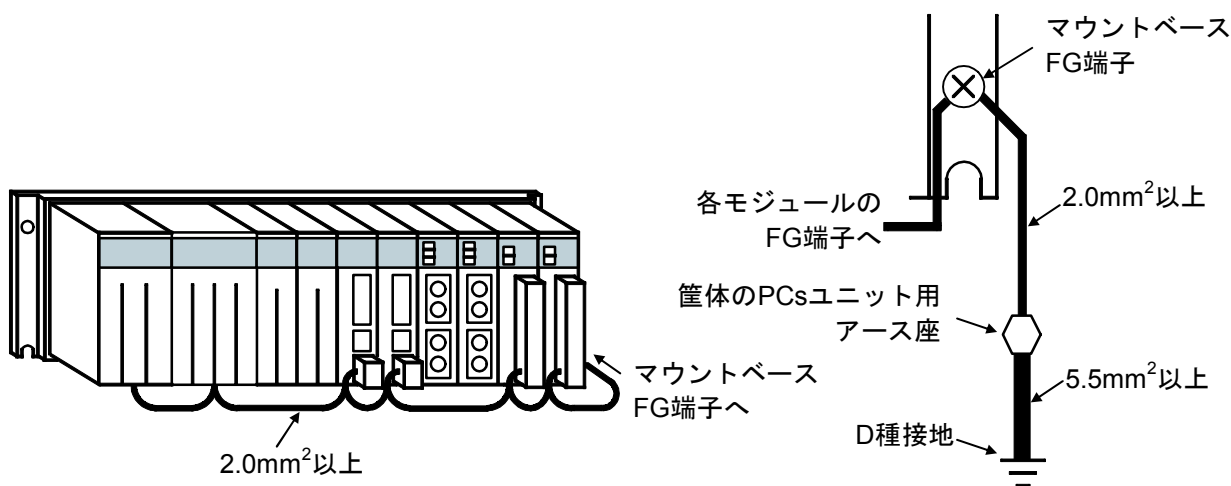
図3-2 アース配線
