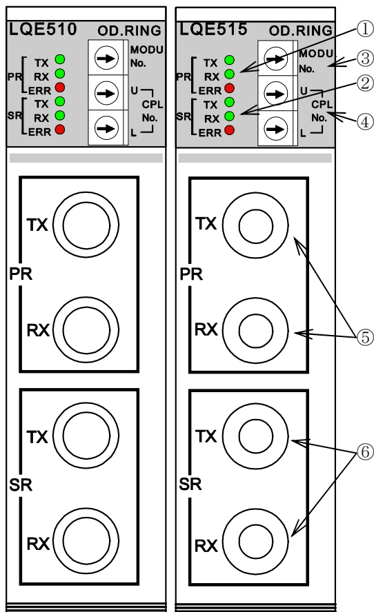
図 2 - 1 OD.RINGモジュール正面
