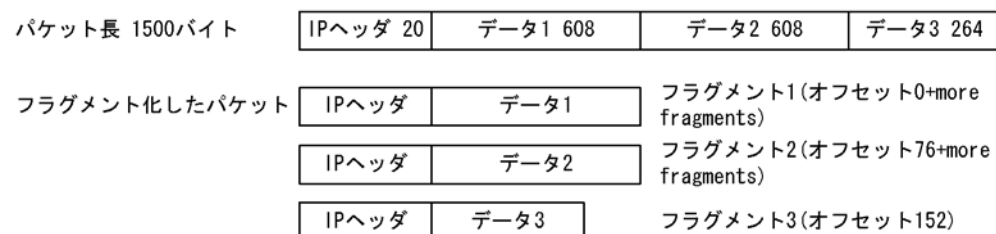
図 1-11 パケットのフラグメント化
