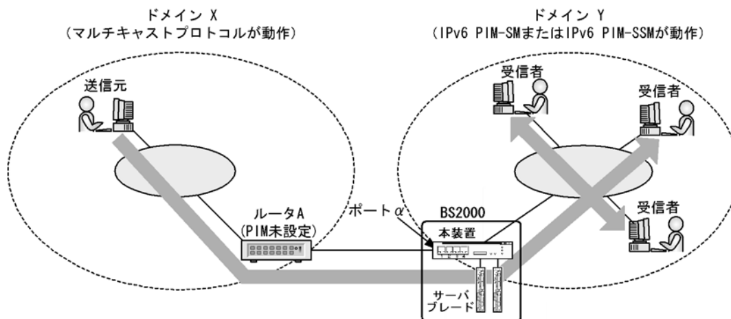
図 27-22 IPv6 上流ポートを指定する場合の適応例
