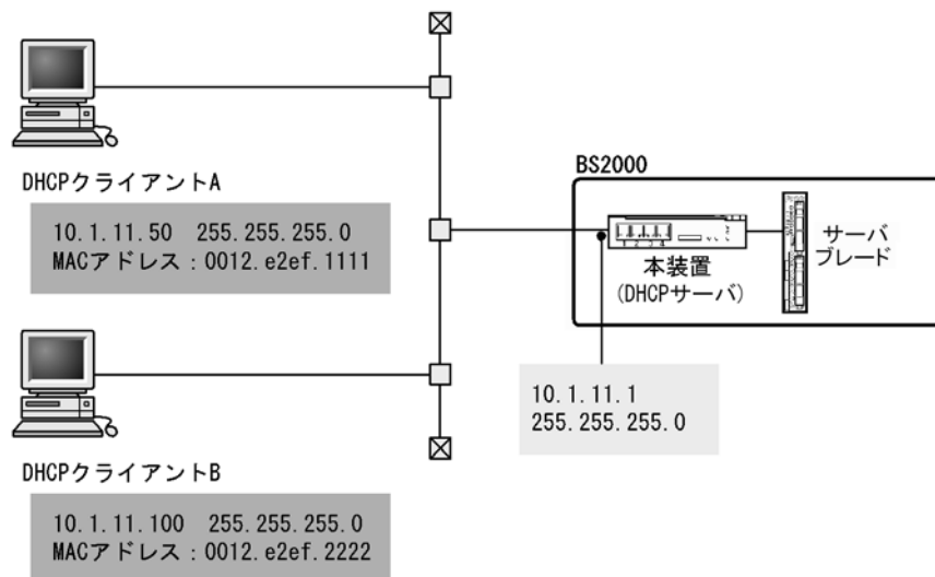
図 5-2 クライアントーサーバ構成（固定 IP アドレス配布時）
