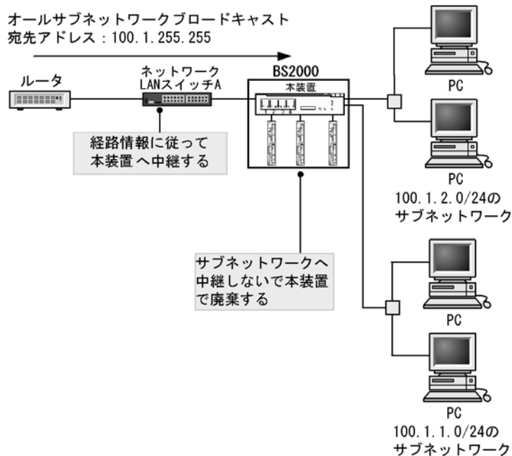
図 1-8 オールサブネットワークブロードキャスト
