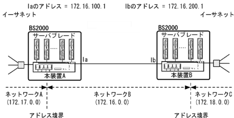
図 6-11 通常のアドレス境界設計例
