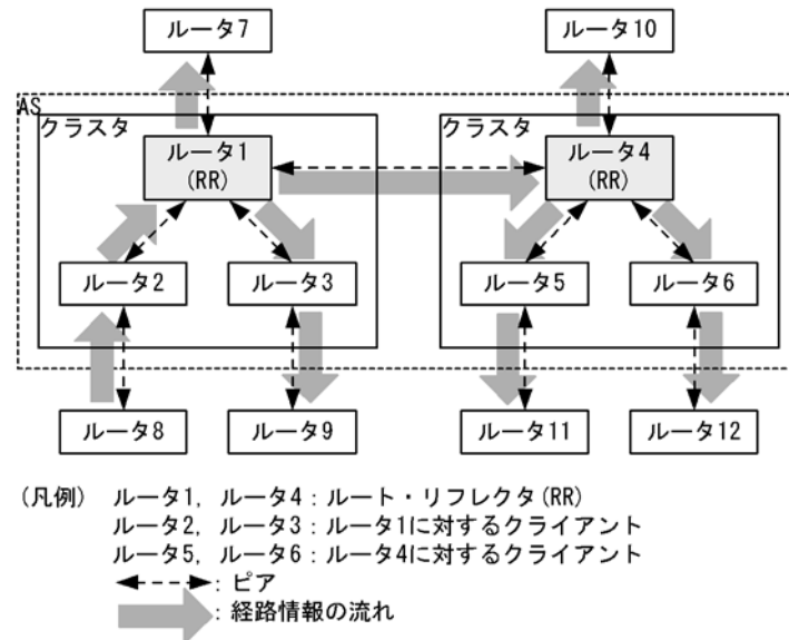
図 11-21 クラスタ内に一つのルート・リフレクタを置く例
