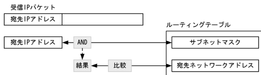
図 1-3 ルーティングテーブルの検索
