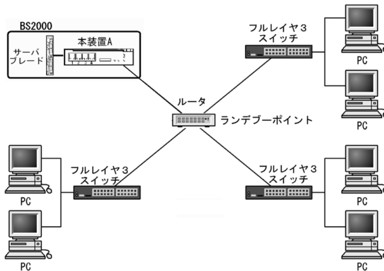
図 13-20 PIM-SM を使用する構成図
