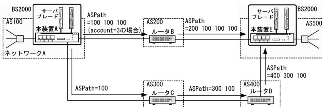
図 11-4 set as-path prepend count コマンドの使用例
