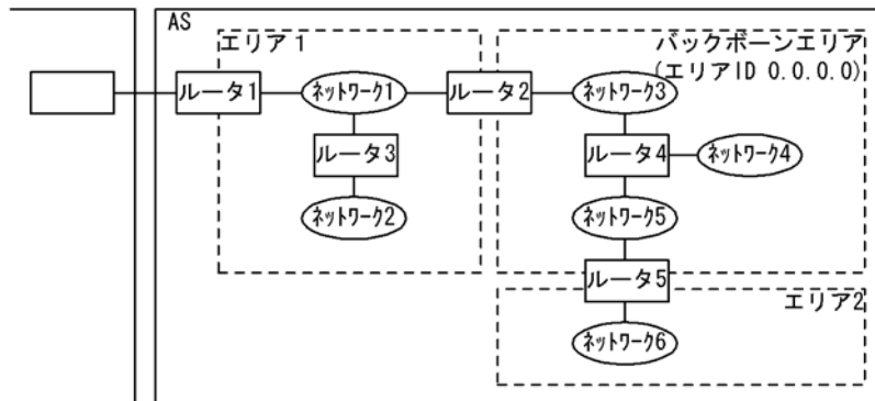
図 24-1 エリア分割を使用した OSPFv3 ネットワークトポロジの例
