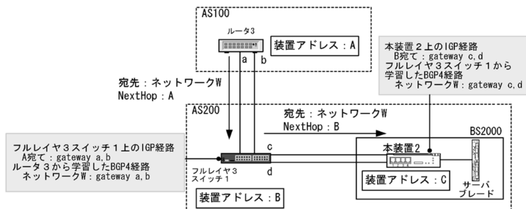
図 11-15 IGP 経路のマルチパス化による BGP4 経路マルチパス化の概念
