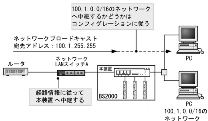
図 1-6 ネットワークブロードキャスト
