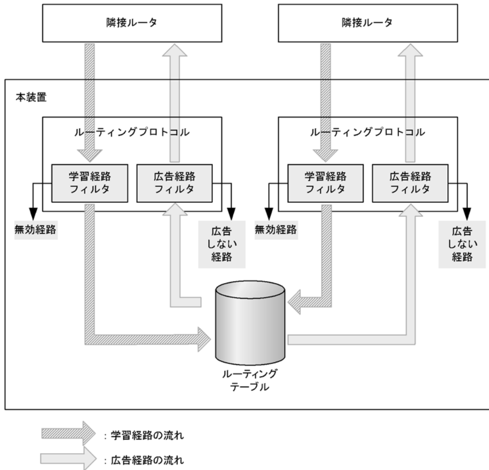
図 26-1 経路フィルタリングの概念図
