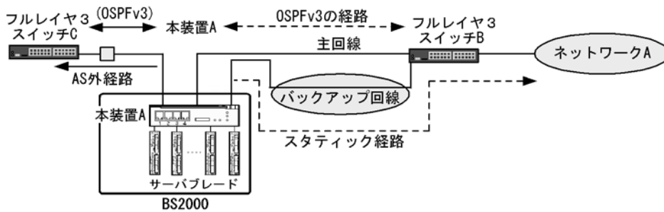
図 23-4 バックアップ回線を使用した構成での AS 外経路の導入例
