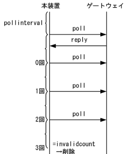
図 7-4 スタティック経路の動的監視による経路削除 (invalidcount=3 の場合)
