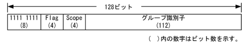
図 15-15 IPv6 マルチキャストアドレス
