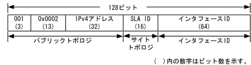
図 15-14 6to4 アドレス
