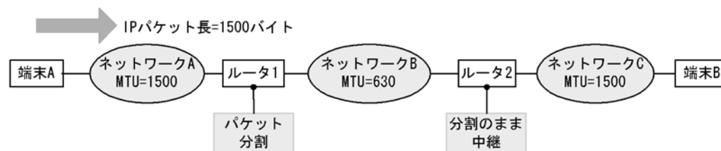
図 1-10 フラグメント化モデル
