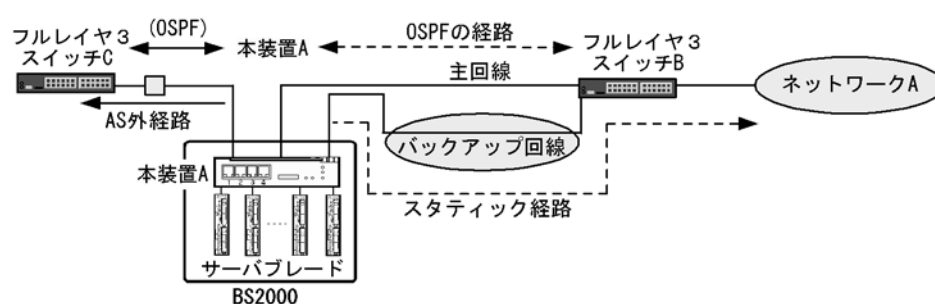
図 9-3 バックアップ回線を使用した構成での AS 外経路の導入例
