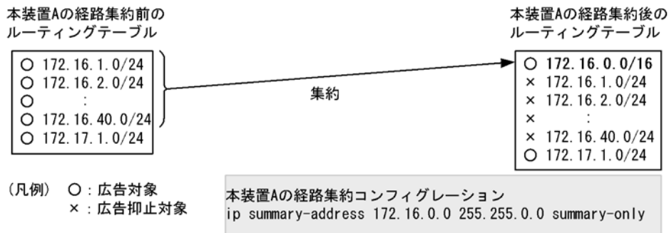
図 6-16 経路集約のコンフィグレーション例と経路集約前後の経路
