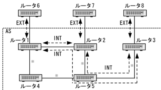
図 25-1 内部ピアと外部ピア
