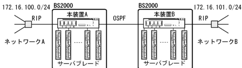
図 6-5 サブネット間の接続の例
