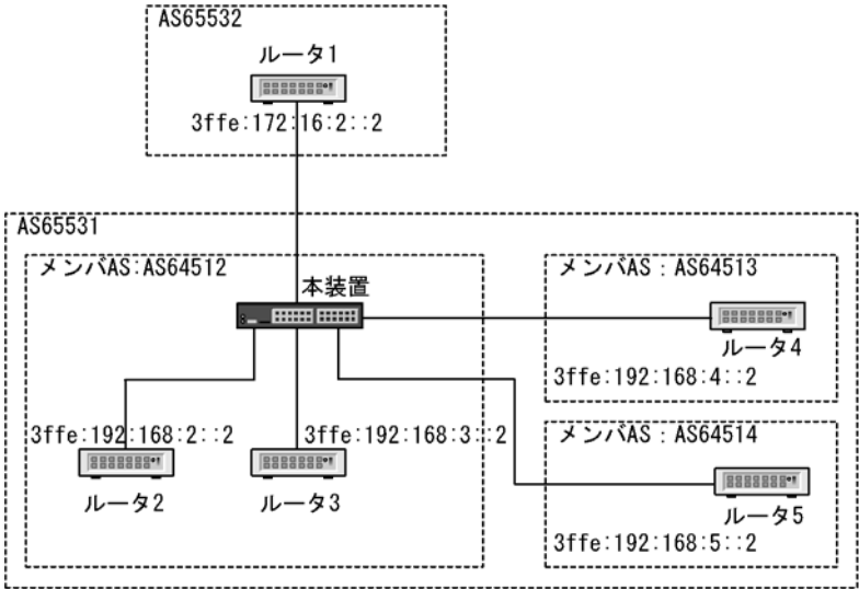
図 25-16 コンフェデレーション構成例
