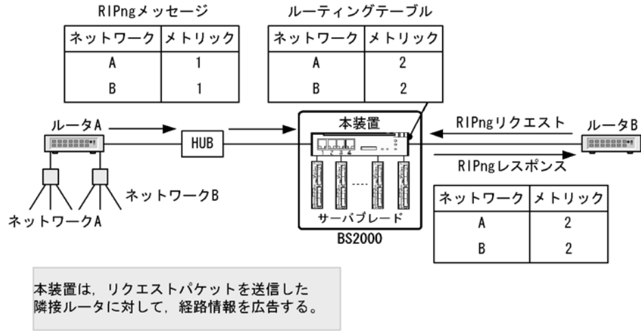
図 22-3 リクエストパケット受信による経路情報の広告
