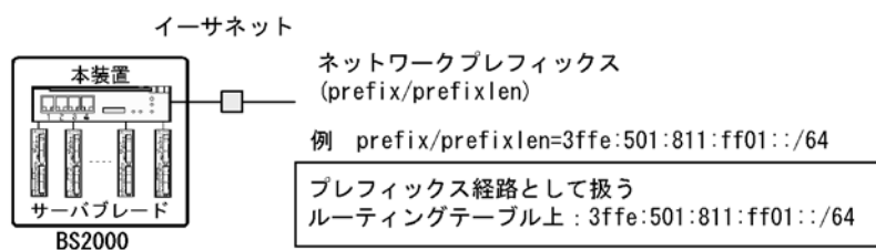
図 20-3 直結経路の取り扱い（ブロードキャスト型の場合）
