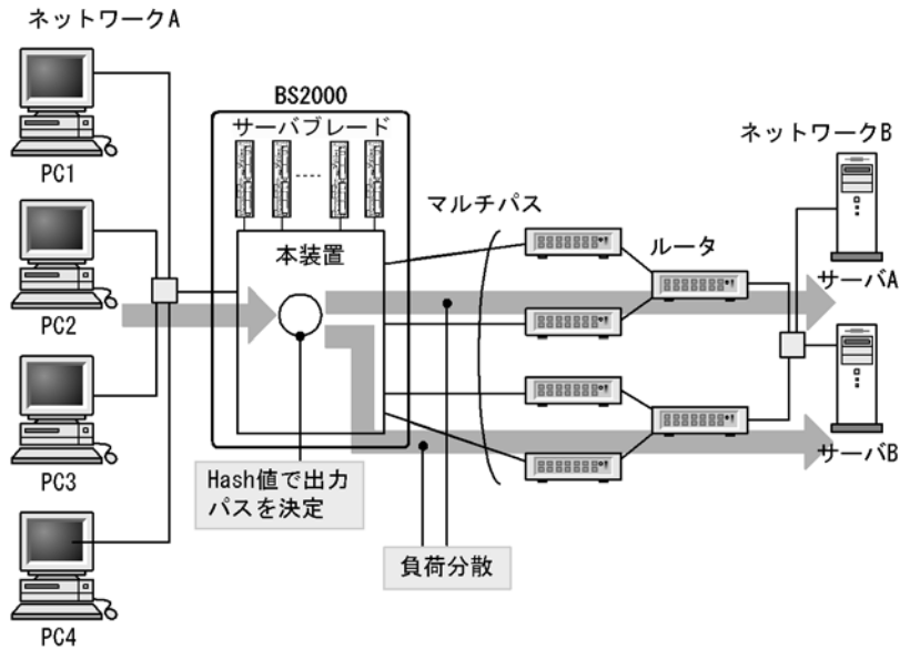
図 6-13 マルチパスを使用した負荷分散（隣接ルータが複数の場合）
