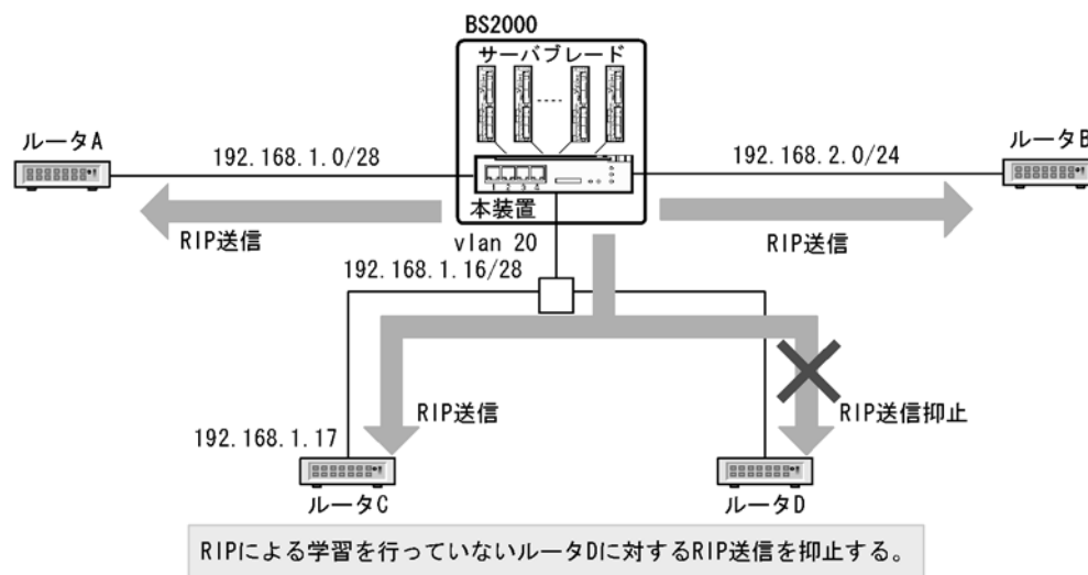
図 8-14 RIP パケット送信相手の限定
