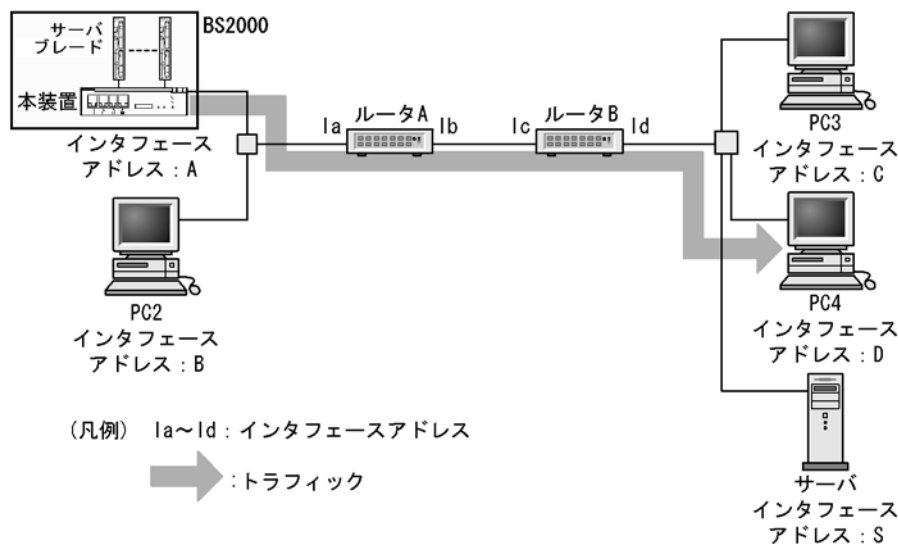
図 15-1 ユニキャストアドレス通信
