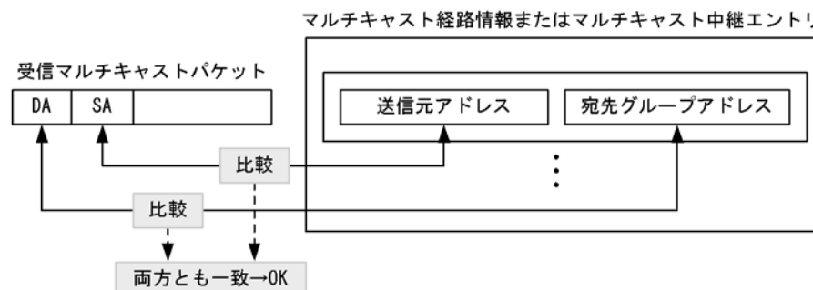
図 13-6 マルチキャスト経路情報またはマルチキャスト中継エントリの検索方法
