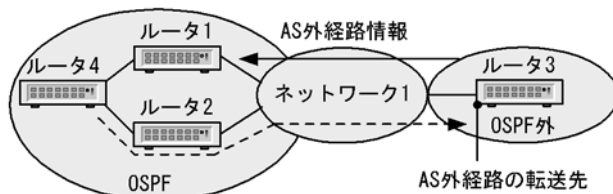
図 9-5 システム構成例（フォワーディングアドレスを目標とする場合）
