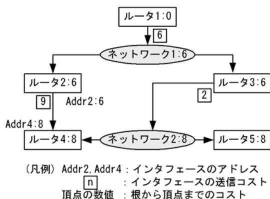
図 23-3 ルータ 1 を根とする最短木
