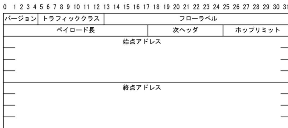
図 15-19 IPv6 ヘッダ形式
