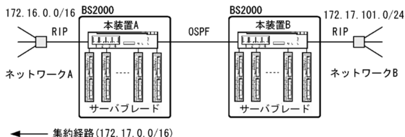
図 6-7 集約経路の広告の例
