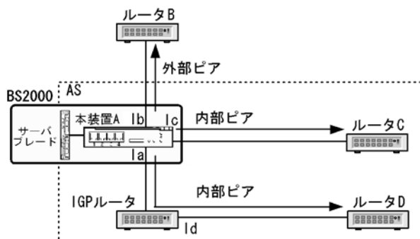
図 25-7 通知する経路情報のネクストホップの設定例
