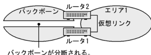
図 24-4 バックボーン分断に対する予備経路
