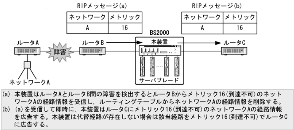
図 8-4 ルートポイズニング
