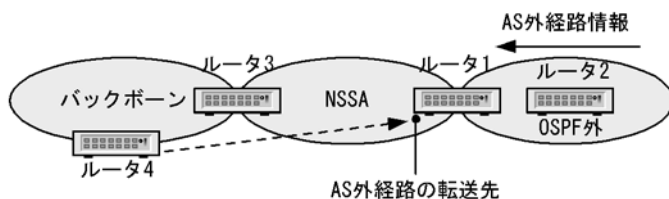
図 9-6 システム構成例（任意のインタフェースを目標とする場合）
