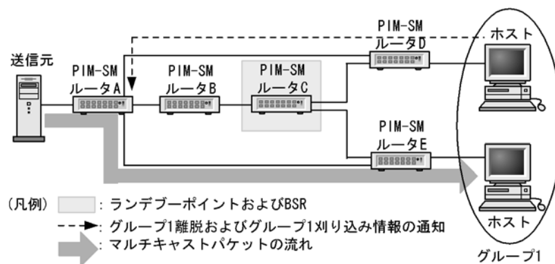
図 27-12 IPv6 マルチキャスト配送ツリーの刈り込み
