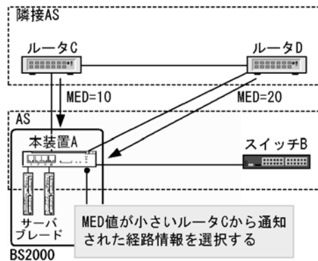
図 11-5 MED 属性による経路選択
