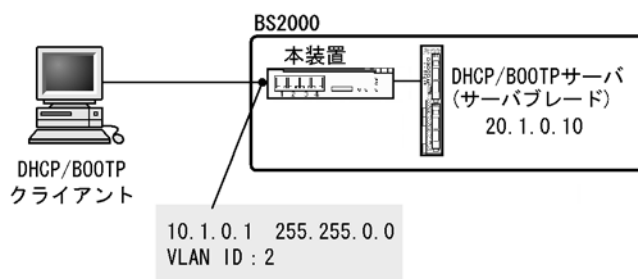
図 4-1 基本構成 (DHCP/BOOTP サーバと DHCP/BOOTP クライアント間にリレーエージェントが 1 台ある場合)
