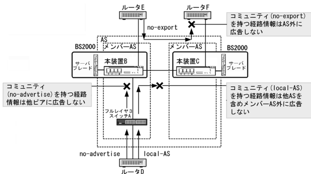
図 11-25 COMMUNITIES 属性を持つ経路情報の広告範囲
