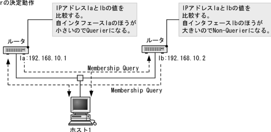
図 13-5 Querier と Non-Querier の決定
