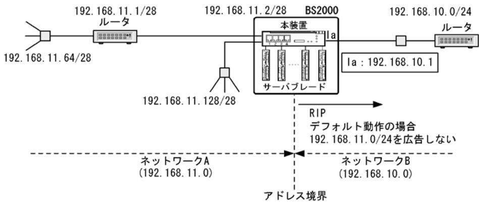
図 8-12 直結経路を広告しない構成例
