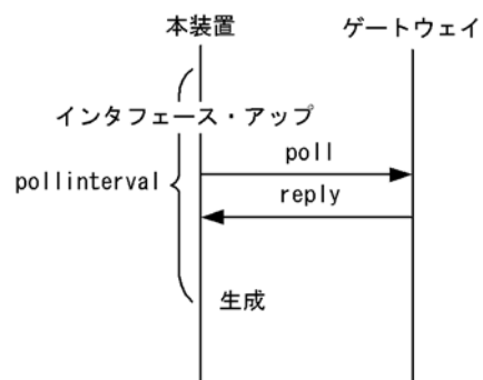
図 21-3 スタティック経路の動的監視による経路生成
