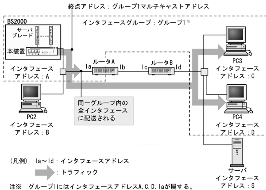
図 15-3 マルチキャストアドレス通信
