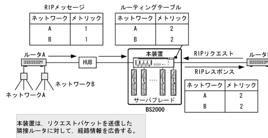
図 8-3 リクエストパケット受信による経路情報の広告
