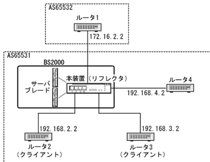
図 11-28 ルート・リフレクション構成例
