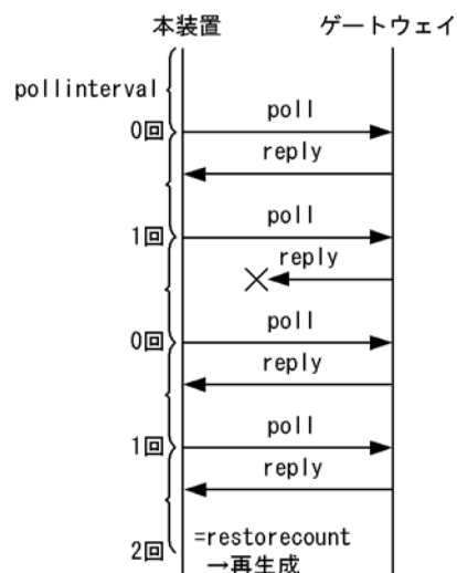
図 7-5 スタティック経路の動的監視による経路再生成 (restorecount =2 の場合)
