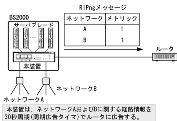
図 22-1 周期的な経路情報広告
