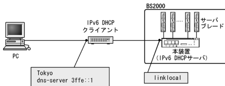
図 19-3 クライアントにオプション情報を配布する構成
