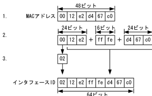
図 18-2 MAC アドレスからのインタフェース ID 生成
