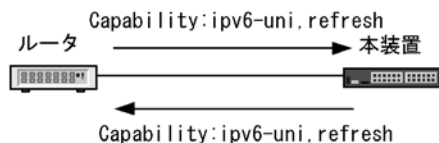
図 25-14 ルート・リフレッシュ機能の動作概念
