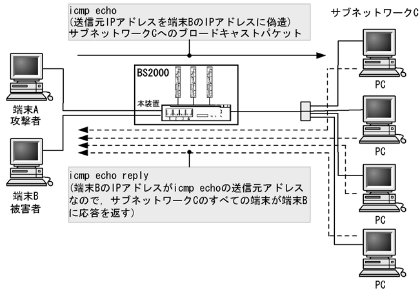
図 1-4 サブネットワークへのブロードキャストパケットを使った攻撃例
