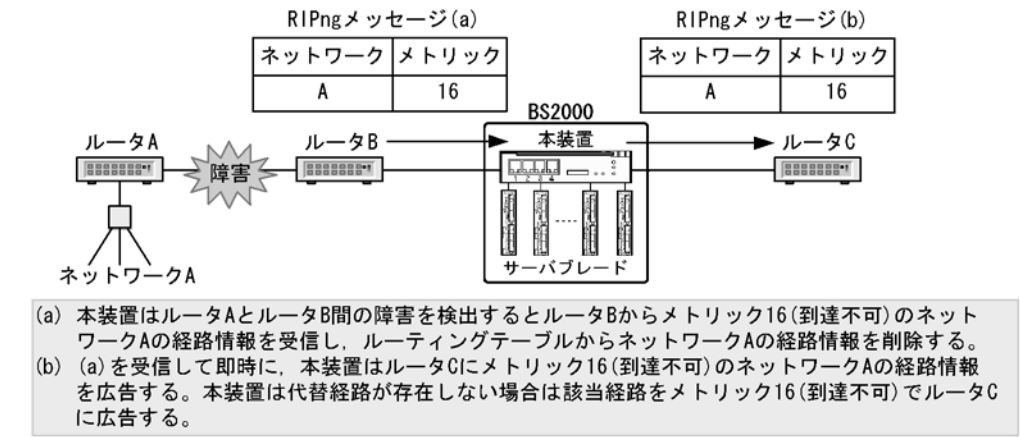
図 22-4 ルートポイズニング
