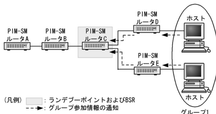
図 13-9 ランデブーポイントへのグループ参加情報の通知
