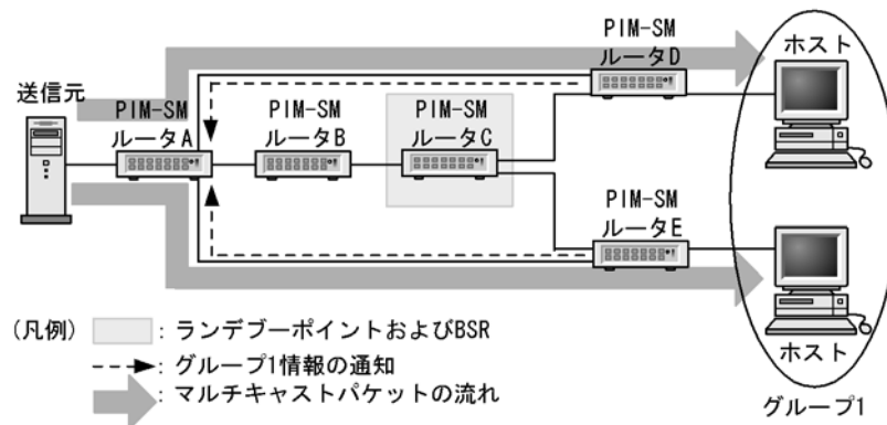
図 27-11 最短パスの IPv6 マルチキャストパケット通信
