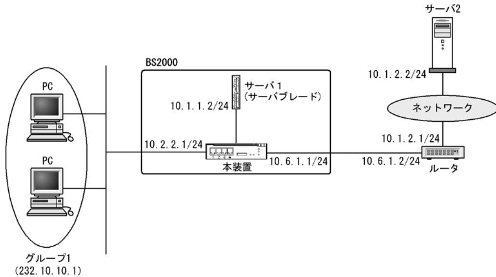
図 14-2 PIM-SSM 構成例
