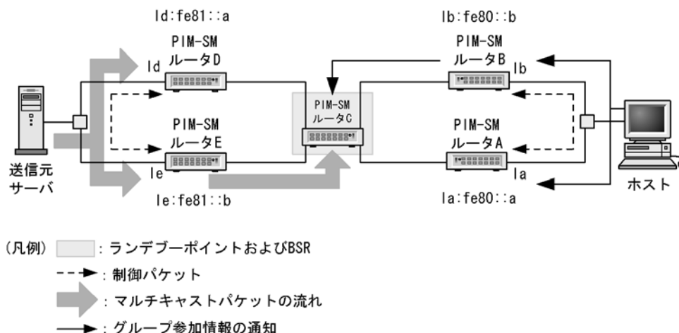
図 27-15 DR の動作
