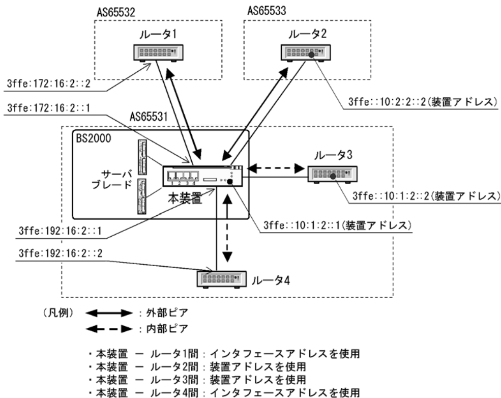
図 25-8 接続構成例
