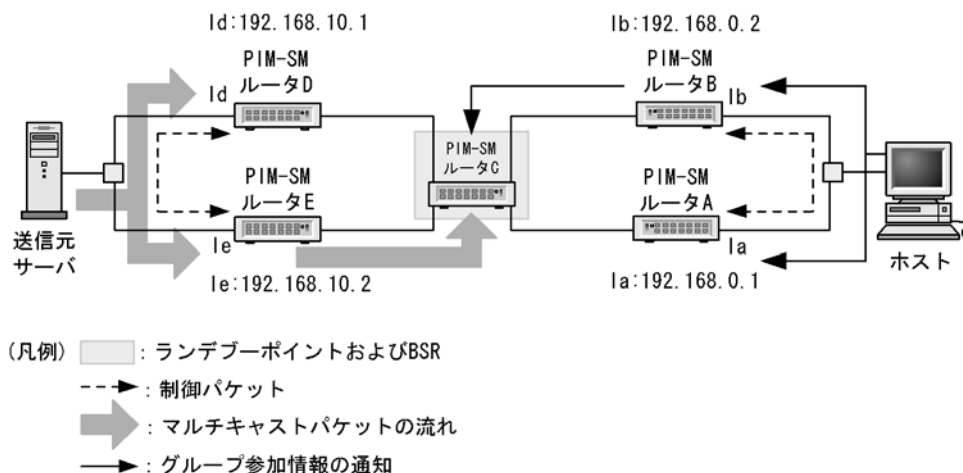
図 13-15 DR の動作
