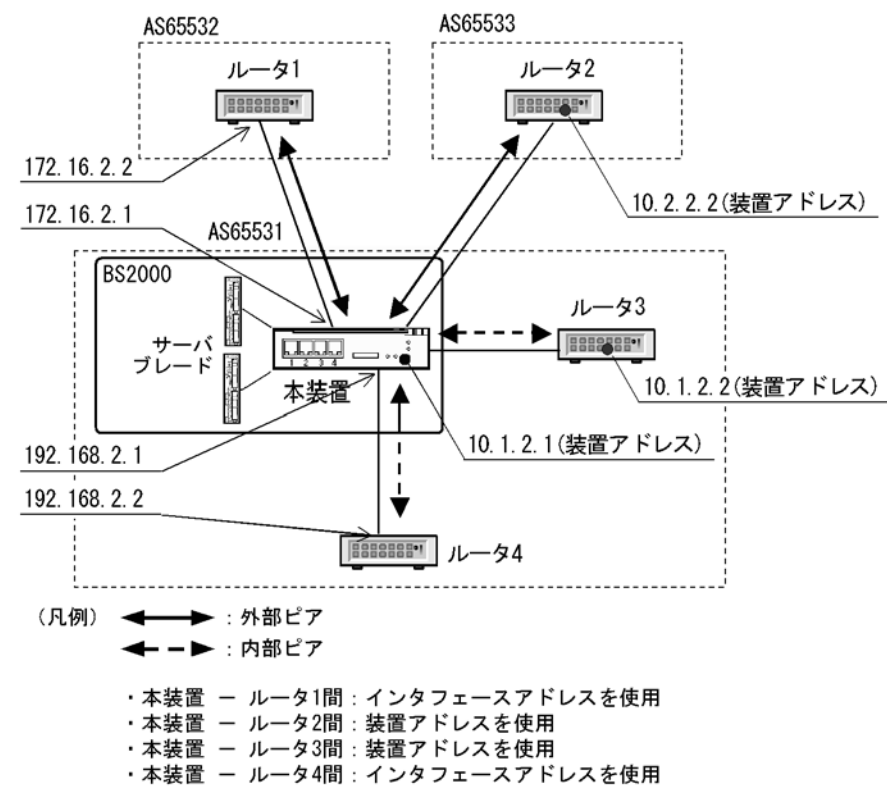
図 11-8 接続構成例
