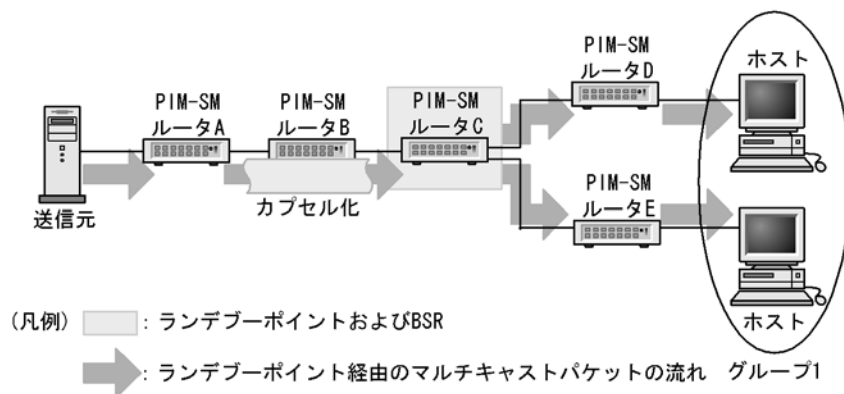
図 27-9 IPv6 マルチキャストパケット通信（カプセル化）
