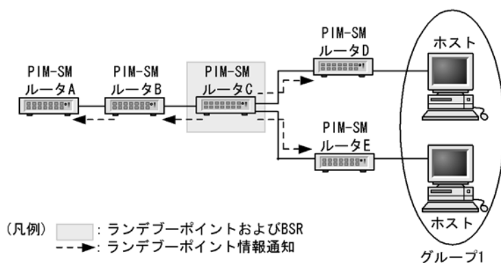
図 27-7 ランデブーポイントおよびブートストラップルータ（BSR）
