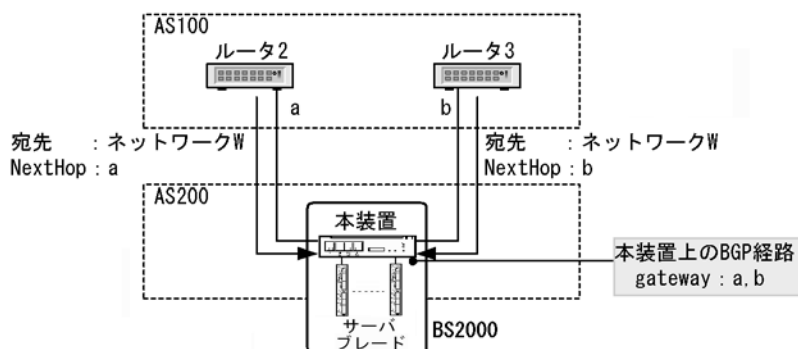
図 11-16 複数のピアから学習した BGP4 経路マルチパス化の概念
