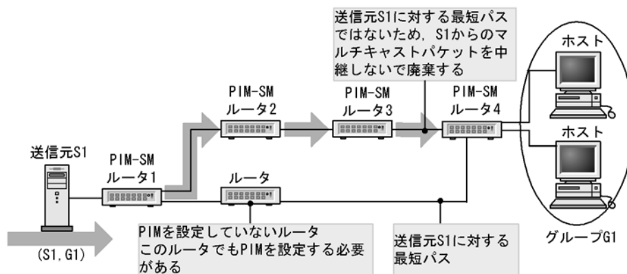
図 13-16 冗長経路時の注意
