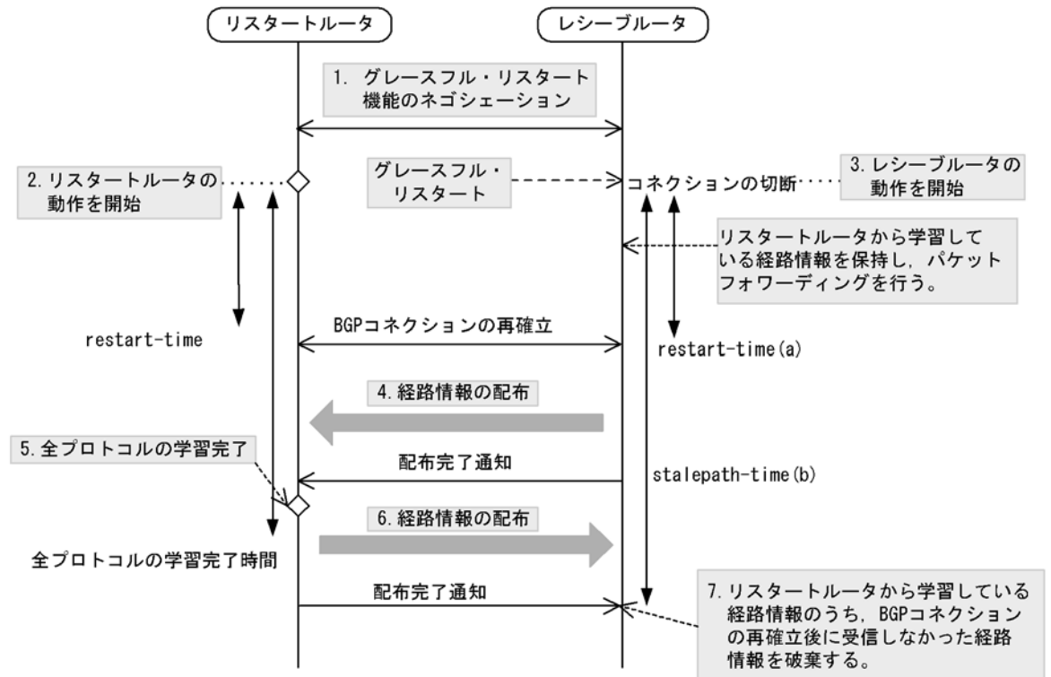
図 11-27 グレースフル・リスタートのシーケンス
