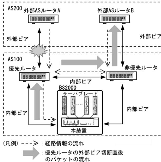
図 6-20 経路削除保留機能の適用例
