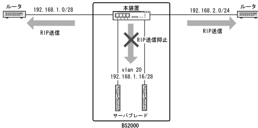
図 8-13 RIP パケットの送信抑制
