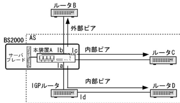
図 11-7 通知する経路情報の NEXT_HOP 属性の設定例
