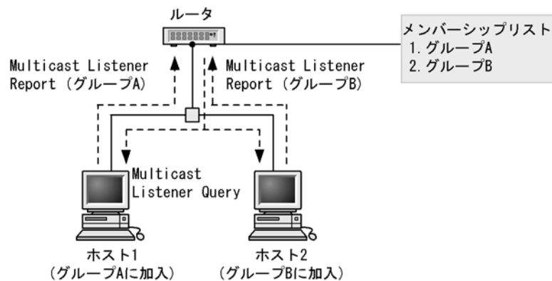
図 27-2 MLDv1 グループ参加・離脱動作
