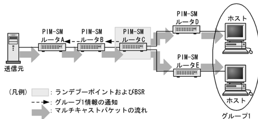
図 27-10 IPv6 マルチキャストパケット通信（デカプセル化）
