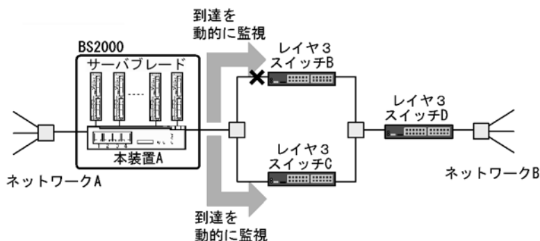
図 7-2 スタティック経路の動的監視の例
