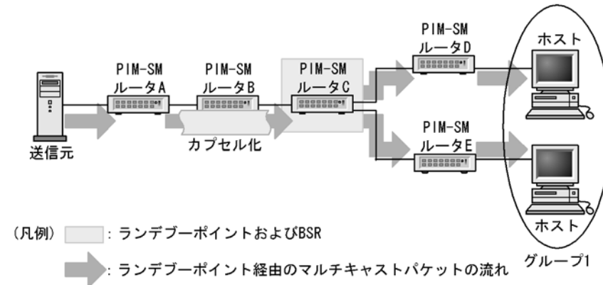
図 13-10 ランデブーポイント経由のマルチキャストパケット通信（カプセル化）
