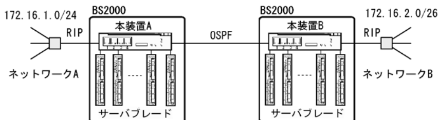
図 6-2 異なるサブネットマスク長のサブネット間の接続
