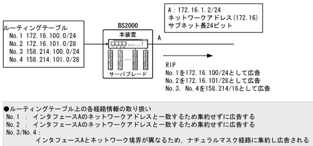
図 8-7 RIP-2 使用時の広告経路自動集約化
