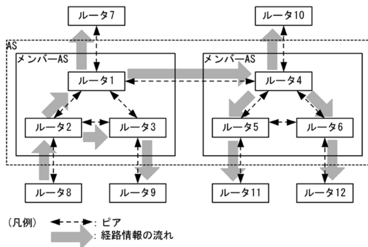
図 11-23 コンフェデレーション構成での経路情報の流れ
