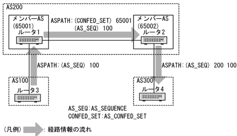
図 11-24 AS_PATH 属性の取り扱い
