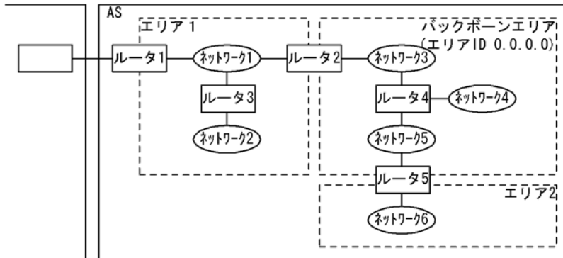
図 10-1 エリア分割を使用した OSPF ネットワークトポロジの例
