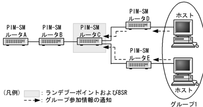
図 27-8 ランデブーポイントへのグループ参加情報の通知
