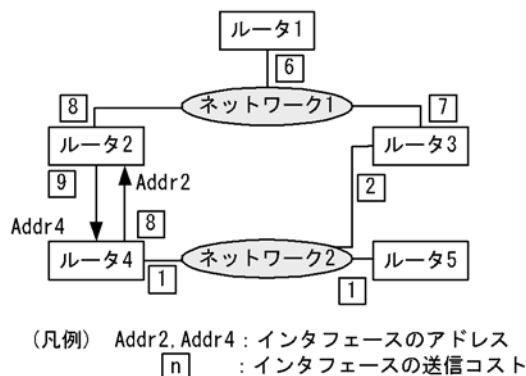
図 23-2 トポロジとコストの設定例
