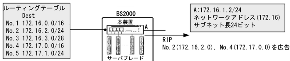
図 8-11 RIP で広告するナチュラルマスク経路およびサブネットマスク経路情報
