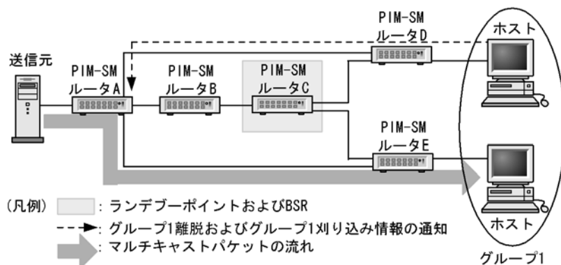
図 13-13 マルチキャスト配送ツリーの刈り込み
