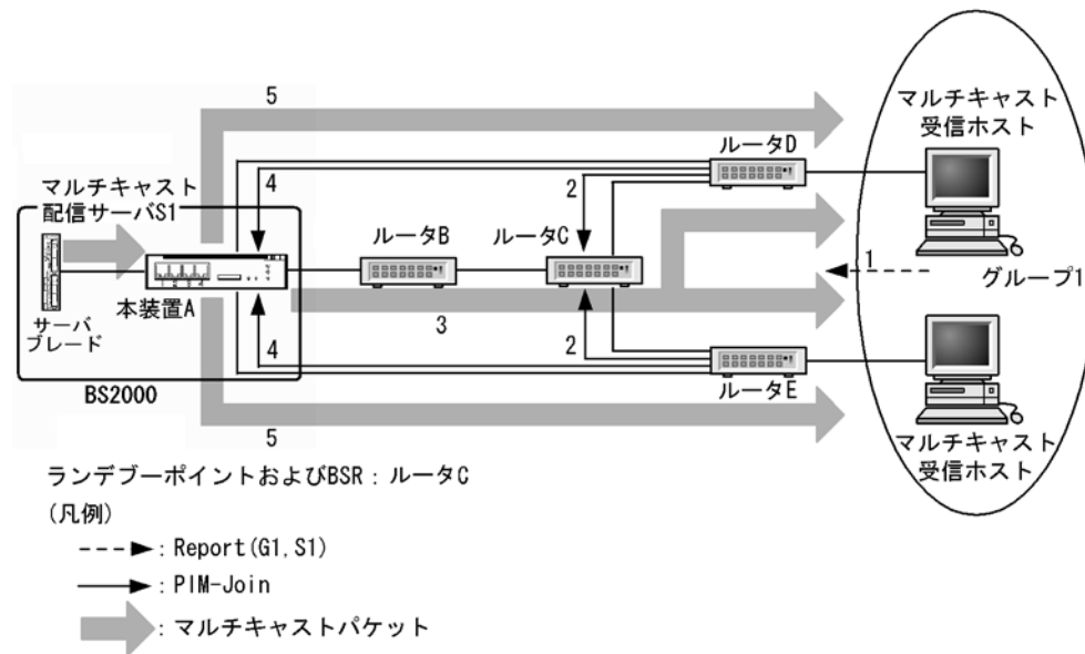
図 13-19 IGMPv3 使用時の IPv4 PIM-SM 動作概要
