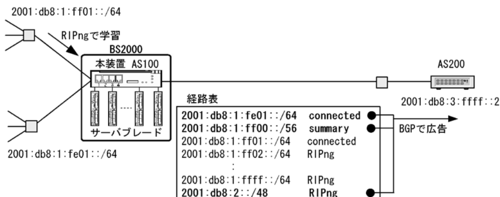
図 20-8 集約経路を BGP4+ で広告する構成
