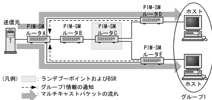
図 13-12 最短パスのマルチキャストパケット通信
