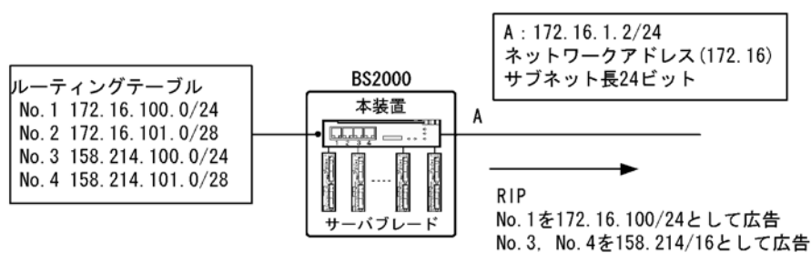
図 8-6 RIP-1 使用時の広告経路自動集約化
