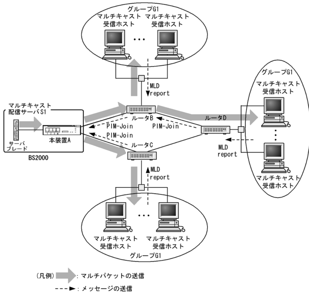
図 27-18 IPv6 PIM-SSM の動作概要（ホストが MLDv1 または MLDv2（EXCLUDE モード）の場合）
