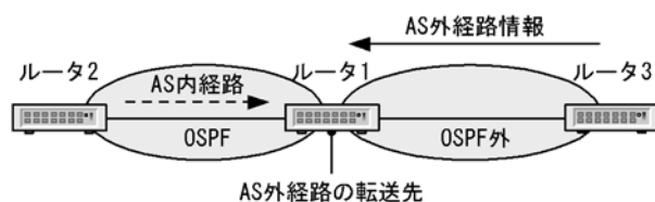
図 9-4 システム構成例（AS 境界ルータを目標とする場合）
