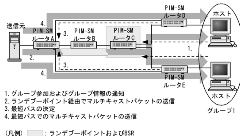
図 13-7 PIM-SM の動作概要
