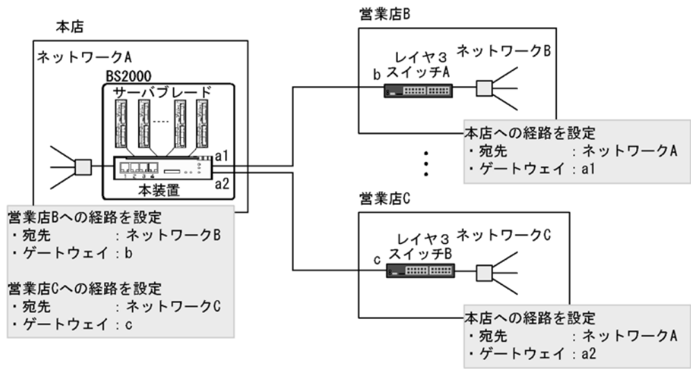
図 21-1 スタティックルーティングのネットワーク構成例
