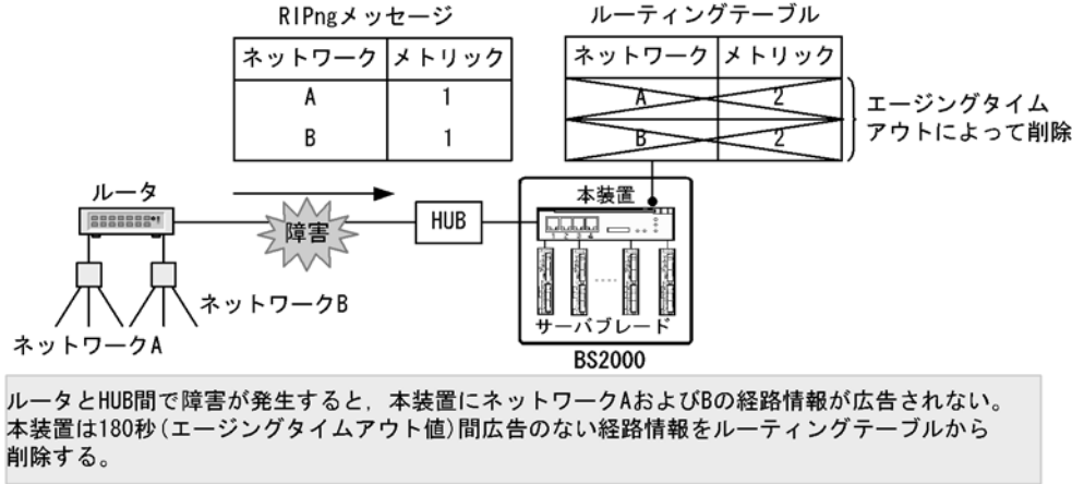
図 22-7 エージングタイムアウトによる経路情報の削除
