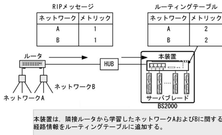
図 8-8 レスポンスパケット受信による経路情報の生成
