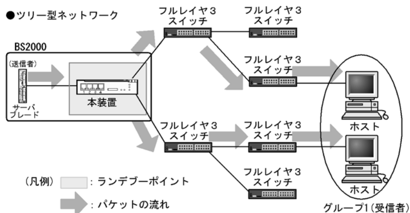
図 13-22 PIM-SM 推奨ネットワーク構成
