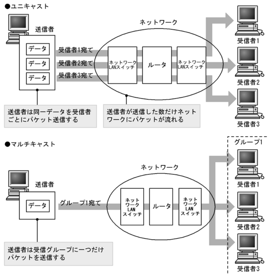
図 13-1 マルチキャストの概要 (IPv4)
