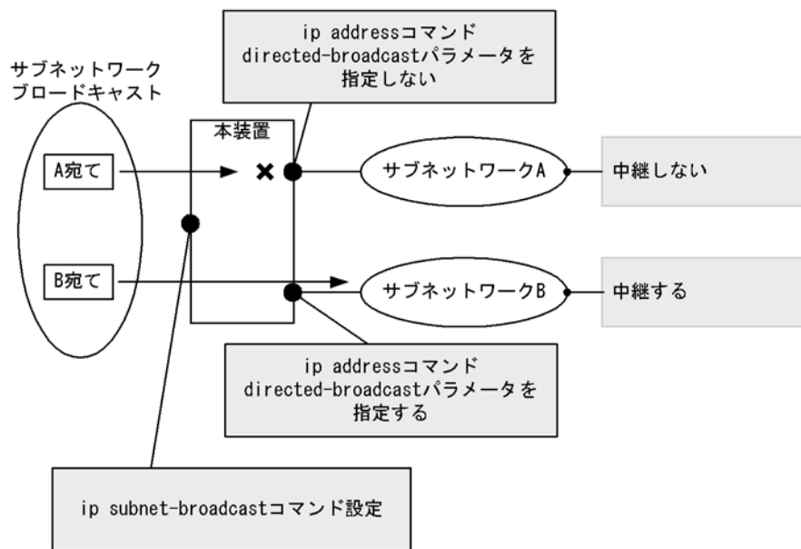
図 1-5 コマンド設定例
