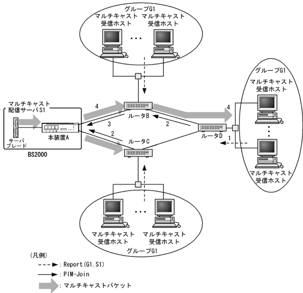
図 27-19 IPv6 PIM-SSM 動作概要（ホストが MLDv2（INCLUDE モード）の場合）
