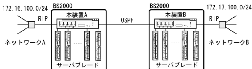
図 6-3 異なるネットワークアドレスのサブネット間の接続
