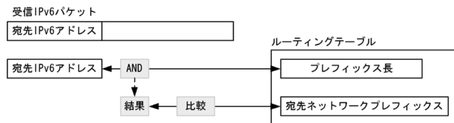
図 15-20 ルーティングテーブルの検索
