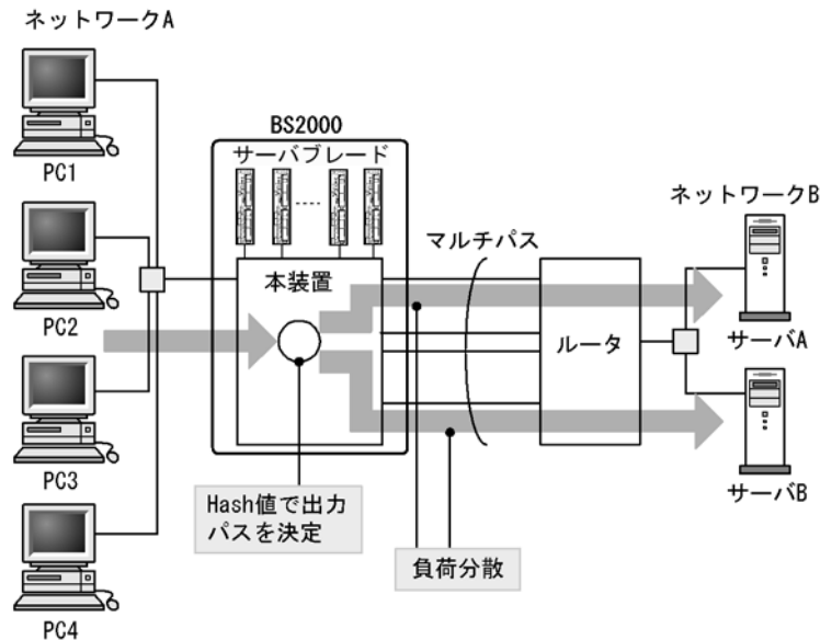
図 6-12 マルチパスを使用した負荷分散（隣接ルータが単一の場合）
