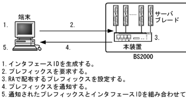
図 18-1 RA による端末のアドレス設定
