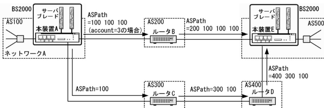
図 25-4 set as-path prepend count コマンドの使用例
