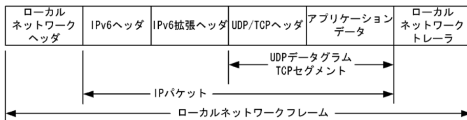
図 15-18 IPv6 パケットフォーマット
