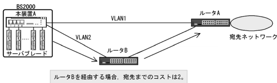
図 9-7 マルチパスの構成
