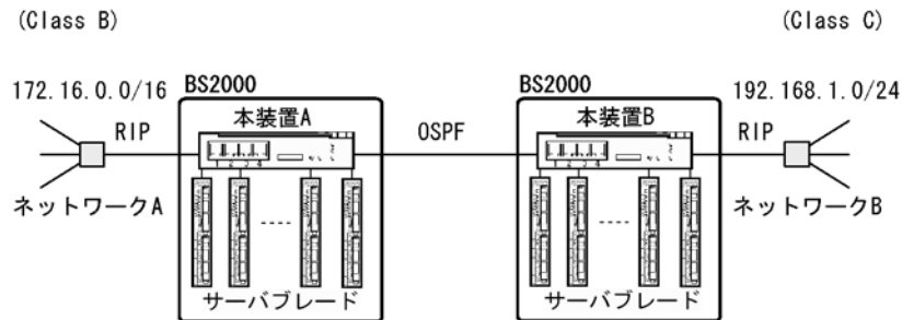
図 6-4 サブネットを使用しない例
