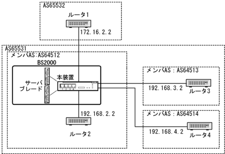
図 11-29 コンフェデレーション構成例
