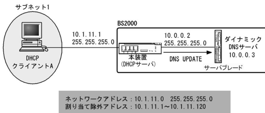
図 5-3 ダイナミック DNS 連携をする場合の接続構成
