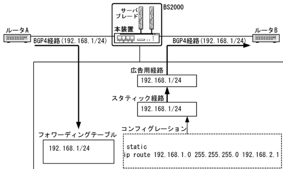
図 11-19 広告用経路生成と広告
