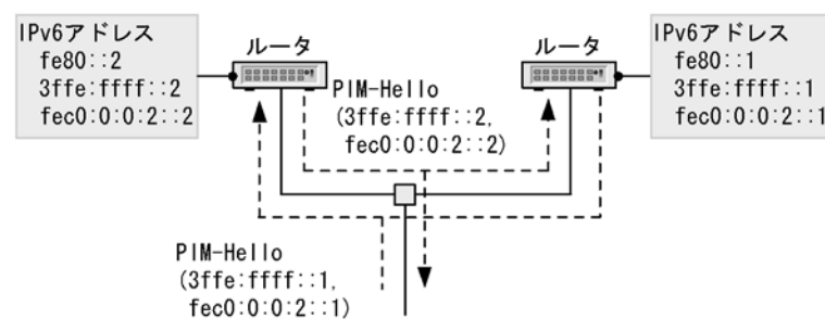
図 27-13 PIM-Hello メッセージによる隣接ルータアドレス受信
