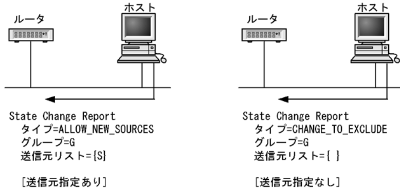
図 27-3 MLDv2 グループ参加・離脱動作
