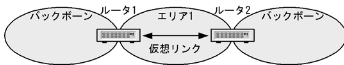
図 24-3 バックボーン間の接続
