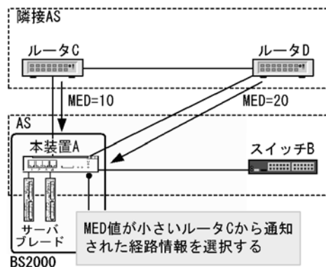
図 25-5 MED 属性による経路選択
