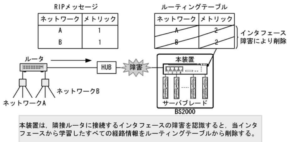
図 8-10 インタフェース障害による経路情報の削除
