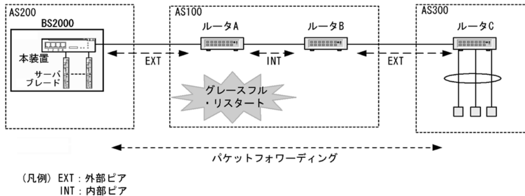
図 11-26 グレースフル・リスタートの例
