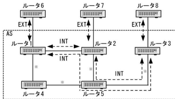
図 11-1 内部ピアと外部ピア
