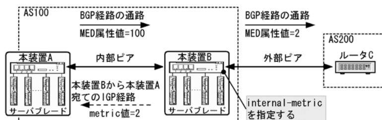
図 25-6 set metric-type internal の使用例
