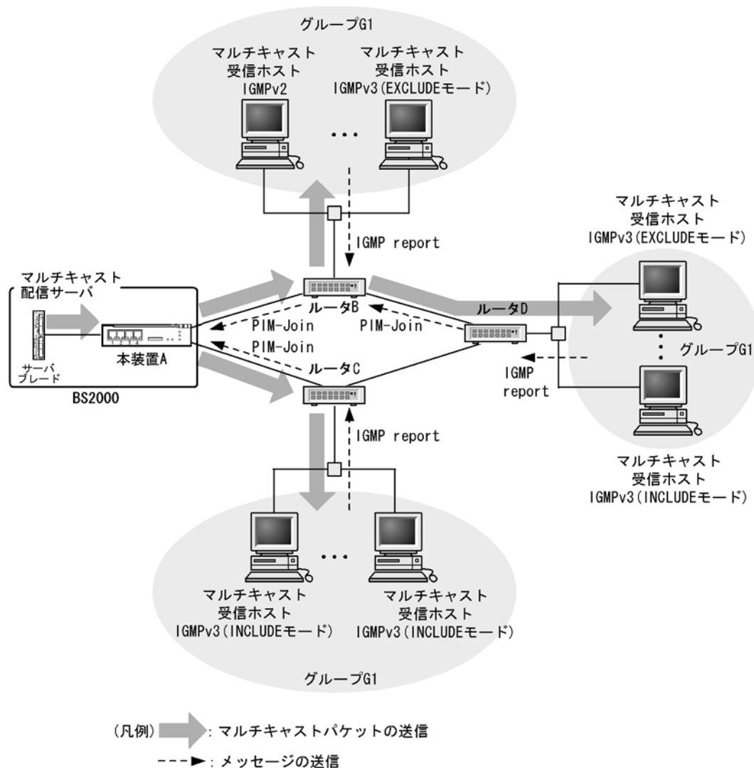
図 13-17 PIM-SSM の動作概要
