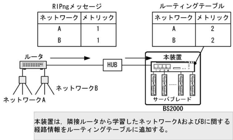
図 22-6 レスポンスパケット受信による経路情報の生成
