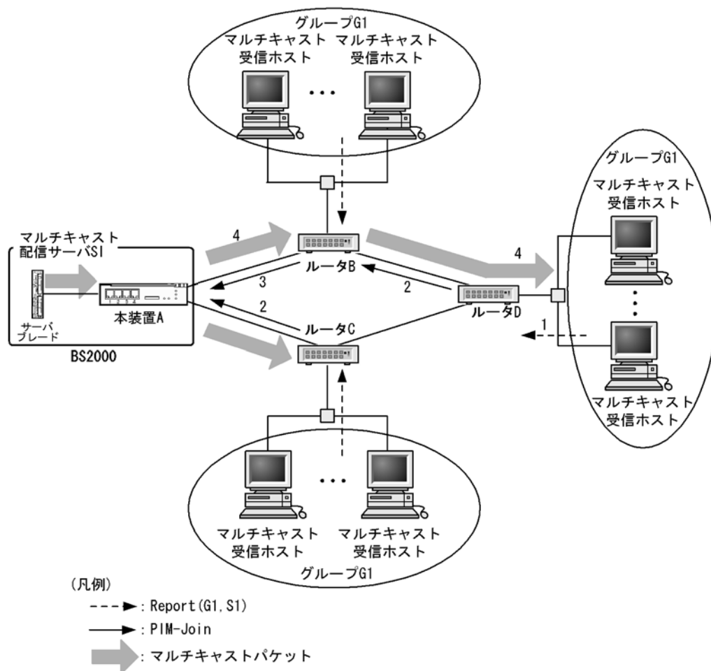
図 13-18 IGMPv3 使用時の IPv4 PIM-SSM 動作概要
