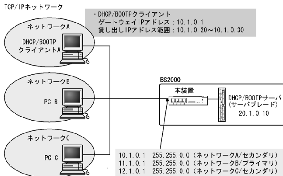
図 4-2 マルチホーム構成
