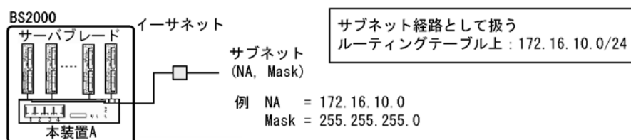
図 6-10 直結経路の取り扱い
