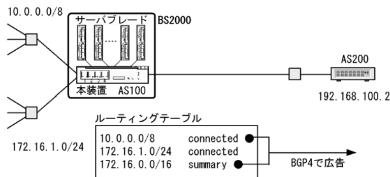
図 6-17 集約経路を BGP4 で広告する構成
