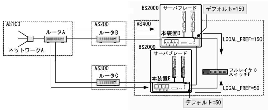
図 25-2 LOCAL_PREF 属性による経路選択
