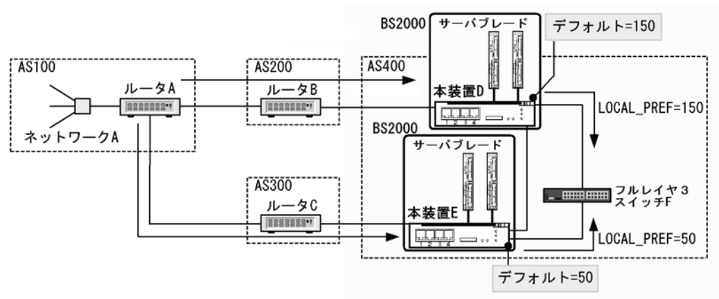
図 11-2 LOCAL_PREF 属性による経路選択
