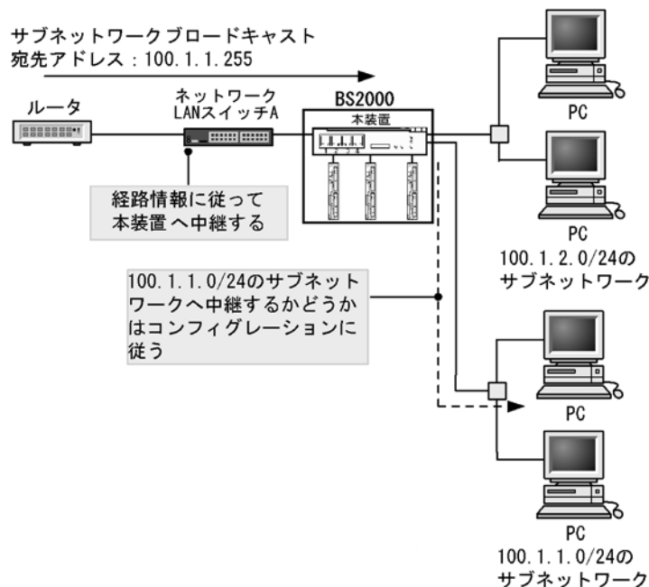
図 1-7 サブネットワークブロードキャスト
