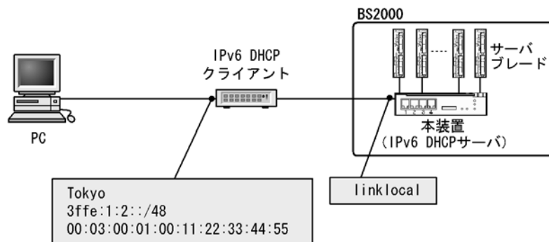
図 19-1 クライアントごとに固定プレフィックスを指定する構成
