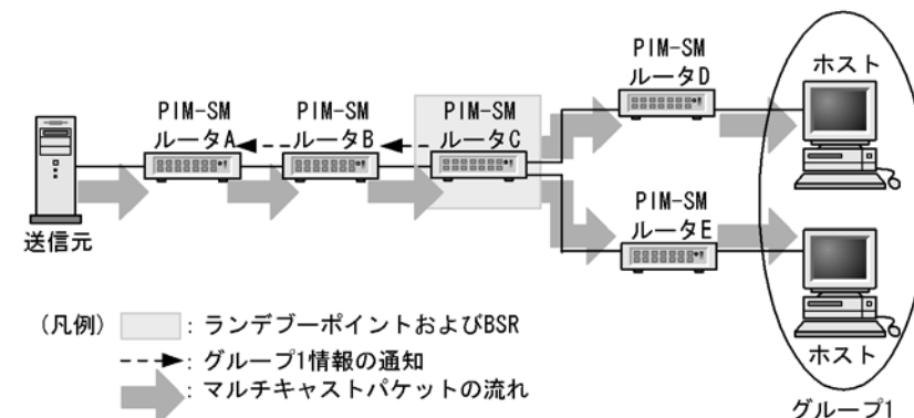
図 13-11 ランデブーポイント経由のマルチキャストパケット通信（デカプセル化）
