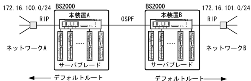
図 6-6 デフォルトルートの広告の例
