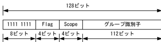
図 27-1 マルチキャストアドレスのフォーマット
