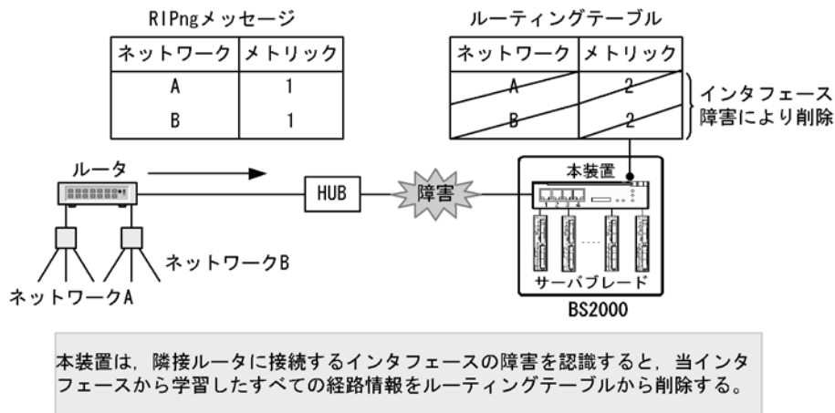
図 22-8 インタフェース障害による経路情報の削除
