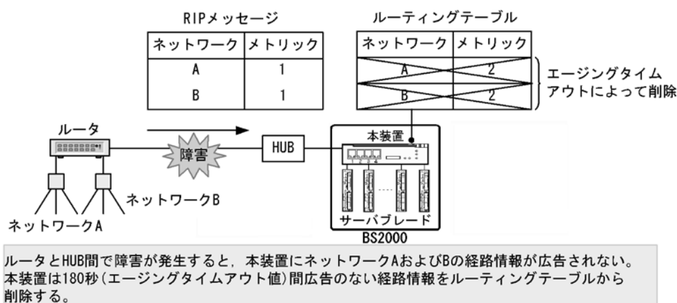
図 8-9 エージングタイムアウトによる経路情報の削除
