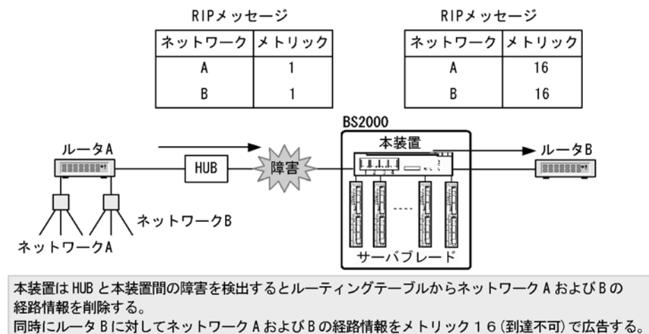
図 8-2 triggered update による経路情報の広告
