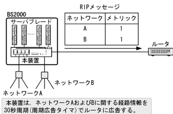
図 8-1 周期的な経路情報広告
