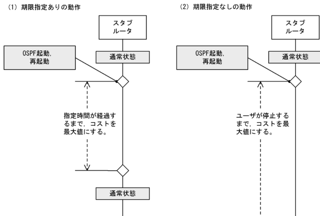
図 10-7 スタブルータの動作
