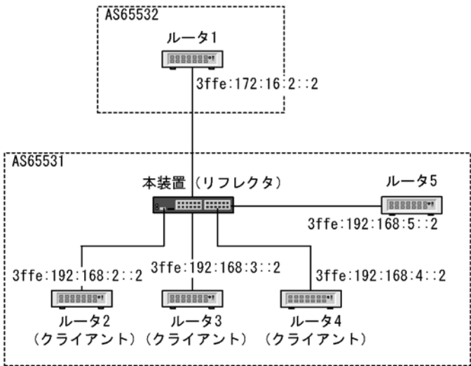
図 25-15 ルート・リフレクション構成例
