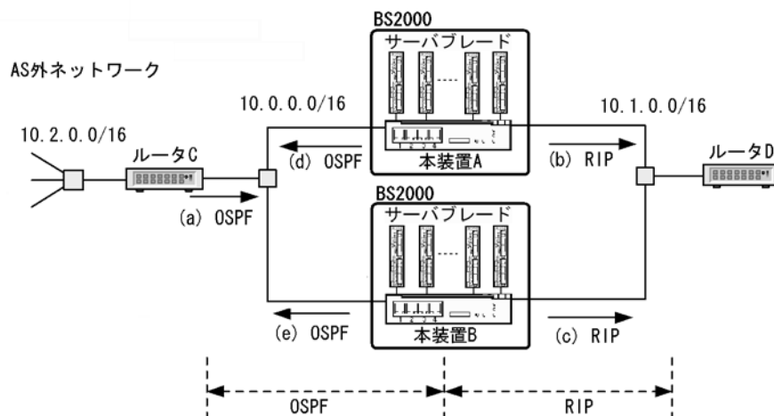
図 6-8 ネットワーク構成例
