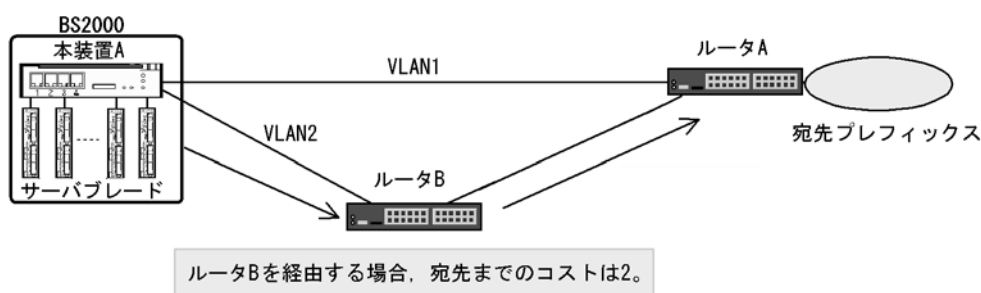
図 23-5 マルチパスの構成
