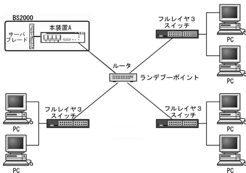
図 27-20 IPv6 PIM-SM を使用する構成図
