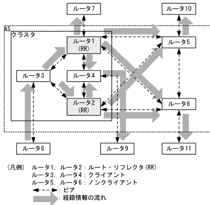
図 11-22 ルート・リフレクタの冗長構成の例
