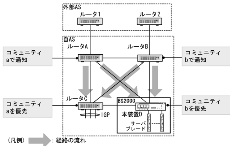
図 11-14 学習経路フィルタリングと COMMUNITIES 属性の使用例
