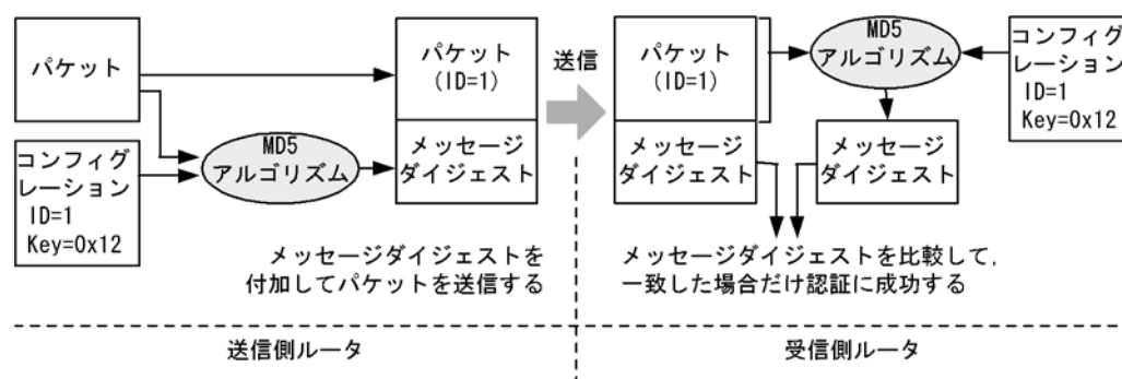
図 10-6 MD5 認証のデータフロー
