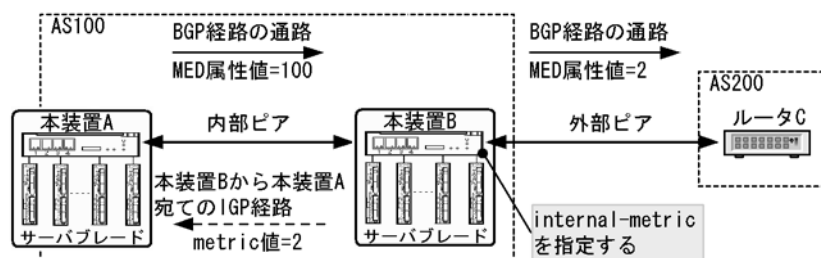
図 11-6 set metric-type internal の使用例
