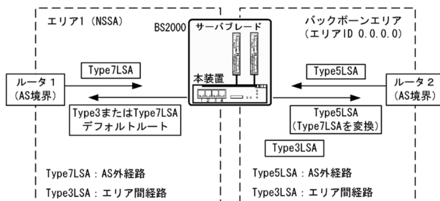
図 10-2 NSSA とバックボーンの間での経路交換
