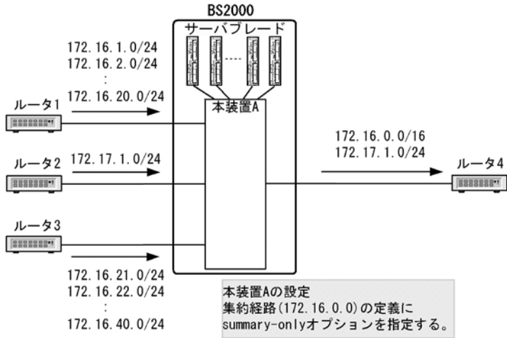
図 6-15 集約元経路の広告抑止の適用例
