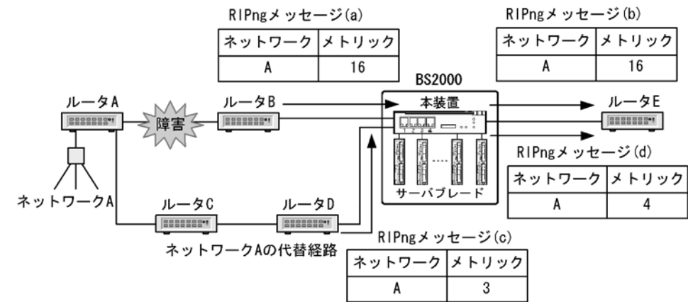
図 22-5 ルートポイズニング期間中の再学習
