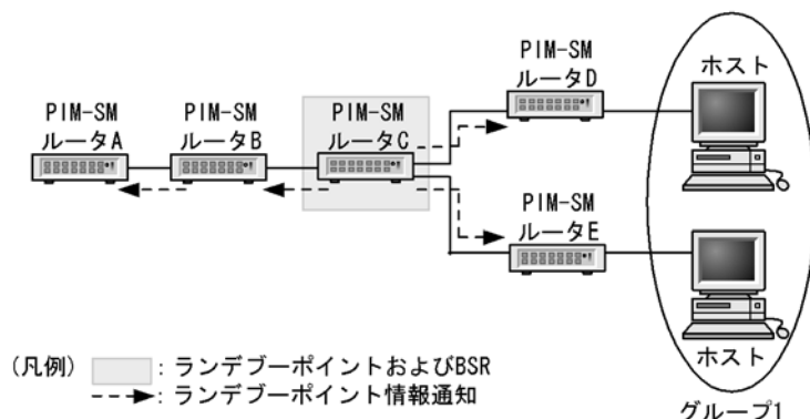
図 13-8 ランデブーポイントおよびブートストラップルータ（BSR）の役割
