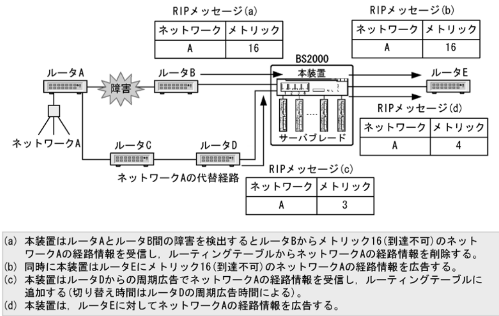
図 8-5 ルートポイズニング期間中の再学習
