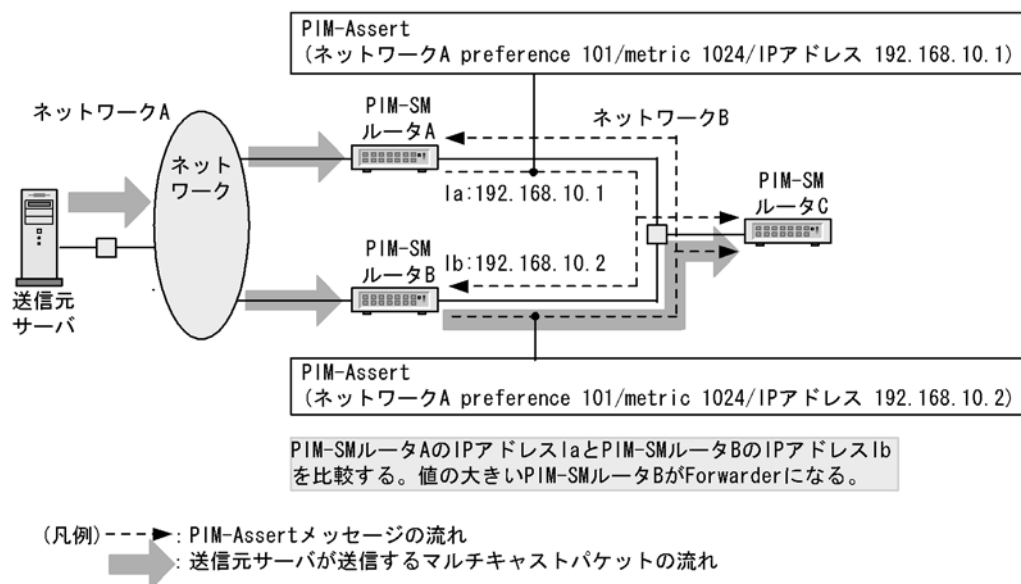
図 13-14 Forwarder の決定
