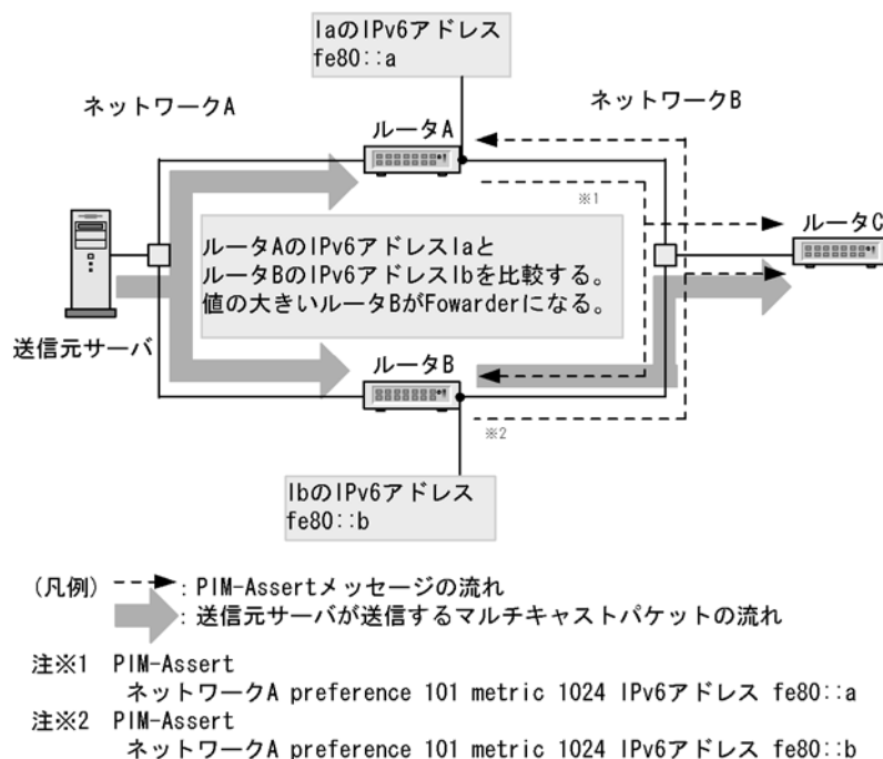
図 27-14 Forwarder の決定
