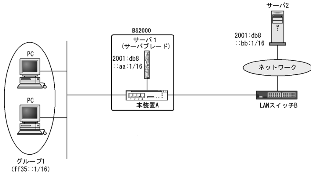
図 28-1 PIM-SSM 構成例
