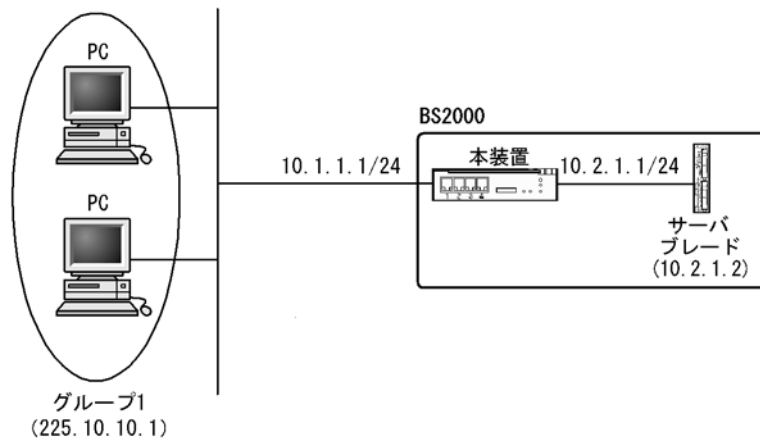
図 14-1 PIM-SM 構成例
