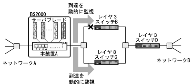
図 21-2 スタティック経路の動的監視の例
