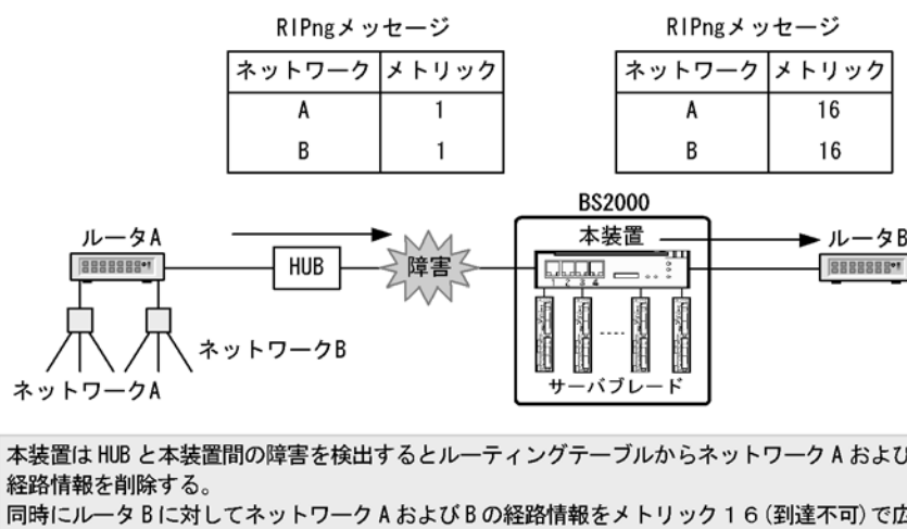
図 22-2 triggered update による経路情報の広告
