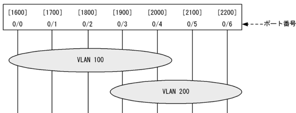
図 1-9 VLAN インタフェースの設定例
