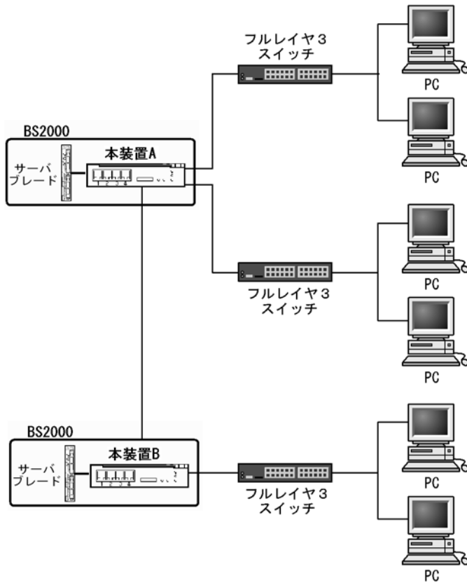
図 13-21 PIM-SSM を使用する構成図
