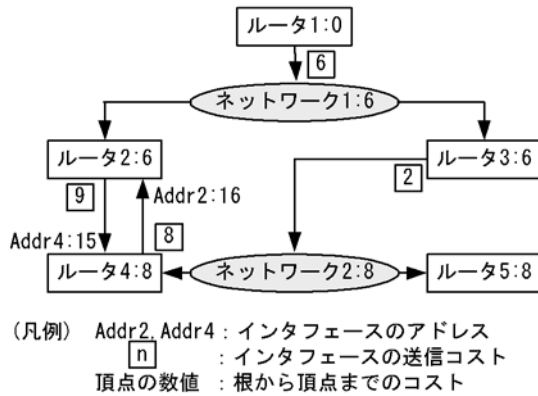
図 9-2 ルータ 1 を根とする最短木
