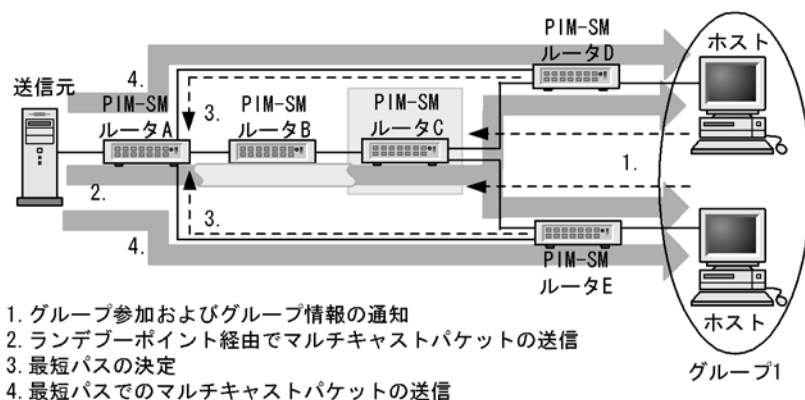
図 27-6 PIM-SM の動作概要
