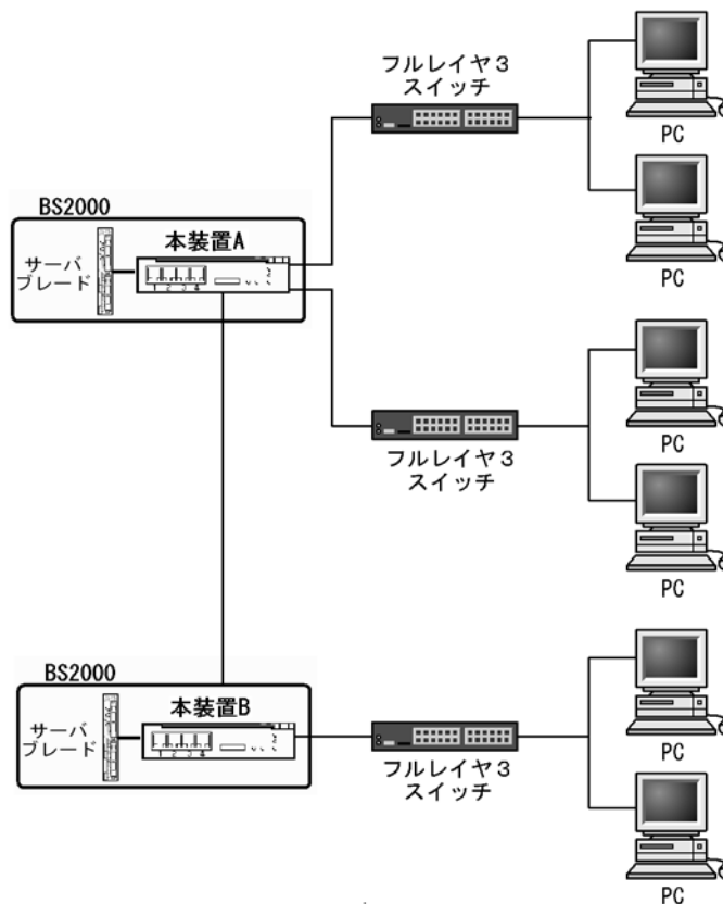
図 27-21 IPv6 PIM-SSM を使用する構成図
