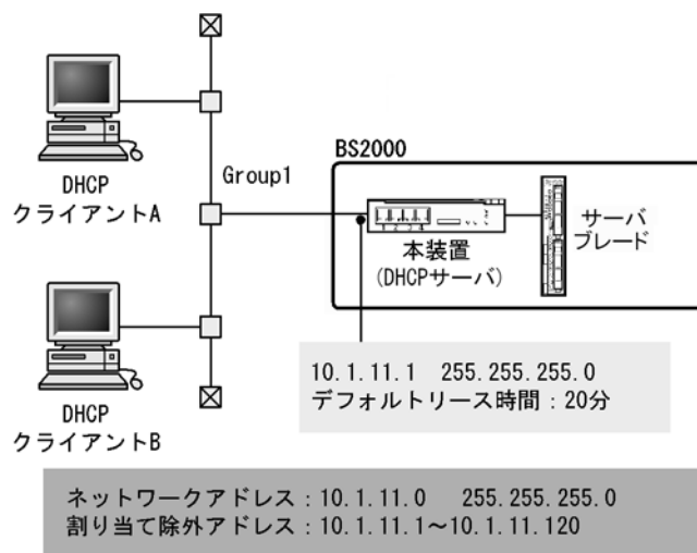
図 5-1 クライアントーサーバ構成（動的 IP アドレス配布時）
