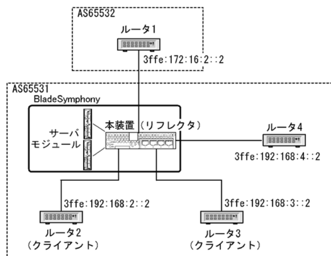
図 26-15 ルート・リフレクション構成例
