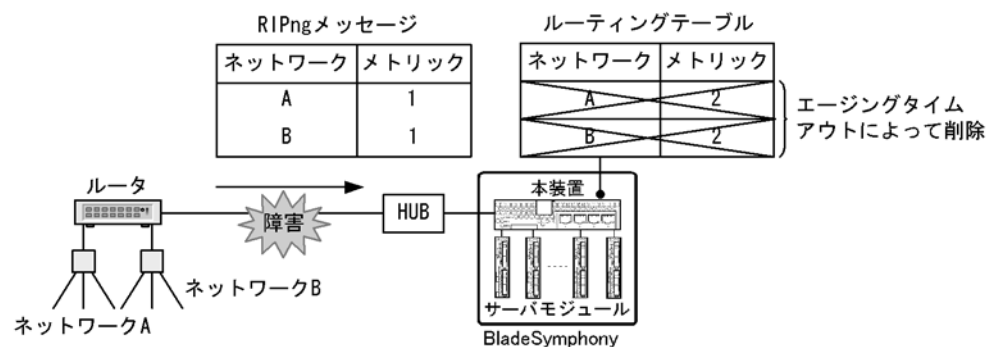
図 23-7 エージングタイムアウトによる経路情報の削除
