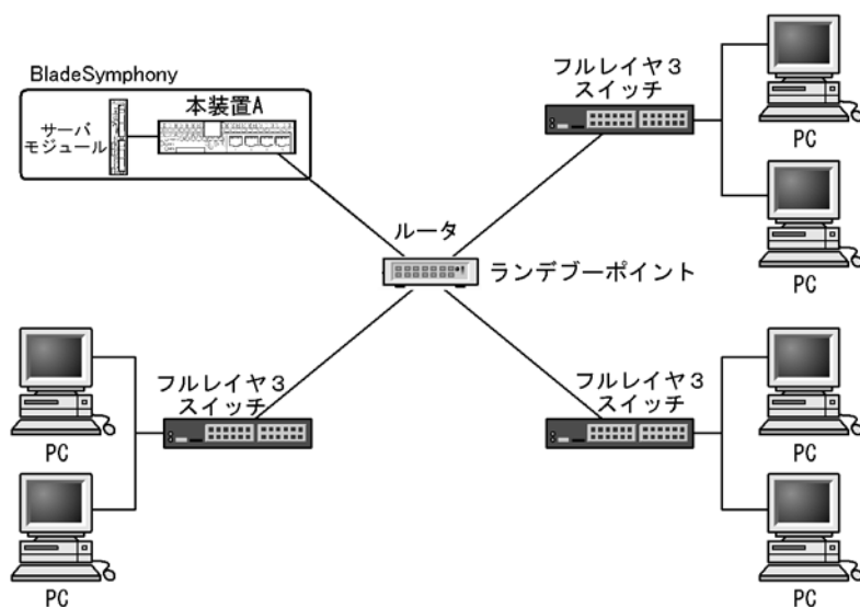
図 28-25 IPv6 PIM-SM を使用する構成図
