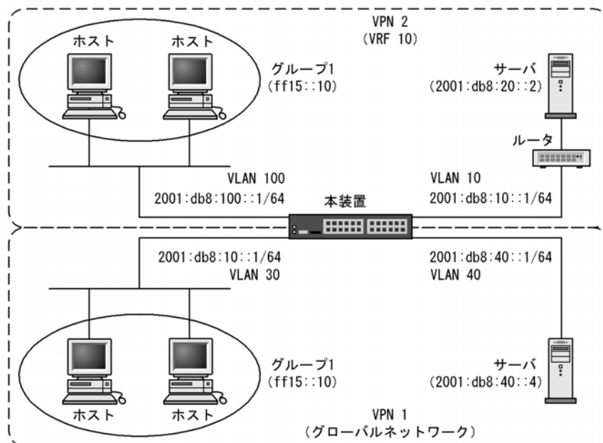
図 29-2 VRF での IPv6 PIM-SM 構成例
