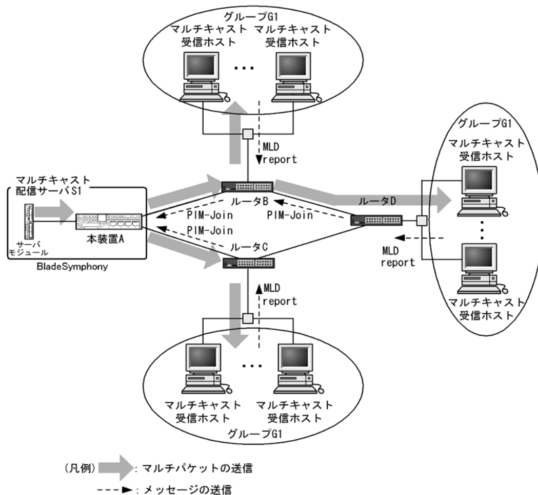
図 28-18 IPv6 PIM-SSM の動作概要
