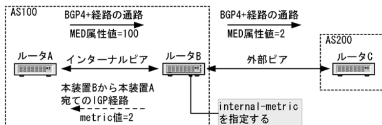
図 26-6 set metric-type internal の使用例
