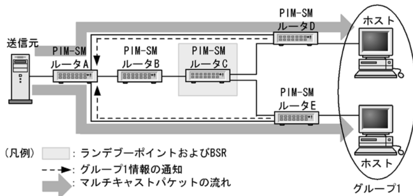
図 28-11 最短パスの IPv6 マルチキャストパケット通信
