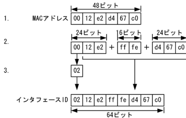
図 19-2 MAC アドレスからのインタフェース ID 生成
