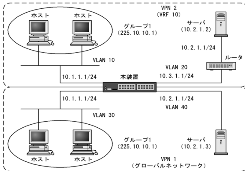
図 14-5 VRF での IGMP 構成例
