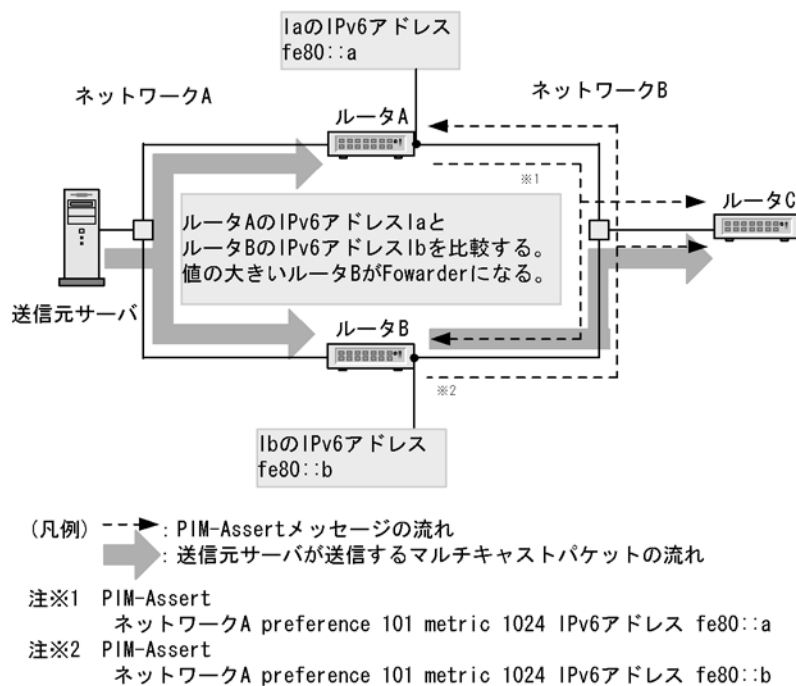
図 28-14 Forwarder の決定
