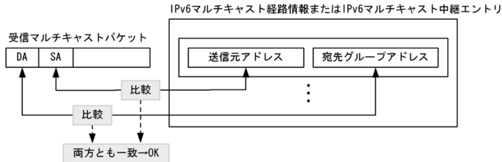
図 28-5 IPv6 マルチキャスト経路情報または IPv6 マルチキャスト中継エントリの検索方法
