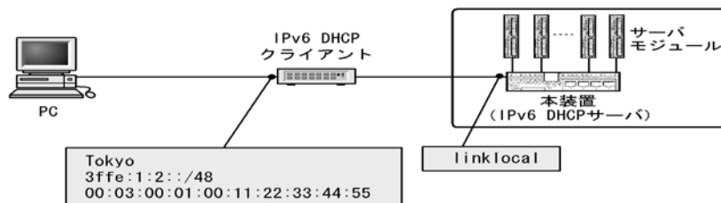
図 20-1 クライアントごとに固定プレフィックスを指定する構成
