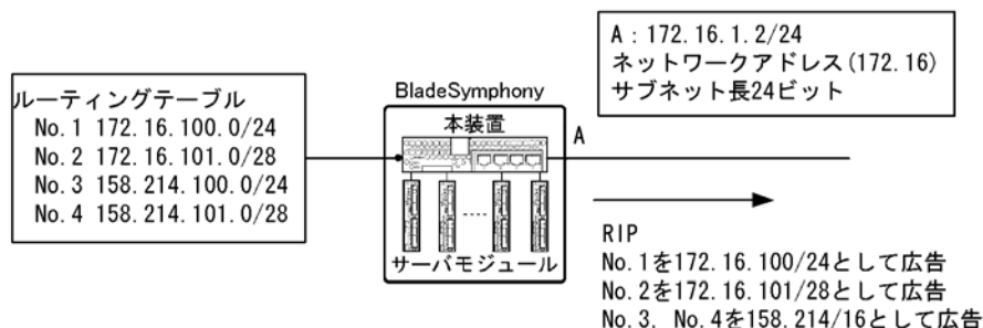
図 8-7 RIP-2 使用時の広告経路自動集約化
