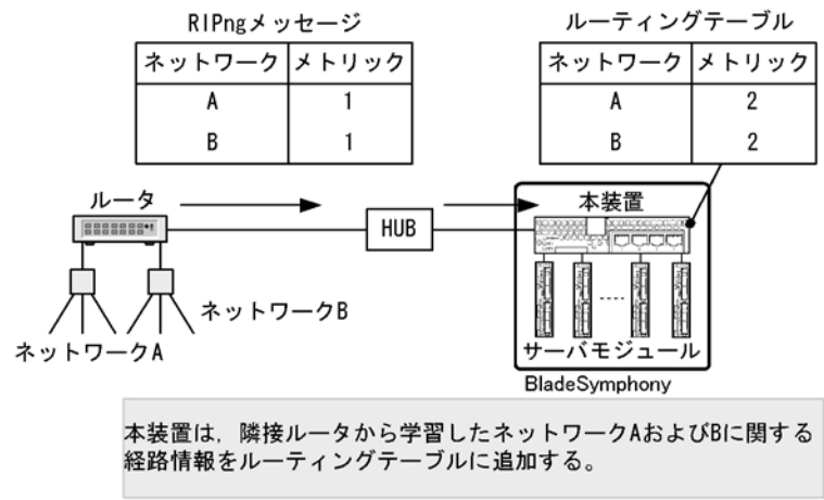
図 23-6 レスポンスパケット受信による経路情報の生成
