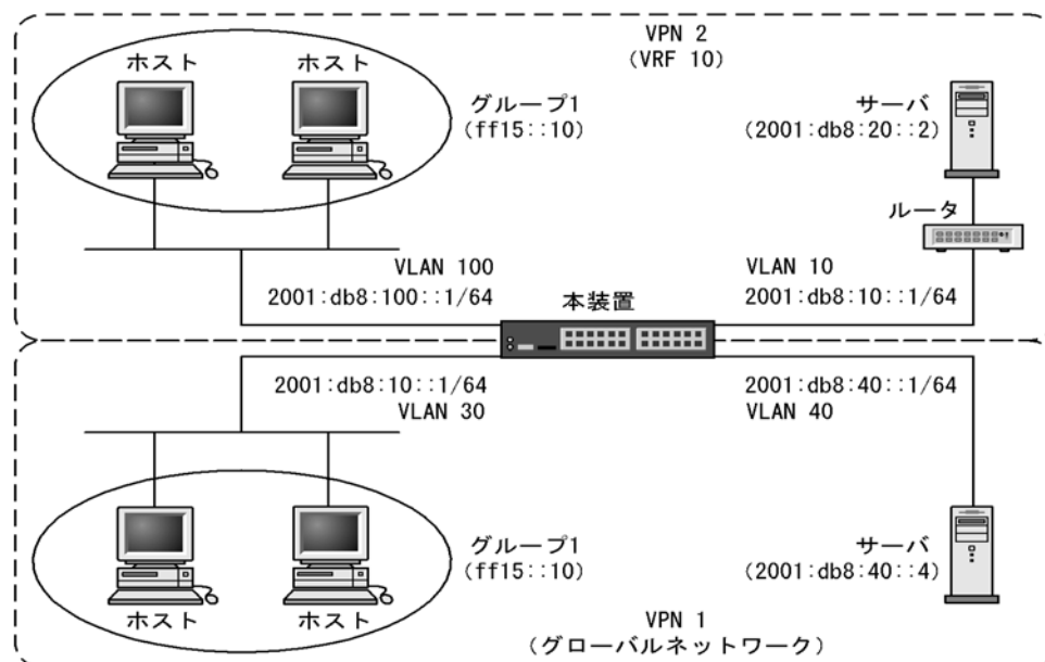
図 29-4 VRF での MLD 構成例
