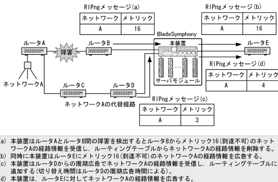
図 23-5 ルートポイズニング期間中の再学習
