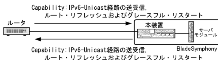
図 26-13 ネゴシエーションの動作概念
