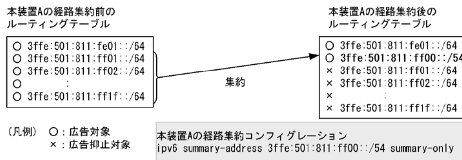
図 21-8 経路集約のコンフィグレーション例と経路集約前後の経路
