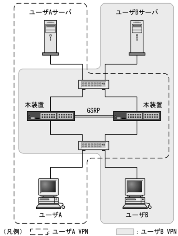
図 31-8 GSRP を使用したネットワーク・パーティション
