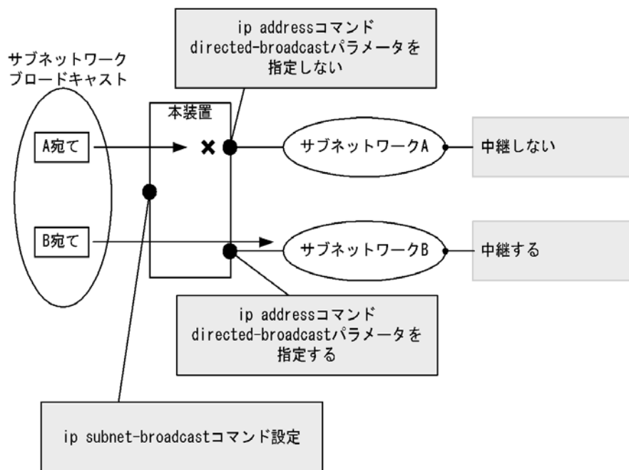
図 1-5 コマンド設定例
