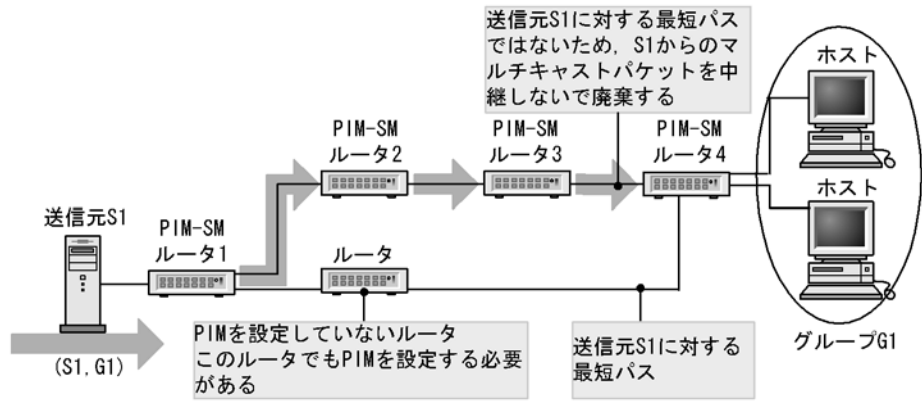
図 28-17 冗長経路時の注意事項
