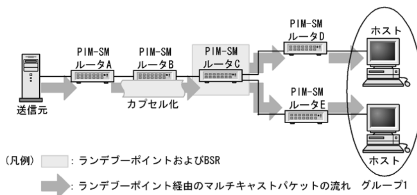
図 28-9 IPv6 マルチキャストパケット通信（カプセル化）
