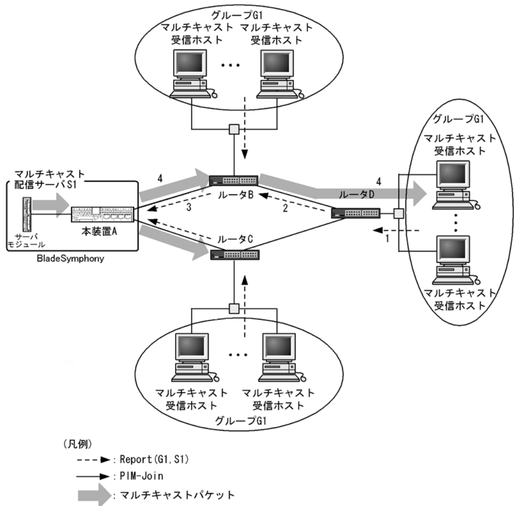
図 28-19 MLDv2 使用時の IPv6 PIM-SSM 動作概要
