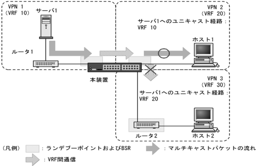
図 13-23 IPv4 マルチキャストエクストラネット使用時に装置内で VRF 中継を禁止している例
