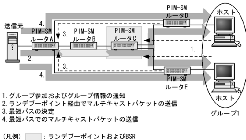
図 28-6 PIM-SM の動作概要
