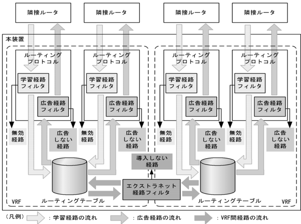
図 12-2 エクストラネットの経路フィルタリングの概念図
