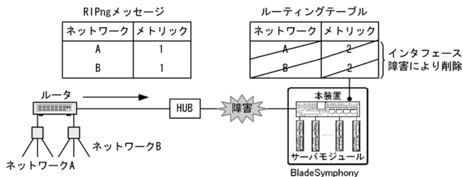
図 23-8 インタフェース障害による経路情報の削除
