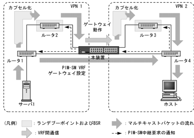
図 13-22 PIM-SM VRF ゲートウェイの動作概要
