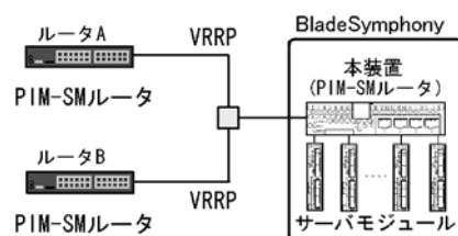
図 28-29 注意が必要な構成（VRRP を設定した場合）
