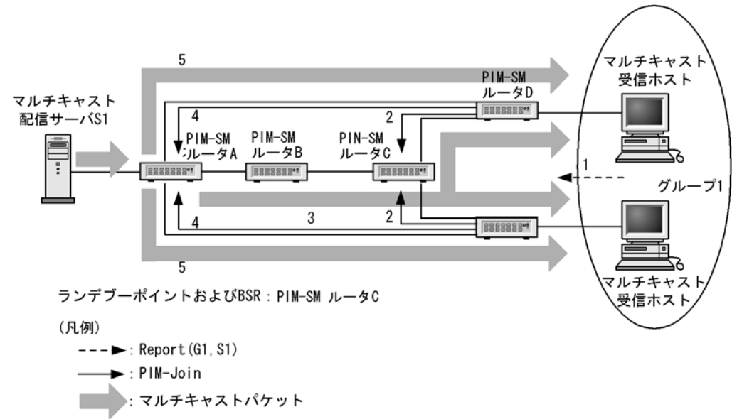
図 28-16 MLDv2 使用時の IPv6 PIM-SM 動作概要
