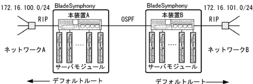
図 6-6 デフォルトルートの広告の例
