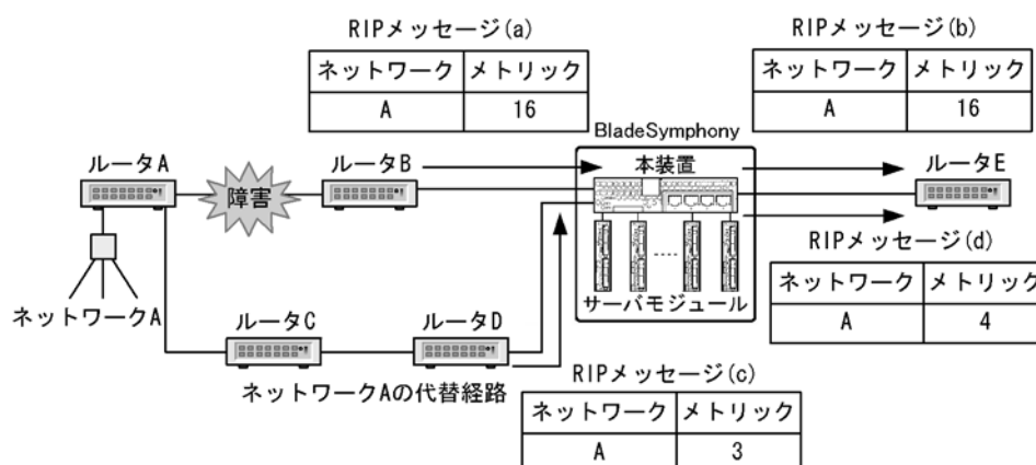
図 8-5 ルートポイズニング期間中の再学習
