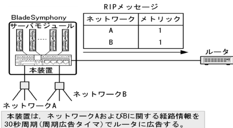
図 8-1 周期的な経路情報広告
