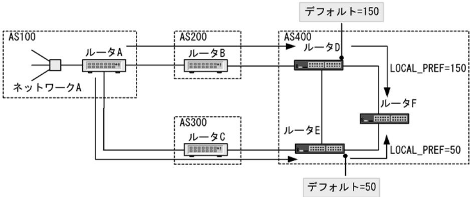
図 26-2 LOCAL_PREF 属性による経路選択
