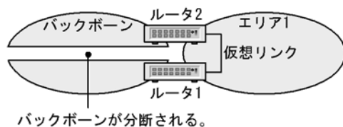
図 25-4 バックボーン分断に対する予備経路
