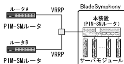
図 13-27 PIM-SSM を使用する構成図
