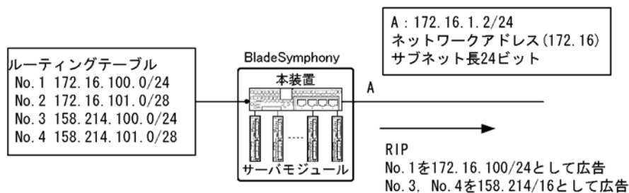
図 8-6 RIP-1 使用時の広告経路自動集約化
