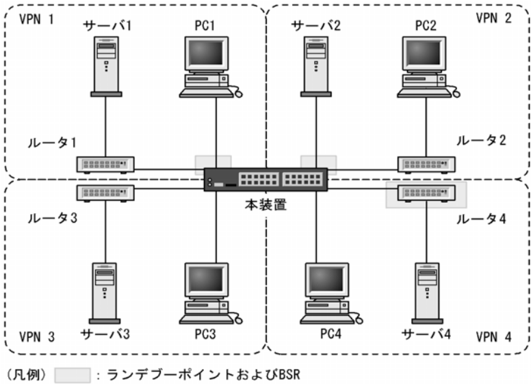
図 28-20 VRF での IPv6 マルチキャスト
