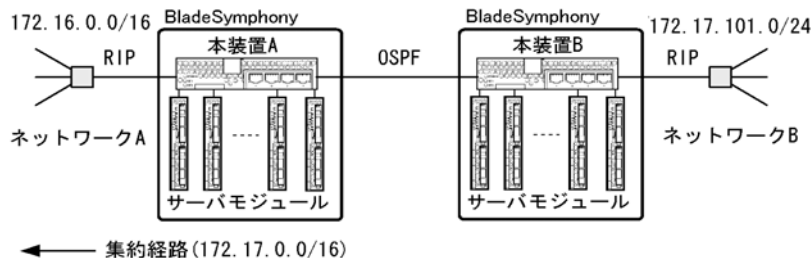
図 6-7 集約経路の広告の例
