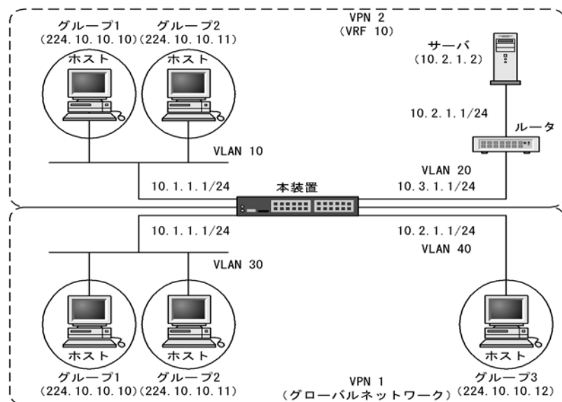
図 14-7 VRF での PIM-SM 構成例 (PIM-SM VRF ゲートウェイ)
