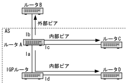
図 26-7 通知する経路情報のネクストホップの設定例
