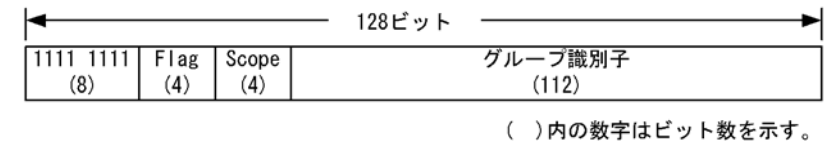
図 16-15 IPv6 マルチキャストアドレス
