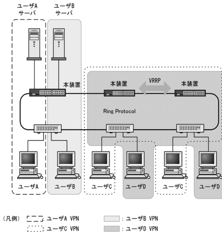
図 31-4 レイヤ 3 集約装置の増設
