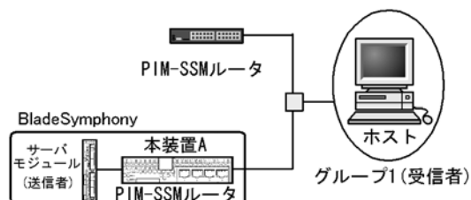
図 13-33 注意が必要な構成（複数ルータとホストの接続）
