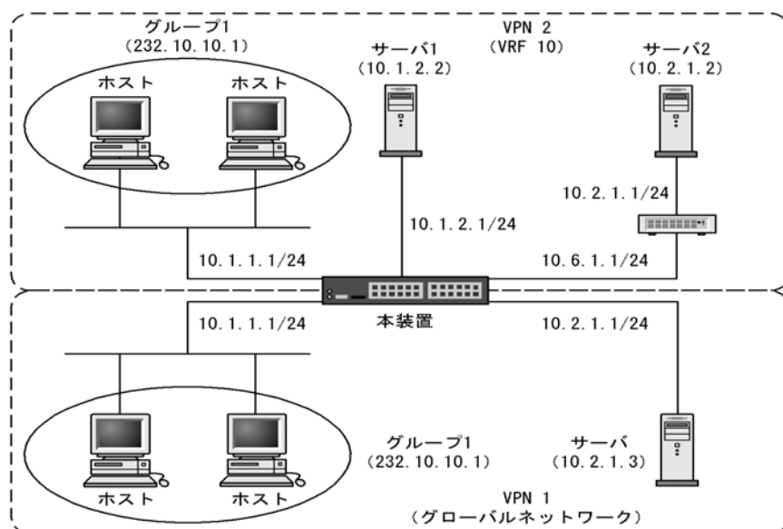
図 14-4 VRF での IPv4 PIM-SSM 構成例
