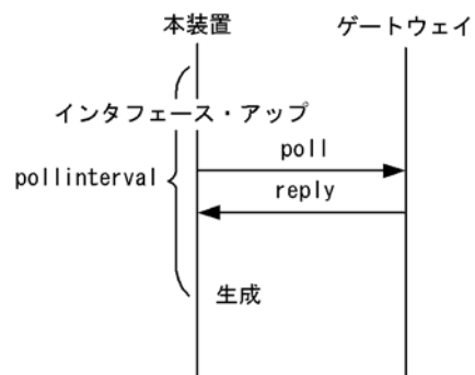
図 22-3 スタティック経路の動的監視による経路生成
