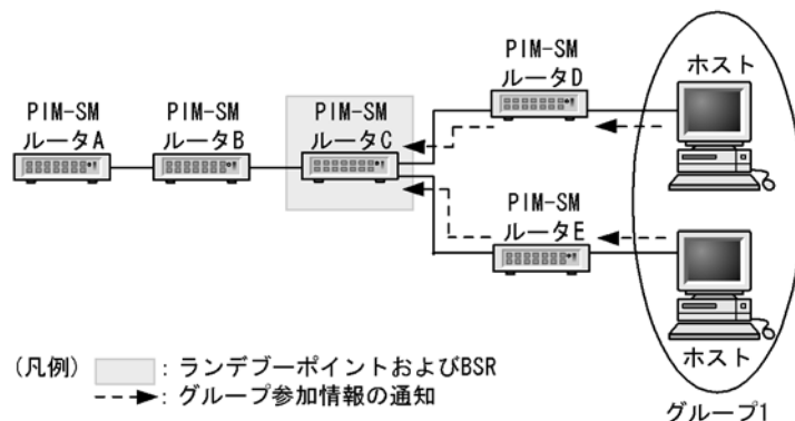
図 28-8 ランデブーポイントへのグループ参加情報の通知
