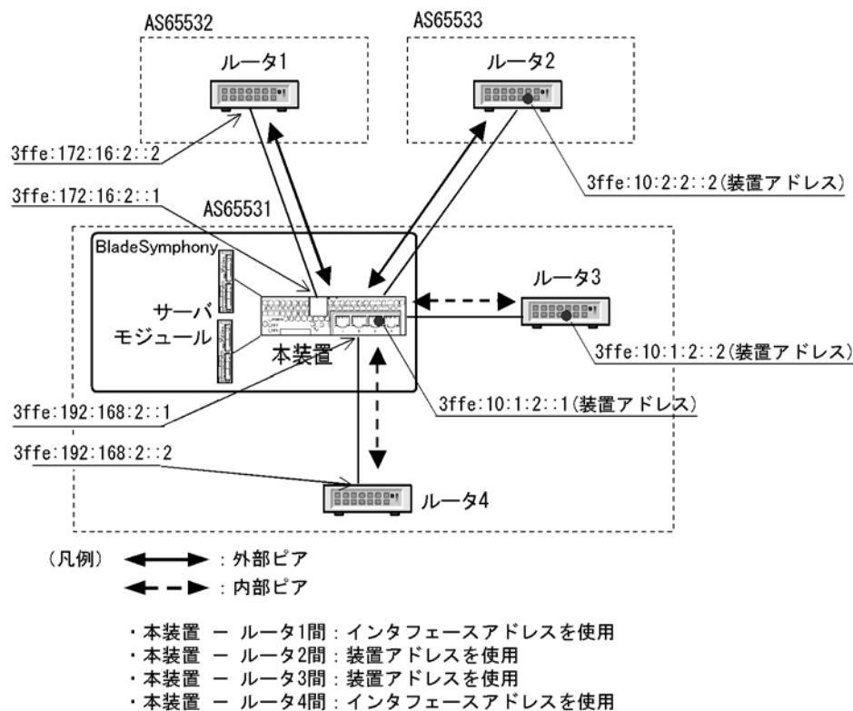
図 26-8 接続構成例
