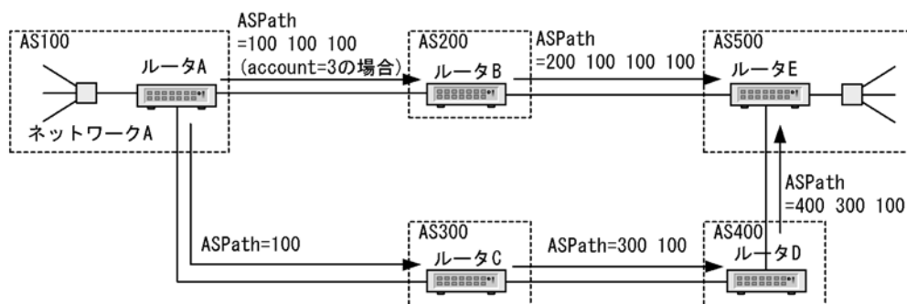
図 26-4 set as-path prepend count コマンドの使用例
