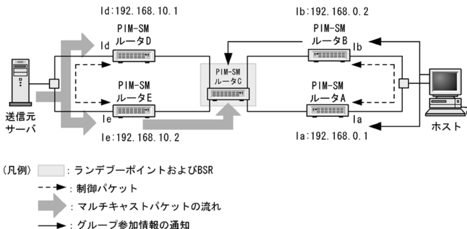
図 13-15 DR の動作
