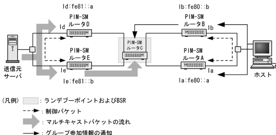
図 28-15 DR の動作
