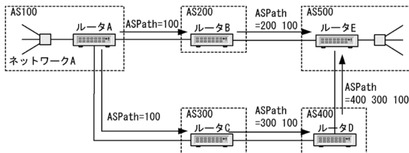
図 26-3 AS_PATH 属性による経路選択
