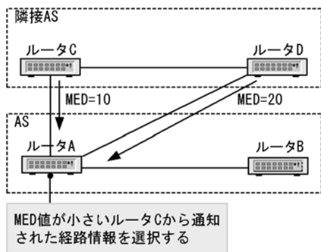
図 11-5 MED 属性による経路選択
