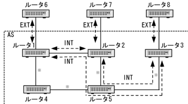
図 11-1 内部ピアと外部ピア
