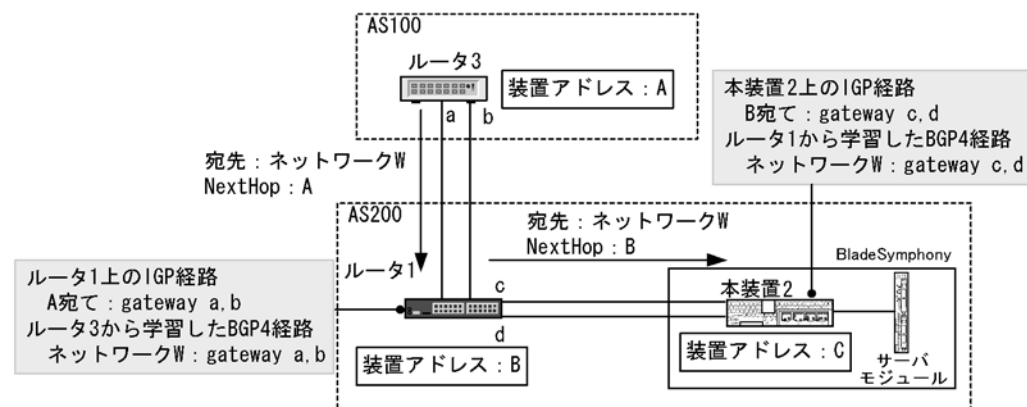
図 11-15 IGP 経路のマルチパス化による BGP4 経路マルチパス化の概念
