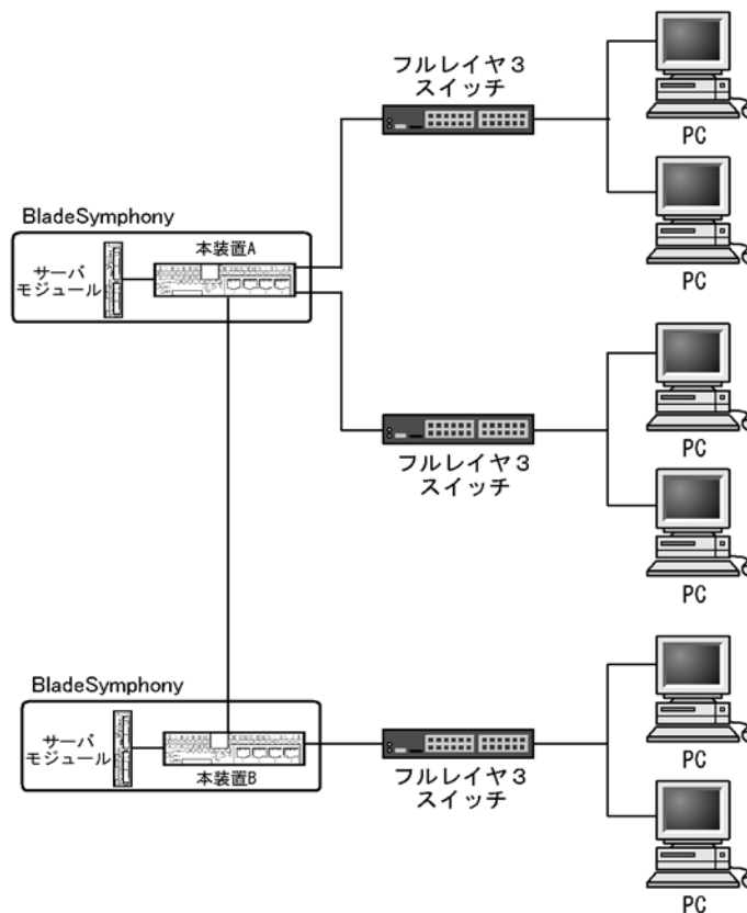
図 28-26 IPv6 PIM-SSM を使用する構成図
