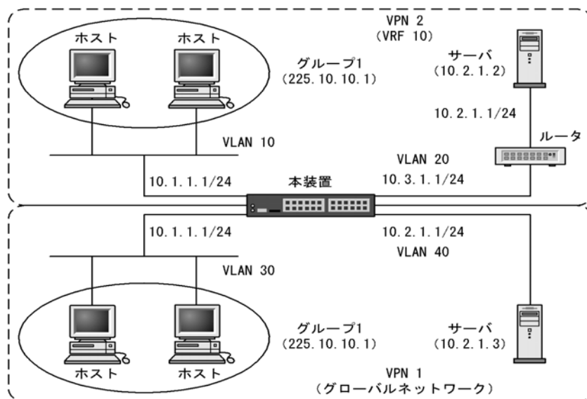
図 14-3 VRF での IPv4 PIM-SM 構成例
