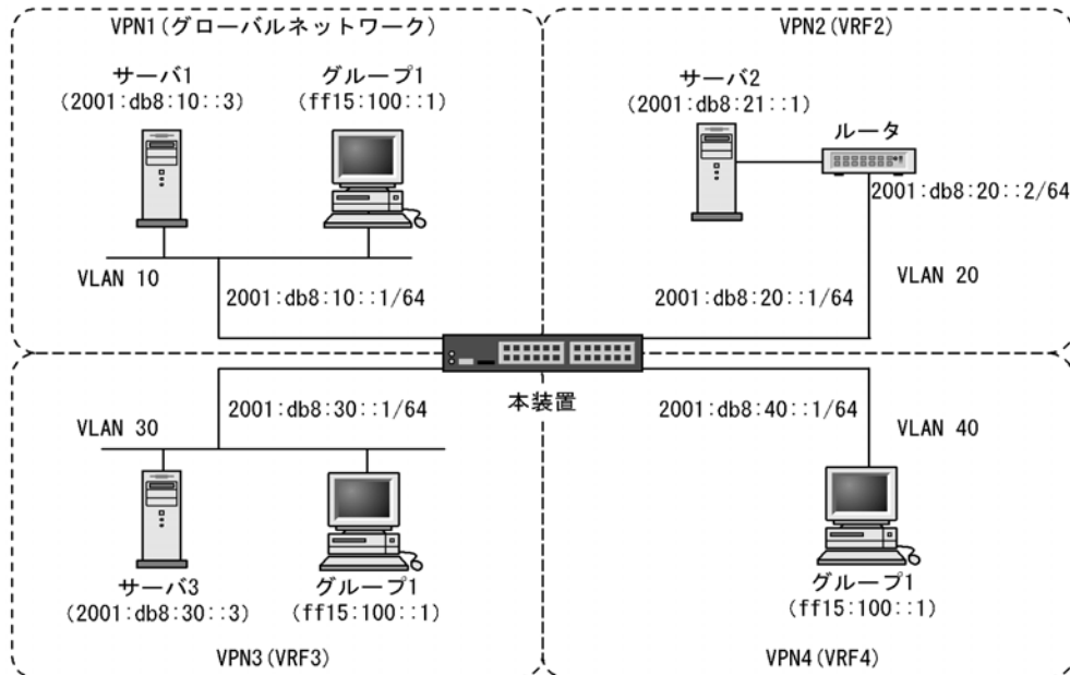
図 30-2 IPv6 マルチキャストエクストラネットの構成例
