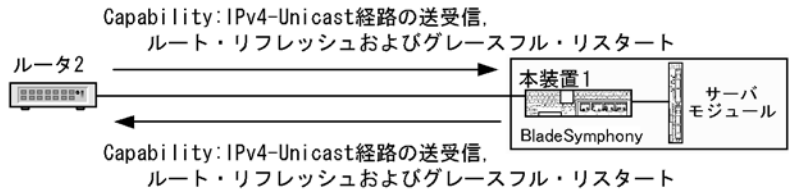
図 11-18 ルート・リフレッシュ機能の動作概念
