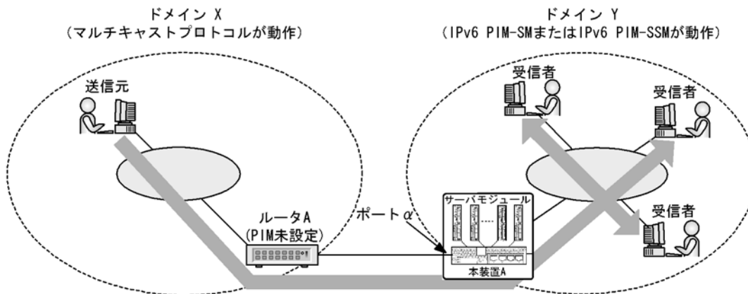
図 28-27 IPv6 上流ポートを指定する場合の適応例
