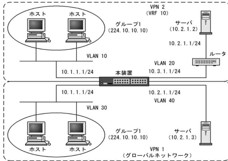
図 14-6 VRF での PIM-SSM 構成例 (IPv4 マルチキャストエクストラネット)
