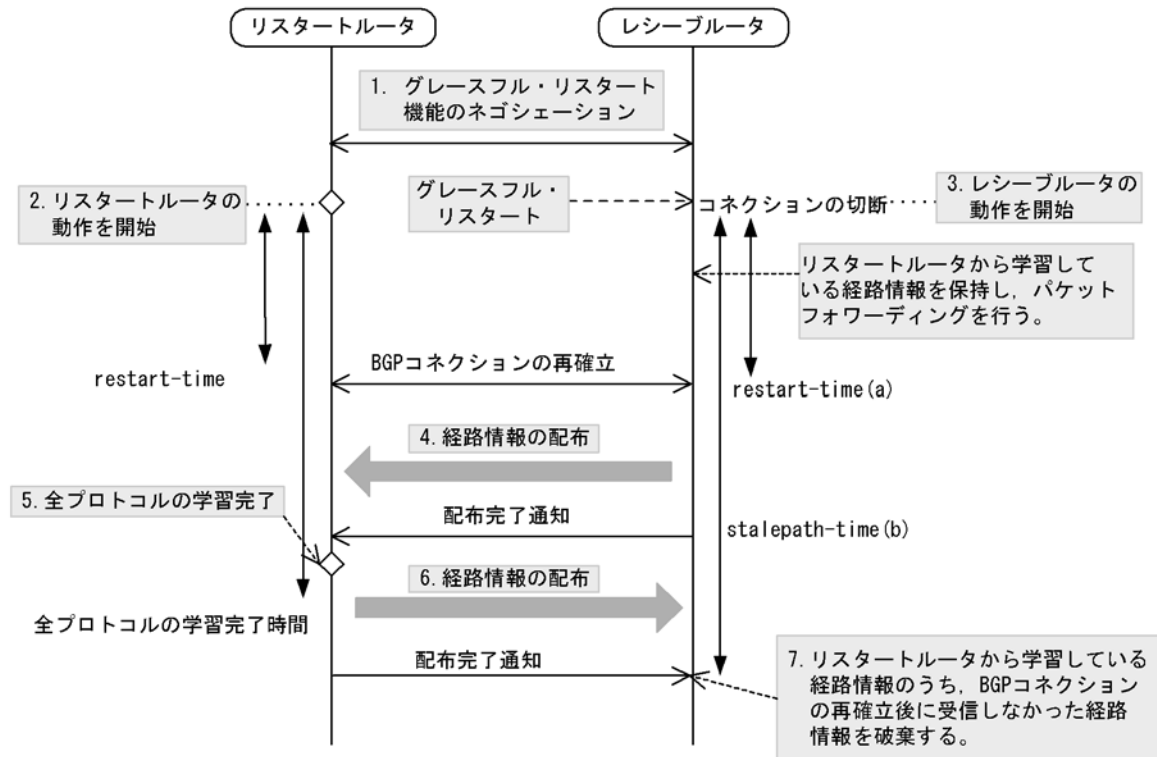
図 11-27 グレースフル・リスタートのシーケンス
