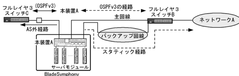
図 24-4 バックアップ回線を使用した構成での AS 外経路の導入例
