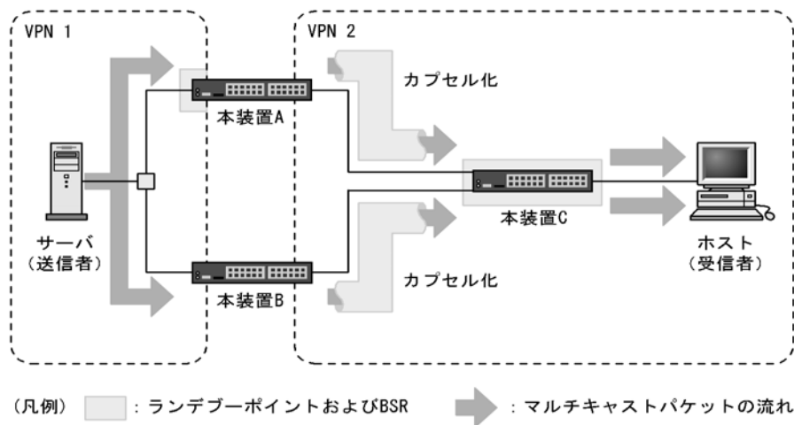
図 13-34 注意が必要な構成（2 台以上の VRF 境界ルータで冗長構成を構築する場合）
