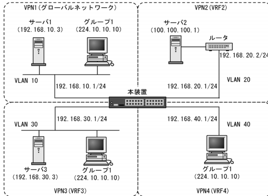
図 15-2 IPv4 マルチキャストエクストラネットの構成例
