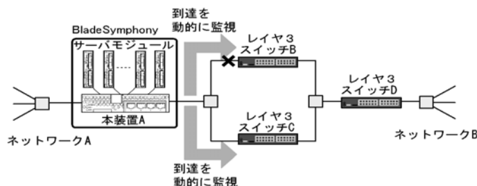
図 7-2 スタティック経路の動的監視の例
