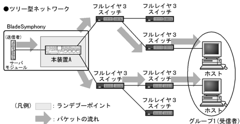
図 13-28 PIM-SM 推奨ネットワーク構成
