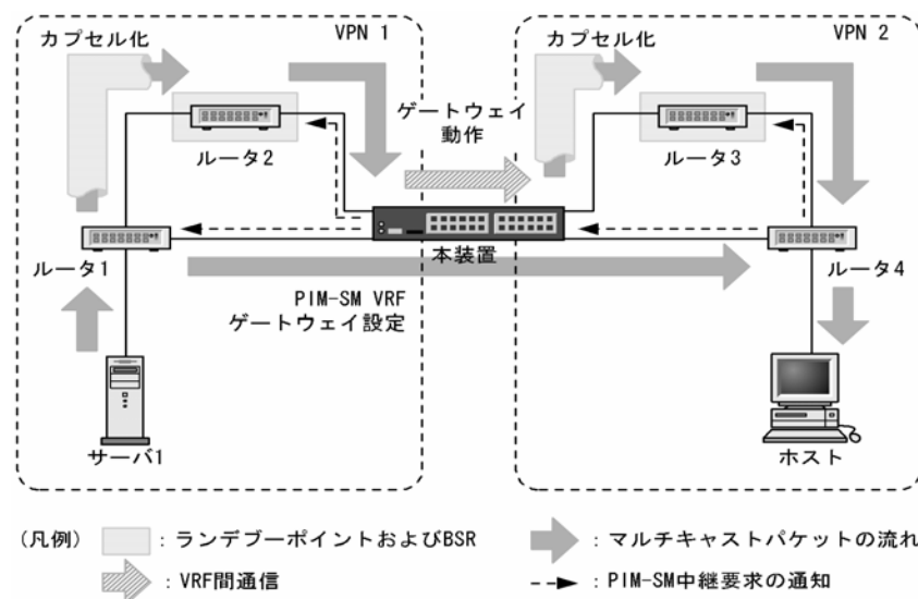
図 28-22 PIM-SM VRF ゲートウェイの動作概要
