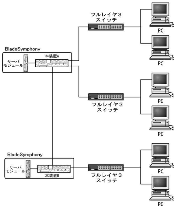
図 13-26 PIM-SSM を使用する構成図
