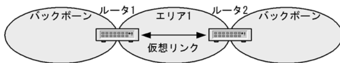
図 25-3 バックボーン間の接続
