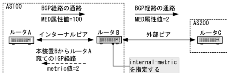
図 11-6 set metric-type internal の使用例
