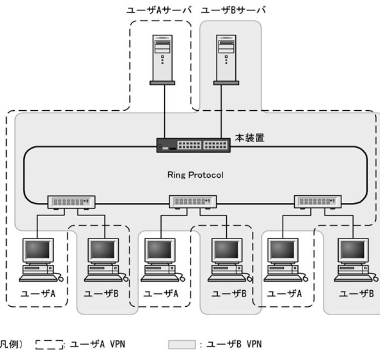
図 31-3 Ring Protocol を使用したネットワーク・パーティション
