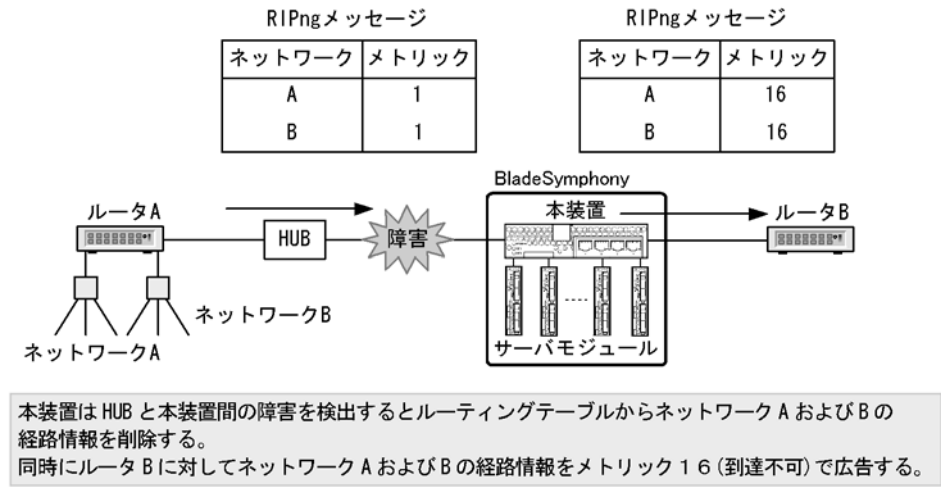
図 23-2 triggered update による経路情報の広告
