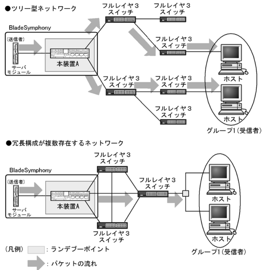
図 28-32 IPv6 PIM-SM 推奨ネットワーク構成
