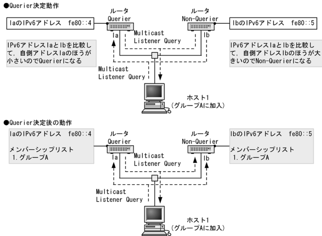
図 28-4 Querier と Non-Querier の決定
