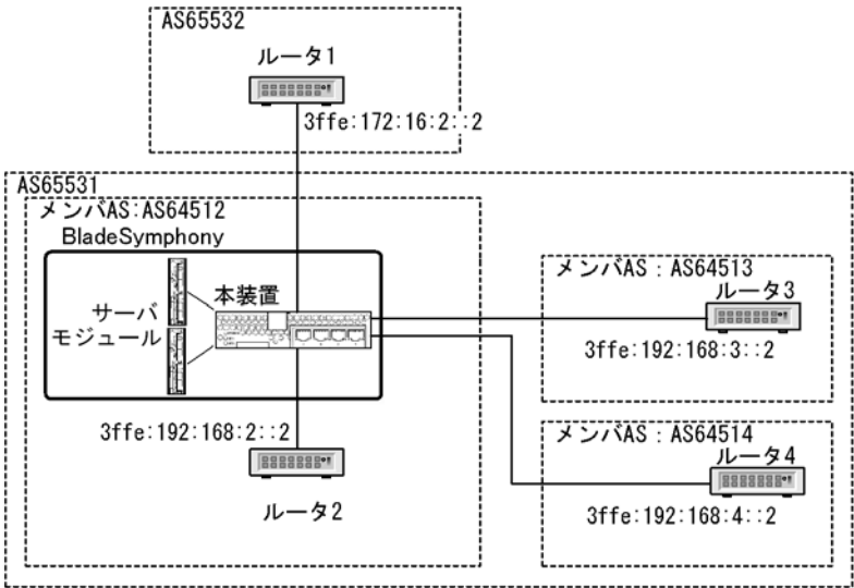
図 26-16 コンフェデレーション構成例
