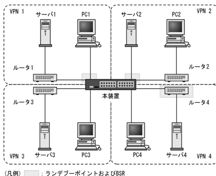
図 13-20 VRF での IPv4 マルチキャスト
