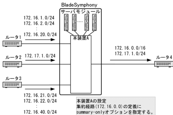
図 6-16 集約元経路の広告抑止の適用例
