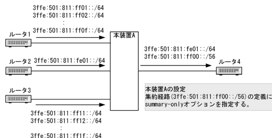
図 21-7 集約元経路の広告抑止の適用例
