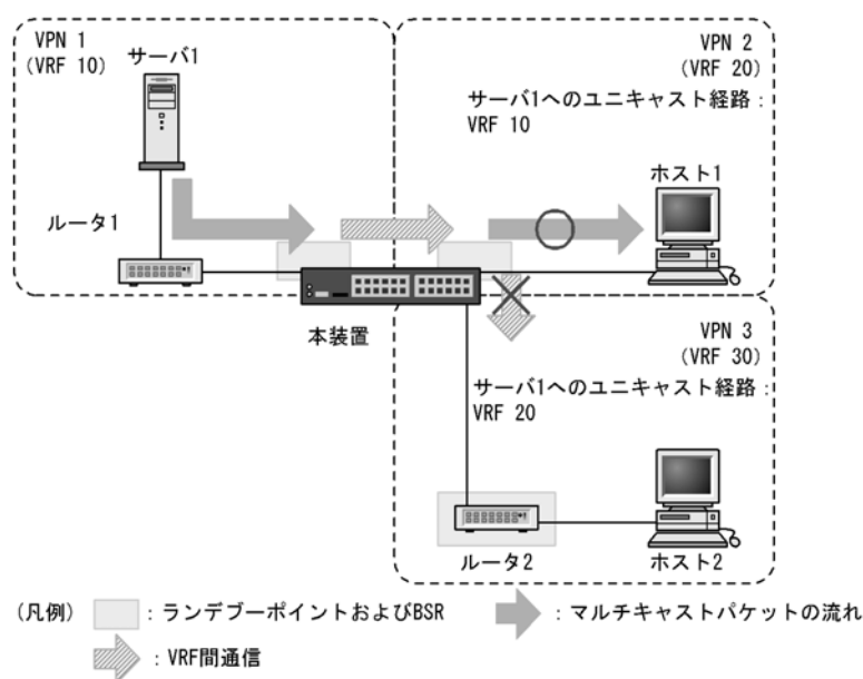
図 28-23 IPv6 マルチキャストエクストラネット使用時に装置内で VRF 中継を禁止している例
