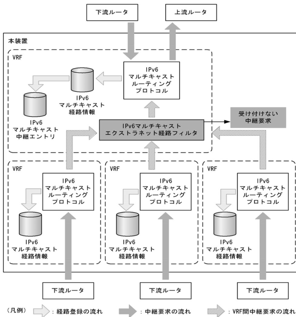
図 30-1 IPv6 マルチキャストエクストラネットの経路フィルタリングの概念図
