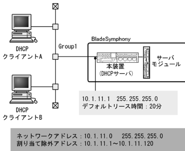
図 5-1 クライアントーサーバ構成（動的 IP アドレス配布時）
