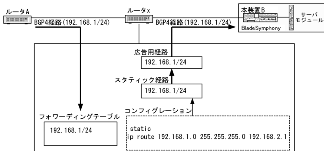
図 11-19 広告用経路生成と広告
