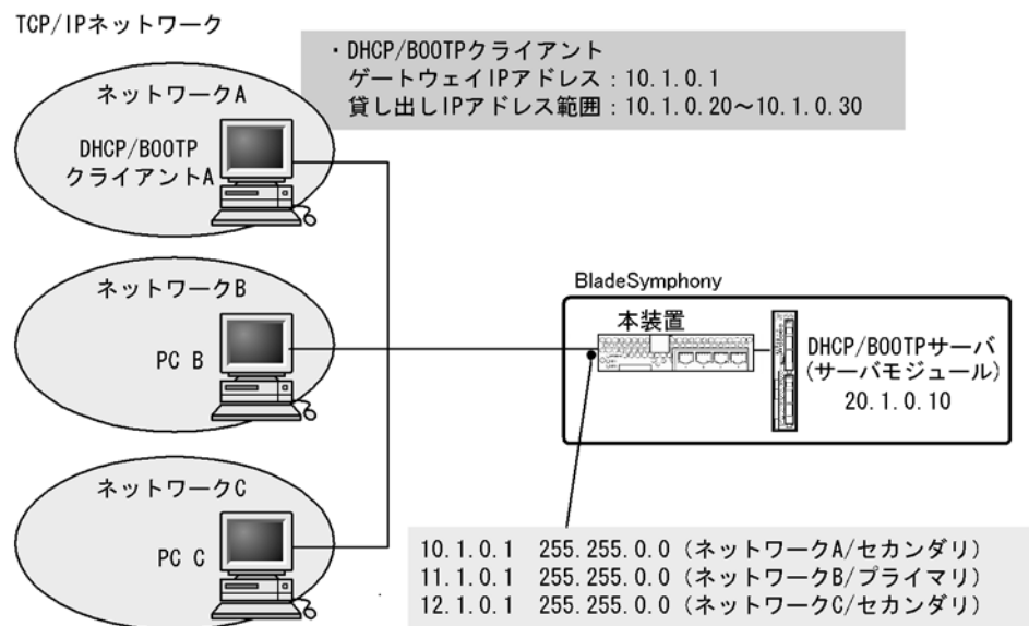
図 4-2 マルチホーム構成
