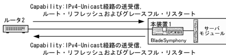
図 11-17 ネゴシエーションの動作概念
