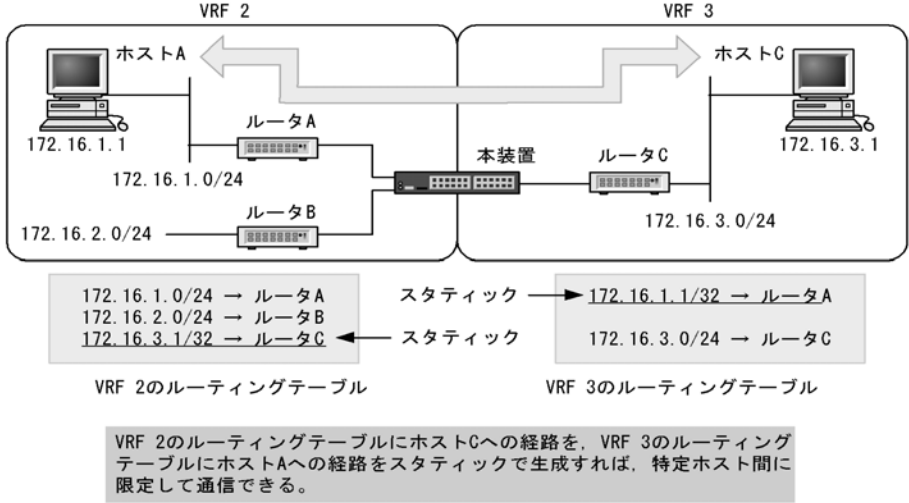
図 6-24 VRF 間にわたるスタティックルーティング
