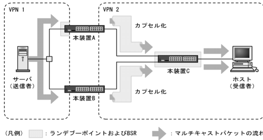
図 28-38 注意が必要な構成（2 台以上の VRF 境界ルータで冗長構成を構築する場合）
