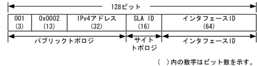
図 16-14 6to4 アドレス
