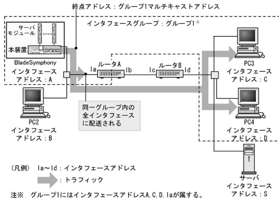
図 16-3 マルチキャストアドレス通信
