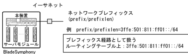
図 21-3 直結経路の取り扱い（ブロードキャスト型の場合）
