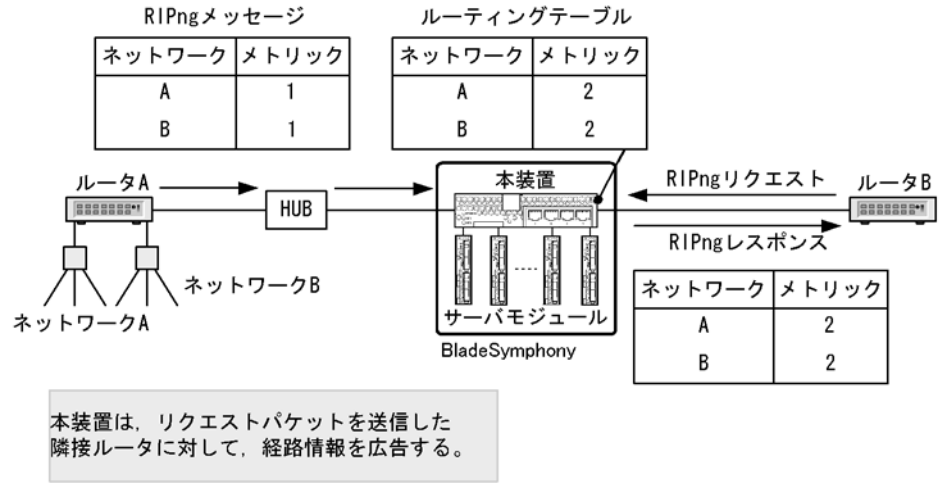
図 23-3 リクエストパケット受信による経路情報の広告
