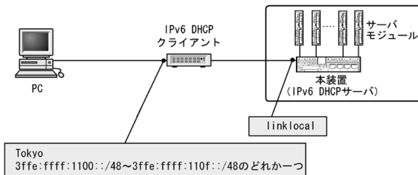
図 20-2 動的にプレフィックスを割り当てる構成
