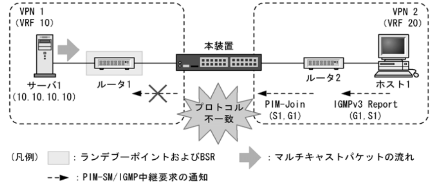
図 13-24 IPv4 マルチキャストエクストラネット使用時に VRF 間プロトコル不一致で中継できない例
