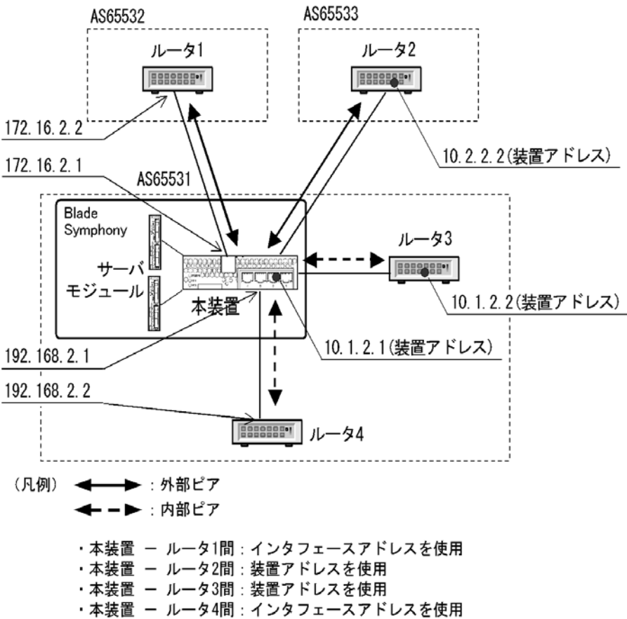
図 11-8 接続構成例
