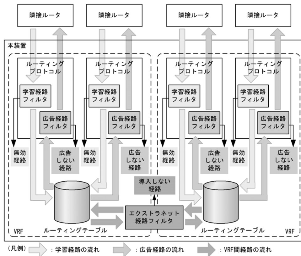
図 27-2 エクストラネットの経路フィルタリングの概念図
