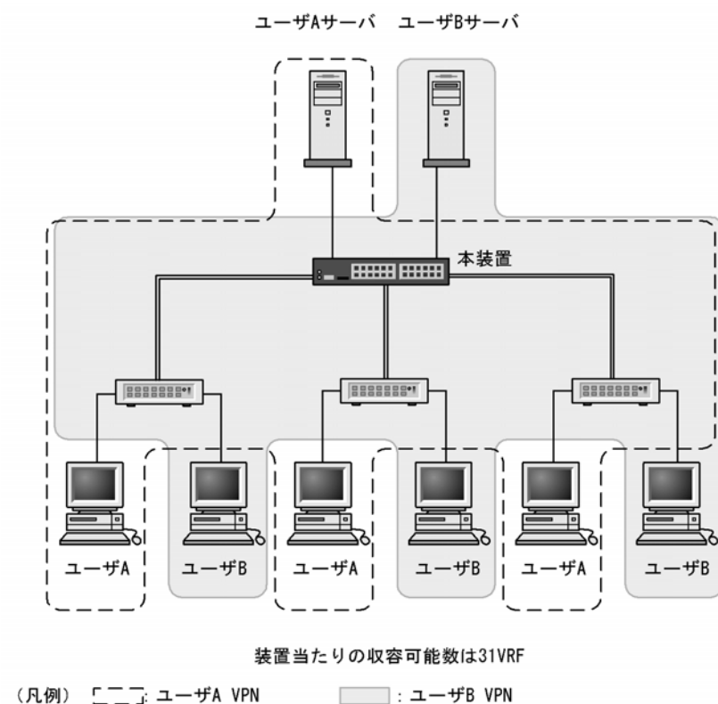
図 31-5 レイヤ 2 プロトコルを使用しない構築
