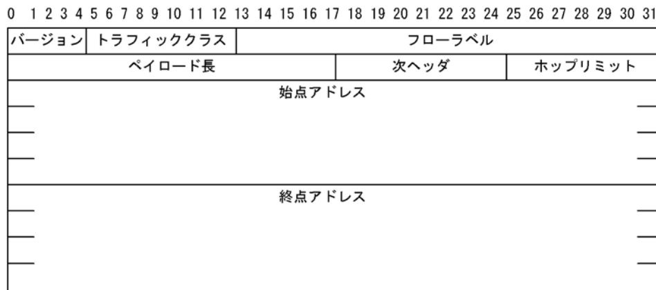
図 16-19 IPv6 ヘッダ形式
