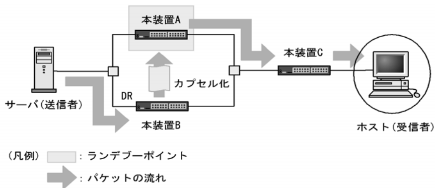
図 13-29 注意が必要な構成（複数ルータと送信者の接続）
