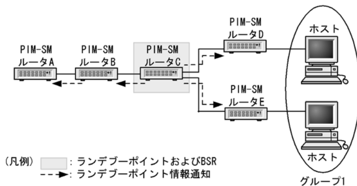
図 28-7 ランデブーポイントおよびブートストラップルータ（BSR）
