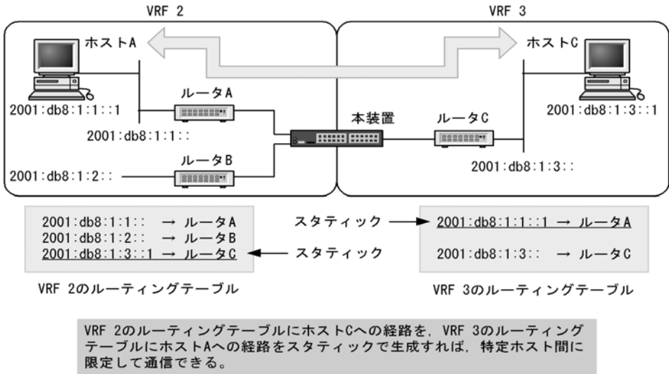
図 21-14 VRF 間にわたるスタティックルーティング
