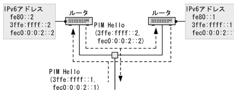
図 28-13 PIM Hello メッセージによる隣接ルータアドレス受信
