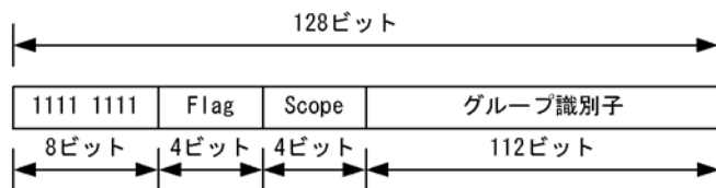
図 28-1 マルチキャストアドレスのフォーマット
