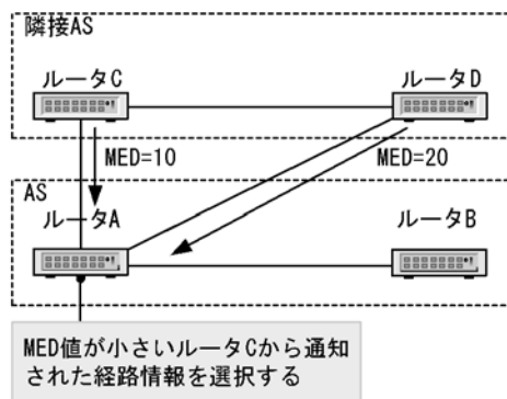
図 26-5 MED 属性による経路選択
