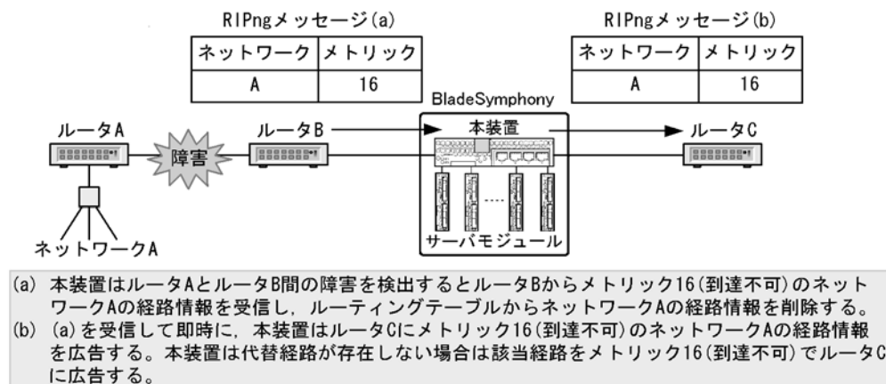
図 23-4 ルートポイズニング
