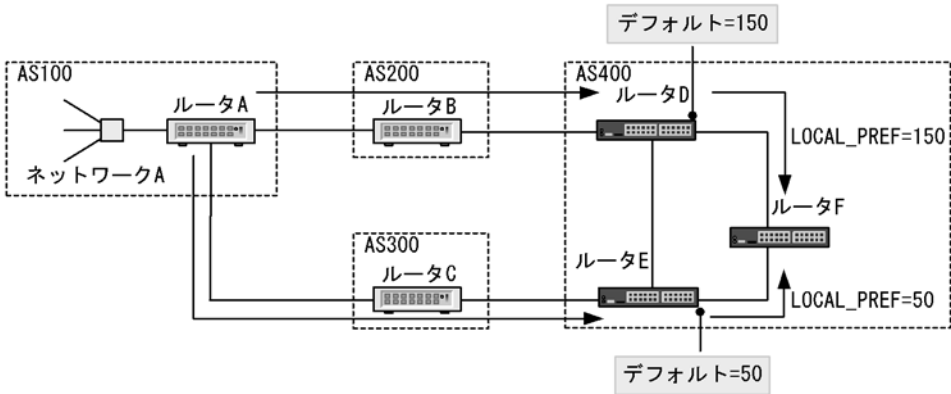
図 11-2 LOCAL_PREF 属性による経路選択
