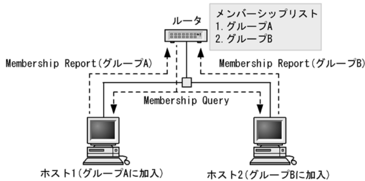
図 13-3 IGMPv2 グループの参加・離脱
