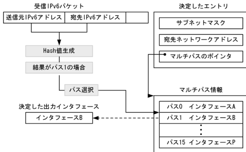
図 21-4 出カインタフェースの決定
