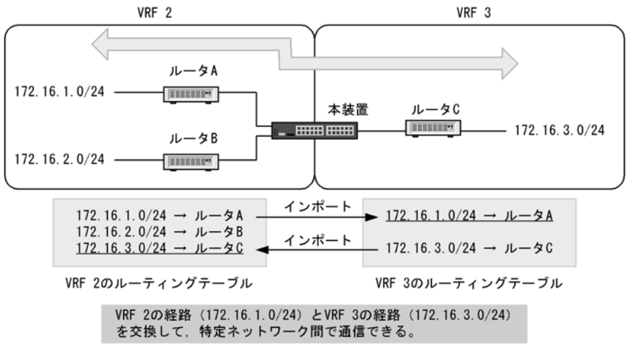
図 6-23 VRF 間の経路交換
