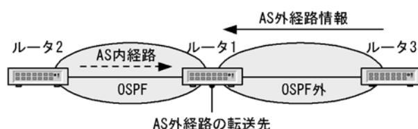
図 9-4 システム構成例（AS 境界ルータを目標とする場合）
