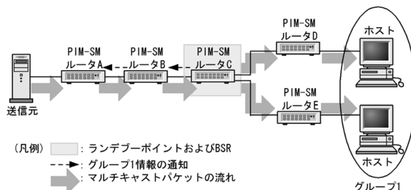
図 28-10 IPv6 マルチキャストパケット通信（デカプセル化）
