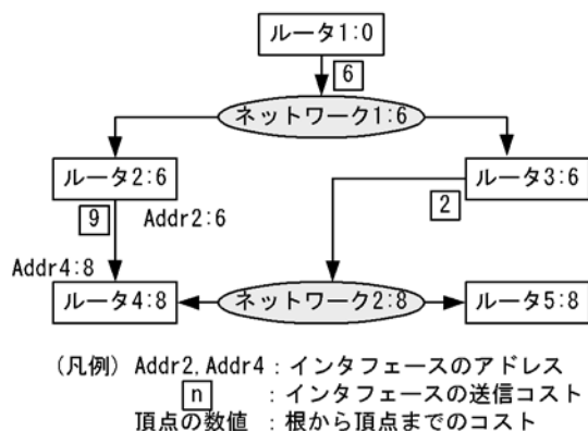
図 24-3 ルータ 1 を根とする最短木
