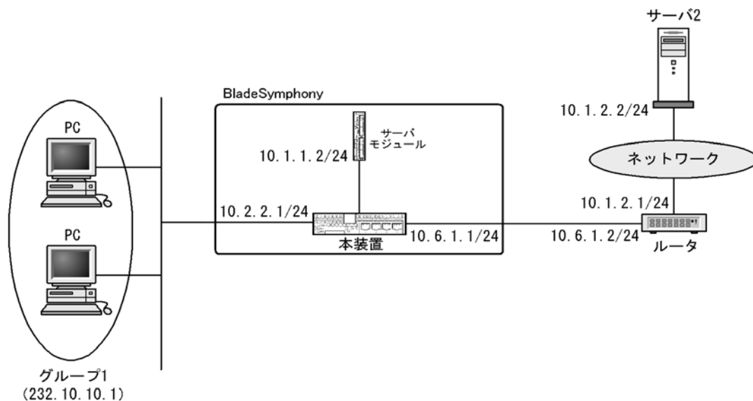
図 14-2 PIM-SSM 構成例
