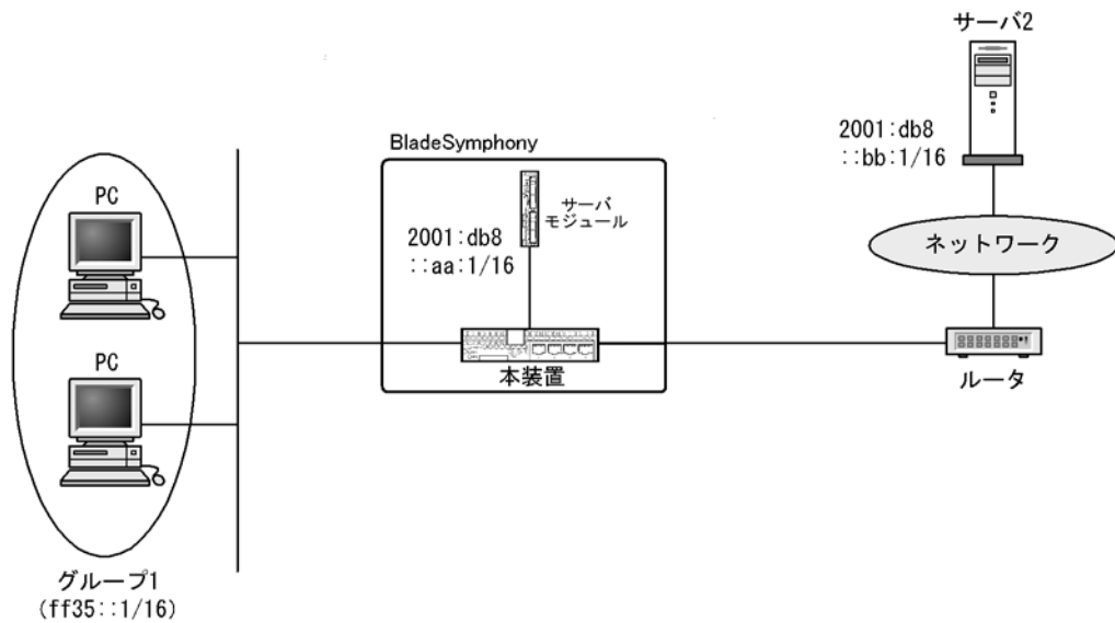
図 29-1 PIM-SSM 構成例
