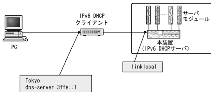
図 20-3 クライアントにオプション情報を配布する構成
