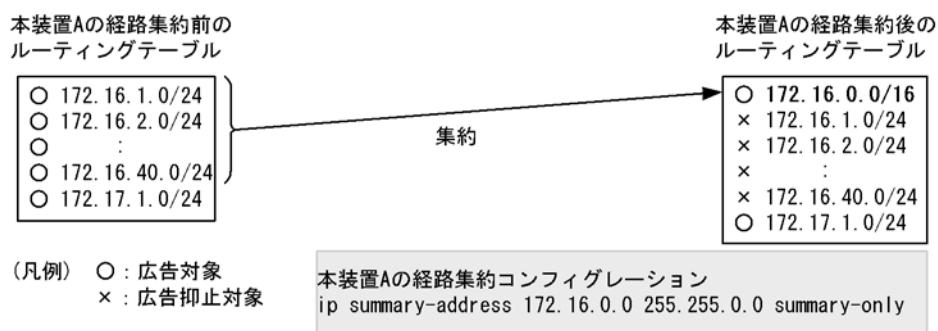
図 6-17 経路集約のコンフィグレーション例と経路集約前後の経路
