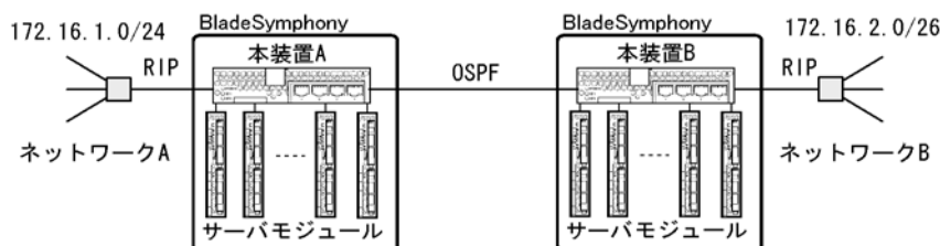
図 6-2 異なるサブネットマスク長のサブネット間の接続
