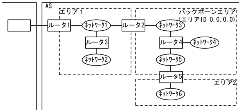
図 25-1 エリア分割を使用した OSPFv3 ネットワークトポロジの例
