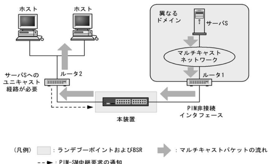
図 28-30 注意が必要な構成（PIM 非接続インタフェース経由の中継）
