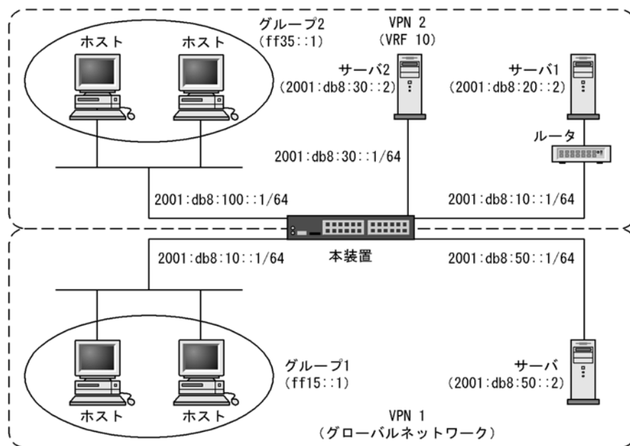
図 29-3 VRF での IPv6 PIM-SSM 構成例
