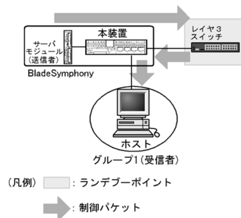
図 28-33 不適応な構成（送信者とランデブーポイントの間に受信者が存在する場合）
