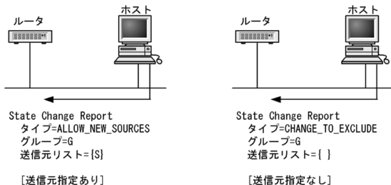
図 28-3 MLDv2 グループ参加・離脱動作
