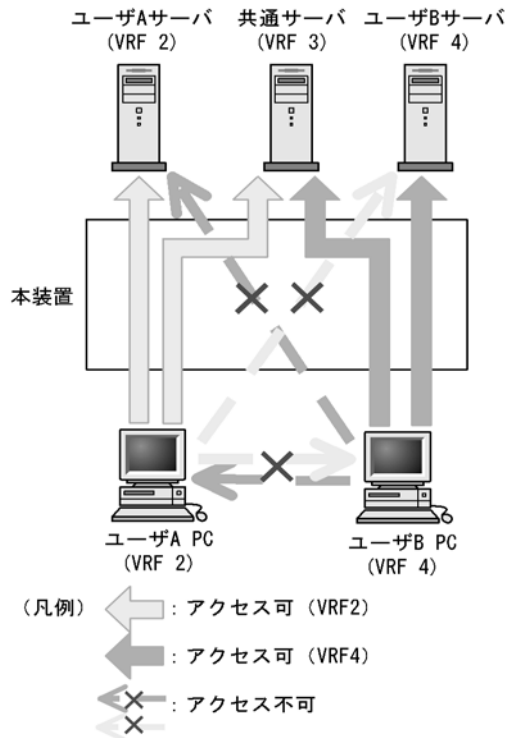
図 31-6 経路交換によるエクストラネット
