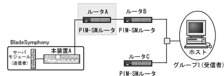
図 28-35 不適応な構成（ランデブーポイントに接続しないルータが存在する場合）
