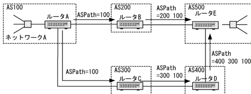
図 11-3 AS_PATH 属性による経路選択
