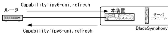
図 26-14 ルート・リフレッシュ機能の動作概念
