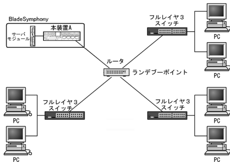
図 13-25 PIM-SM を使用する構成図
