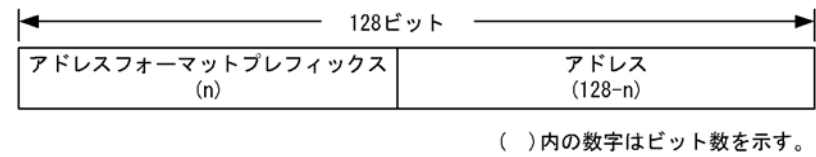
図 16-4 アドレスフォーマットプレフィックス
