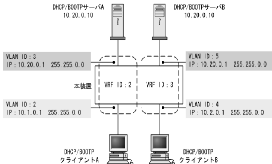
図 4-3 VRF 構成
