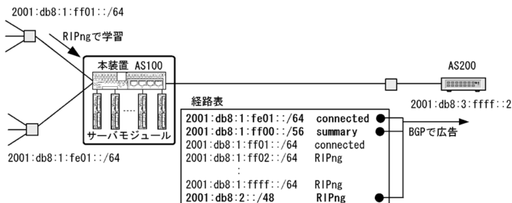
図 21-9 集約経路を BGP4+ で広告する構成
