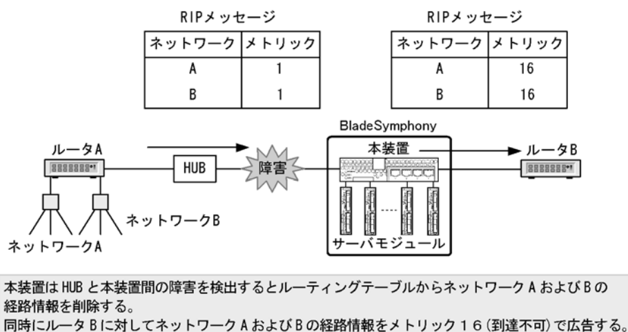
図 8-2 triggered update による経路情報の広告
