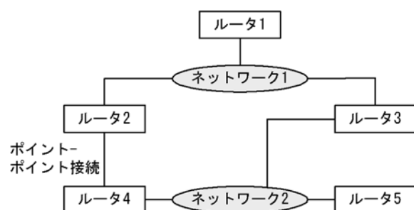
図 9-1 ネットワーク構成例
