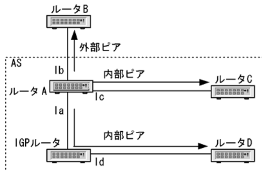
図 11-7 通知する経路情報の NEXT_HOP 属性の設定例
