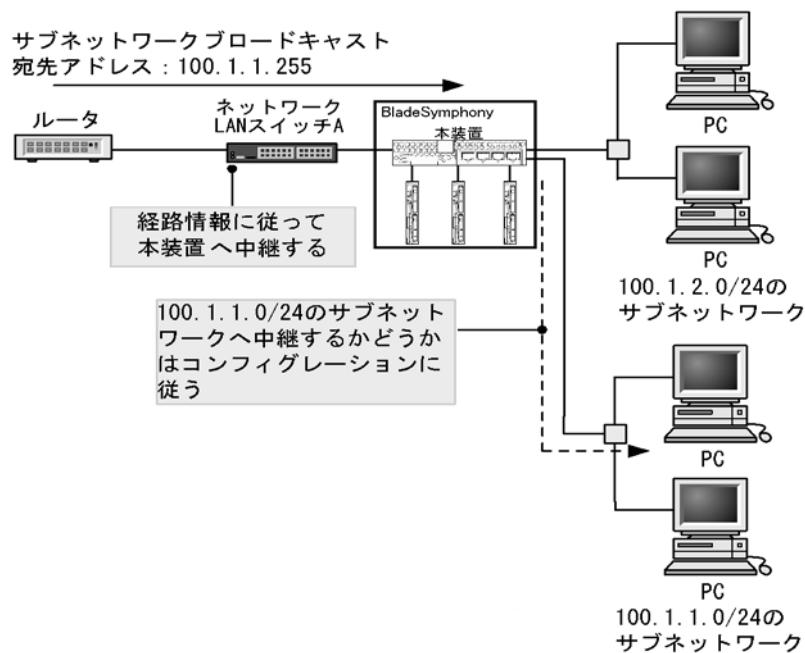
図 1-7 サブネットワークブロードキャスト
