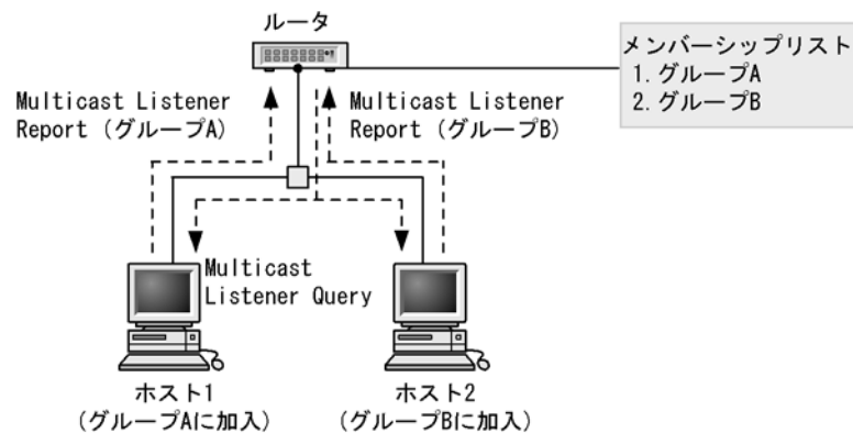
図 28-2 MLDv1 グループ参加・離脱動作
