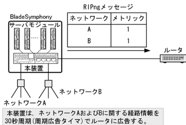
図 23-1 周期的な経路情報広告
