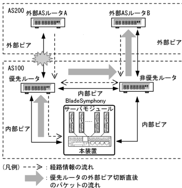
図 6-21 経路削除保留機能の適用例
