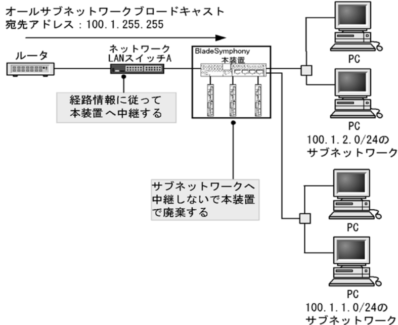
図 1-8 オールサブネットワークブロードキャスト
