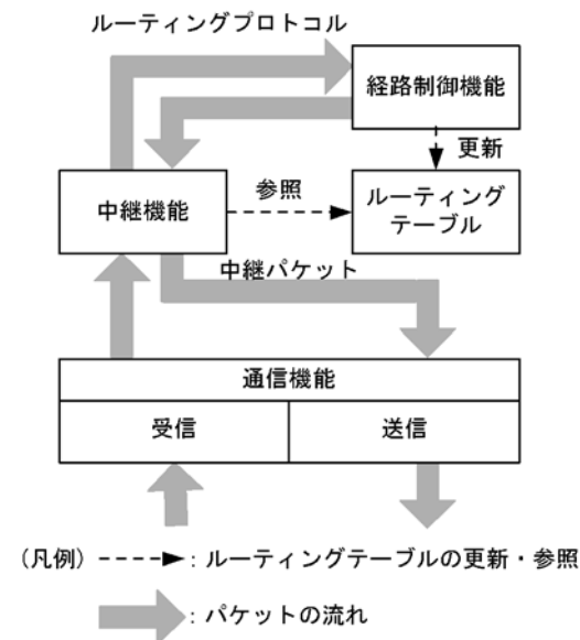
図 16-17 IPv6 ルーティング機能の概要
