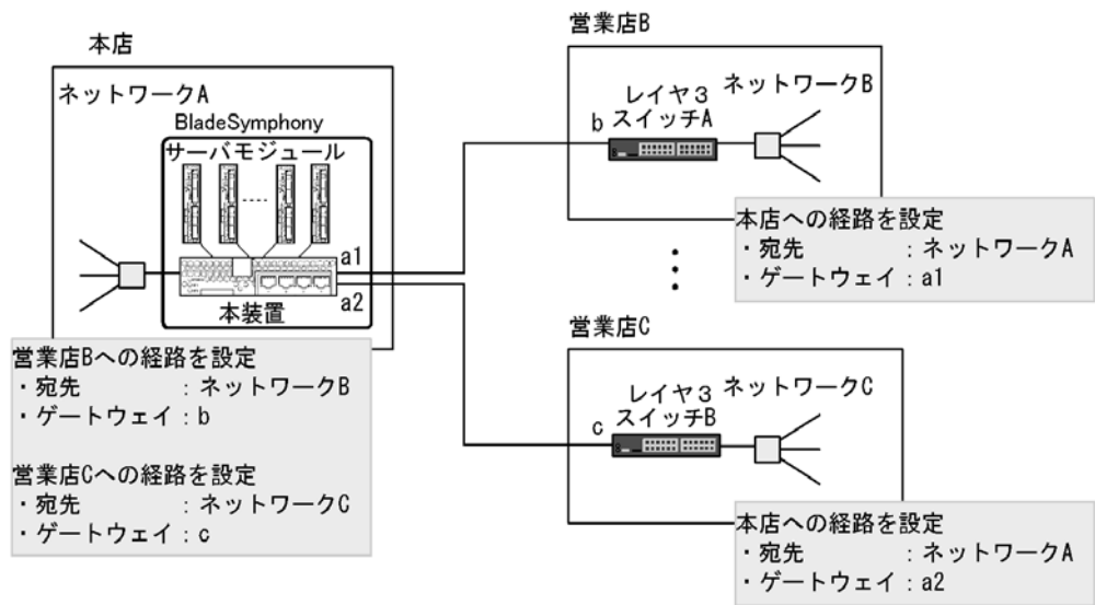
図 22-1 スタティックルーティングのネットワーク構成例
