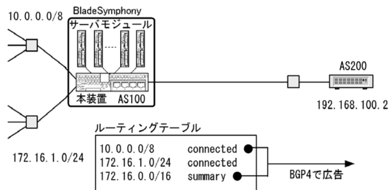
図 6-18 集約経路を BGP4 で広告する構成
