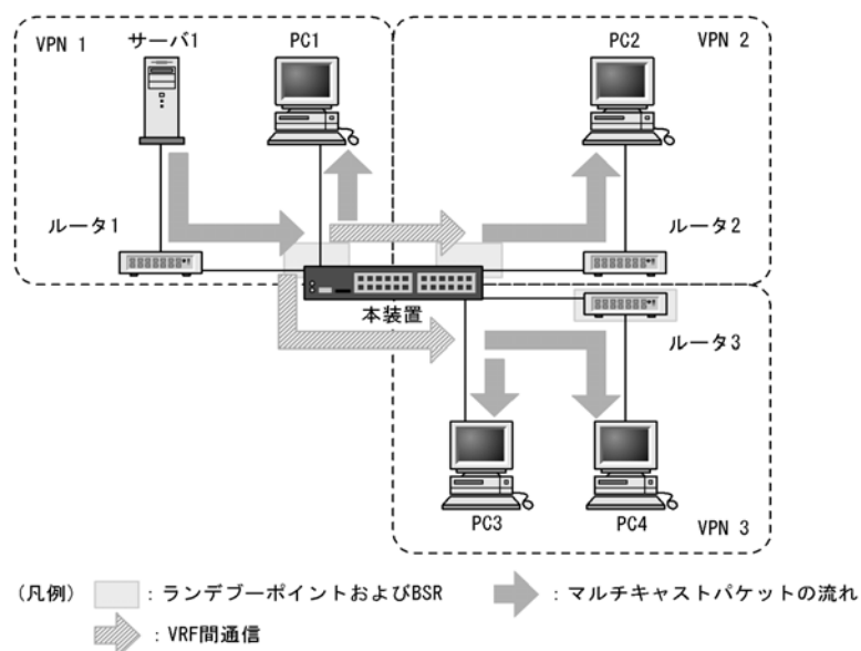
図 13-21 IPv4 マルチキャストエクストラネットの動作概要
