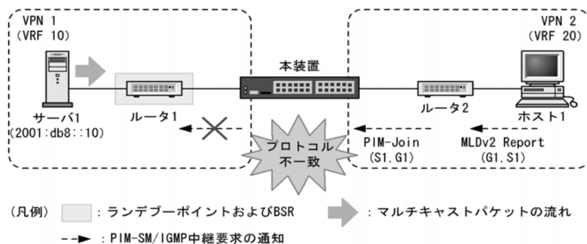
図 28-24 IPv6 マルチキャストエクストラネット使用時に VRF 間プロトコル不一致で中継できない例
