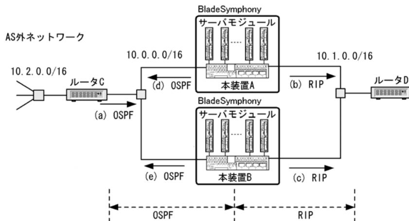
図 6-8 ネットワーク構成例
