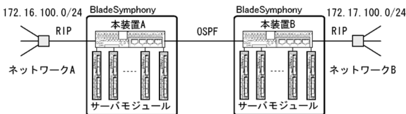
図 6-3 異なるネットワークアドレスのサブネット間の接続
