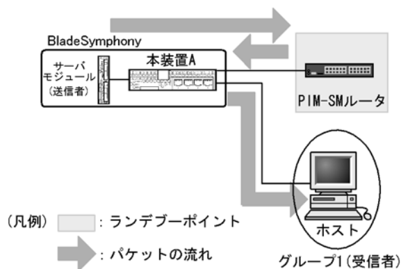
図 13-30 不適応な構成（送信者とランデブーポイントの間に受信者が存在する場合）
