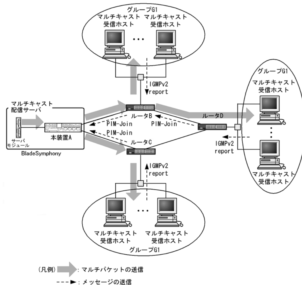
図 13-17 PIM-SSM の動作概要
