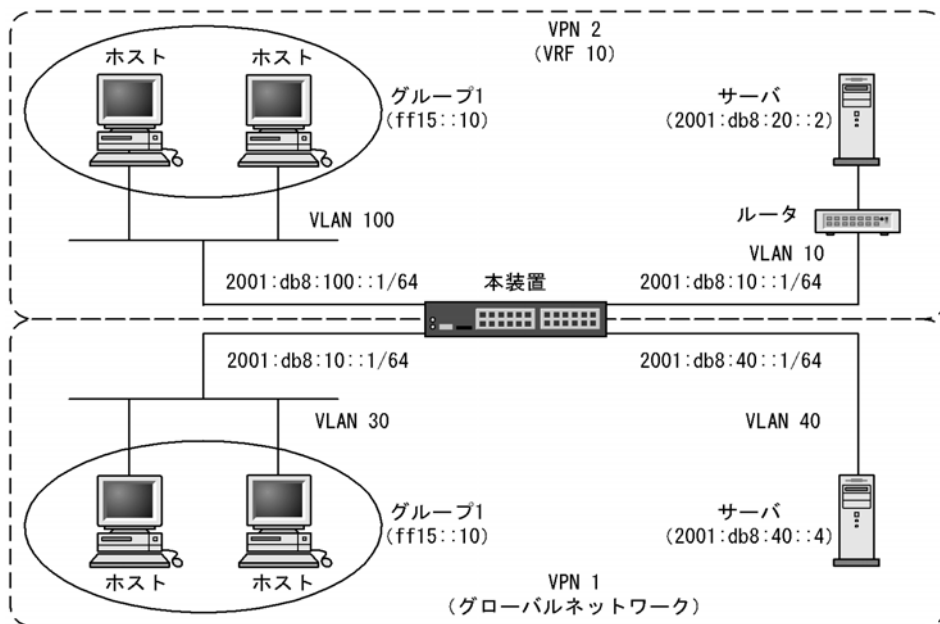
図 29-5 VRF での PIM-SSM 構成例（IPv6 マルチキャストエクストラネット）
