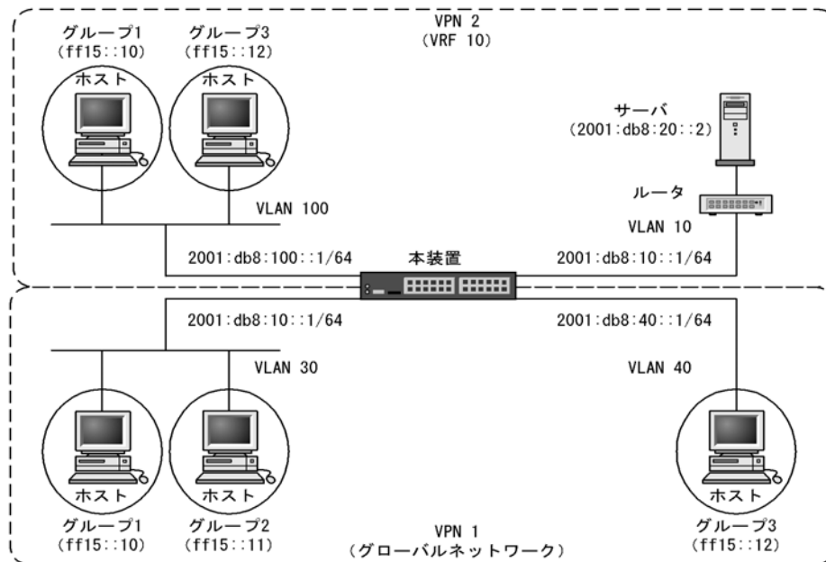
図 29-6 VRF での PIM-SM 構成例（PIM-SM VRF ゲートウェイ）
