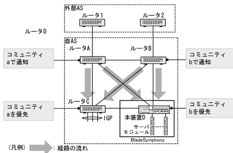
図 11-14 学習経路フィルタリングと COMMUNITIES 属性の使用例
