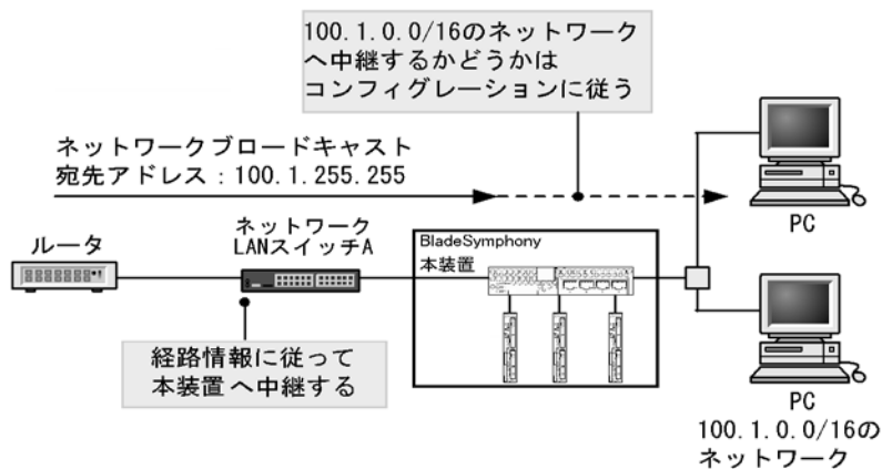
図 1-6 ネットワークブロードキャスト
