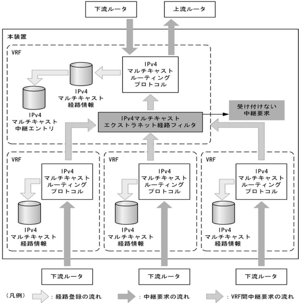
図 15-1 IPv4 マルチキャストエクストラネットの経路フィルタリングの概念図
