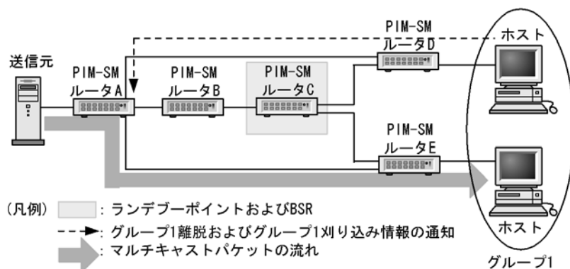
図 28-12 IPv6 マルチキャスト配送ツリーの刈り込み
