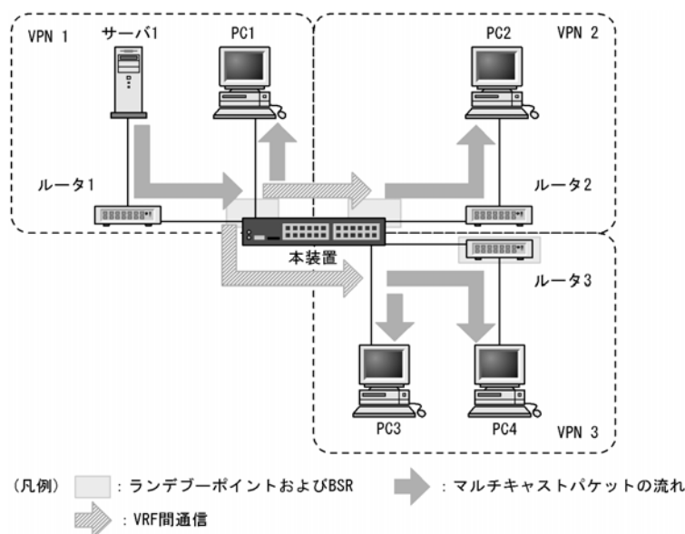
図 28-21 IPv6 マルチキャストエクストラネットの動作概要
