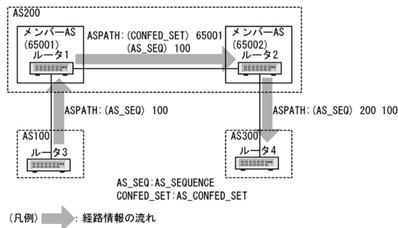
図 11-24 AS_PATH 属性の取り扱い
