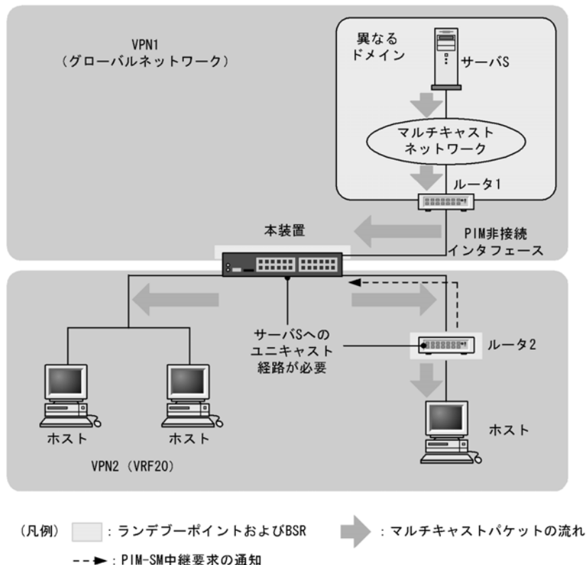
図 28-31 注意が必要な構成（エクストラネットでの PIM 非接続インタフェース経由の中継）
