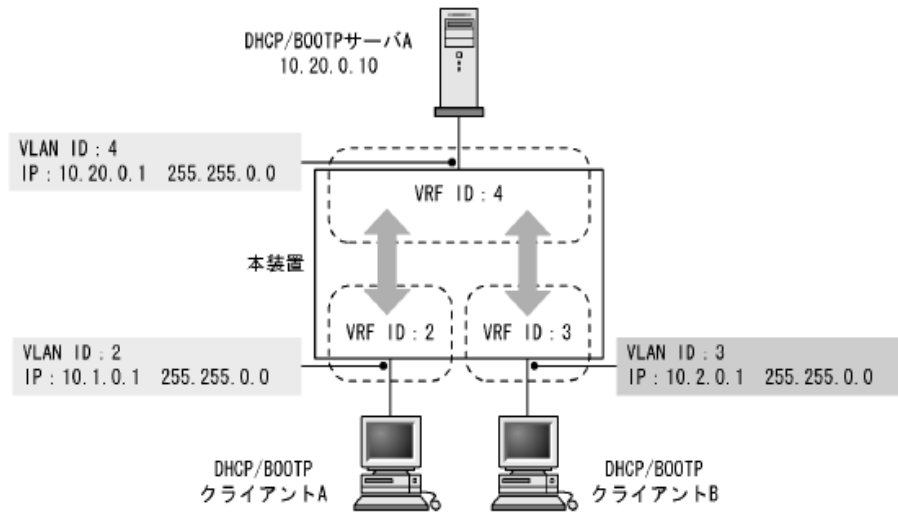
図 4-4 エクストラネット構成
