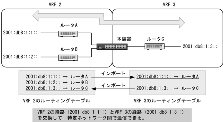
図 21-13 VRF 間の経路交換
