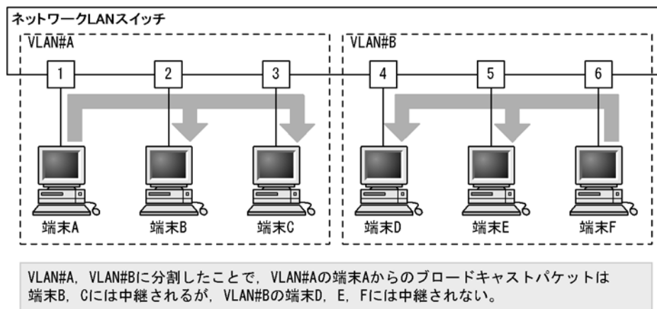
図 15-1 VLAN の概要
