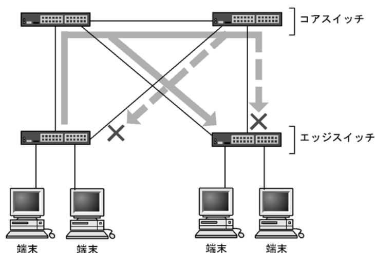
図 19-1 スパニングツリーを適用したネットワークの概要
