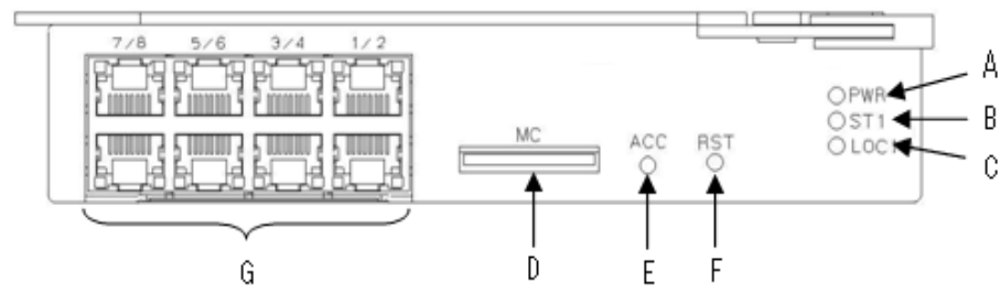
図 1-5 BS500 GG-BE3LSW4 (1Gbps 40 ポート LAN スイッチモジュール)
