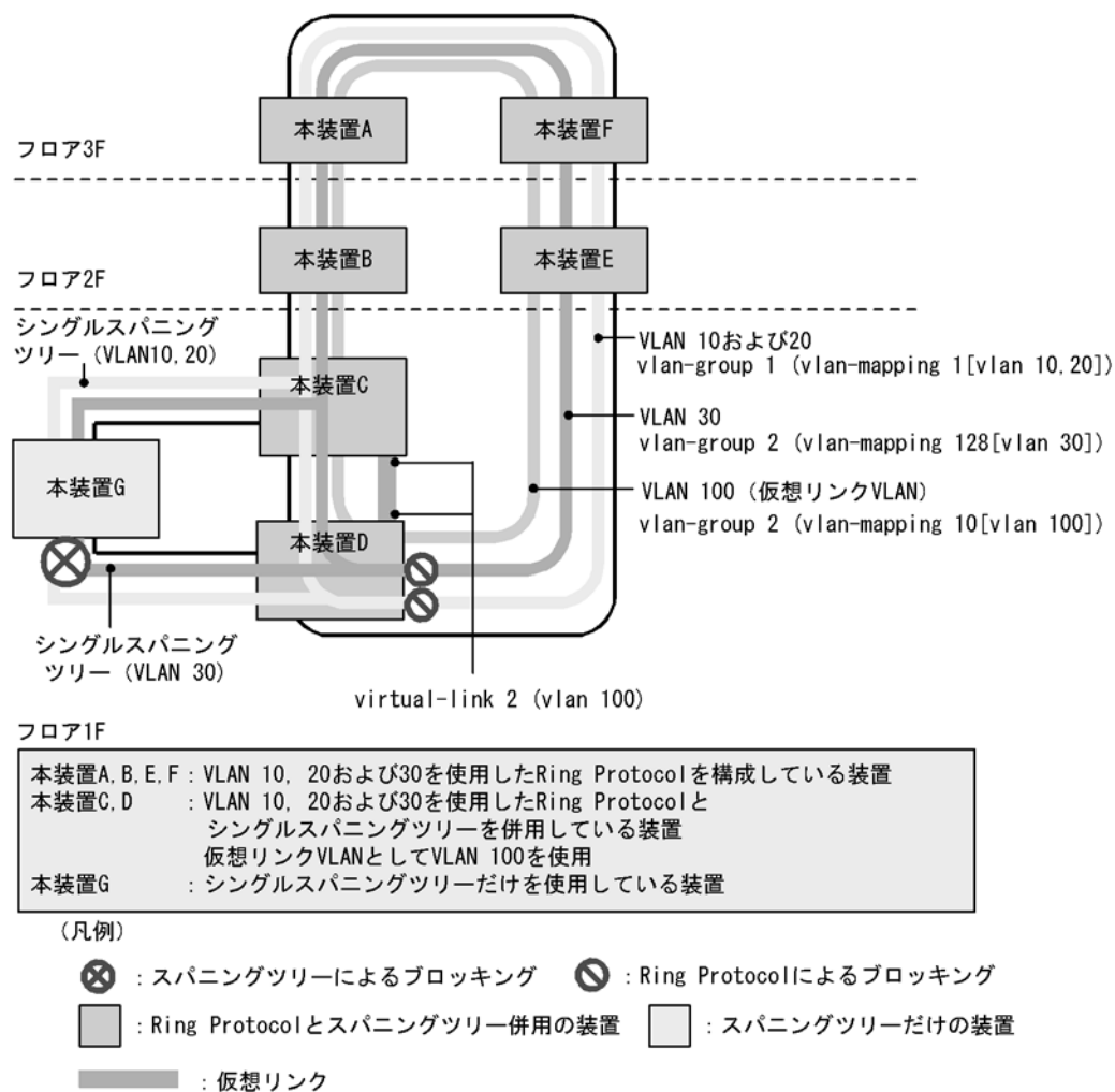
図 22-5 シングルスパニングツリーと Ring Protocol の共存構成
