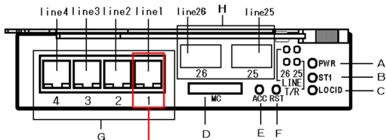
図 1-4 BS2000 GV-BE2LSW2, BS500 GG-BE3LSW2 (BS2000, BS500 1/10Gbps LAN スイッチモジュール)
