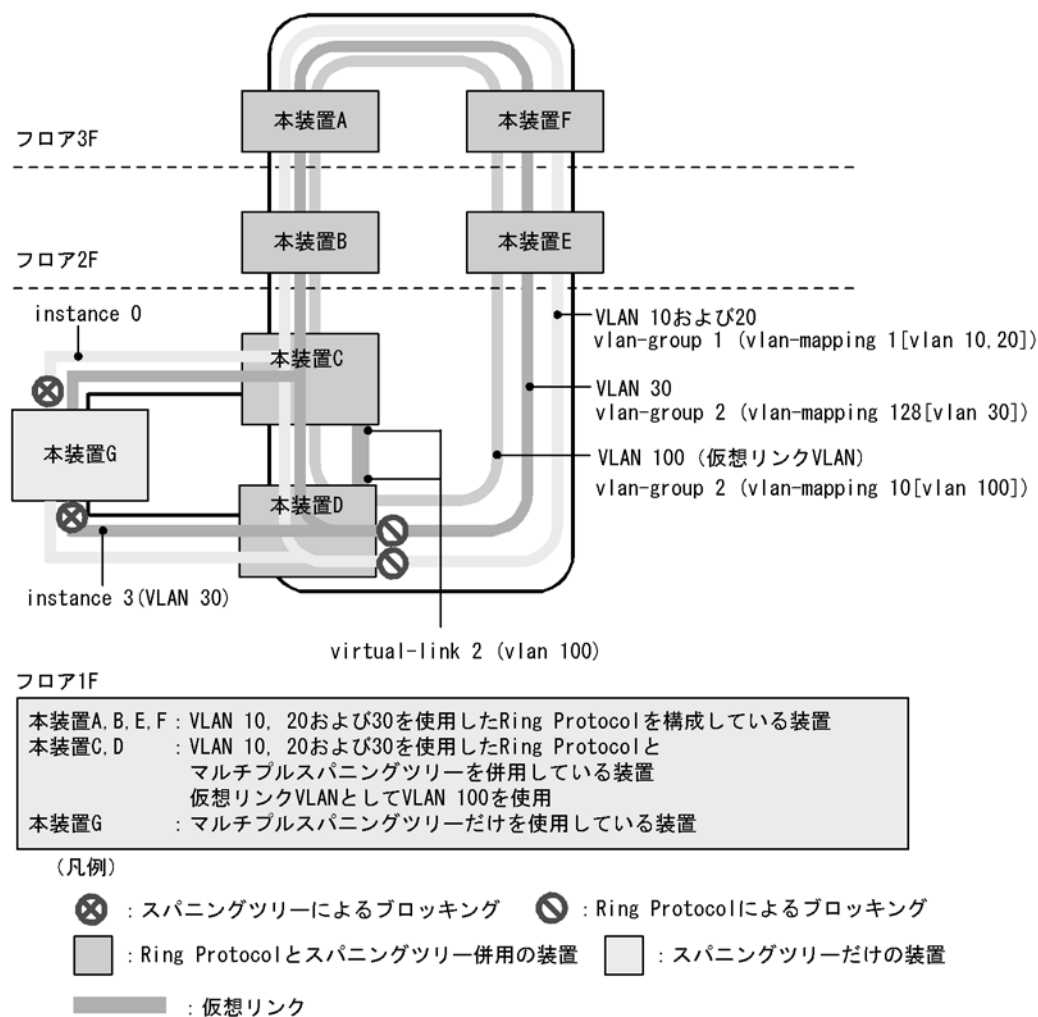
図 22-7 マルチプルスパニングツリーと Ring Protocol の共存構成
