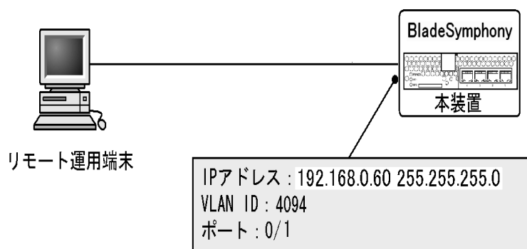
図 6-2 BS320 または、BS2000 LAN スイッチモジュールの工場出荷設定を使用したリモート運用端末との接続例
