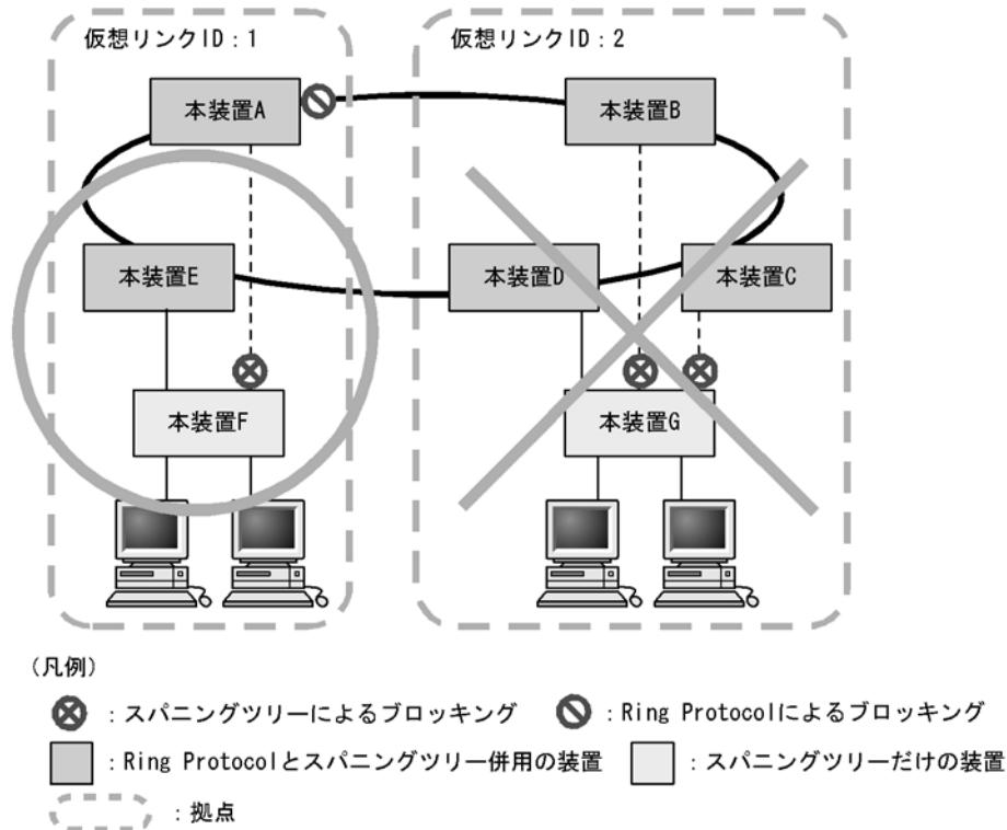
図 22-8 仮想リンクの禁止構成
