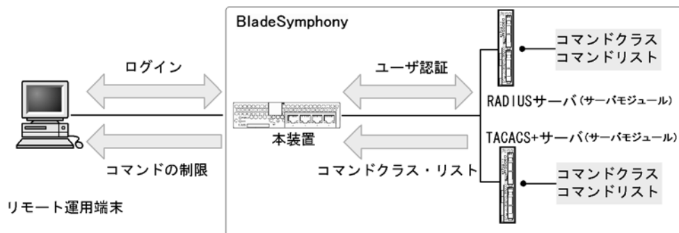
図 7-15 RADIUS/TACACS+ サーバによるログイン認証、コマンド承認
