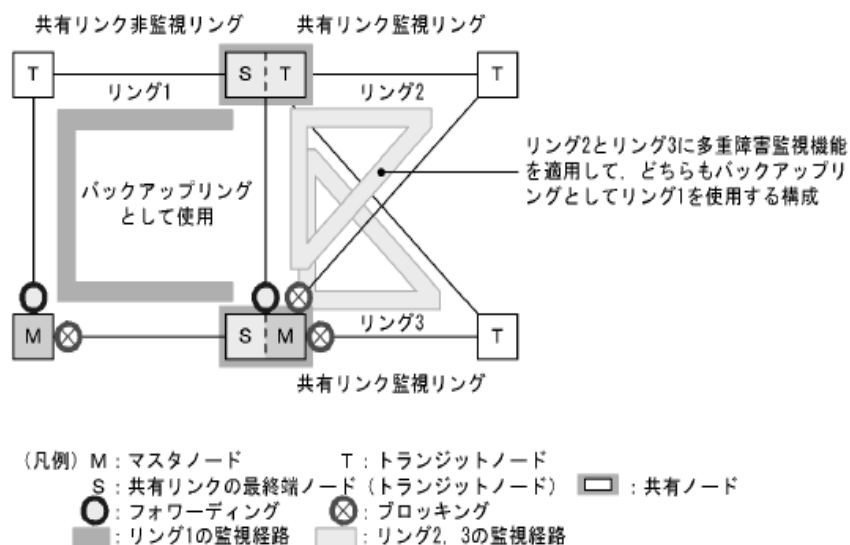
図 20-37 複数の共有リンク監視リングが同じバックアップリングを使用する構成
