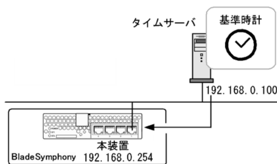
図 8-1 NTP 構成図（タイムサーバへの時刻の同期）
