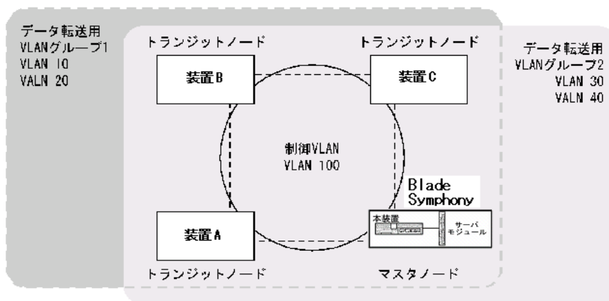
図 20-4 シングルリング構成
