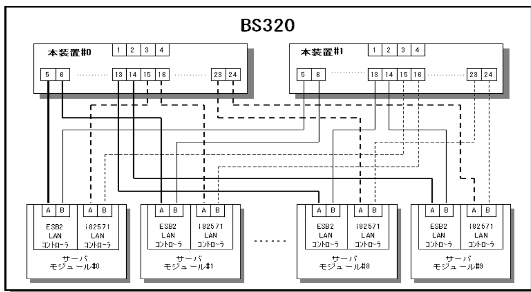
図 13-7 BS320 のサーバ接続ポートとサーバモジュールの接続
