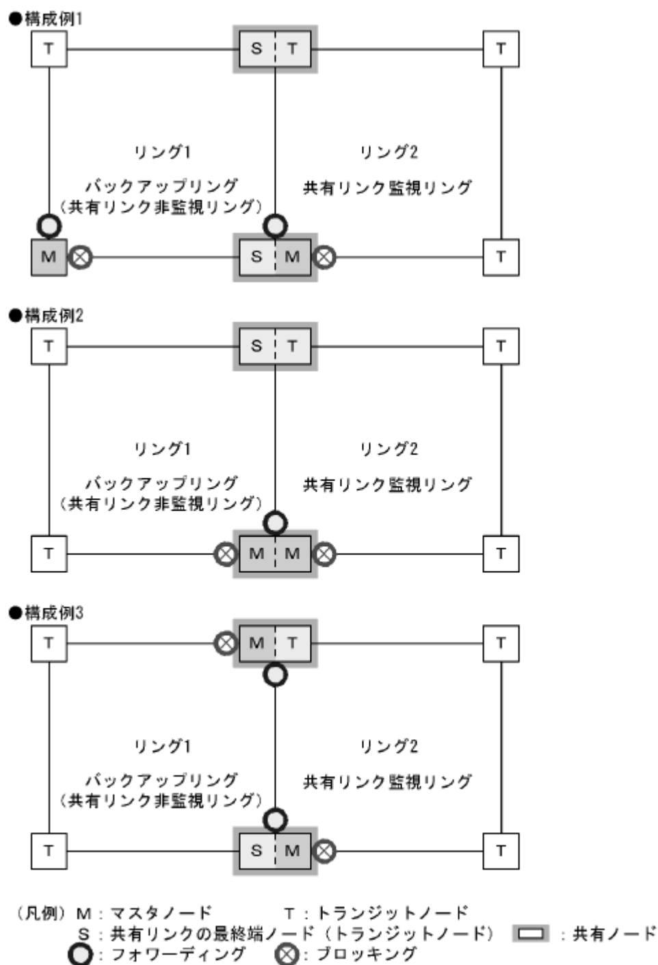
図 20-22 多重障害監視機能の基本構成例
