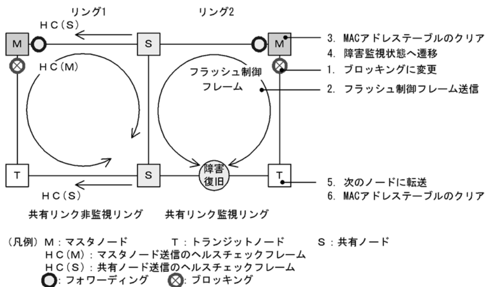
図 20-20 共有リンク監視リングでの共有リンク以外のリング障害復旧時の動作
