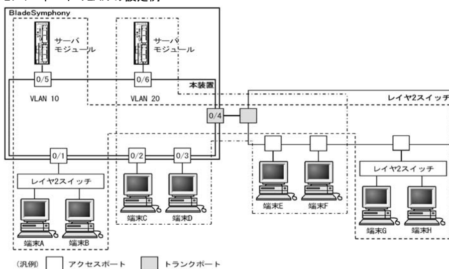
図 17-4 ポート VLAN の設定例
