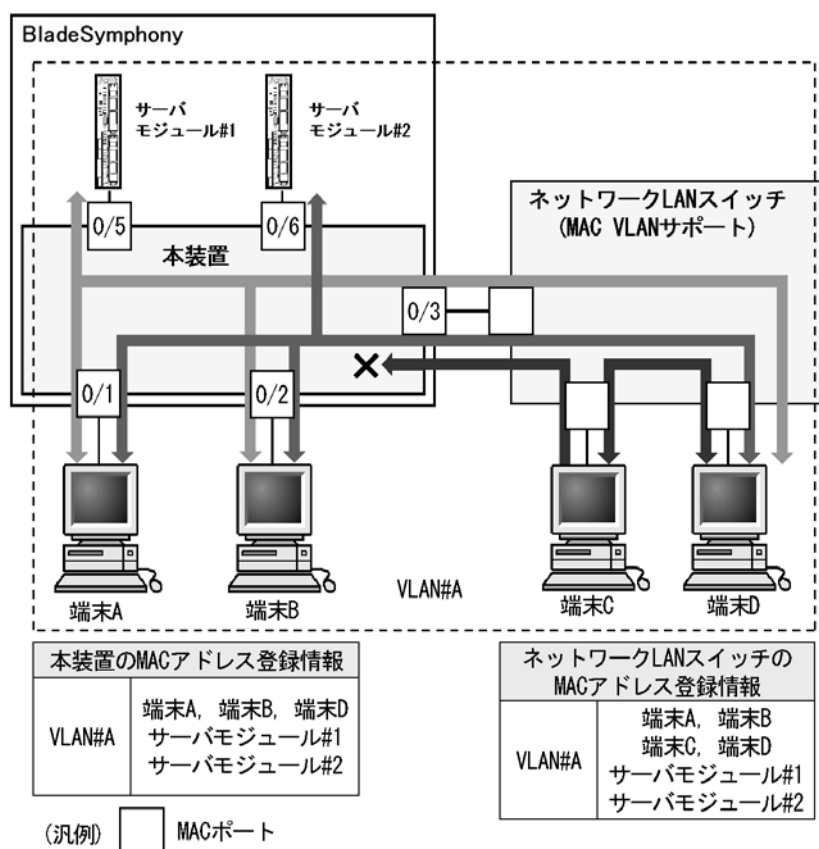
図 17-9 装置間を MAC ポートで接続した場合
