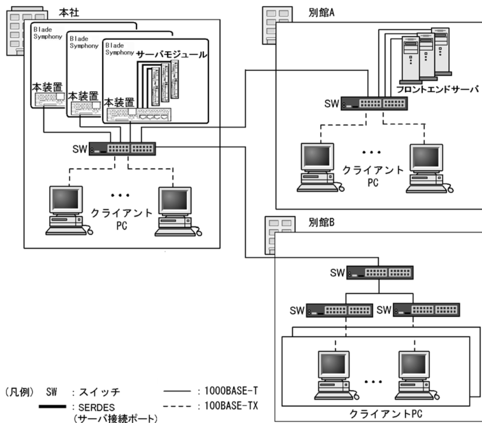
図 13-1 イーサネットの構成例
