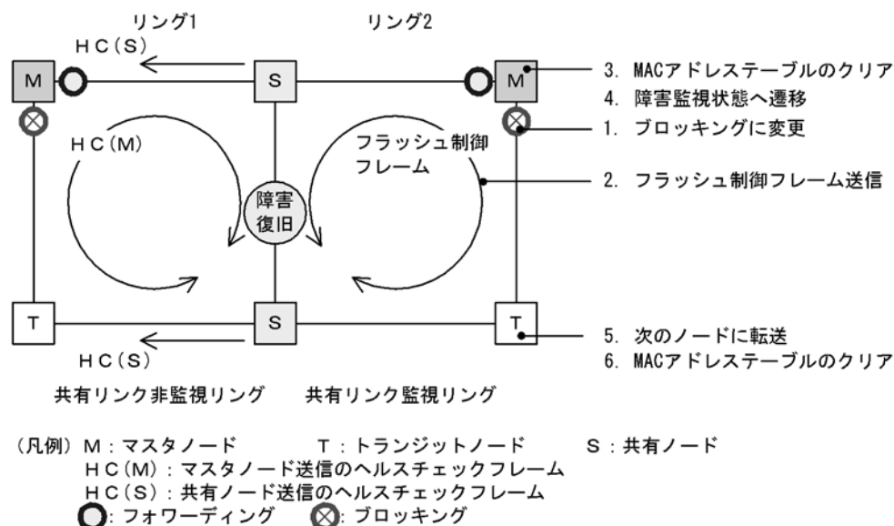
図 20-16 共有リンク復旧時の動作
