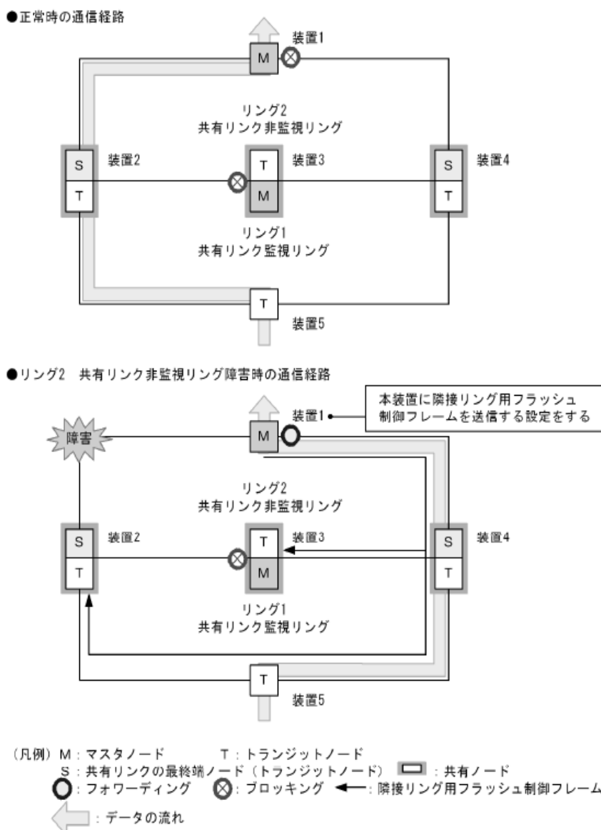
図 20-39 マスタノードの両リングポートが共有リンクとなる構成例
