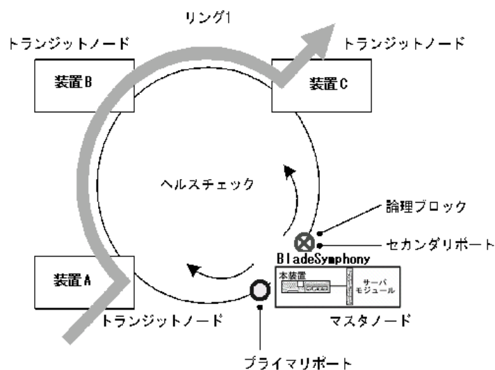
図 20-3 Ring Protocol の概要
