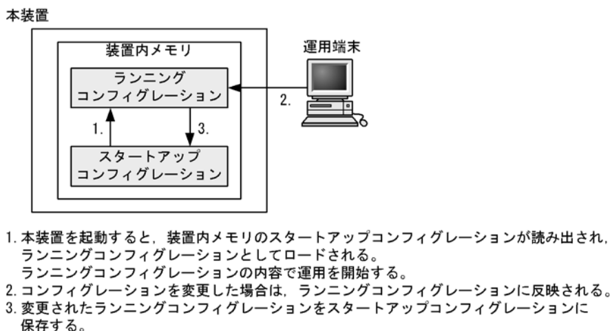
図 5-1 起動時、および運用中のコンフィグレーションの概要
