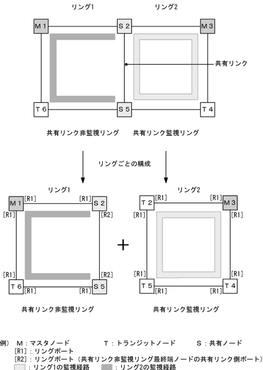
図 21-3 共有リンクありマルチリング構成（基本構成）
