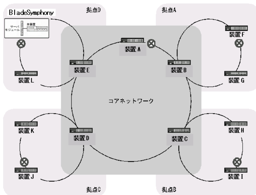
図 20-2 Ring Protocol の適用例（その 2）
