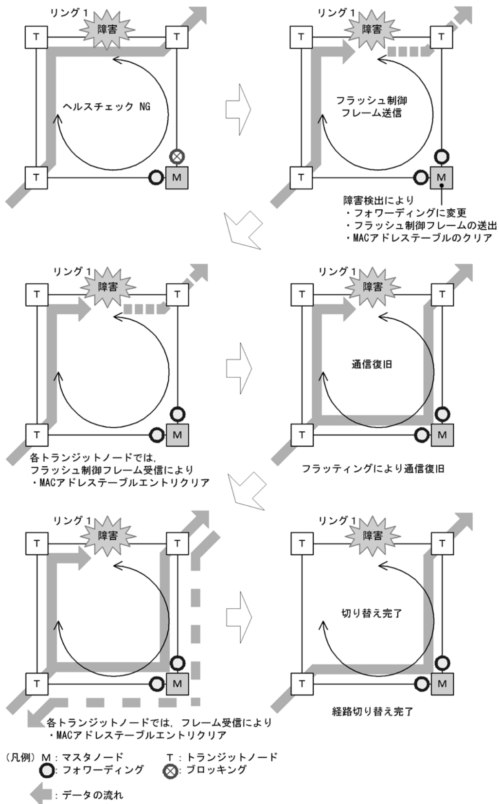
図 20-7 Ring Protocol の経路切り替え動作概要
