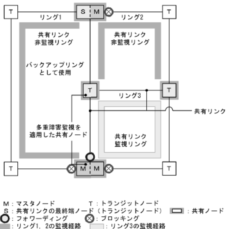
図 20-38 共有リンク内の共有ノードで多重障害を監視する構成
