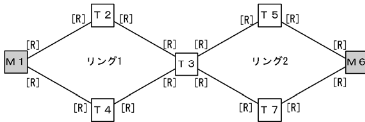
図 21-2 共有リンクなしマルチリング構成
