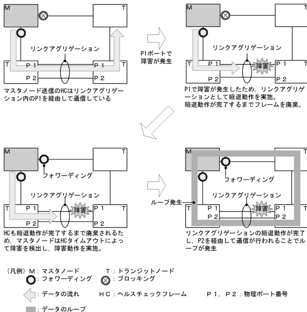
図 20-32 リンクアグリゲーション使用時の障害検出
