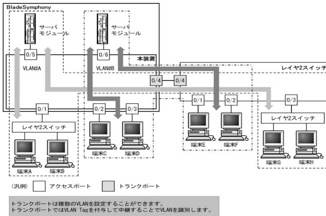
図 17-3 ポート VLAN の構成例
