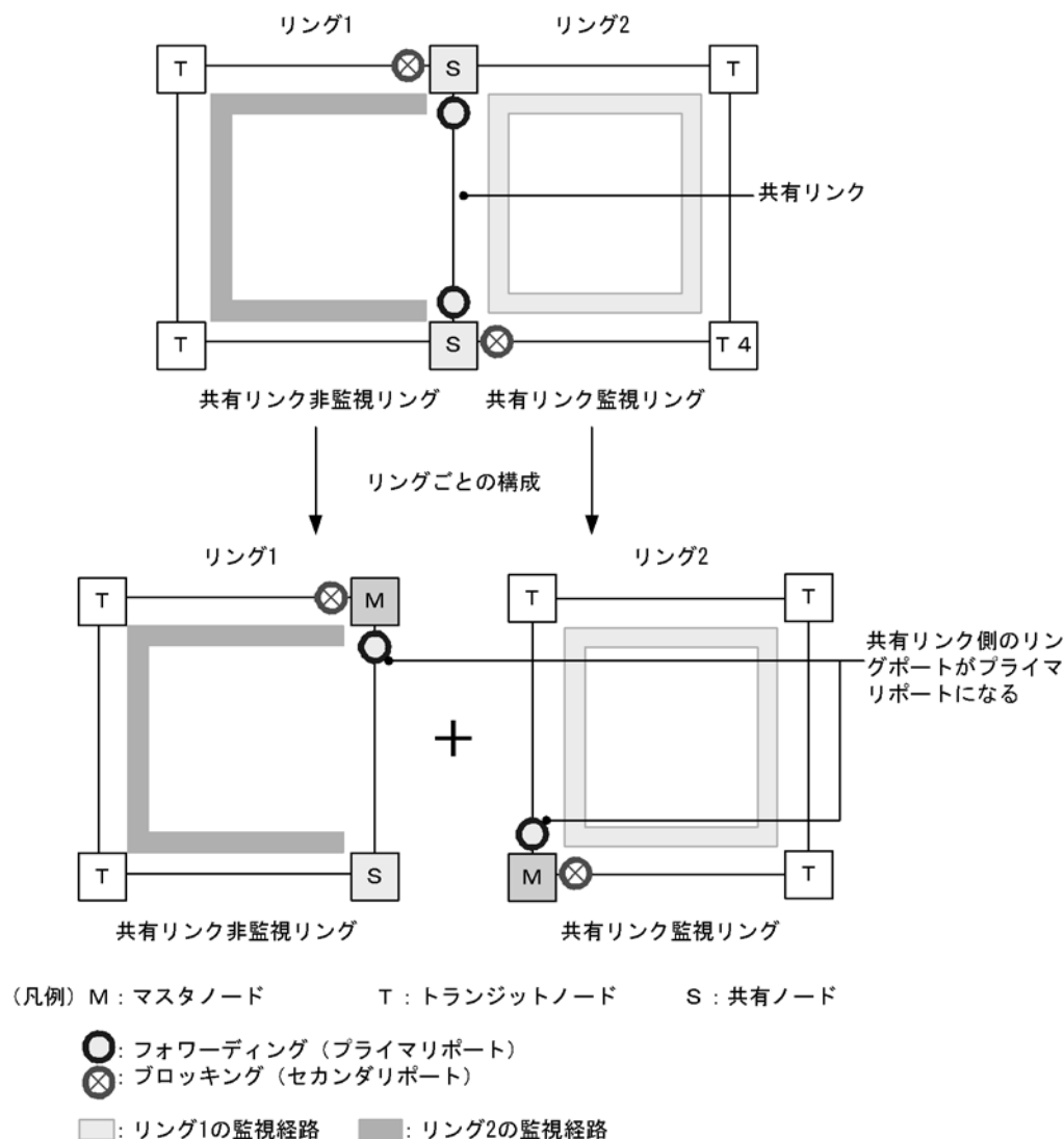
図 20-31 共有ノードをマスタノードとした場合のポート状態
