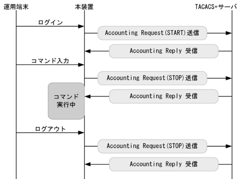
図 7-29 TACACS+ アカウンティングのシーケンス（ログインアカウンティング START-STOP, コマンドアカウンティング STOP-ONLY 送信モード時）
