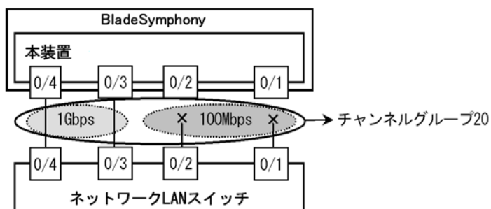
図 14-7 異速度混在モード状態 (100Mbit/s の 2 ポートと 1Gbit/s の 2 ポート)
