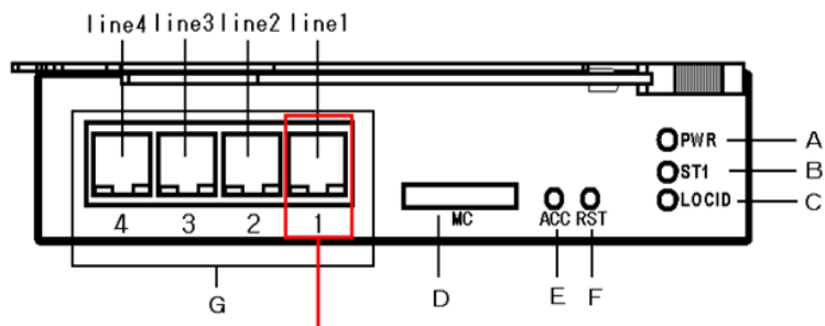
図 1-3 BS2000 GV-BE2LSW1, BS500 GG-BE3LSW1 (BS2000, BS500 1Gbps LAN スイッチモジュール)
