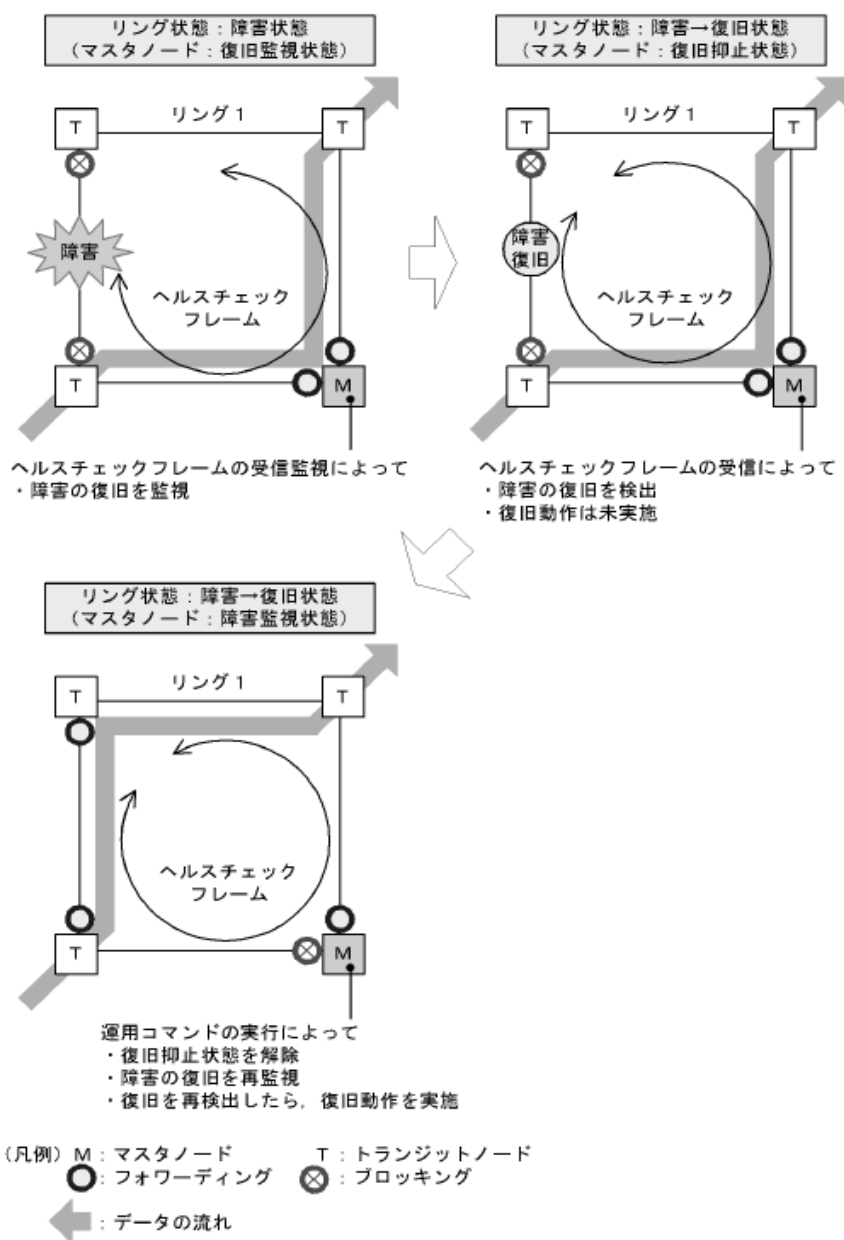
図 20-11 運用コマンドの実行によって経路切り戻し抑止を解除した場合の動作
