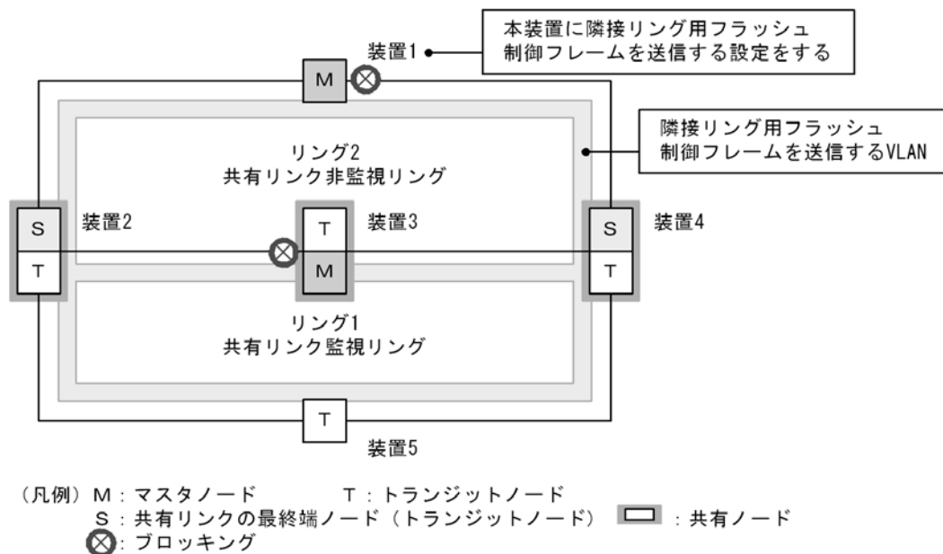
図 21-5 マスタノードの両リングポートが共有リンクとなる構成
