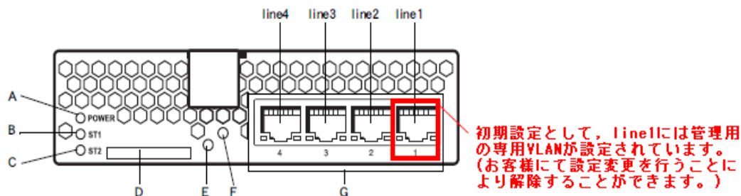
図 1-1 BS320 GG-BE9LSWM1 (BS320 1GbpsLAN スイッチモジュール)
