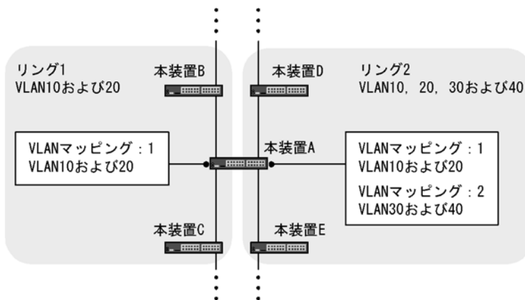
図 20-30 リングごとの VLAN マッピングの割り当て例
