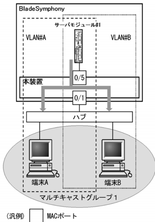
図 17-10 VLAN 混在時のマルチキャスト
