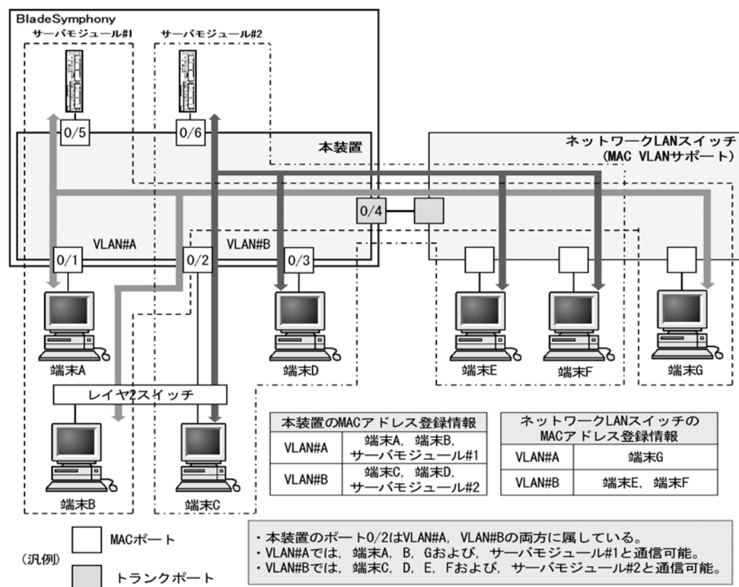
図 17-8 MAC VLAN の構成例
