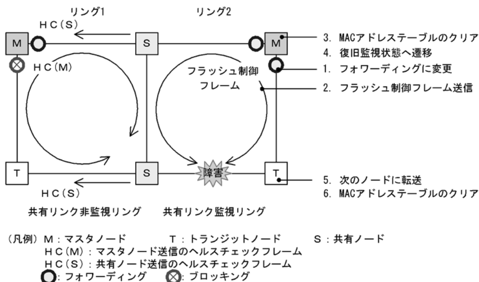
図 20-19 共有リンク監視リングでの共有リンク以外のリング障害時の動作
