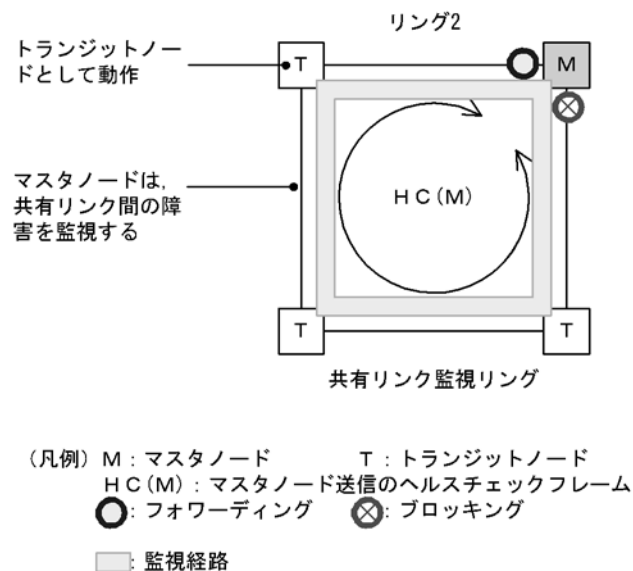
図 20-14 共有リンク監視リングでの正常時の動作
