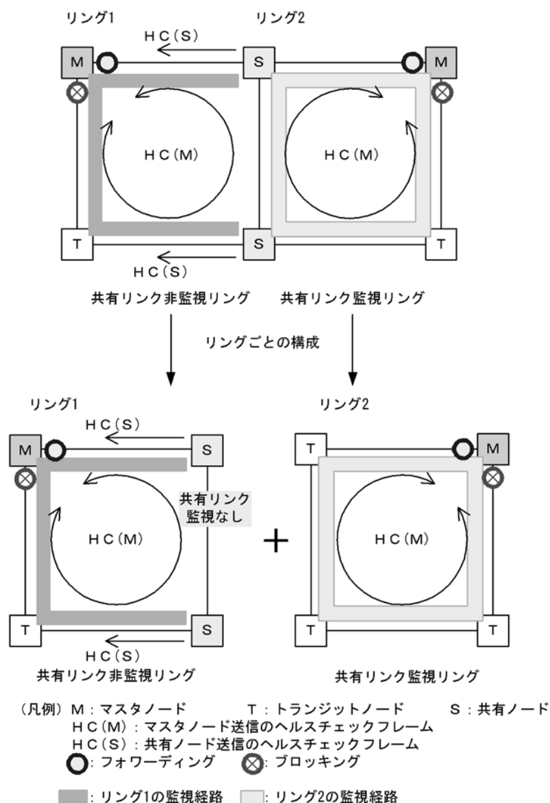
図 20-12 リング正常時の状態
