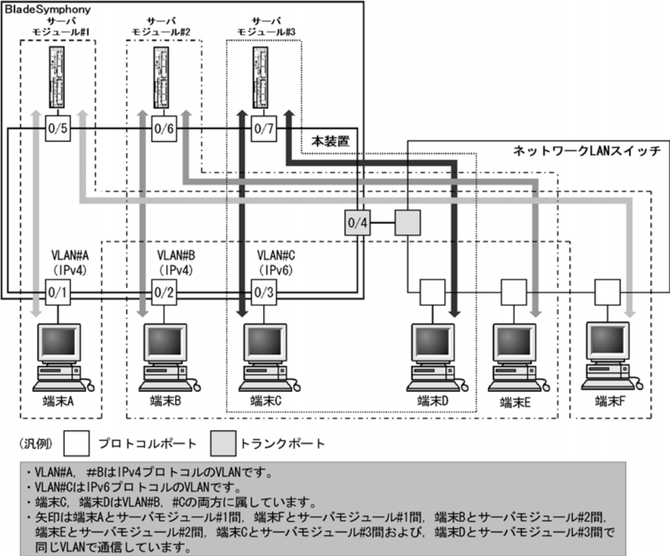
図 17-5 プロトコル VLAN の構成例
