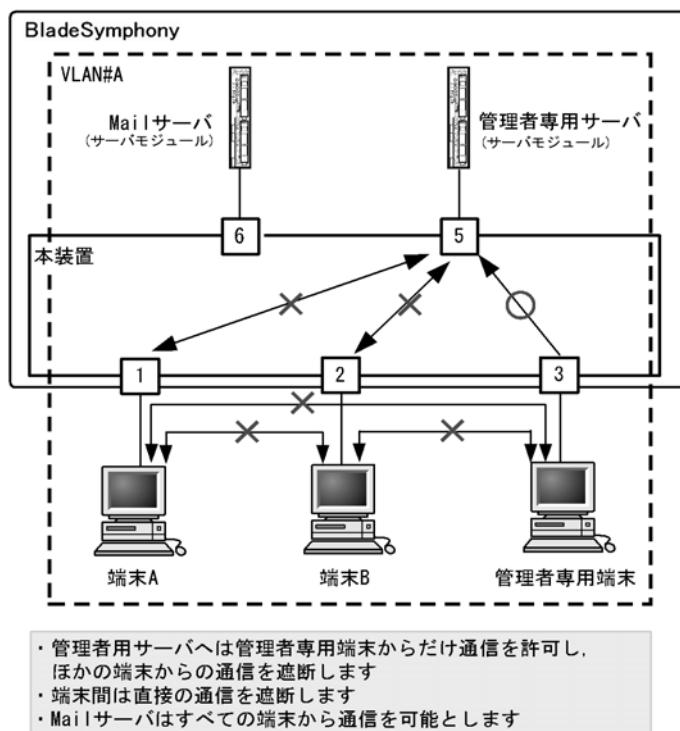
図 18-5 ポート間中継遮断機能の適用例
