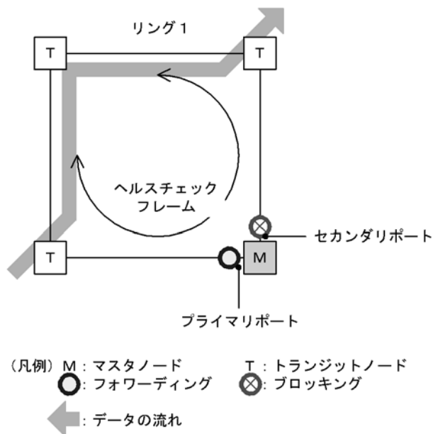
図 20-8 リング正常時の動作
