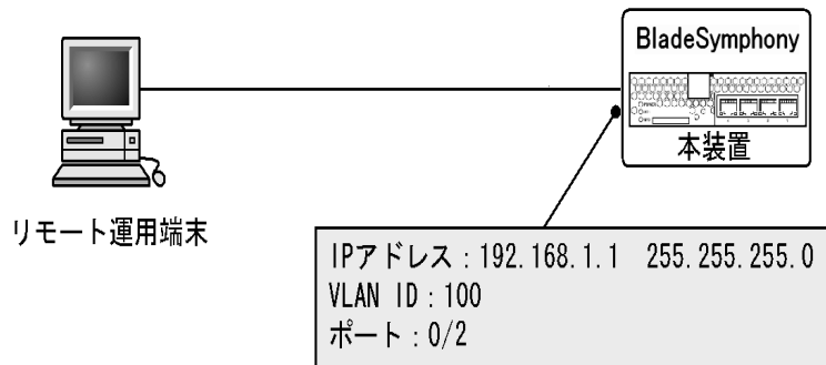
図 6-3 新規にリモート運用端末との接続例
