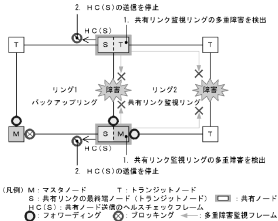
図 20-25 多重障害発生時の動作
