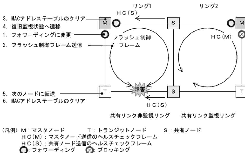
図 20-17 共有リンク非監視リングにおける共有リンク以外のリング障害時の動作
