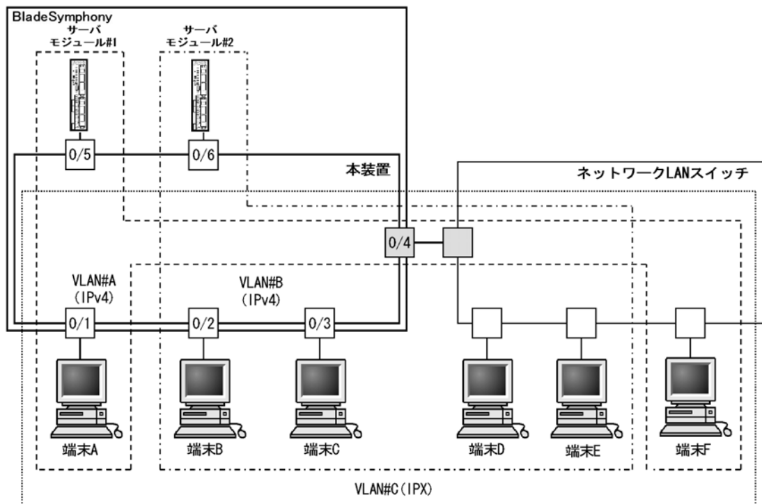
図 17-6 プロトコルポートでネイティブ VLAN を使用する構成例
