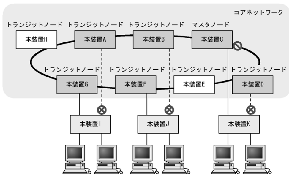
図 22-1 Ring Protocol とスパニングツリーの併用例（シングルリング構成）
