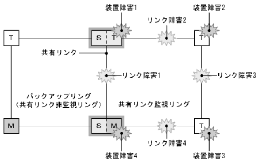
図 20-21 共有リンク監視リングでの障害発生例
