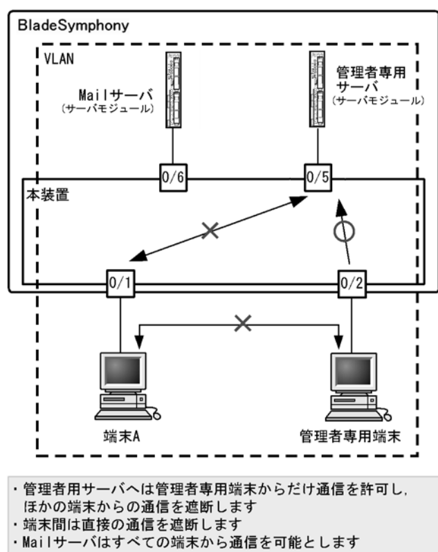
図 18-6 ポート間中継遮断機能の設定例
