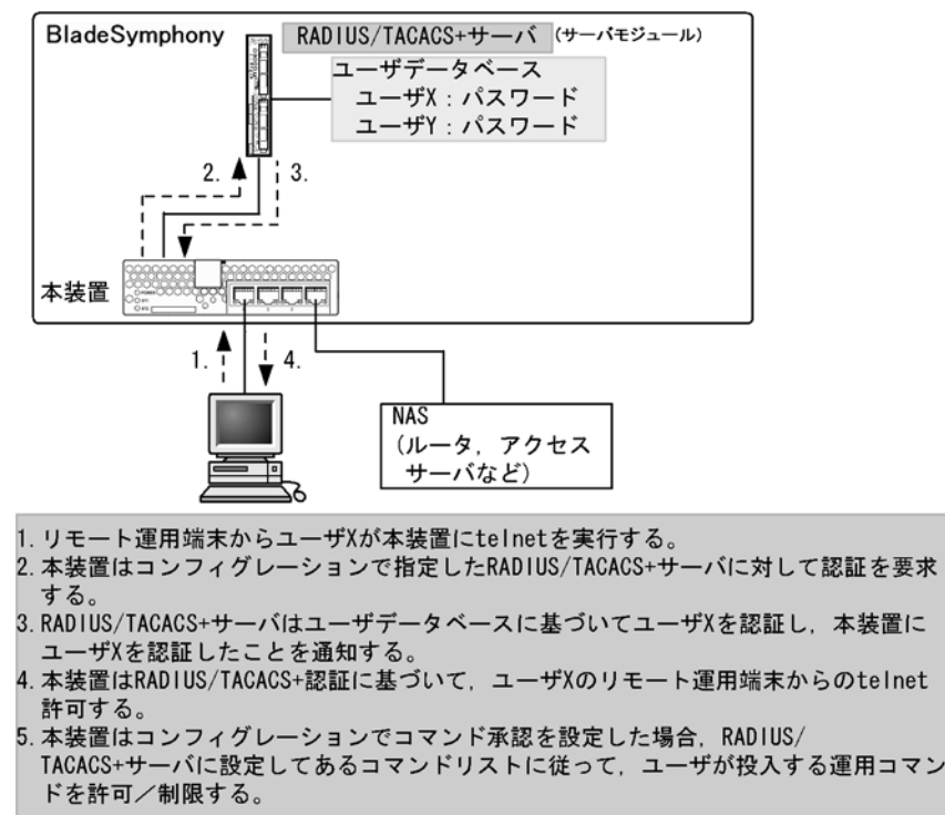
図 7-11 RADIUS/TACACS+ 認証の流れ
