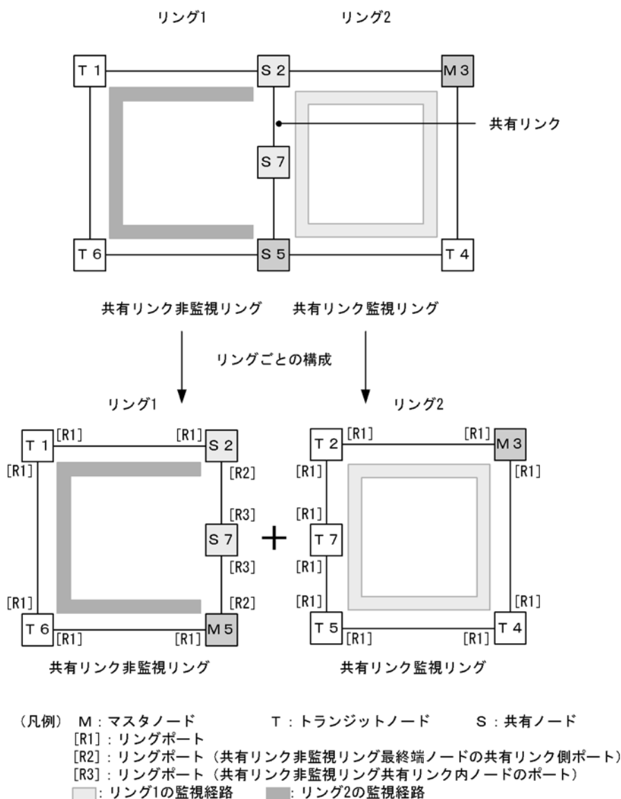
図 21-4 共有リンクありのマルチリング構成（拡張構成）
