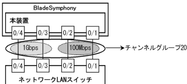
図 14-6 異速度混在モード状態 (100Mbit/s の 2 ポートと 1Gbit/s の 2 ポート)
