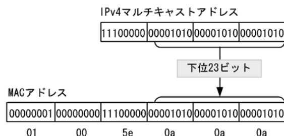
図 23-3 IPv4 マルチキャストアドレスと MAC アドレスの対応
