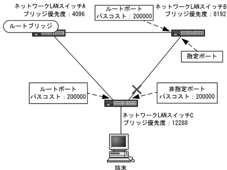
図 19-4 スパニングツリーのトポロジー設計
