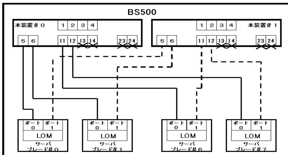
図 13-9 BS500 のサーバ接続ポートとサーバモジュールの接続
