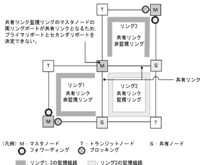
図 20-36 マスタノードのプライマリポートが決定できない構成
