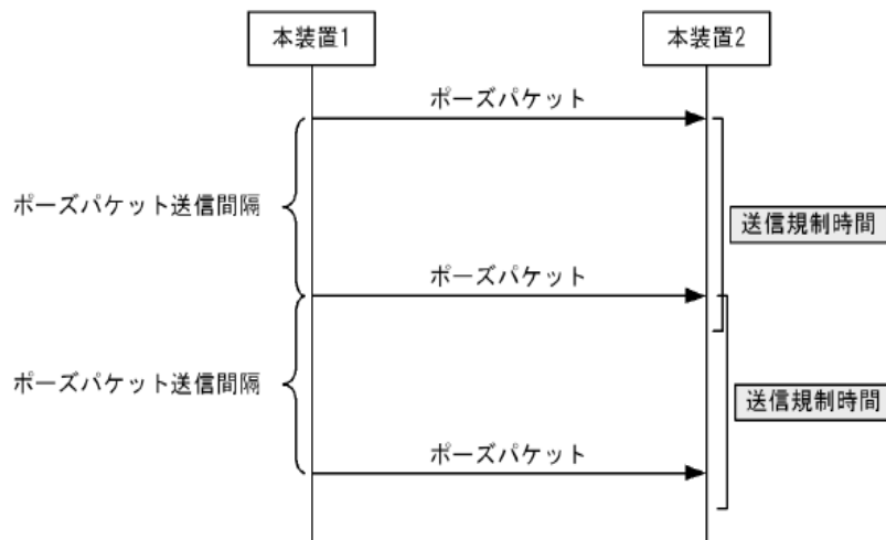
図 13-4 デフォルトでの動作シーケンス
