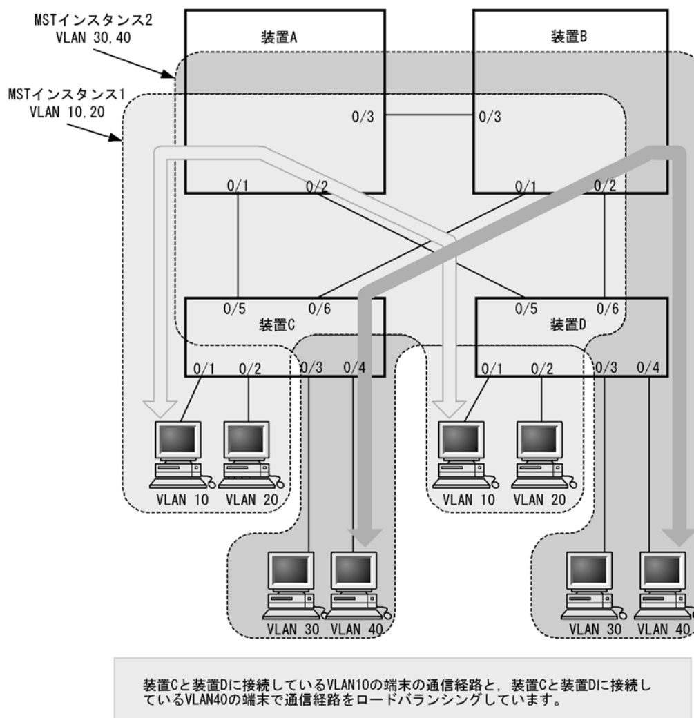
図 19-13 マルチプルスパニングツリーのロードバランシング構成
