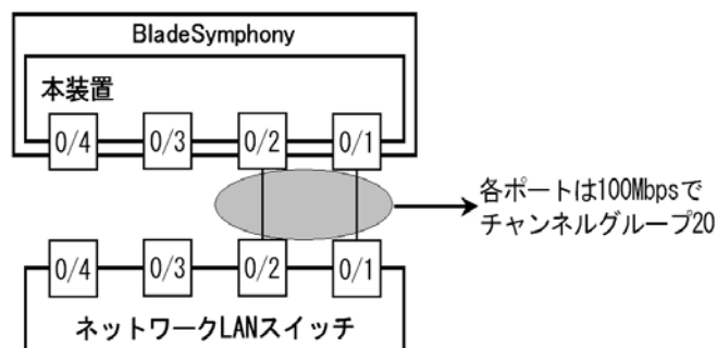
図 14-4 従来状態で運用
