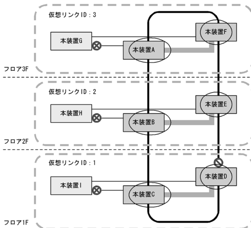
図 22-3 仮想リンクの概要
