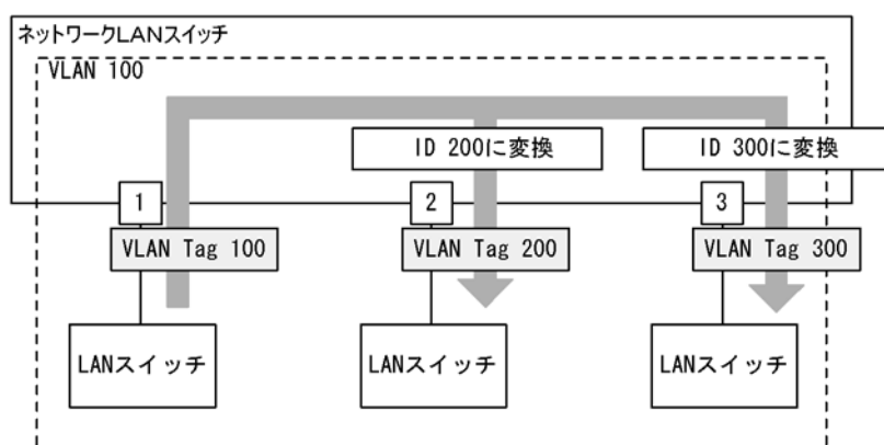
図 18-2 Tag 変換機能の構成例
