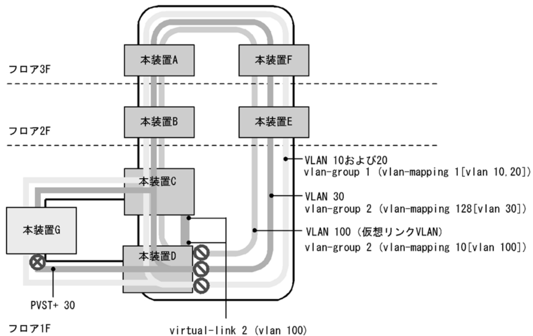
図 22-4 PVST+ と Ring Protocol の共存構成
