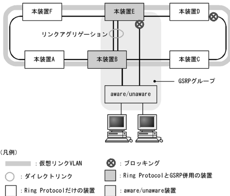
図 22-10 Ring Protocol と GSRP の併用例（ダイレクトリンクをリングネットワークで使用しない場合）
