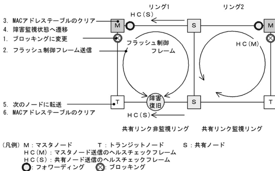
図 20-18 共有リンク非監視リングでの共有リンク以外のリング障害復旧時の動作
