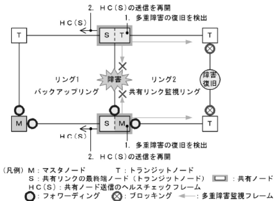
図 20-27 多重障害からの一部復旧時の動作
