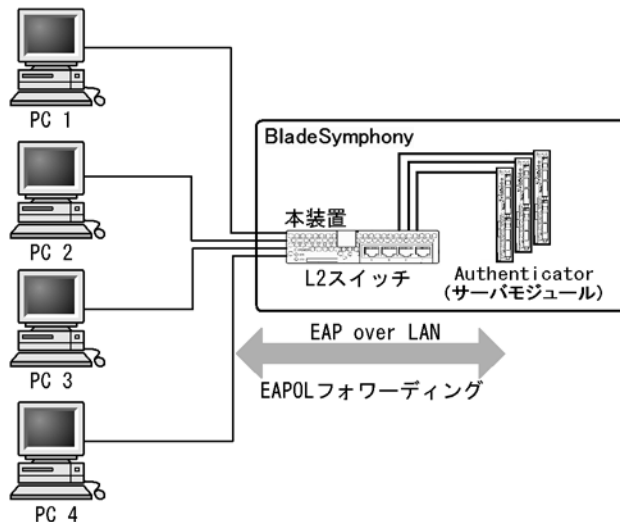
図 18-4 EAPOL フォワーディング機能の適用例
