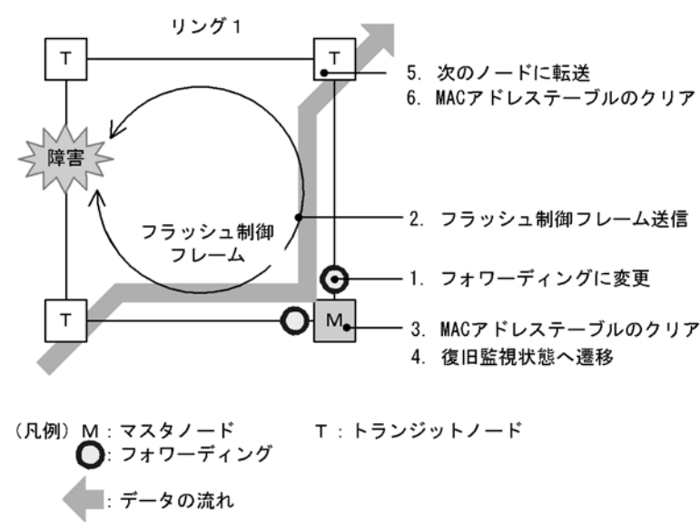
図 20-9 リング障害時の動作
