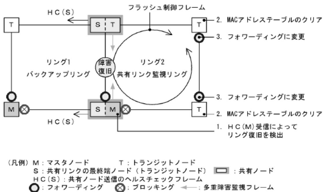
図 20-29 共有リンク障害復旧時の動作
