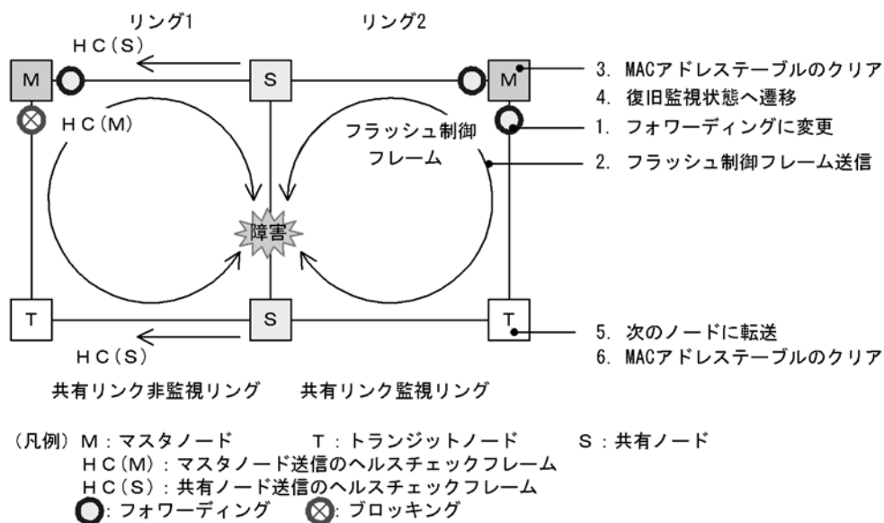
図 20-15 共有リンク障害時の動作
