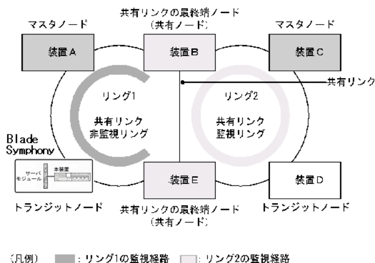
図 20-6 共有リンクありのマルチリング構成
