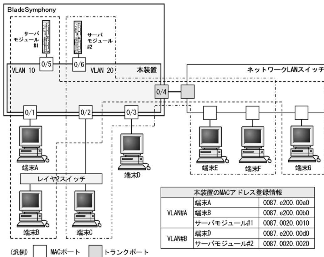
図 17-11 MAC VLAN の設定例
