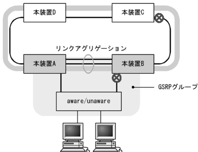
図 22-9 Ring Protocol と GSRP の併用例（ダイレクトリンクをリングネットワークで使用する場合）
