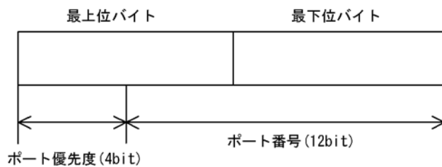
図 19-3 ポート識別子
