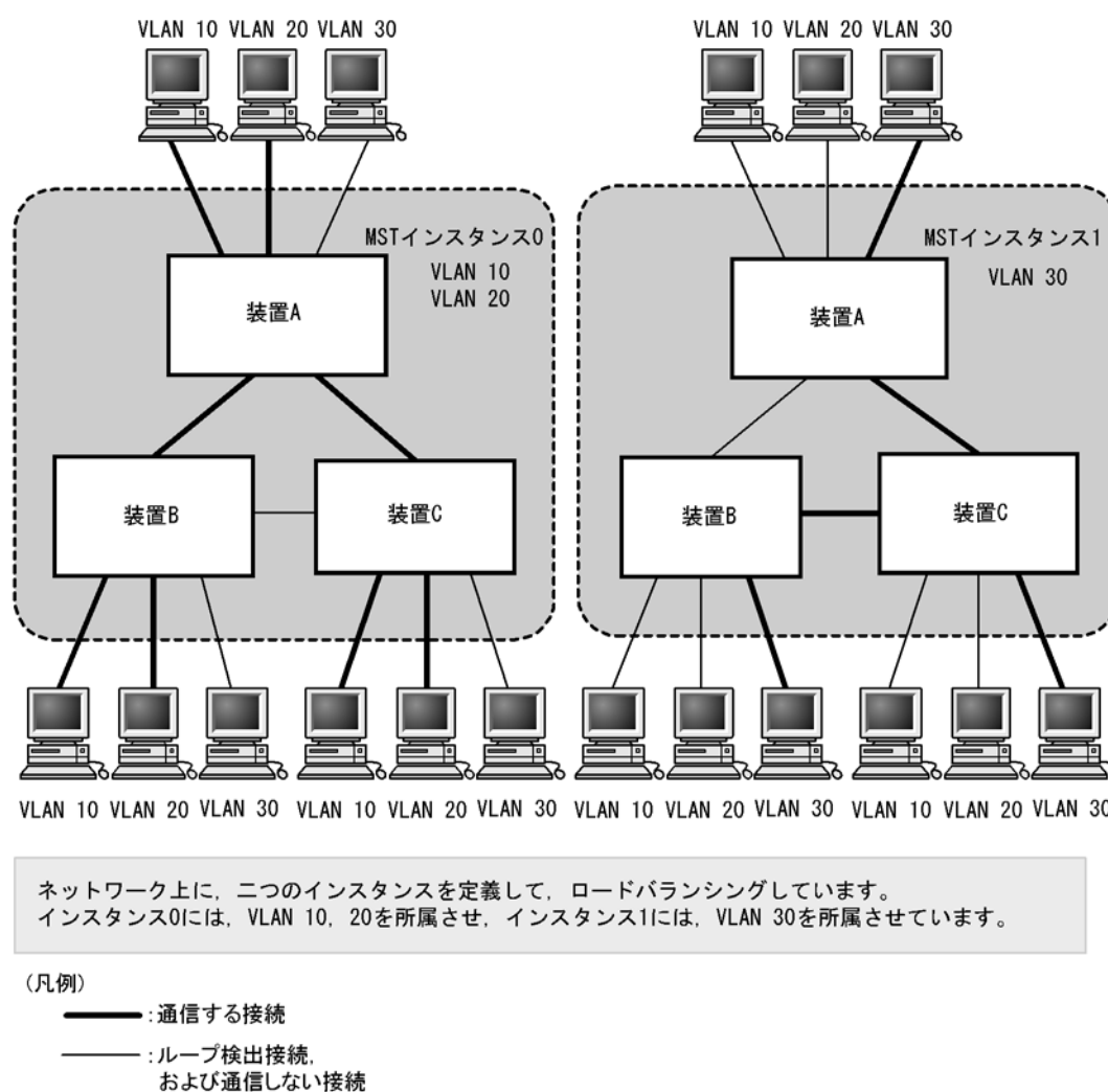
図 19-11 MST インスタンスイメージ
