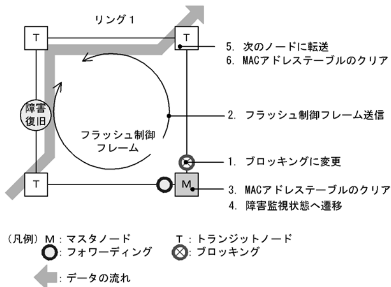
図 20-10 障害復旧時の動作
