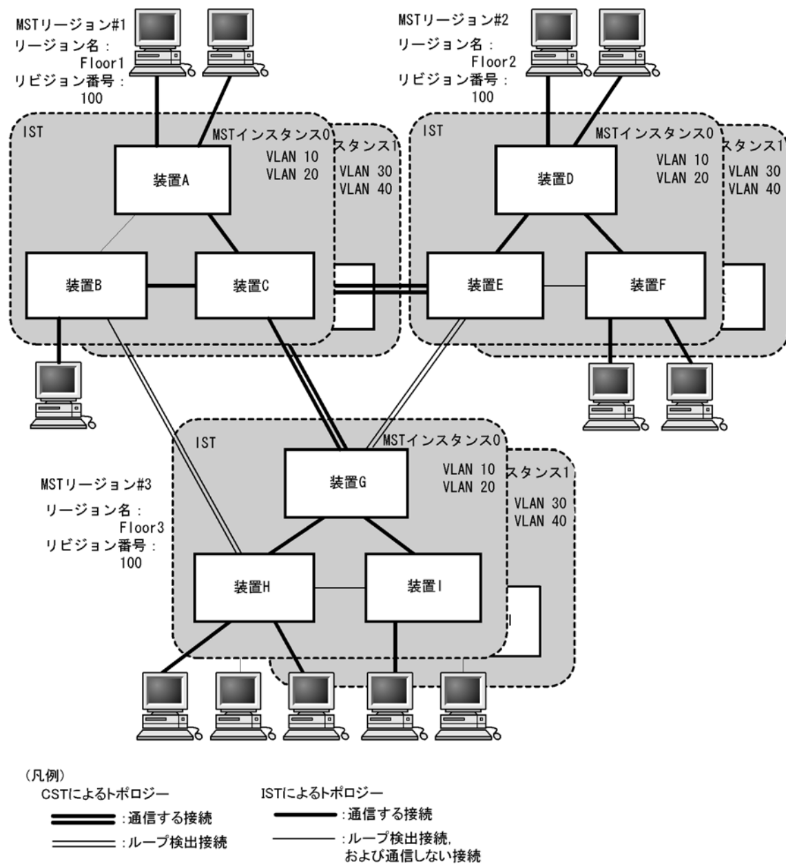
図 19-14 MST リージョンによるネットワーク構成
