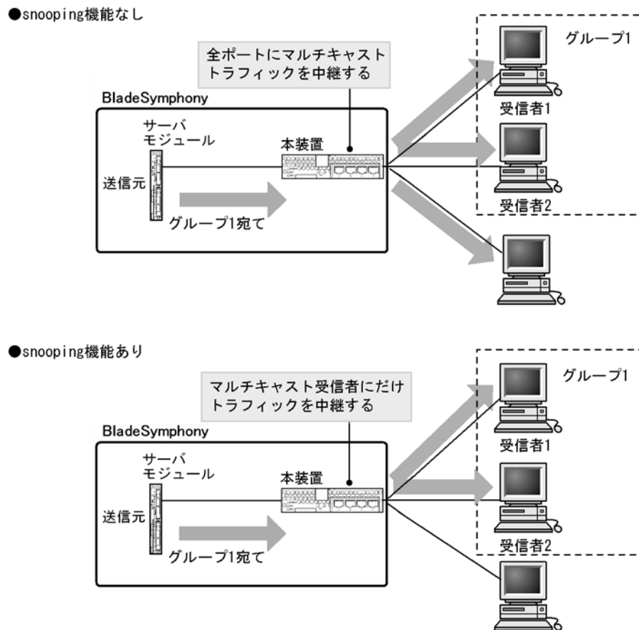
図 23-2 IGMP snooping/MLD snooping 概要
