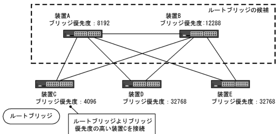
図 19-18 装置 A、装置 B よりブリッジ優先度の高い装置 C を接続
