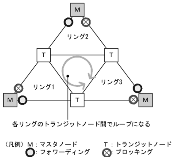
図 20-35 ループになるマルチリング構成
