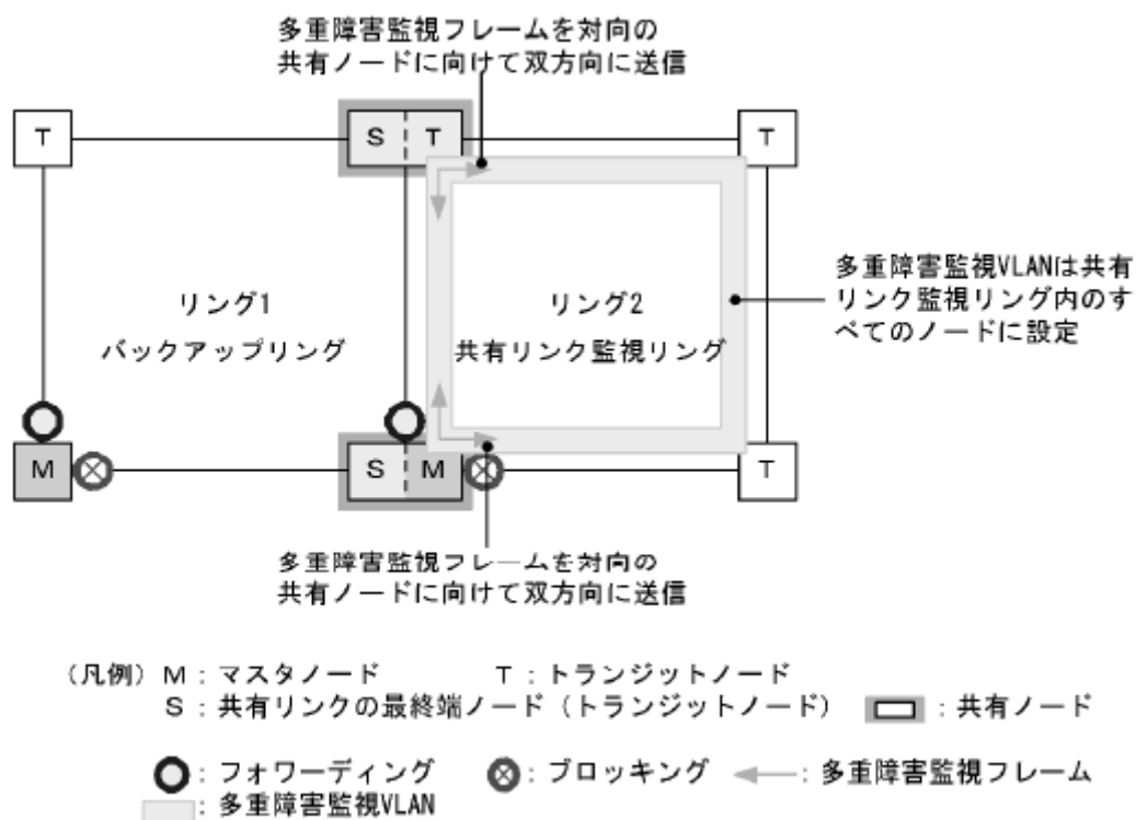
図 20-23 多重障害監視の動作概要
