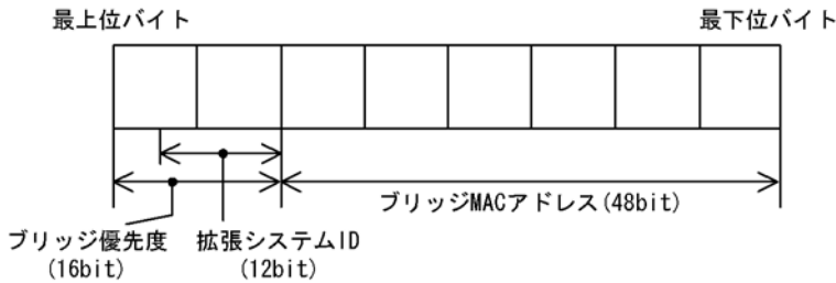
図 19-2 ブリッジ識別子
