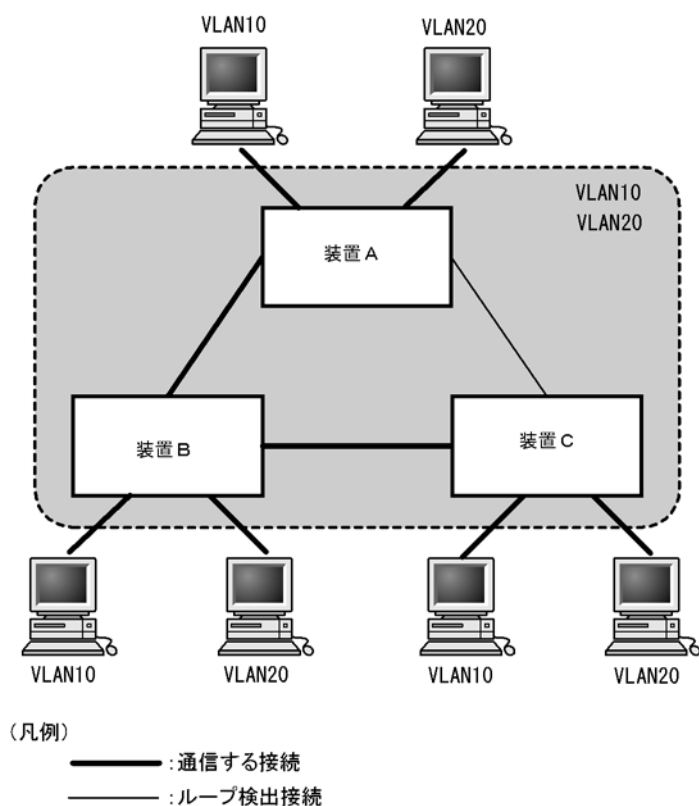
図 19-9 シングルスパニングツリーによるネットワーク構成
