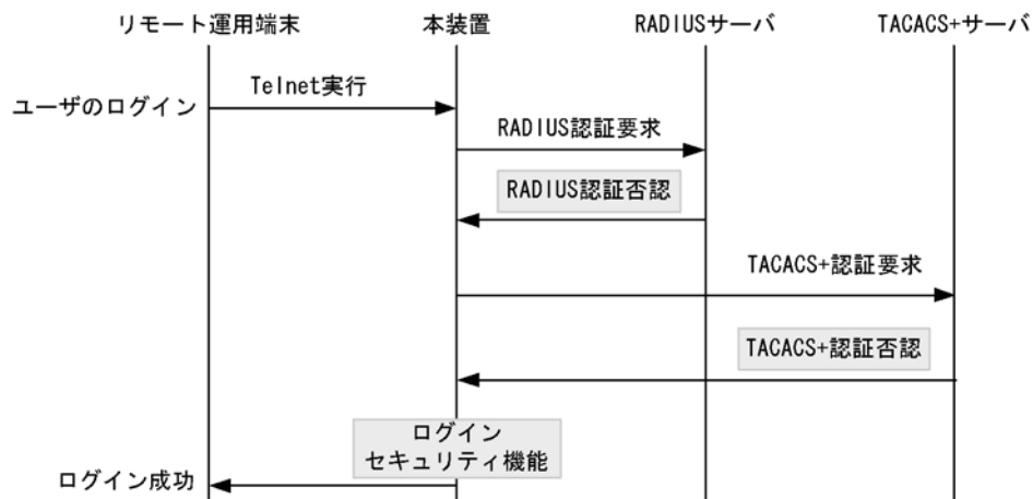
図 7-12 認証方式シーケンス
