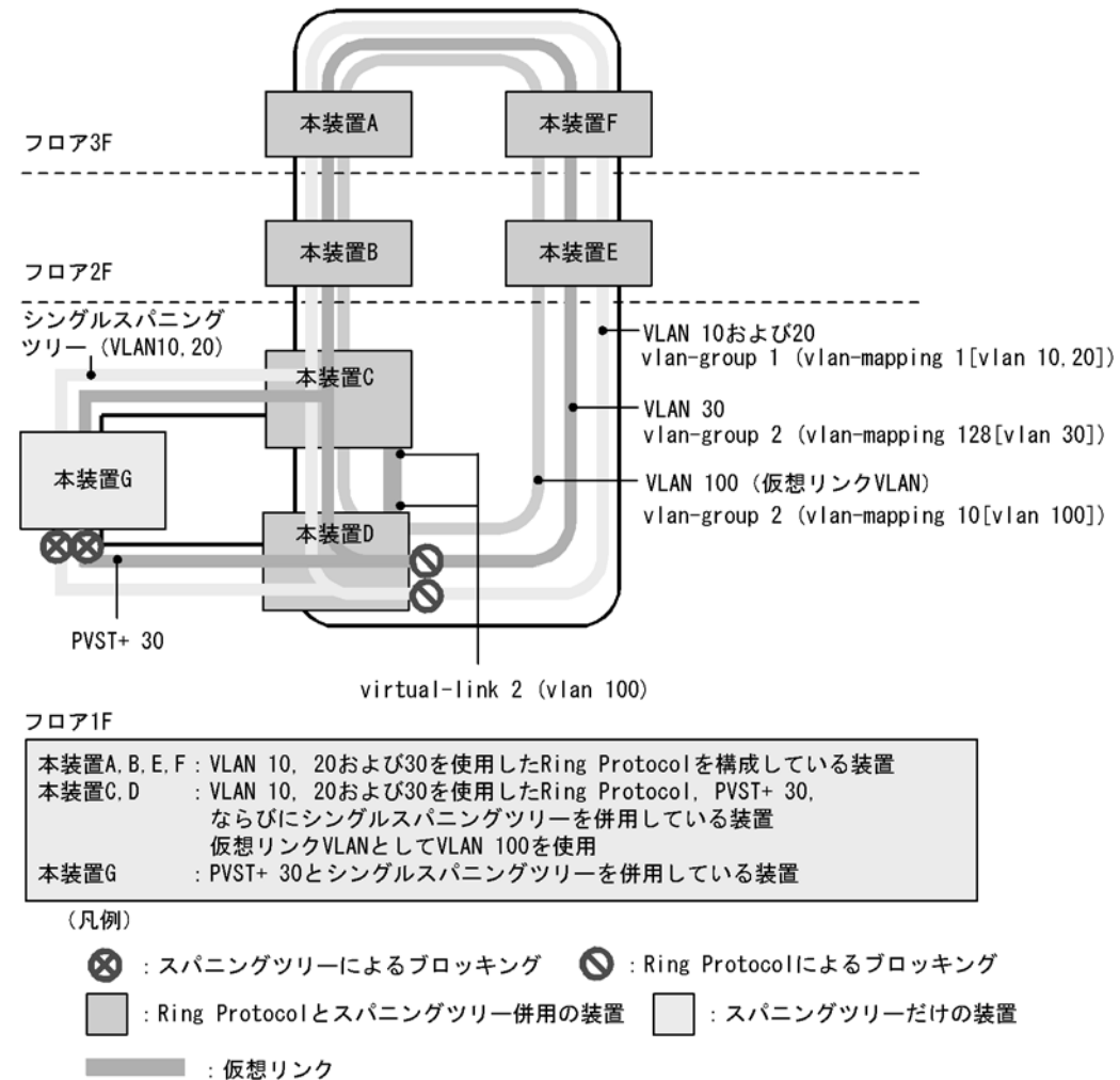
図 22-6 シングルスパニングツリー, PVST+, および Ring Protocol の共存構成
