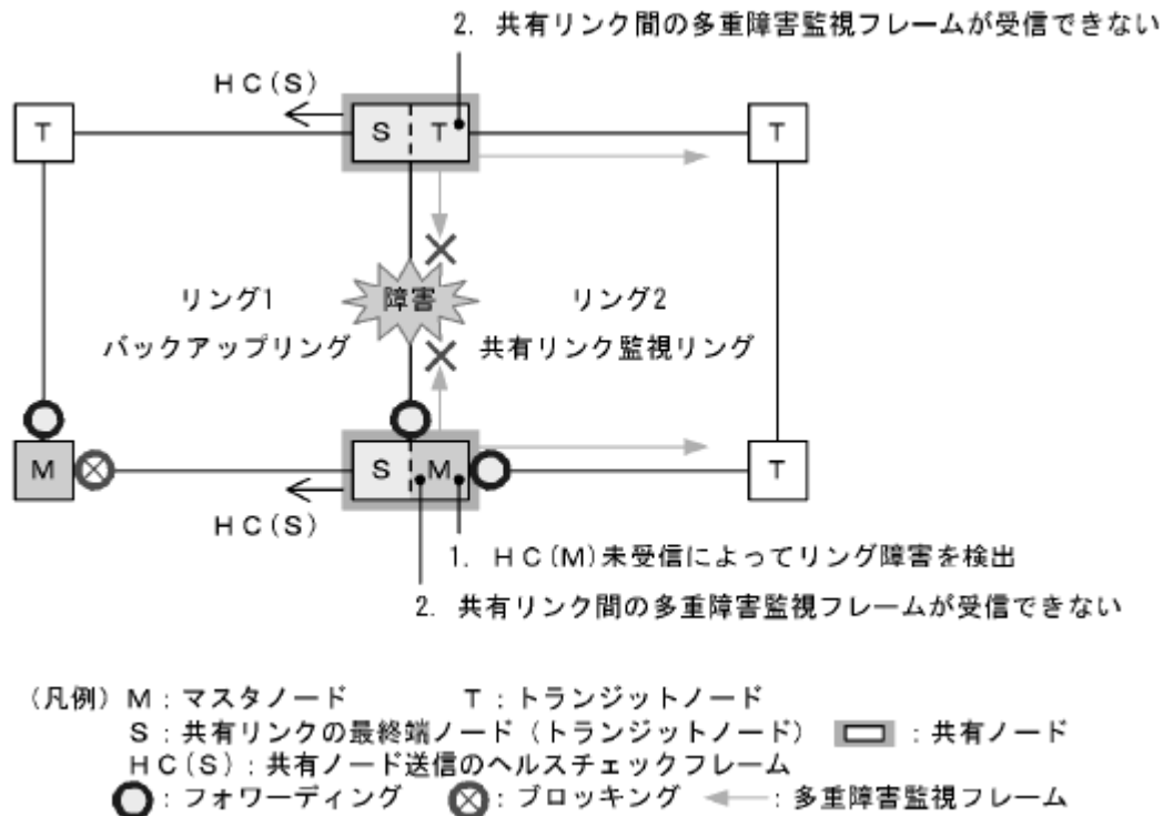
図 20-24 共有リンク障害時の動作
