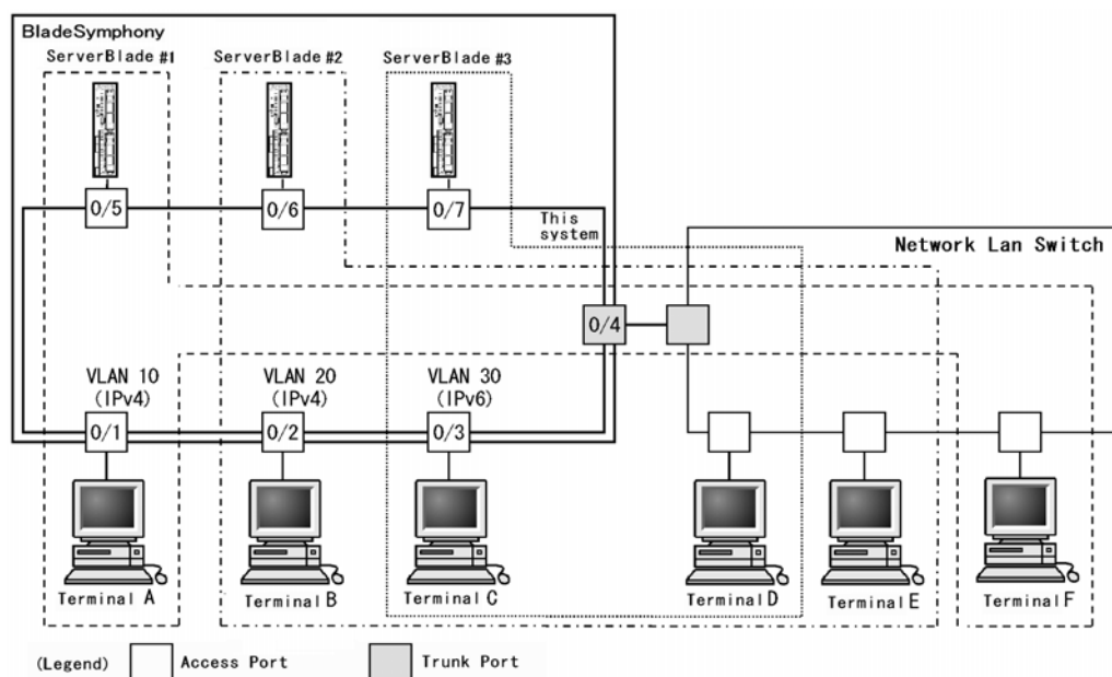
図 17-7 プロトコル VLAN の設定例
