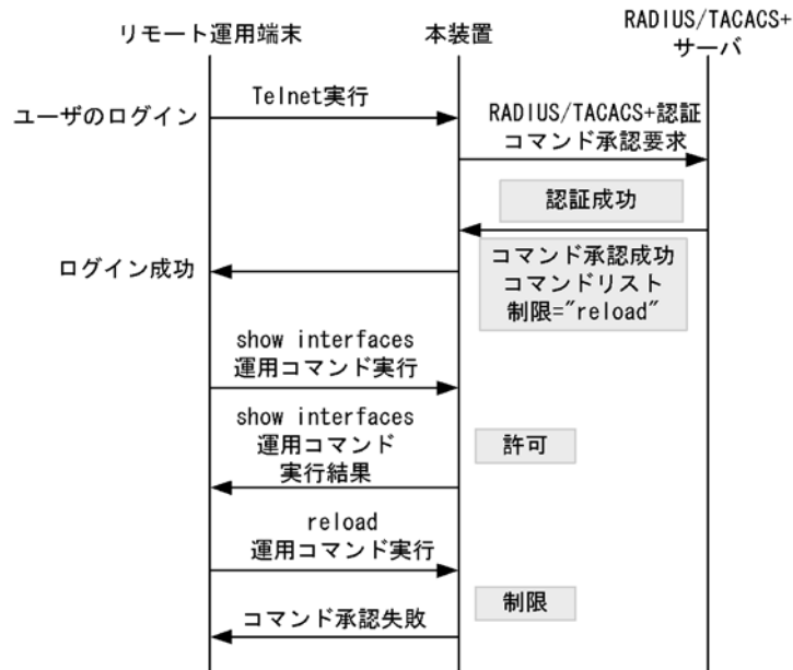
図 7-17 RADIUS/TACACS+ サーバによるコマンド承認のシーケンス
