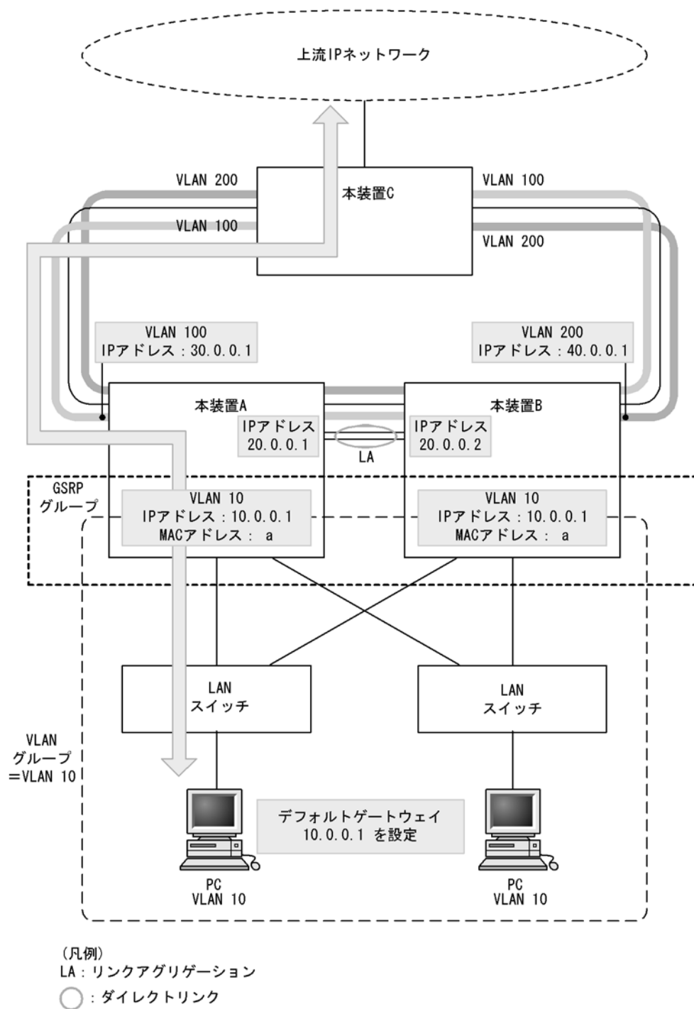
図 22-12 レイヤ 3 冗長切替機能（通常運用時）
