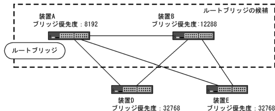
図 19-17 装置 A, 装置 B をルートブリッジの候補として運用
