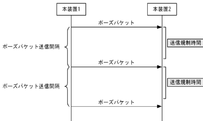
図 13-5 ルーズモードでの動作シーケンス
