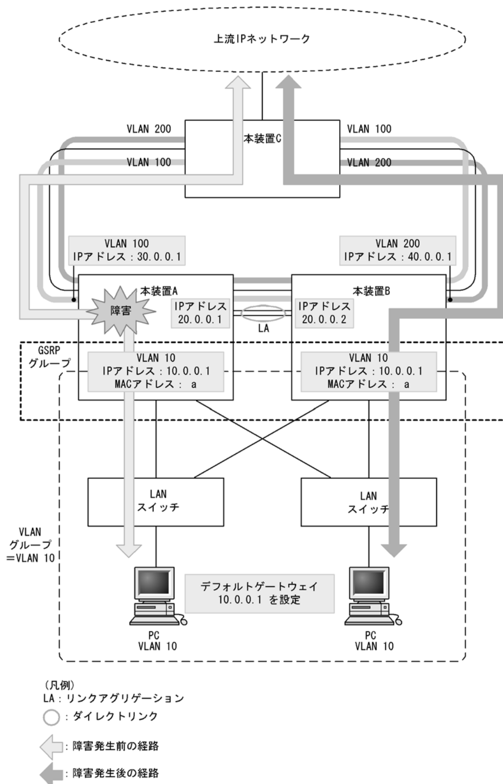
図 22-13 レイヤ 3 冗長切替機能（障害発生時）
