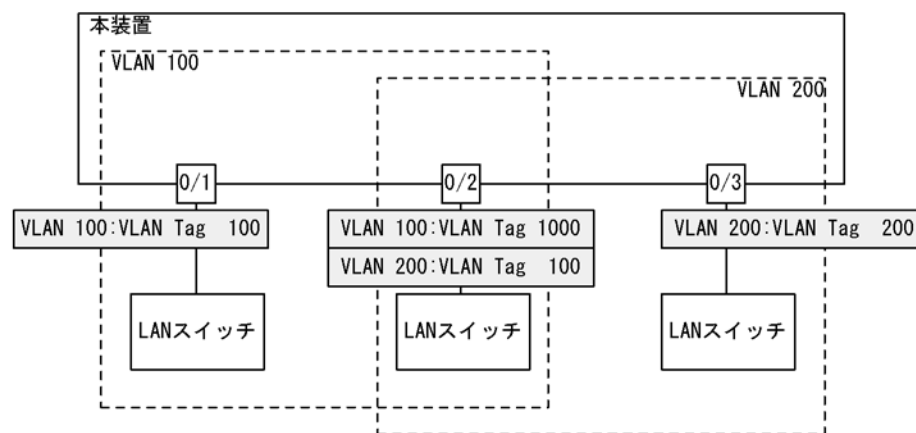
図 18-3 Tag 変換の設定例
