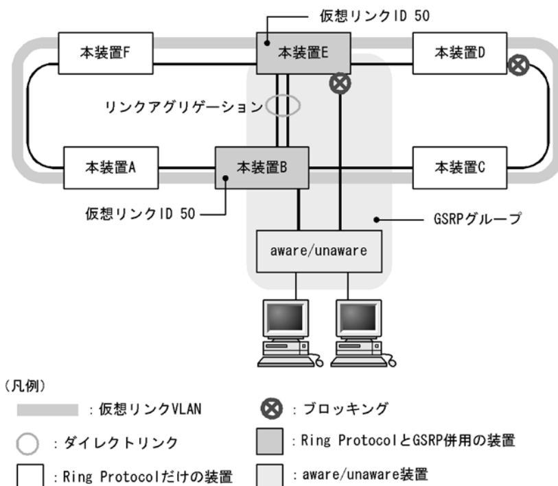
図 22-11 仮想リンク ID の設定
