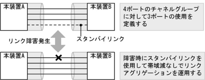
図 14-3 スタンバイリンク機能の構成例
