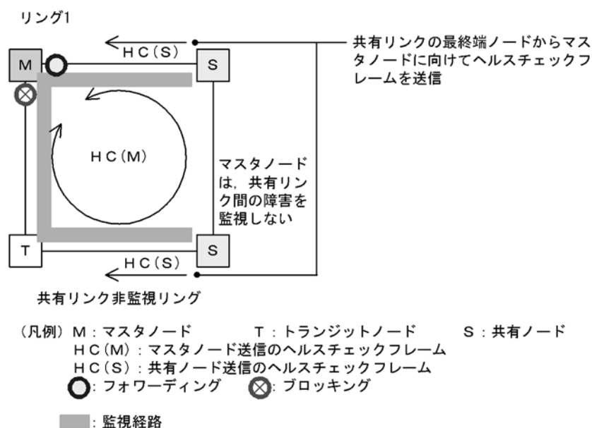
図 20-13 共有リンク非監視リングでの正常時の動作
