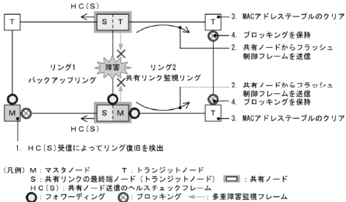
図 20-28 バックアップリングからの切り戻し動作
