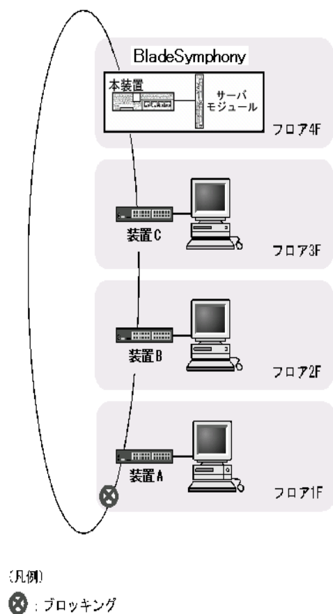
図 20-1 Ring Protocol の適用例（その 1）
