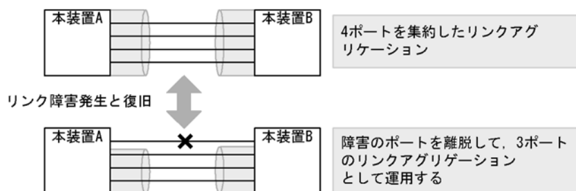
図 14-1 リンクアグリゲーションの構成例
