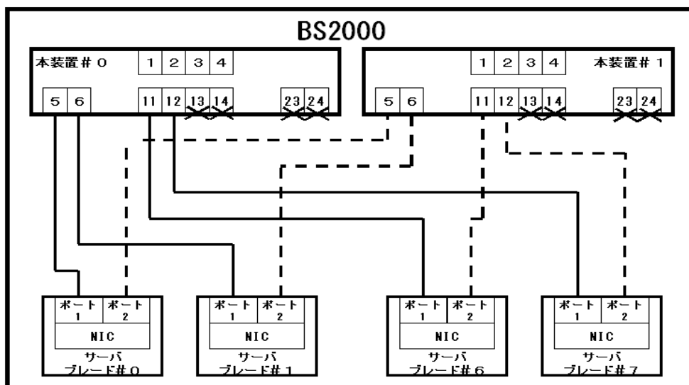
図 13-8 BS2000 のサーバ接続ポートとサーバモジュールの接続
