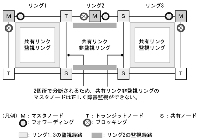
図 20-34 共有リンク監視リングが複数ある構成
