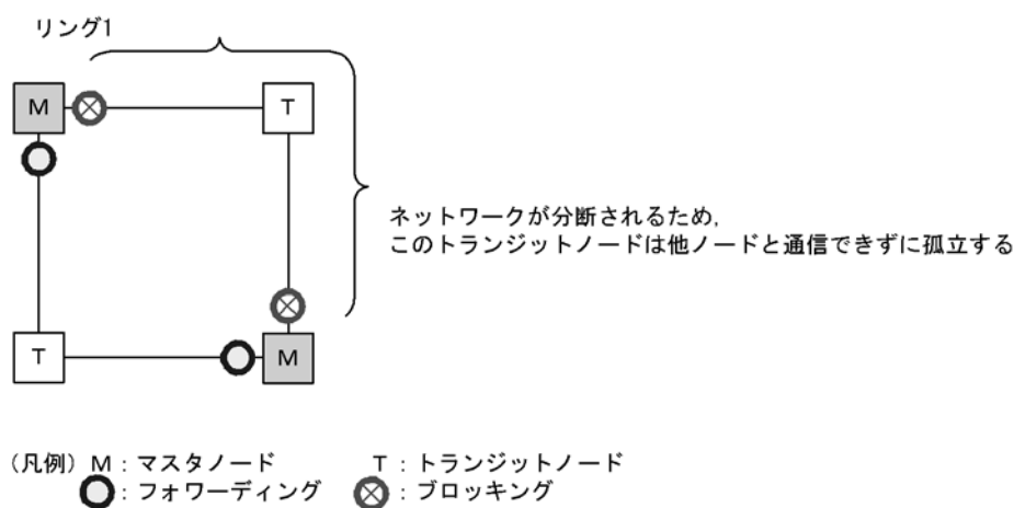
図 20-33 同一リング内に複数のマスタノードを設定
