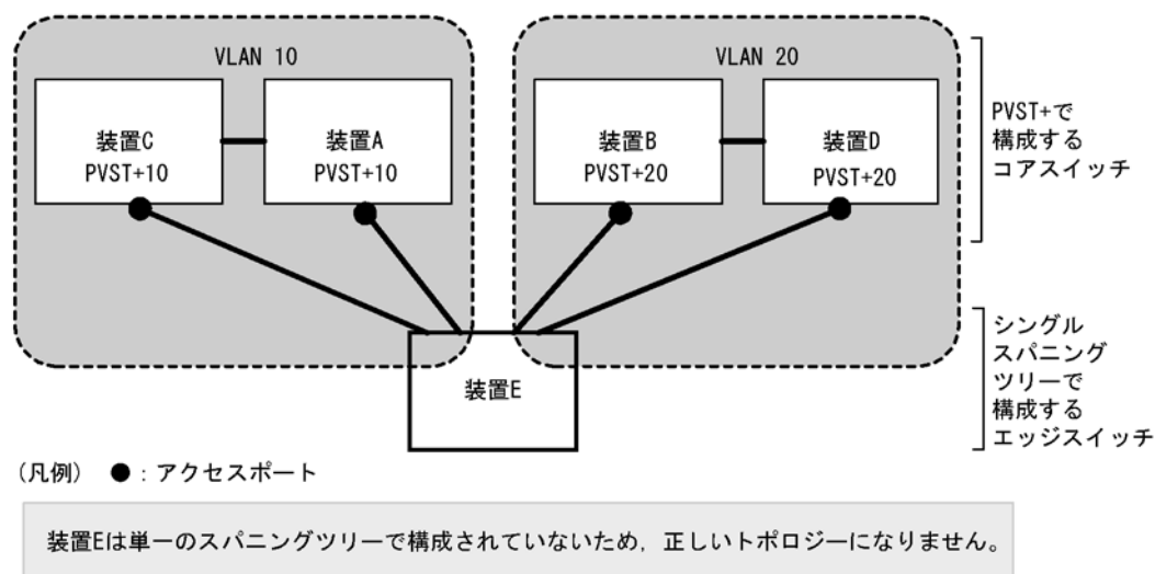
図 19-7 シングルスパニングツリーとの禁止構成例
