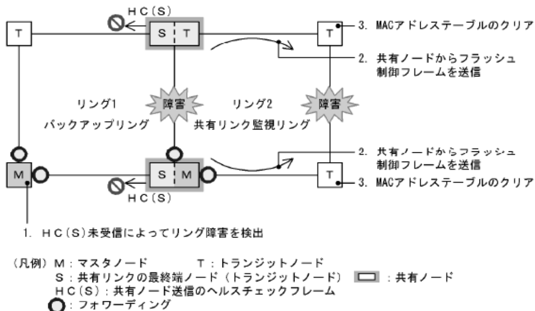
図 20-26 バックアップリングへの切り替え動作
