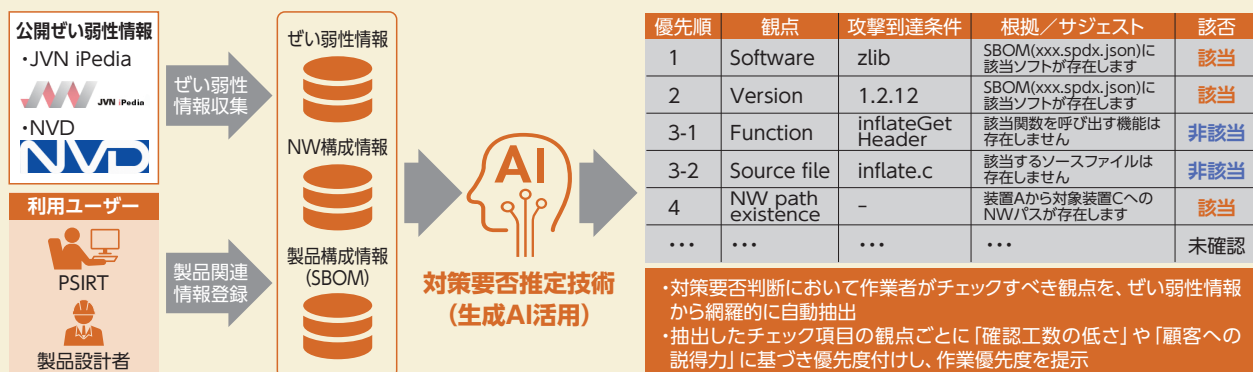
図表4-② ぜい弱性対策要否推定技術の概要
