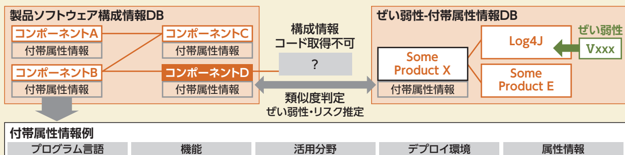
図表4-③ ソフトウェアの類似度に基づくぜい弱性リスク推定技術の概要
