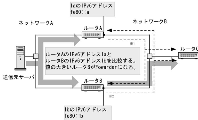
図 27-14 Forwarder の決定
