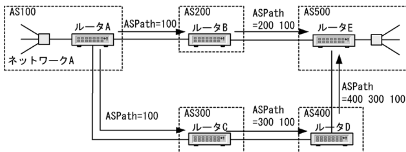
図 25-3 AS_PATH 属性による経路選択
