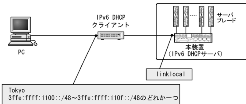
図 19-2 動的にプレフィックスを割り当てる構成
