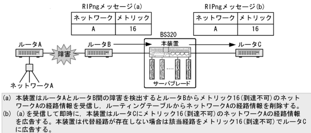
図 22-4 ルートポイズニング
