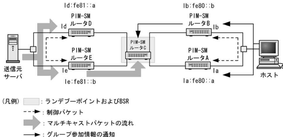
図 27-15 DR の動作
