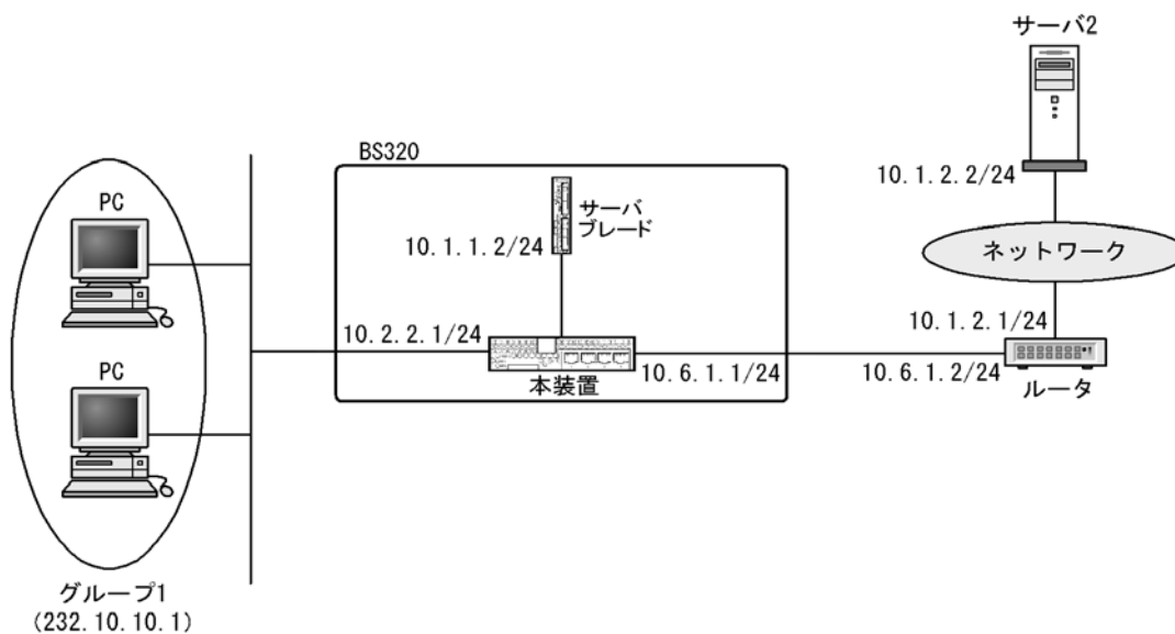
図 14-2 PIM-SSM 構成例
