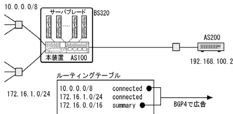
図 6-17 集約経路を BGP4 で広告する構成
