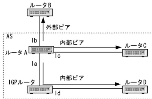
図 11-7 通知する経路情報の NEXT_HOP 属性の設定例
