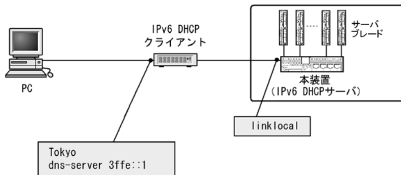
図 19-3 クライアントにオプション情報を配布する構成
