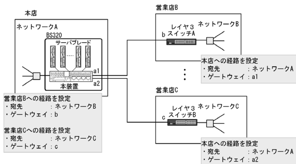
図 21-1 スタティックルーティングのネットワーク構成例
