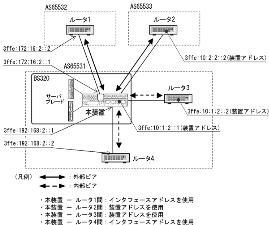
図 25-8 接続構成例
