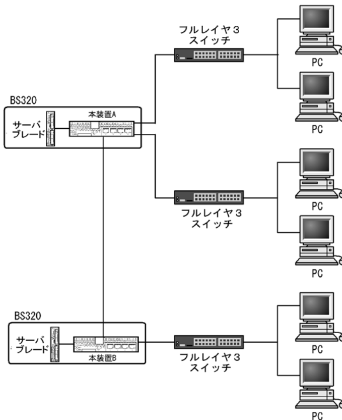
図 27-21 IPv6 PIM-SSM を使用する構成図
