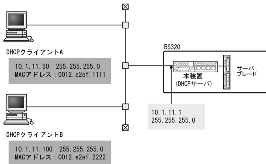
図 5-2 クライアント-サーバ構成 (固定 IP アドレス配布時)
