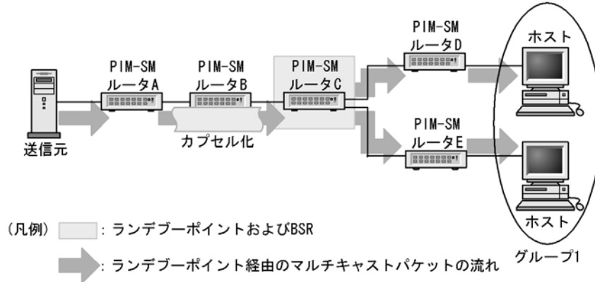
(d) ランデブーポイント経由のマルチキャストパケット通信（デカプセル化）
