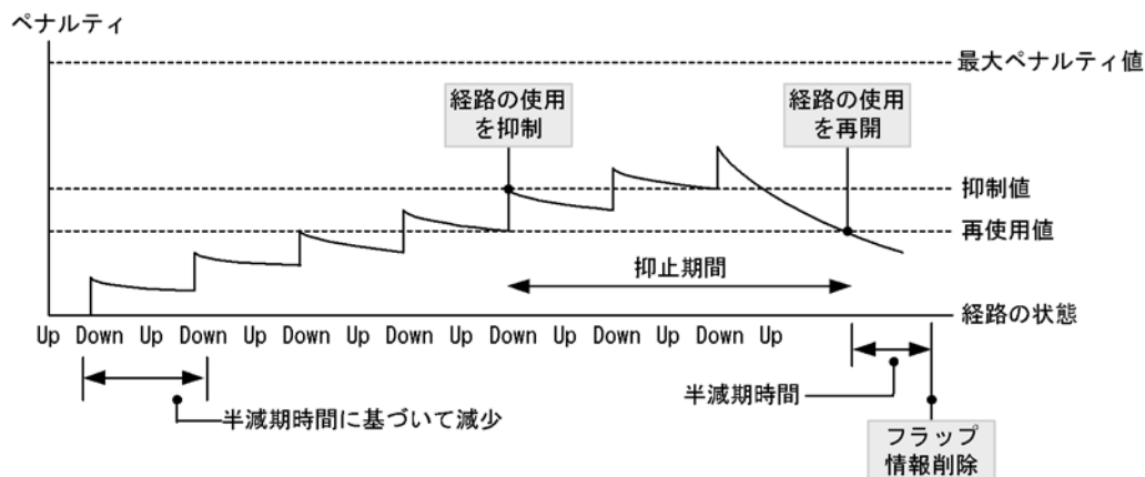
図 11-20 ルート・フラップ・ダンプニングの動作概念
