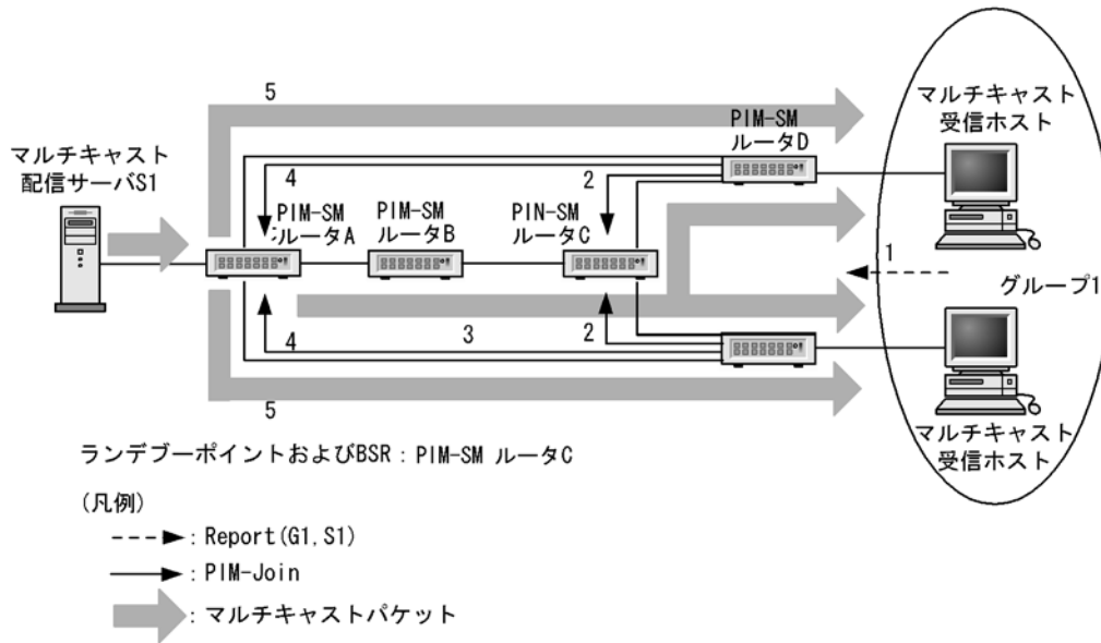
図 27-16 MLDv2 使用時の IPv6 PIM-SM 動作概要
