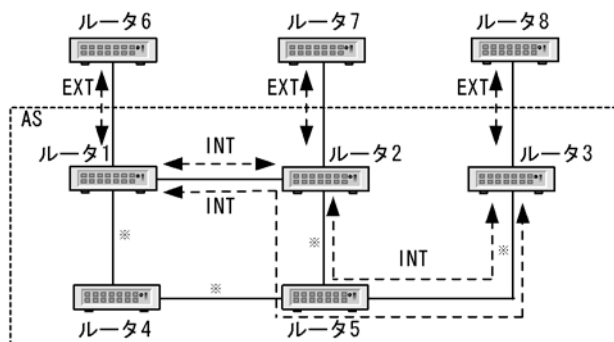
図 25-1 内部ピアと外部ピア
