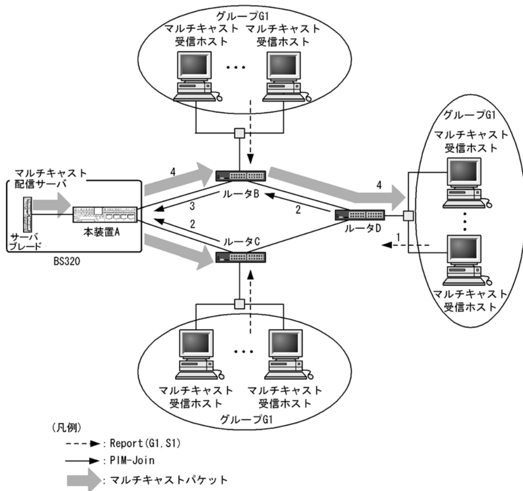
図 13-18 IGMPv3 使用時の IPv4 PIM-SSM 動作概要
