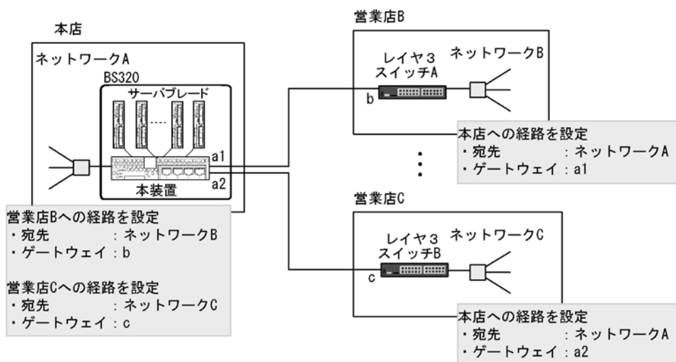
図 7-1 スタティックルーティングのネットワーク構成例
