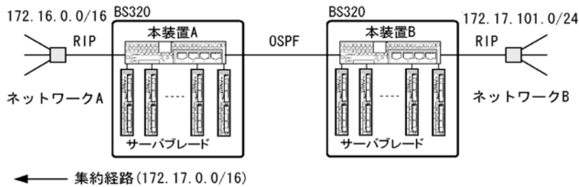
図 6-7 集約経路の広告の例
