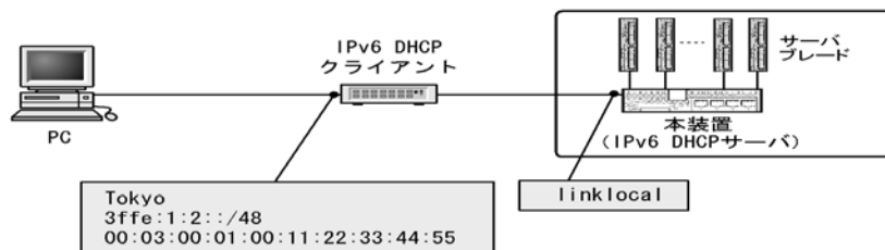
図 19-1 クライアントごとに固定プレフィックスを指定する構成
