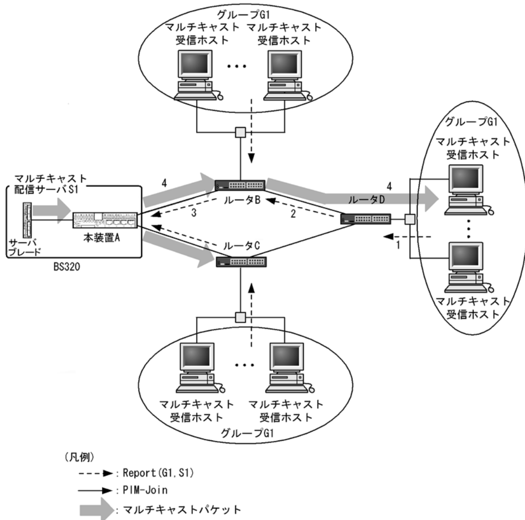
図 27-19 MLDv2 使用時の IPv6 PIM-SSM 動作概要
