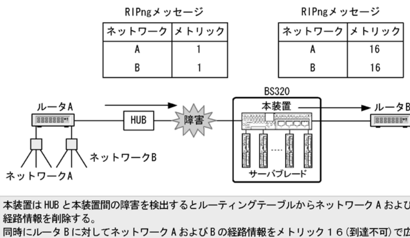
図 22-2 triggered update による経路情報の広告
