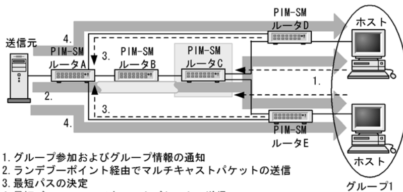
図 13-7 PIM-SM の動作概要
