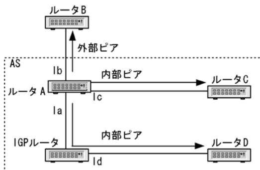
図 25-7 通知する経路情報のネクストホップの設定例
