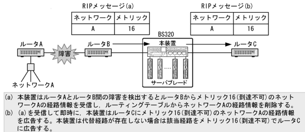
図 8-4 ルートポイズニング
