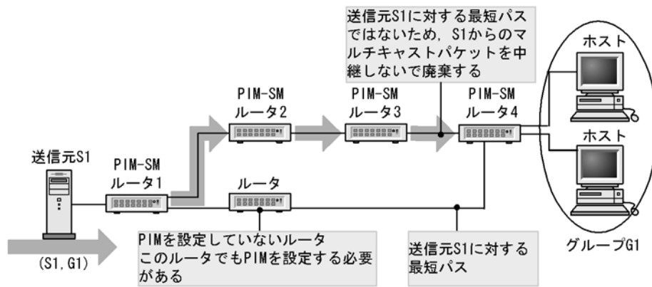
図 27-17 冗長経路時の注意事項
