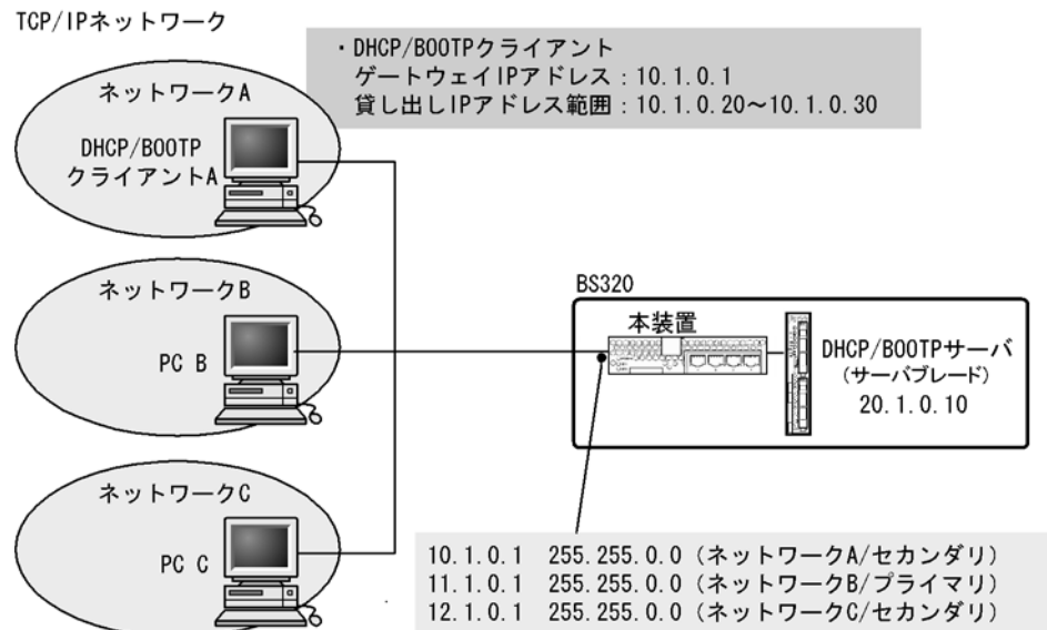
図 4-2 マルチホーム構成
