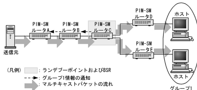
図 27-10 IPv6 マルチキャストパケット通信（デカプセル化）
