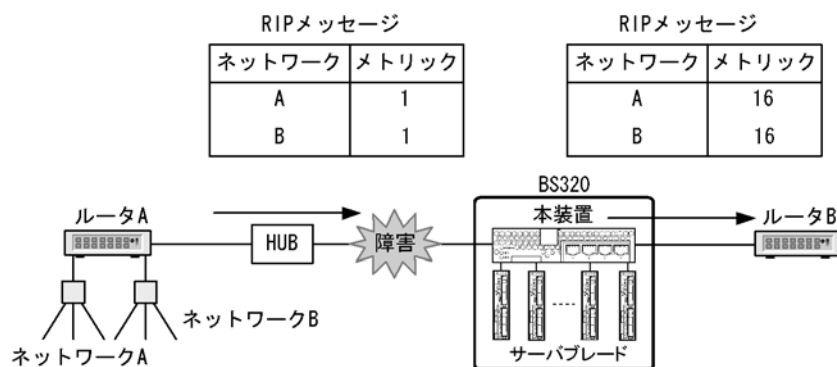
図 8-2 triggered update による経路情報の広告
