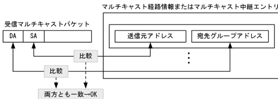
図 13-6 マルチキャスト経路情報またはマルチキャスト中継エントリの検索方法
