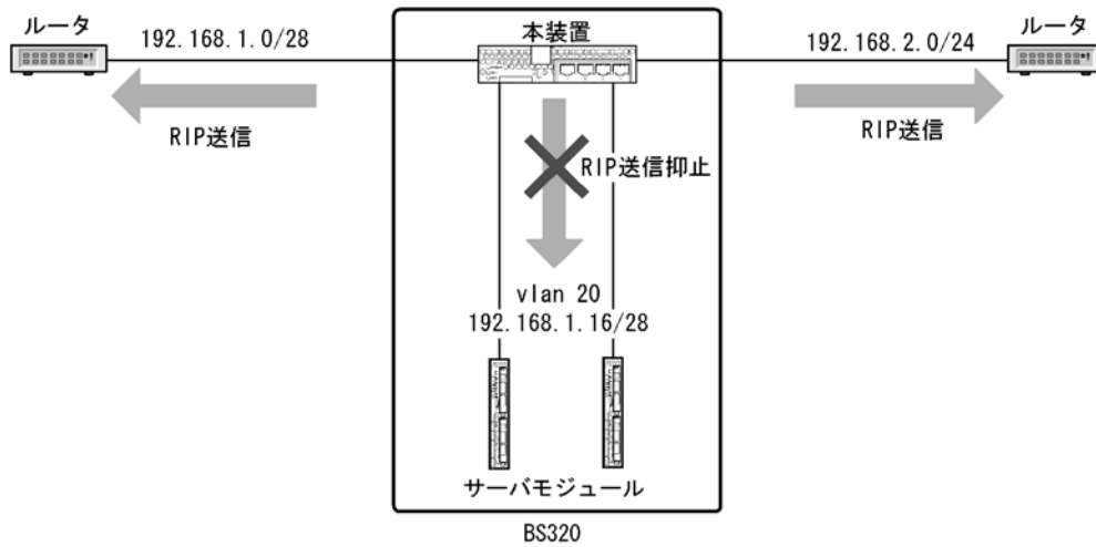
図 8-13 RIP パケットの送信抑制
