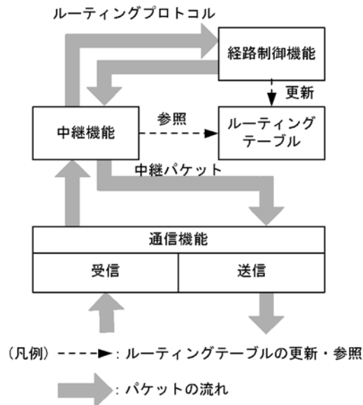
図 15-17 IPv6 ルーティング機能の概要
