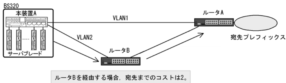
図 23-5 マルチパスの構成
