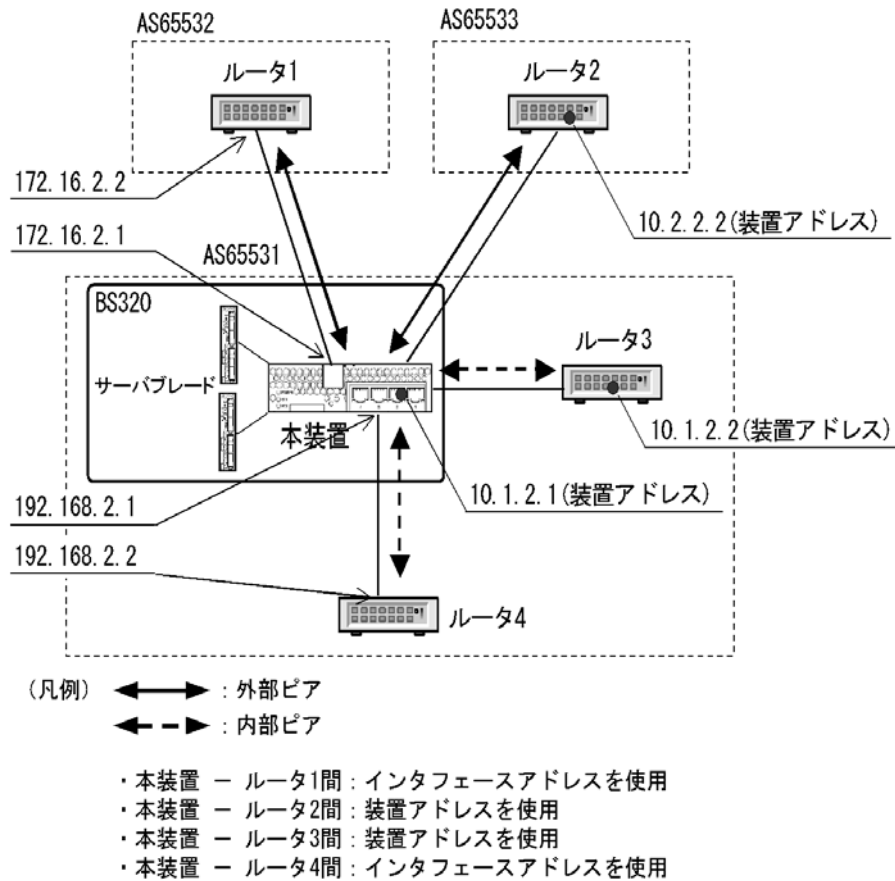
図 11-8 接続構成例
