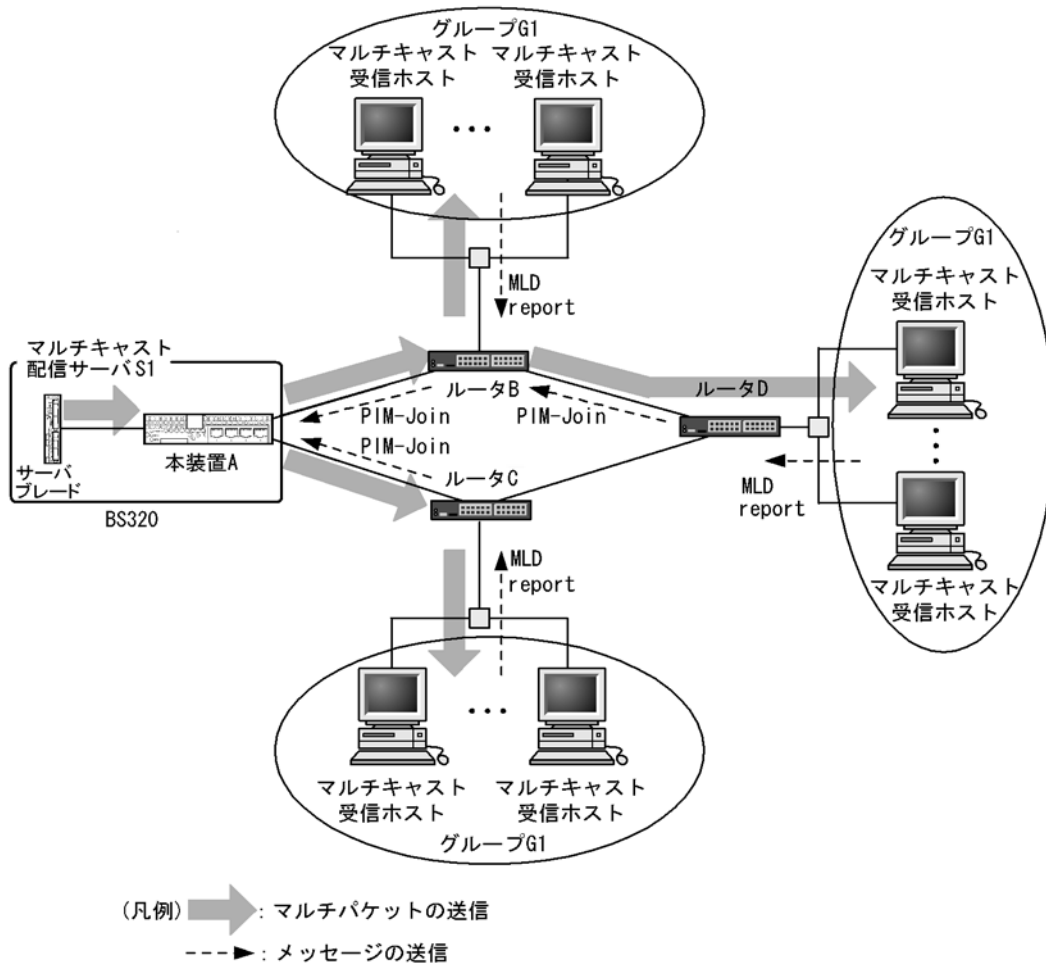
図 27-18 IPv6 PIM-SSM の動作概要
