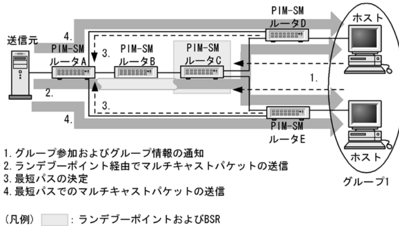
図 27-6 PIM-SM の動作概要
