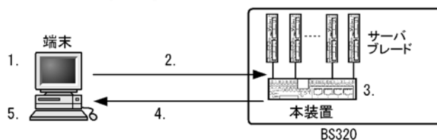
図 18-1 RA による端末のアドレス設定
