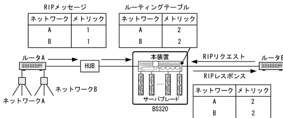
図 8-3 リクエストパケット受信による経路情報の広告
