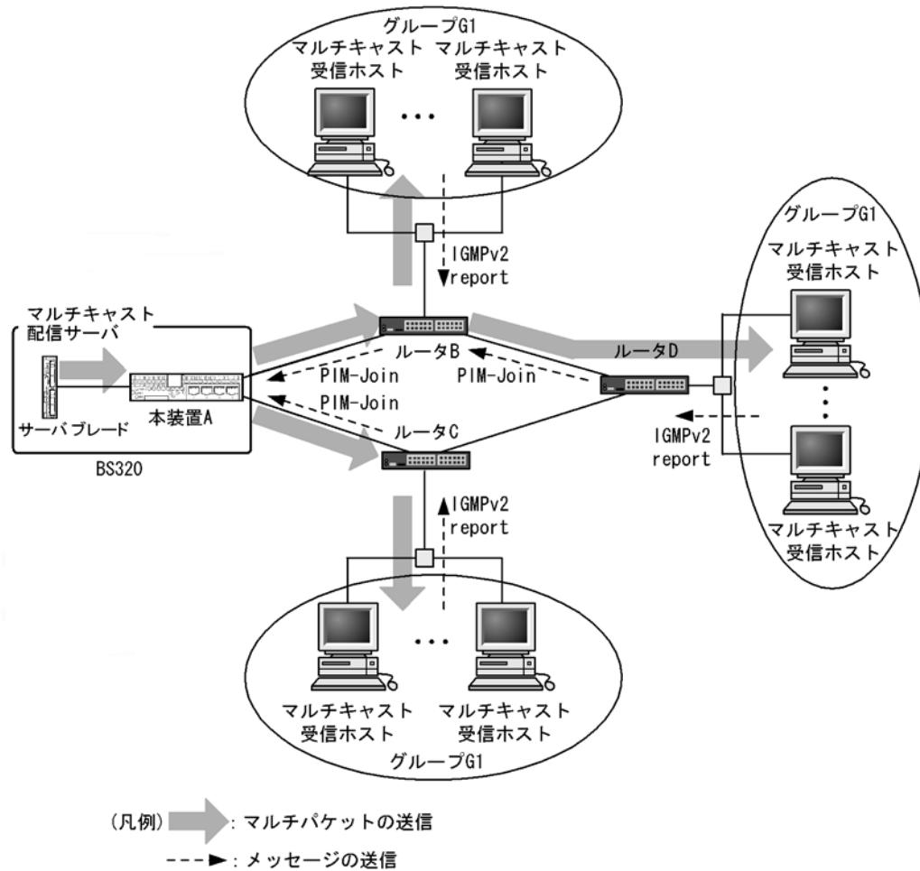
図 13-17 PIM-SSM の動作概要
