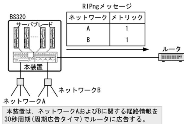
図 22-1 周期的な経路情報広告
