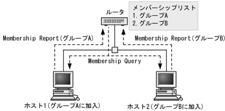
図 13-3 IGMPv2 グループの参加・離脱
