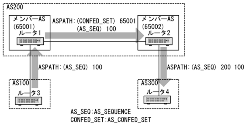
図 11-24 AS_PATH 属性の取り扱い
