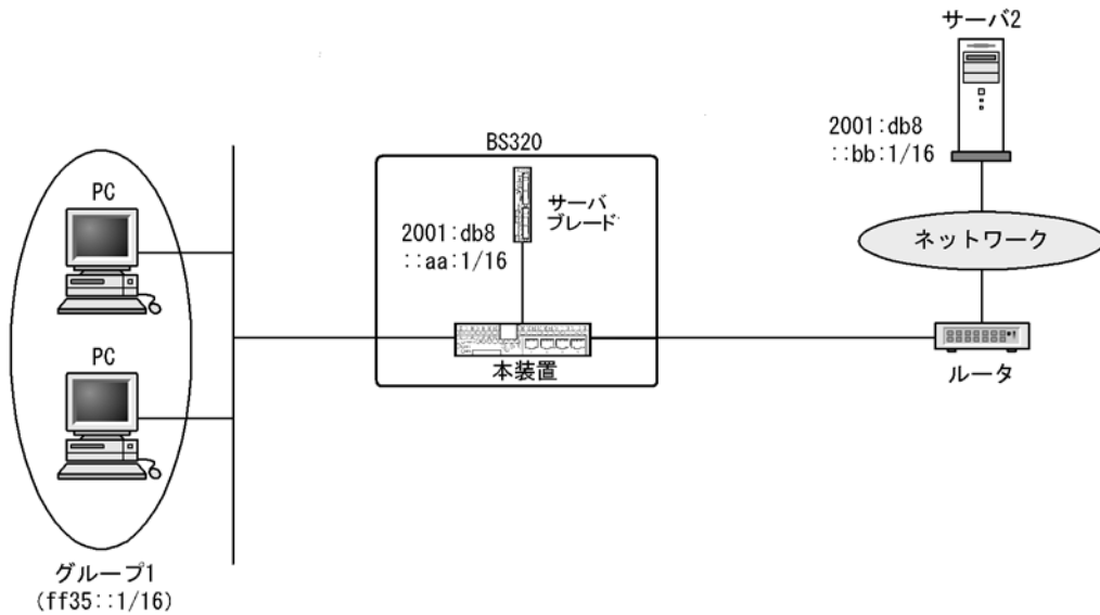
図 28-1 PIM-SSM 構成例
