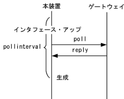
図 7-3 スタティック経路の動的監視による経路生成
