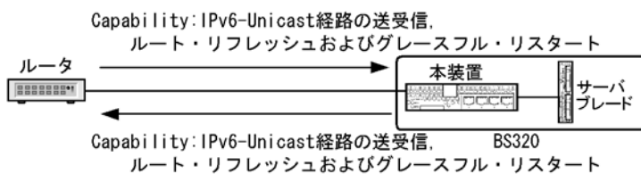
図 25-13 ネゴシエーションの動作概念
