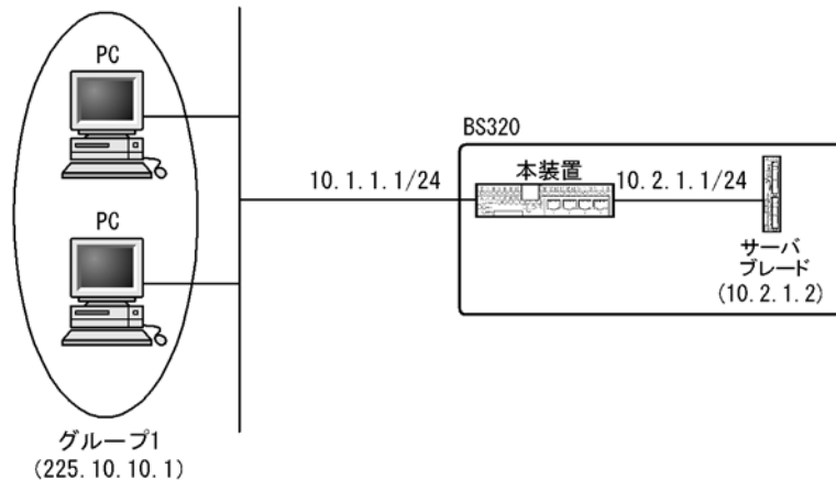
図 14-1 PIM-SM 構成例
