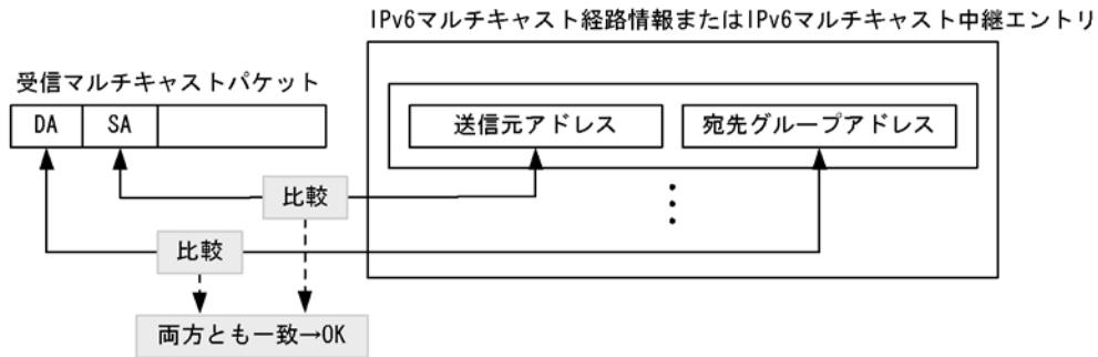
図 27-5 IPv6 マルチキャスト経路情報または IPv6 マルチキャスト中継エントリの検索方法
