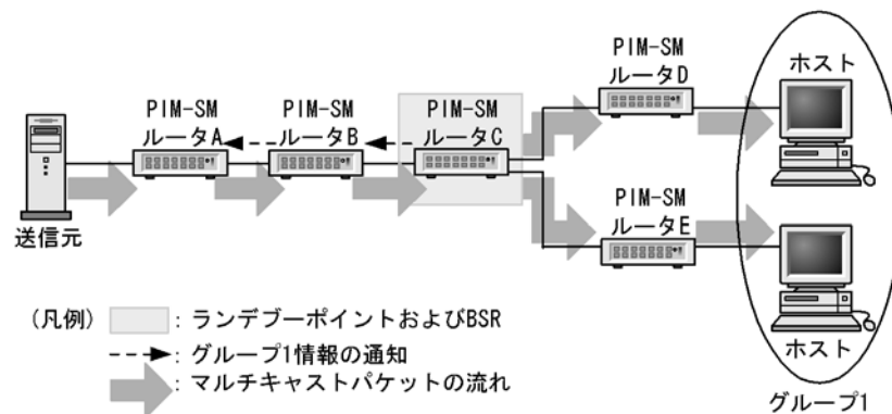
図 13-11 ランデブーポイント経由のマルチキャストパケット通信（デカプセル化）
