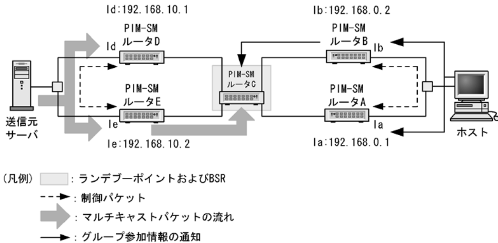
図 13-15 DR の動作
