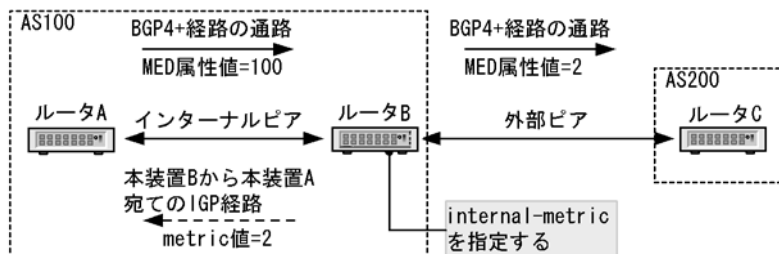
図 25-6 set metric-type internal の使用例
