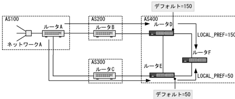
図 25-2 LOCAL_PREF 属性による経路選択
