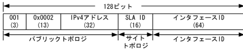
図 15-14 6to4 アドレス
