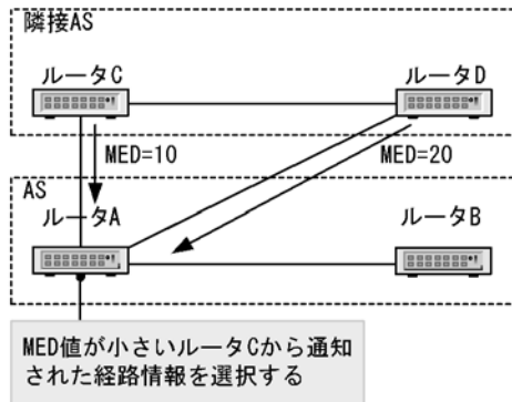
図 25-5 MED 属性による経路選択
