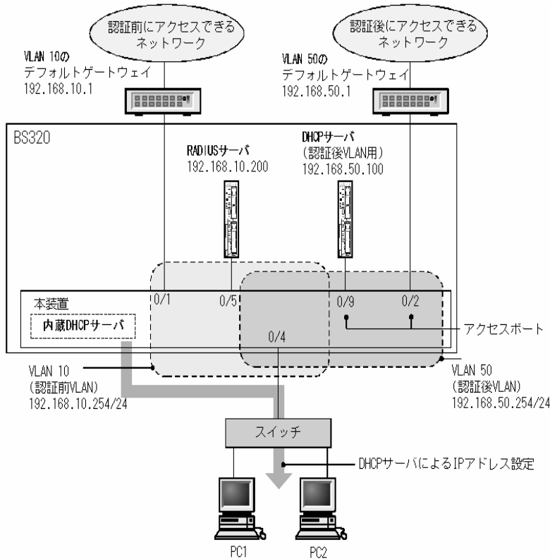
図 7-33 ダイナミック VLAN モードの RADIUS 認証方式の基本構成
