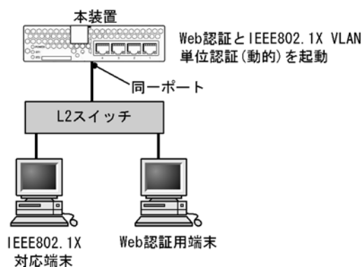
図 7-25 IEEE802.1X（VLAN 単位認証（動的））との共存
