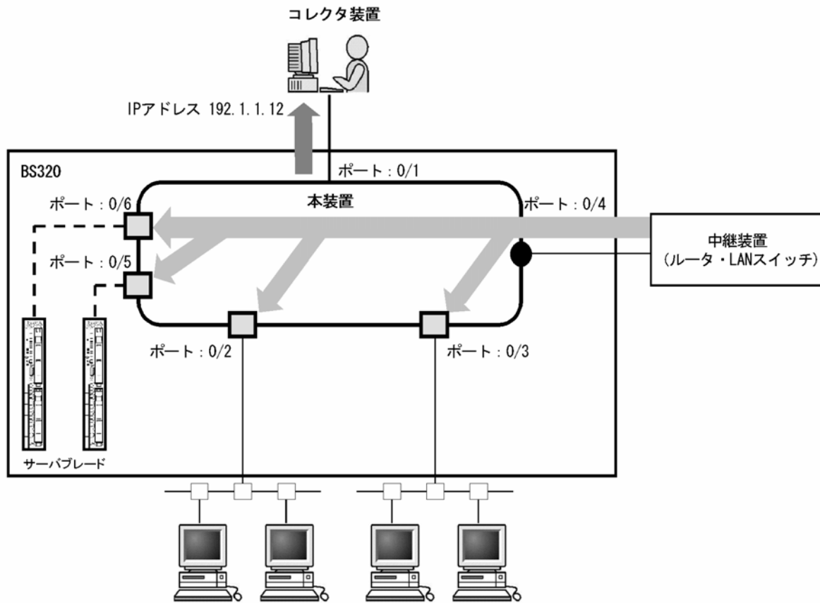
図 18-7 ポート 0/4 の受信パケットをモニタする設定例
