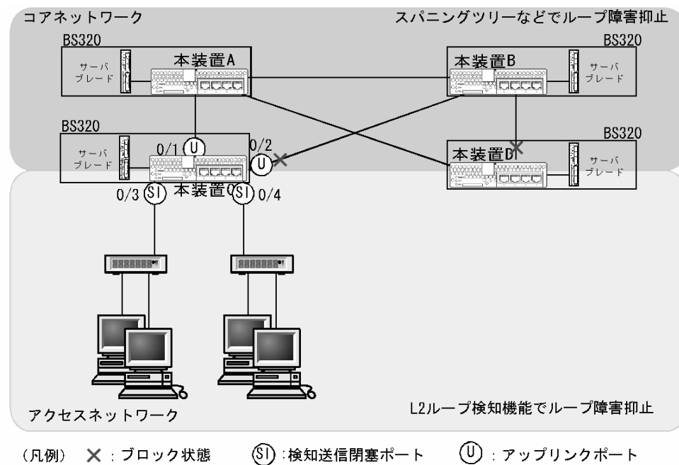
図 15-3 L2 ループ検知の設定例
