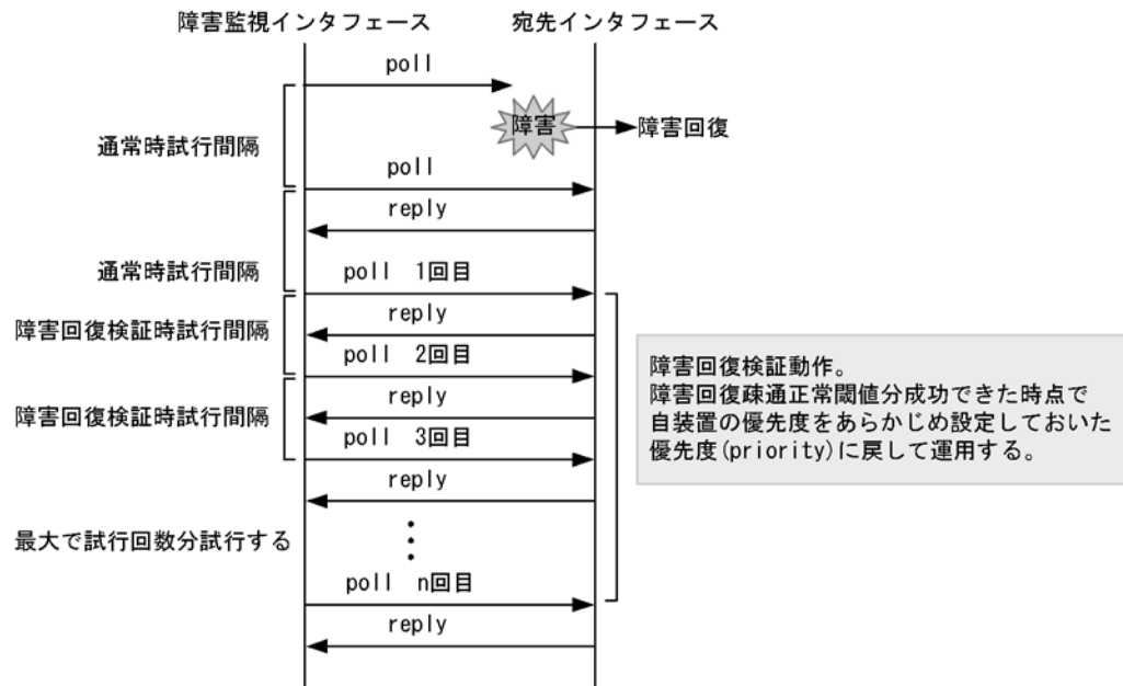
図 11-9 障害回復動作シーケンス
