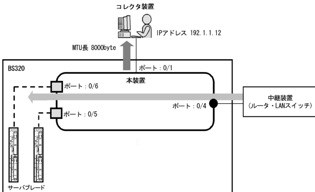
図 18-9 コレクタ装置への送信を MTU=8000byte に設定する例
