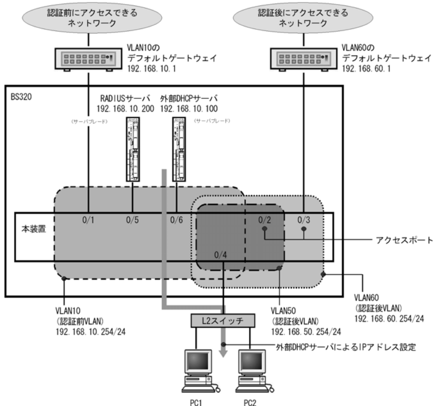
図 7-38 Web 認証の RADIUS 認証方式+外部 DHCP サーバ+複数認証後 VLAN 使用時の構成例
