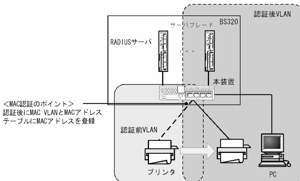
図 8-5 ダイナミック VLAN モードの RADIUS 認証方式の構成
