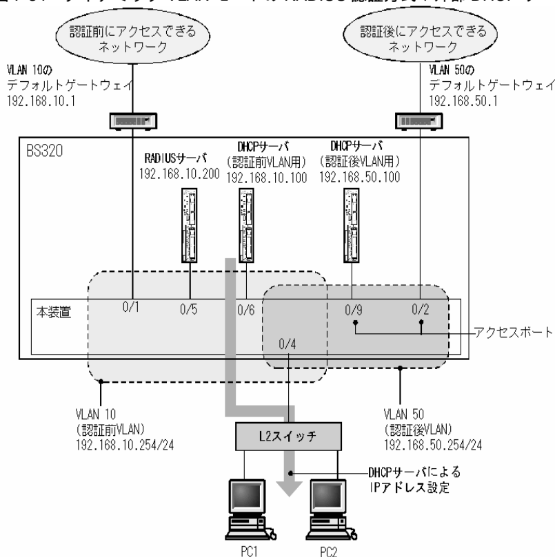
図 7-34 ダイナミック VLAN モードの RADIUS 認証方式+外部 DHCP サーバ使用時の構成
