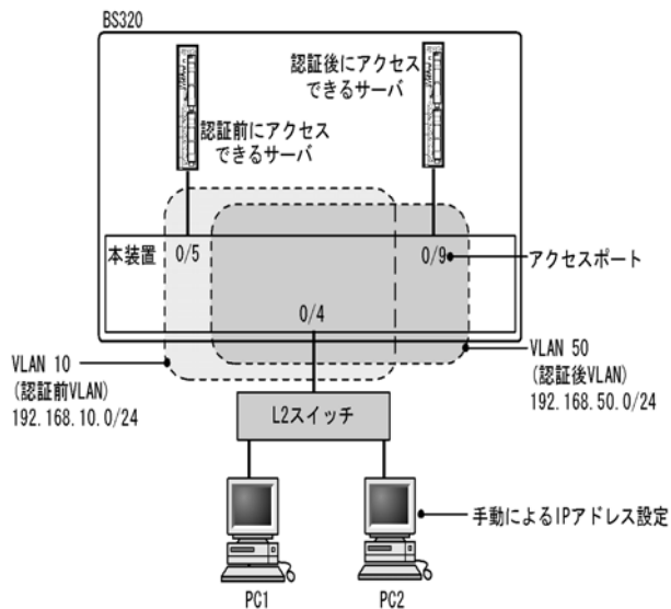
図 7-35 ローカル認証方式の構成例
