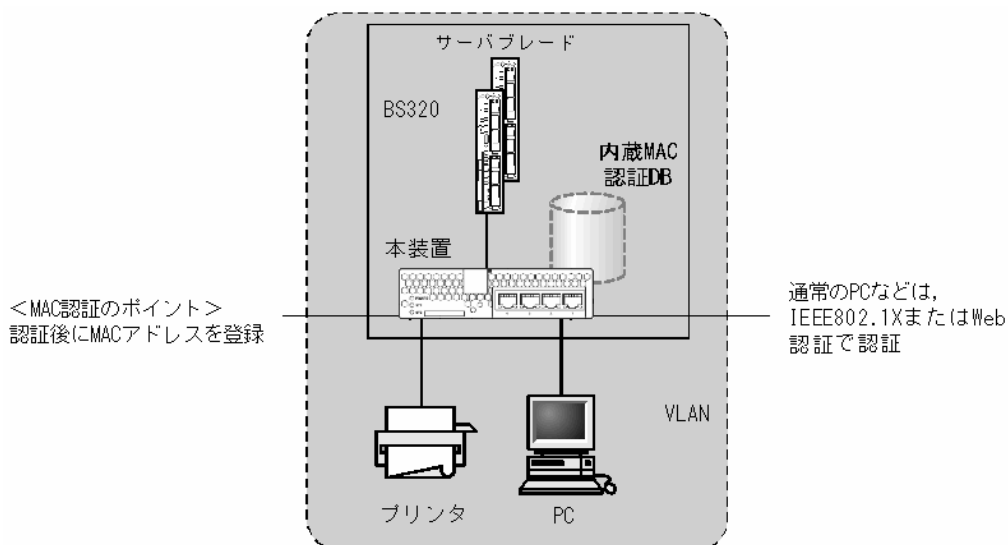
図 8-1 固定 VLAN モードのローカル認証方式の構成
