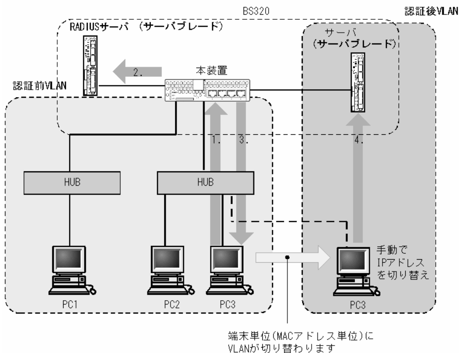
図 7-11 ダイナミック VLAN モードの RADIUS 認証方式の構成
