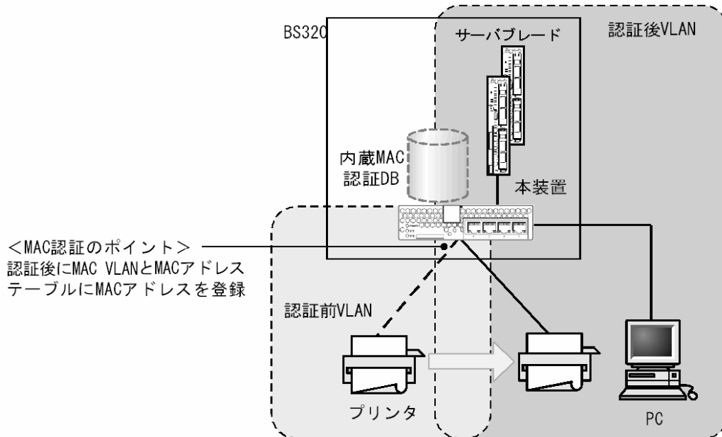
図 8-4 ダイナミック VLAN モードのローカル認証方式の構成
