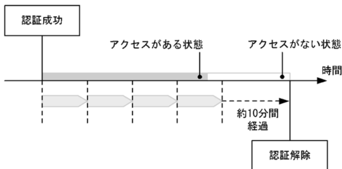
図 7-20 認証済み端末の MAC アドレステーブルエージングによるログアウト
