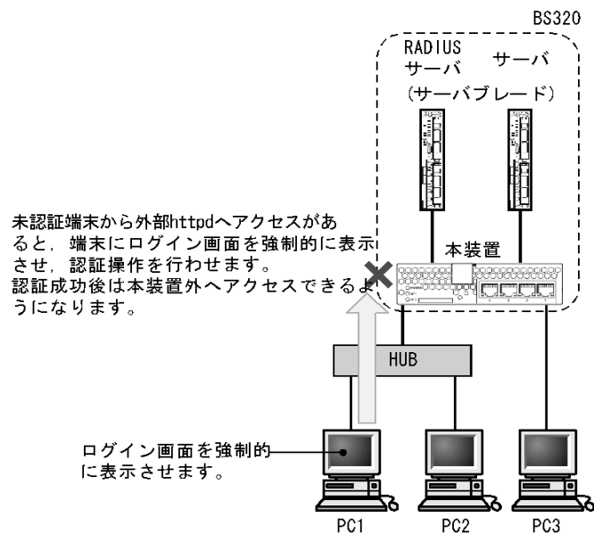
図 7-1 固定 VLAN モード時の URL リダイレクト機能
