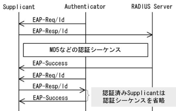
図 5-9 shortcut, disable, full の EAP-Request/Identity のシーケンス
