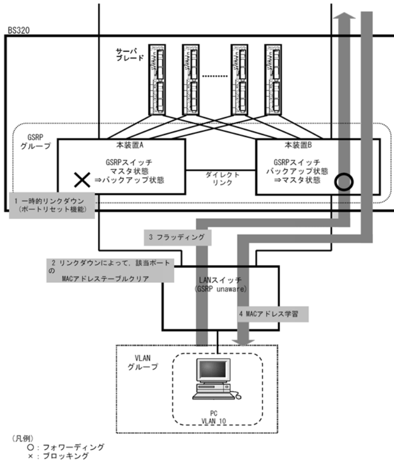
図 9-4 ポートリセット機能による切り替え制御の概要
