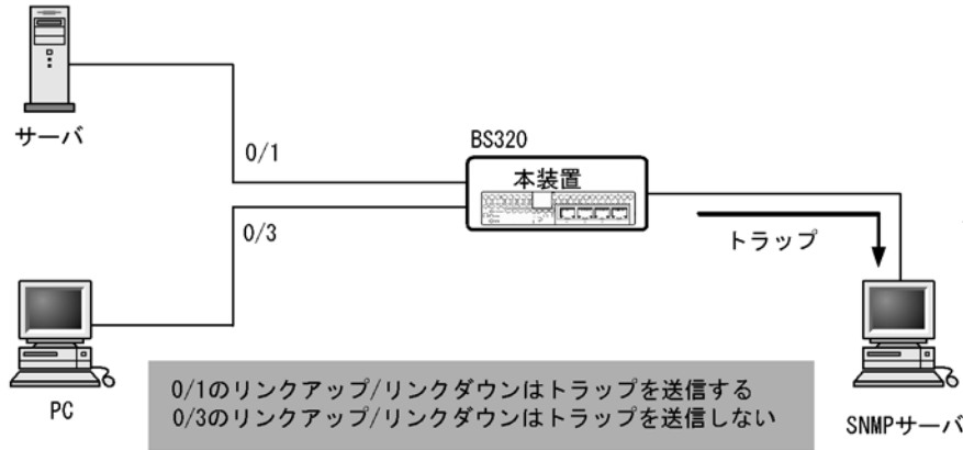
図 16-26 リンクトラップの構成図
