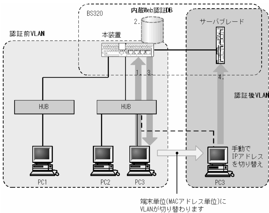
図 7-10 ダイナミック VLAN モードのローカル認証方式の構成
