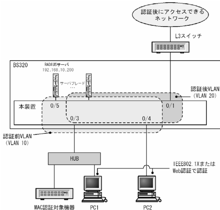
図 8-15 ダイナミック VLAN モードの RADIUS 認証方式の基本構成
