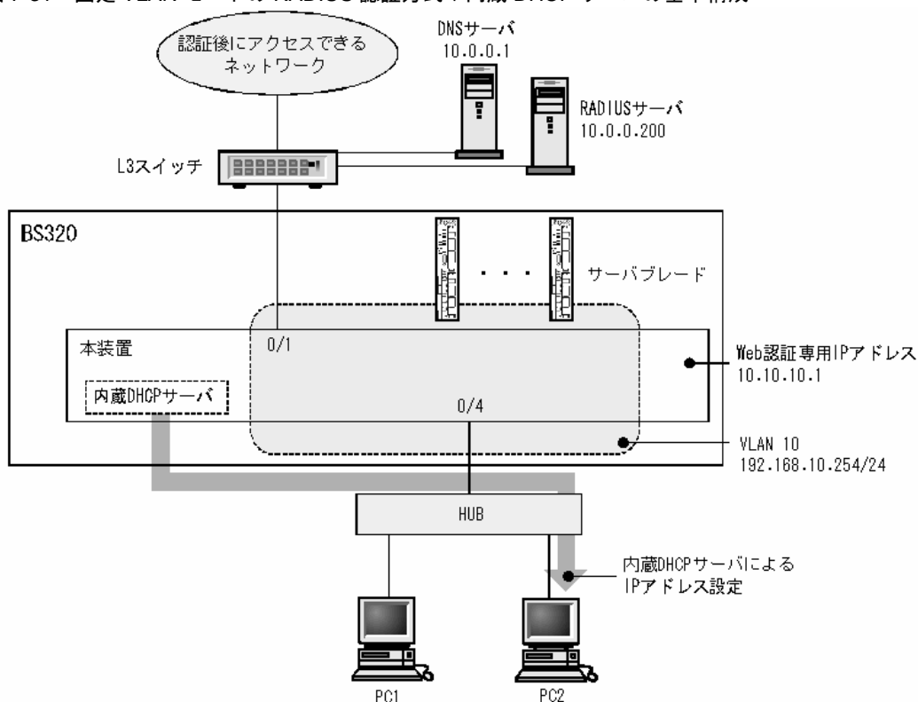
図 7-31 固定 VLAN モードの RADIUS 認証方式+内蔵 DHCP サーバの基本構成
