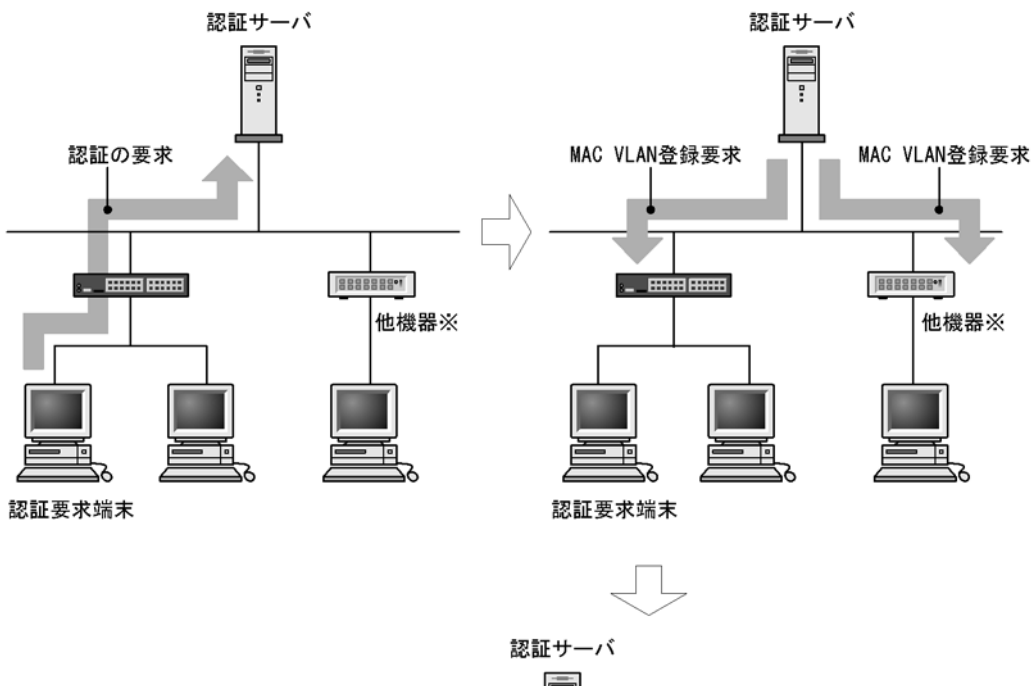
図 11-7 VRRP ポーリングを設定した場合と設定していない場合の比較
