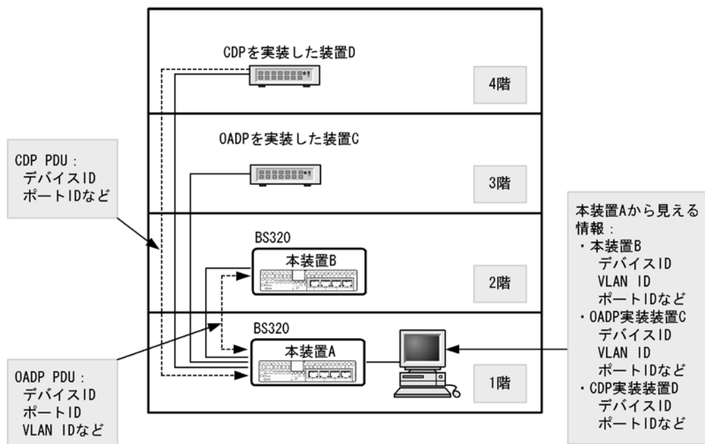
図 20-1 OADP の適用例
