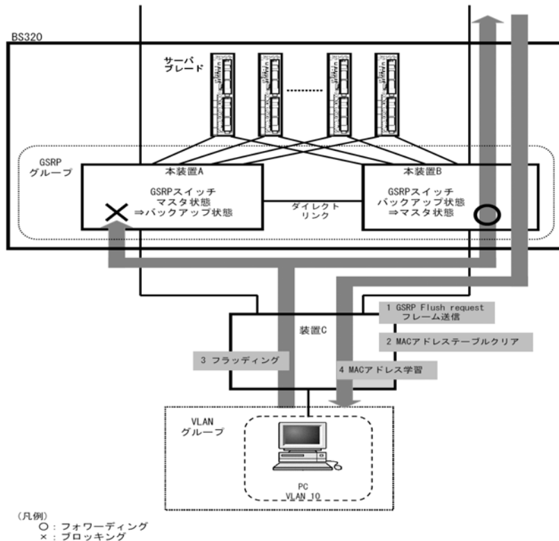
図 9-3 GSRP Flush request フレームによる切り替え制御の概要
