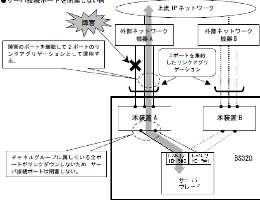
図 12-2 リンクアグリゲーション機能 (スタティック) と併用時の本機能の動作例
