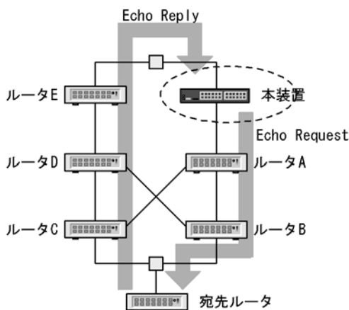
図 11-10 送受信インタフェースが一致しない場合
