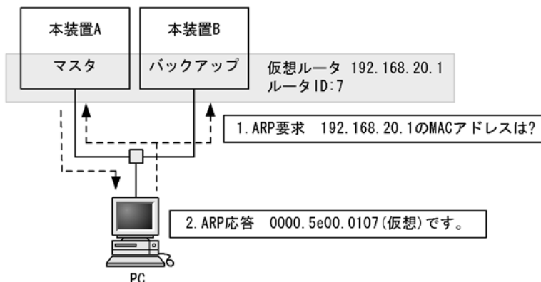
図 11-2 仮想 MAC アドレスによる ARP 応答および NDP 応答
