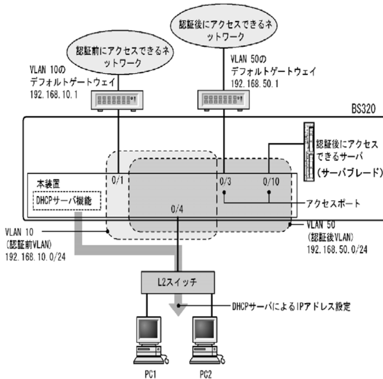
図 7-36 ローカル認証方式+内蔵 DHCP 使用時の構成例
