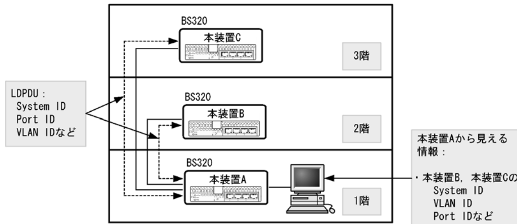
図 19-1 LLDP の適用例
