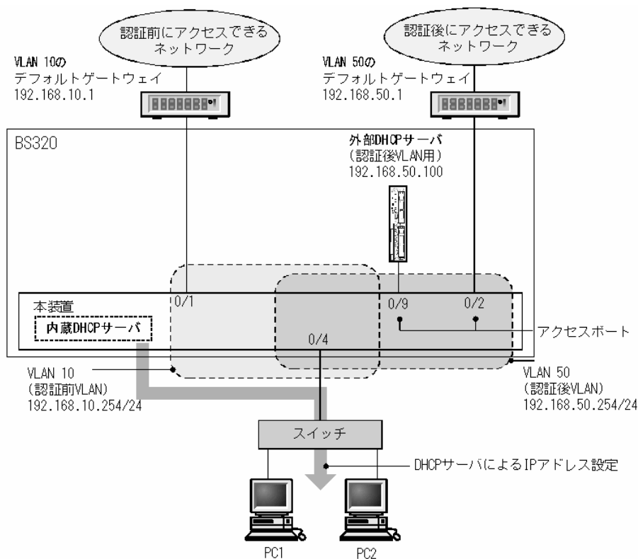
図 7-32 ダイナミック VLAN モードのローカル認証方式の基本構成
