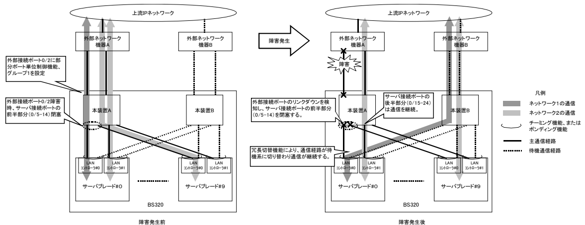
図 12-3 部分ポート単位制御機能を使用した構築例
