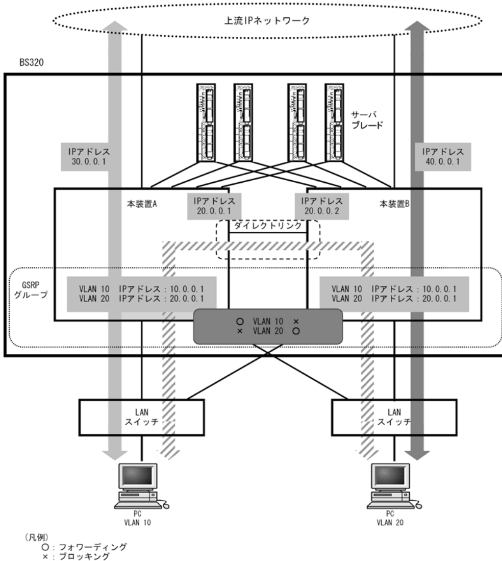
図 9-11 レイヤ 3 冗長切替機能使用時のロードバランス構成
