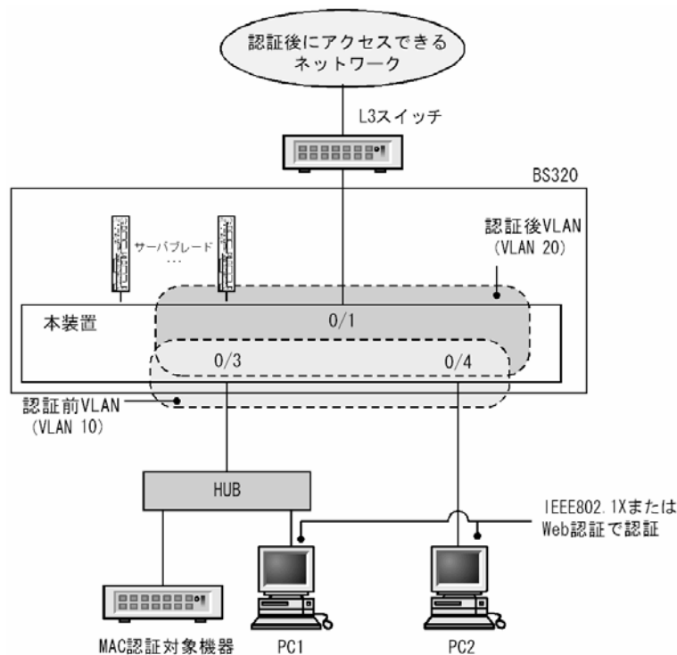
図 8-14 ダイナミック VLAN モードのローカル認証方式の基本構成
