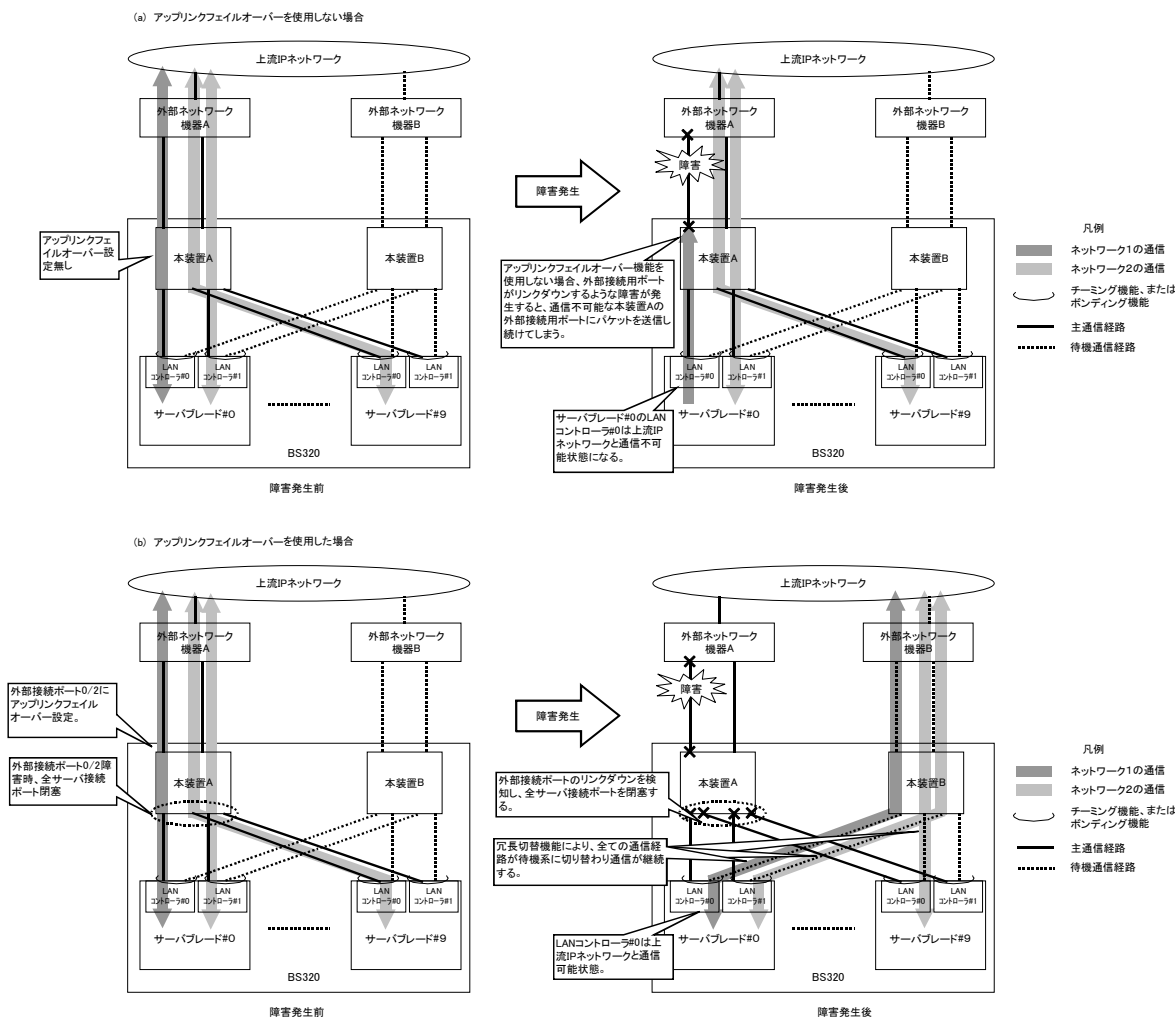
図 12-1 アップリンクフェイルオーバーの構築例
