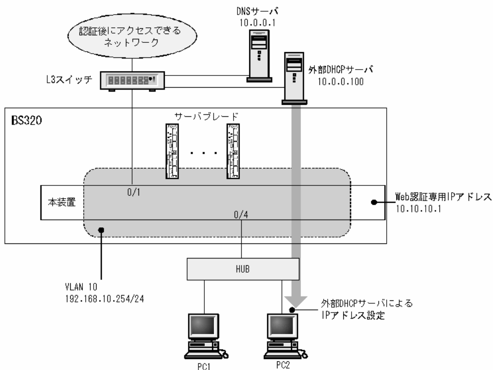
図 7-29 固定 VLAN モードのローカル認証方式の基本構成
