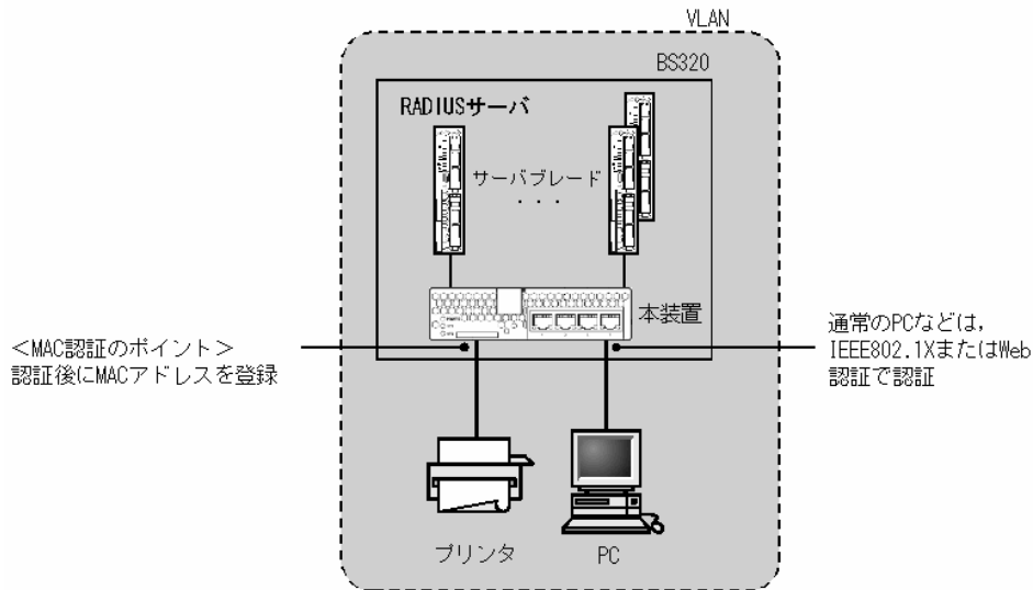
図 8-2 固定 VLAN モードの RADIUS 認証方式の構成
