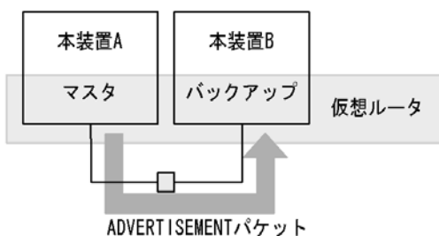
図 11-3 ADVERTISEMENT パケットの送出
