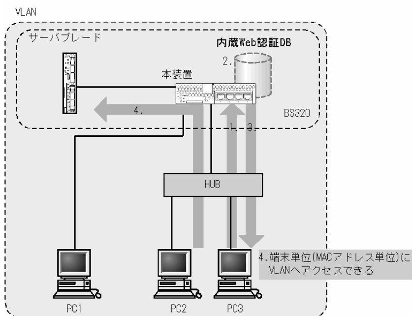
図 7-7 固定 VLAN モード時のローカル認証方式の構成
