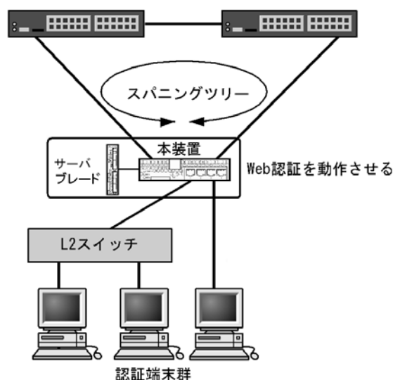
図 7-27 スパニングツリー使用時の構成例
