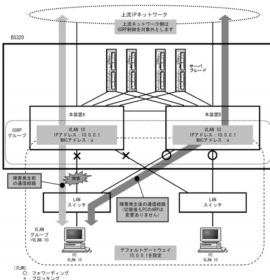
図 9-8 GSRP レイヤ 3 冗長切替機能の概要
