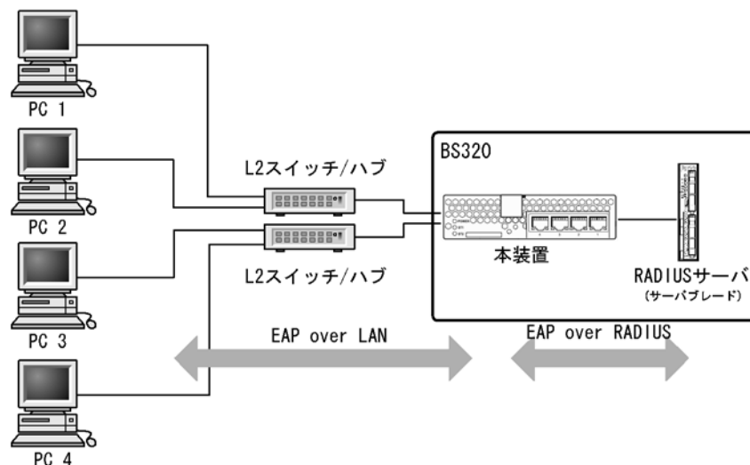
図 5-2 端末との間に L2 スイッチを配置した IEEE802.1X 構成
