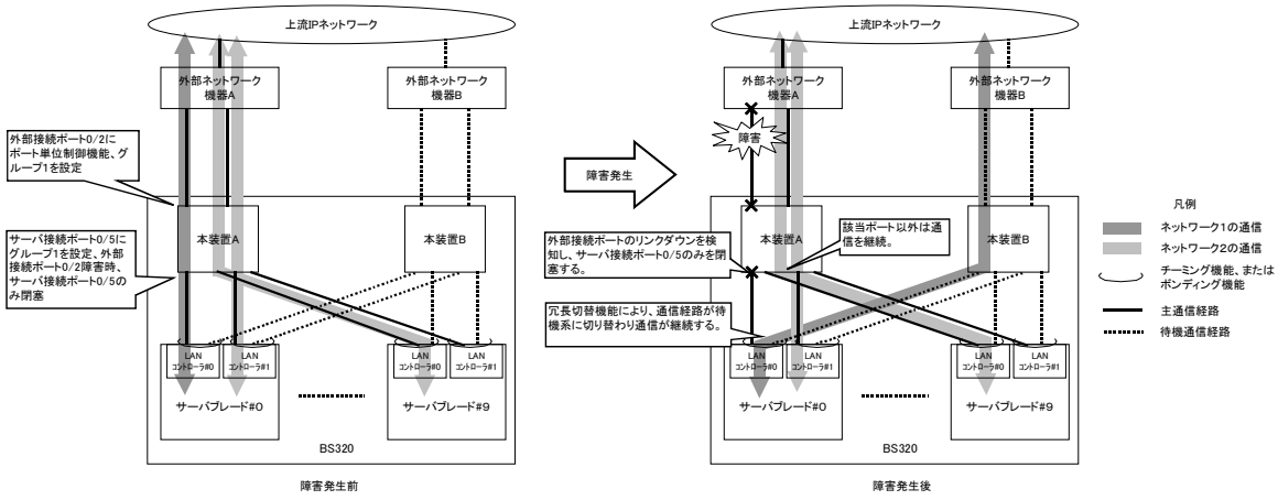
図 12-4 部分ポート単位制御機能を使用した構築例
