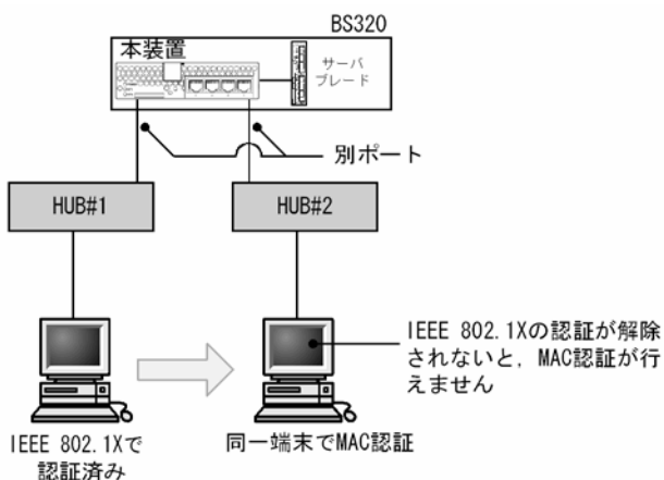
図 8-11 IEEE802.1X で認証されている端末のポート移動後の MAC 認証使用
