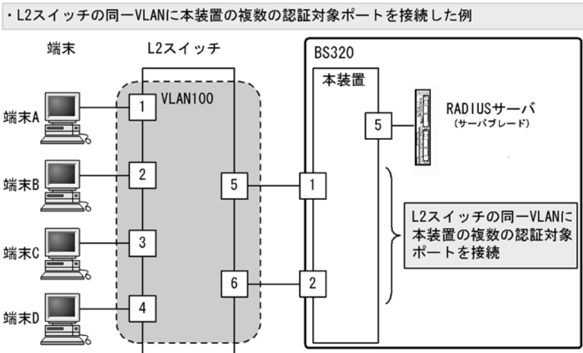
図 5-10 禁止構成例
