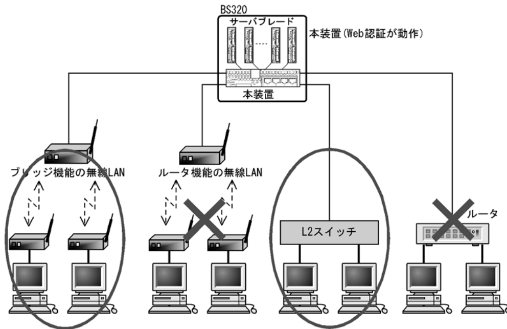
図 7-28 本装置と端末間の接続
