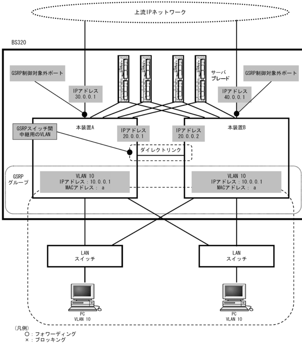
図 9-13 上流ネットワークの障害に対応した設定
