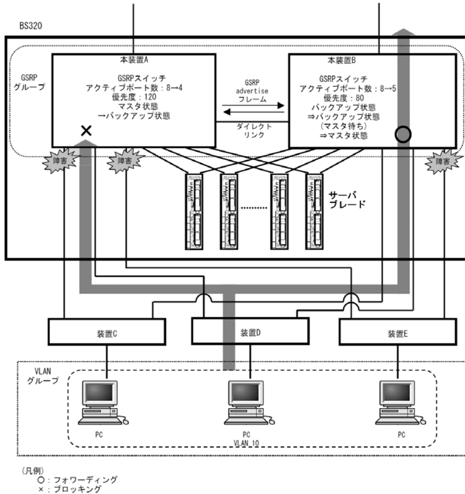
図 9-7 リンク障害時の動作例
