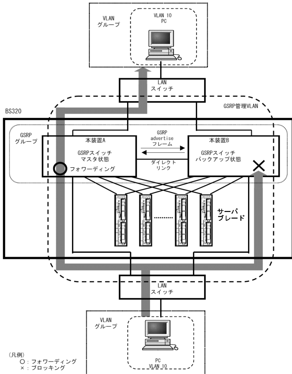
図 9-2 GSRP のネットワーク構成
