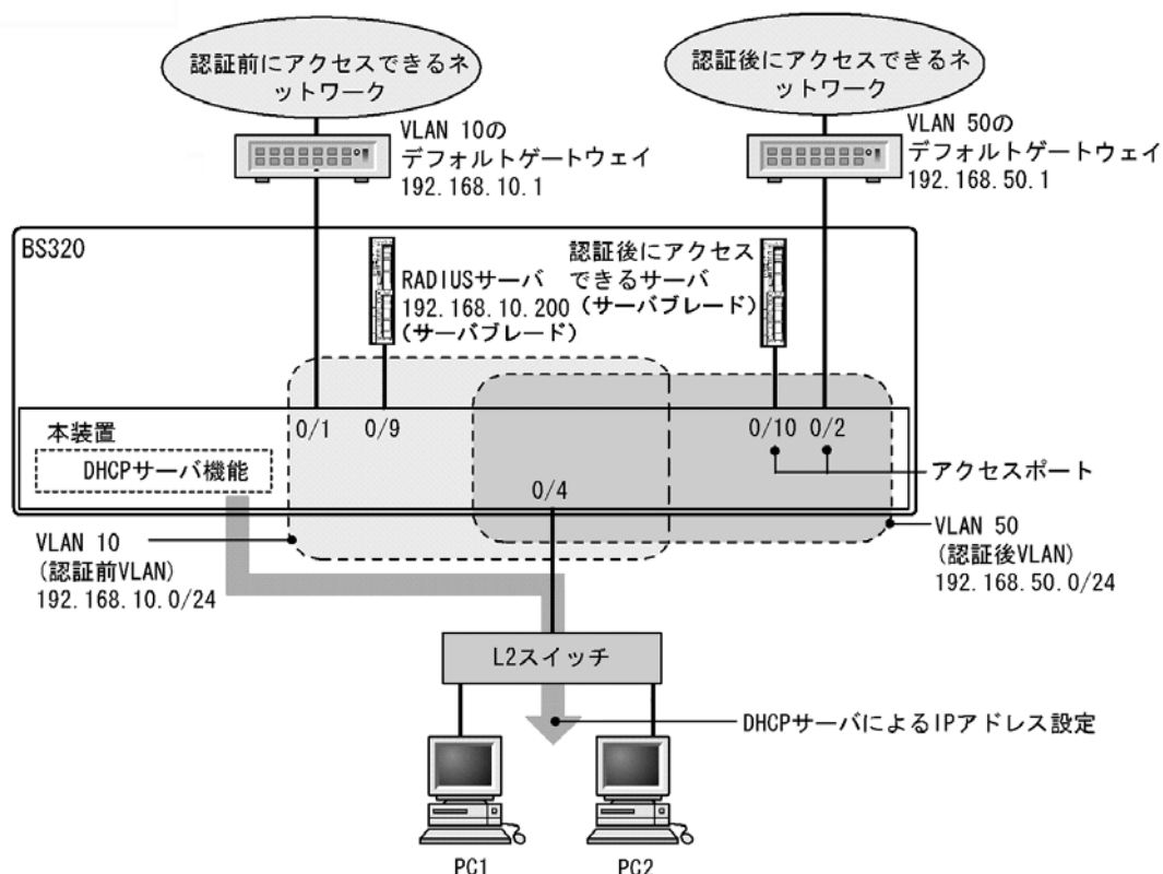
図 7-37 Web 認証の RADIUS 認証方式+内蔵 DHCP 使用時の構成例
