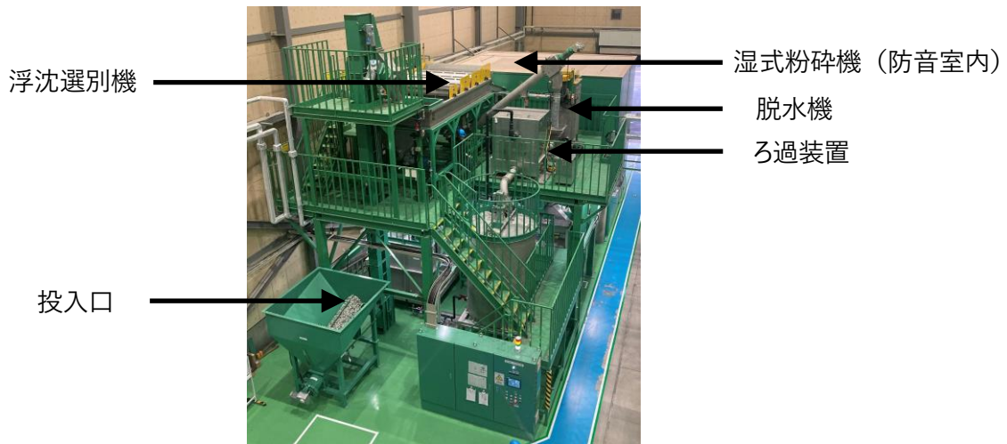
ミックスプラスチック選別装置
