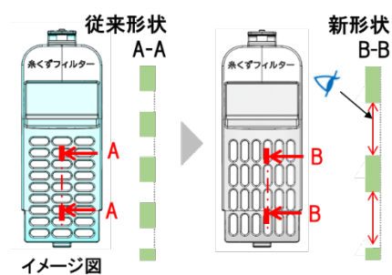
[図 6 糸くずフィルター開口形状]
