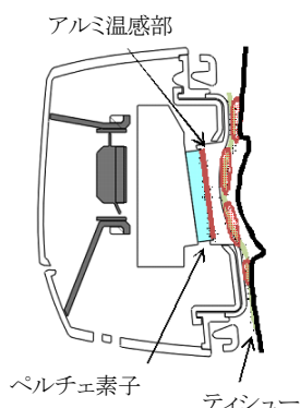
【図1 本体断面図】
