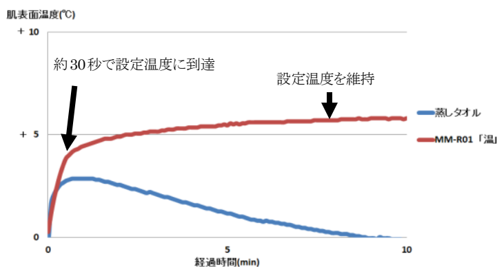
【図3 温度推移グラフ(温モード使用時)*2】
