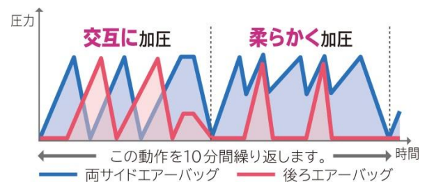
[ くつろぎモード動作イメージ (ふくらはぎ用) ]
