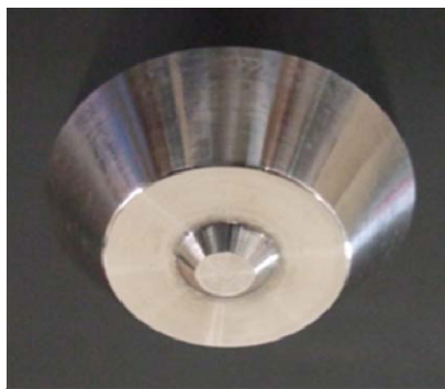
【写真】今回、開発した FSW ツールの先端部分
